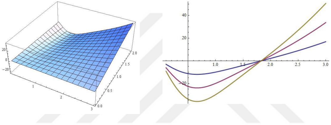
Şekil 4.5. \kappa(s, t) evölüsyonu
