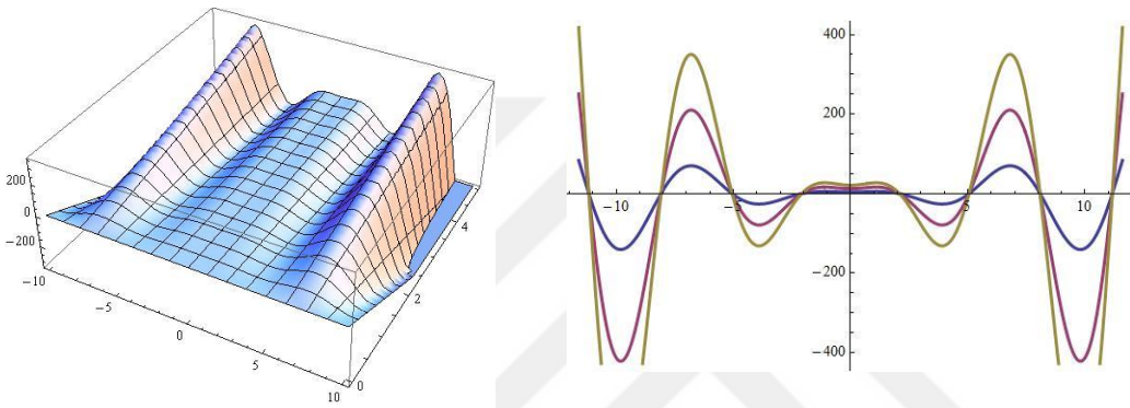
Şekil 4.2. k(s, t) evölüsyonu
