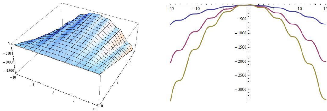
Şekil 4.1. \kappa(s, t) evölüsyonu
