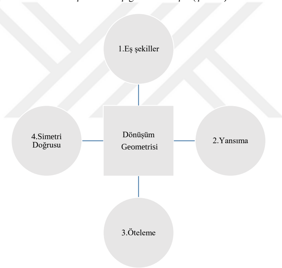
Şekil 2. Dönüşüm geometrisi kavramları şeması
