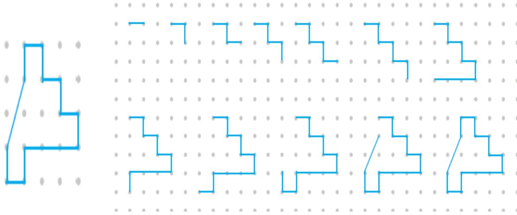
Şekil 3. Eş şekil oluşturma örneği
