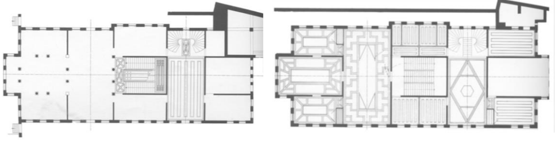
Şekil 5. 82: Esma Sultan Yalısı özgün zemin kat tavan planı (Eldem, 1993: 50)
