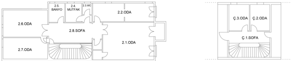
Şekil 5. 41: Sandalciyan Yalısı rekonstrüksiyon öncesi 2. kat plan düzeni Şekil 5. 42: Sandalciyan Yalısı rekonstrüksiyon öncesi çatı katı düzeni
