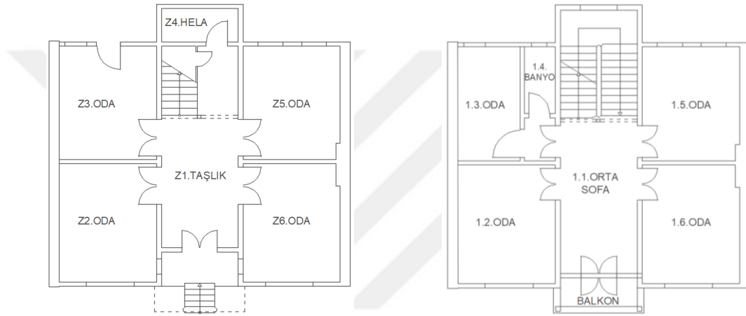
Şekil 5. 123: Dikranyan Yalısı özgün zemin kat planı (Restitüsyon raporları doğrultusunda çizilmiştir)
