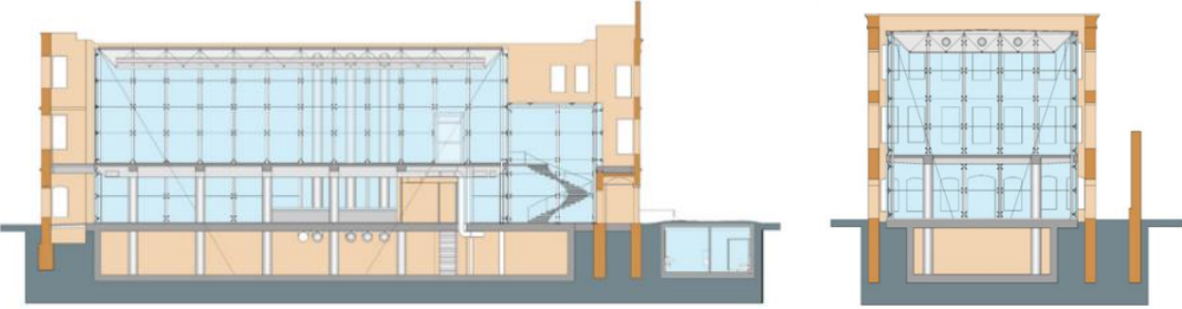
Şekil 5. 93: Esmâ Sultan Yalısı mevcut kuzey-güney yönü kesiti (URL 40)
