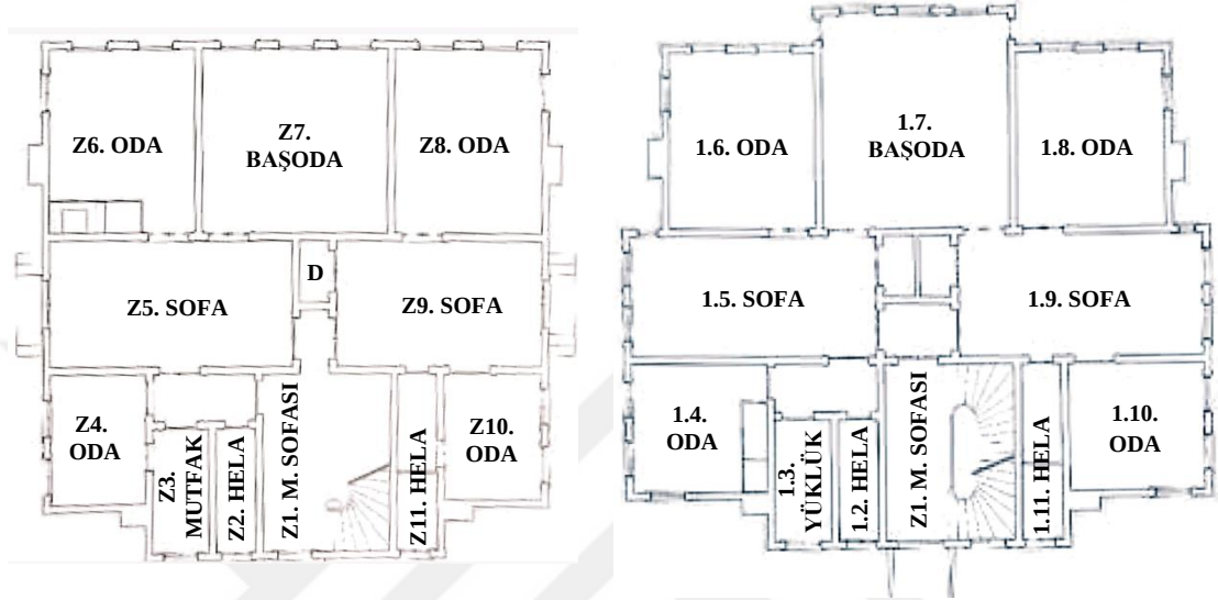
Şekil 5. 141: Baras Yalısı zemin kat restitüsyon çizimi (Öztek Mimarlık Arşivi)
