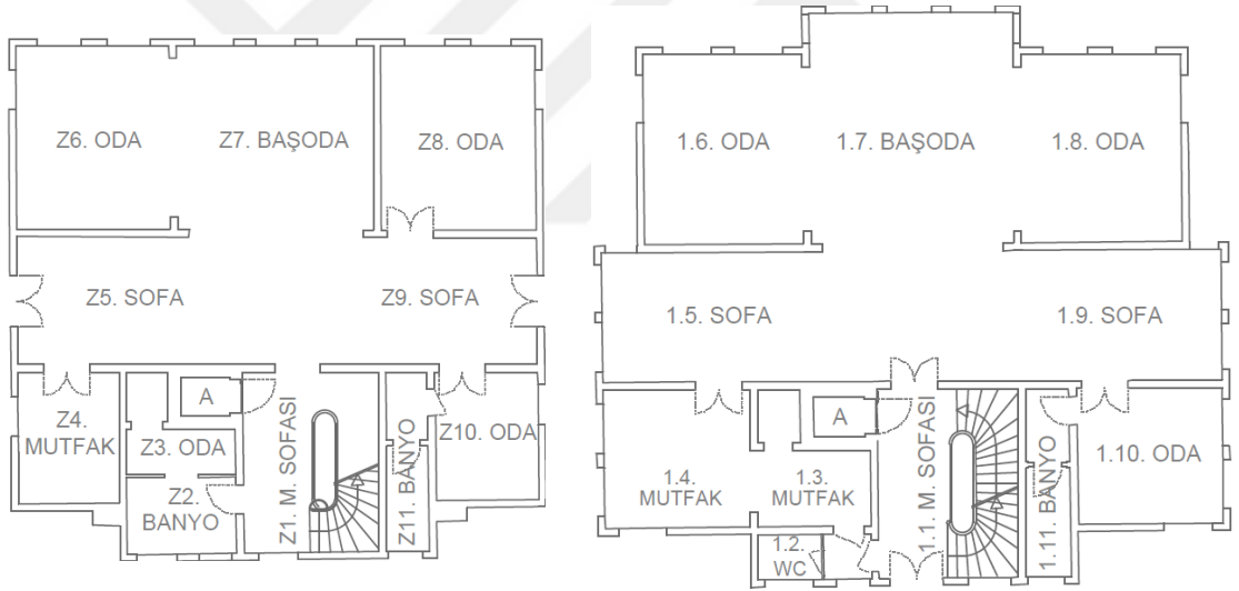
Şekil 5. 147: Baras Yalısı zemin kat restorasyon çizimi (Öztek Mimarlık Arşivi)
