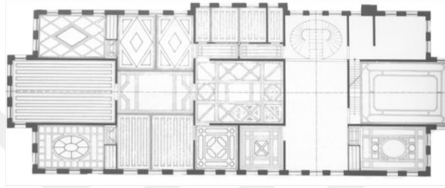
Şekil 5. 84: Esma Sultan Yalısı özgün 2. kat tavan planı (Eldem, 1993: 50)
