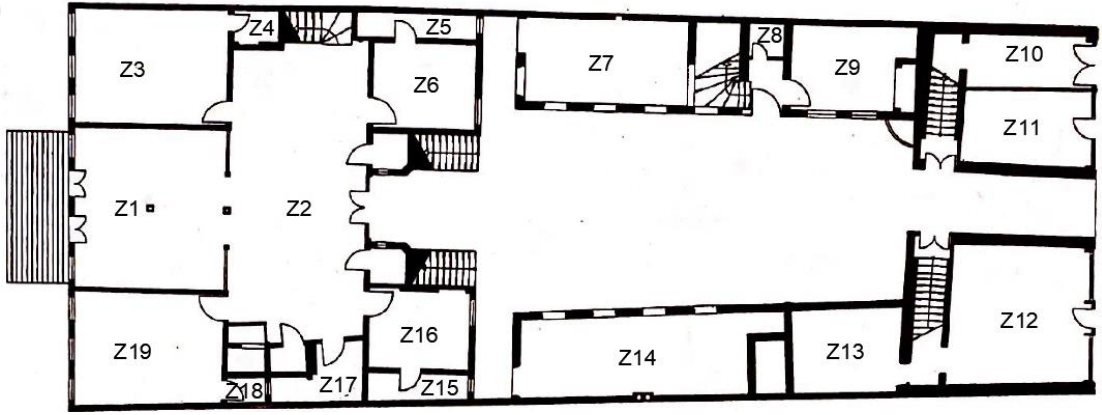
Şekil 5. 24: Fuad Paşa Yalısı rekonstrüksiyon öncesi zemin kat plan çizimi (Erdenen, 2006: 81)
