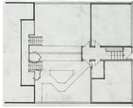
Şekil 5. 105: Faik Bey ve Bekir Bey Yalıları müştemilatı (Özgül, 2019)
