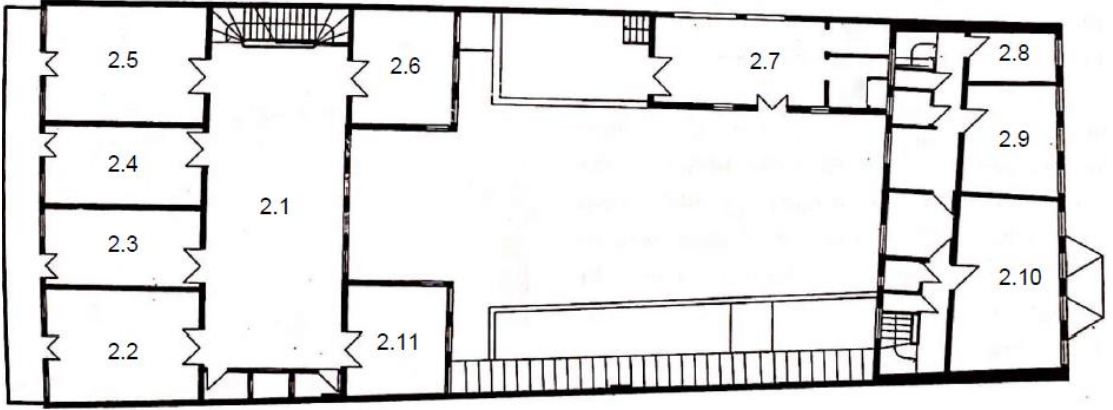
Şekil 5. 26: Fuad Paşa Yalısı rekonstrüksiyon öncesi 2. kat planı (Erdenen, 2006: 81)
