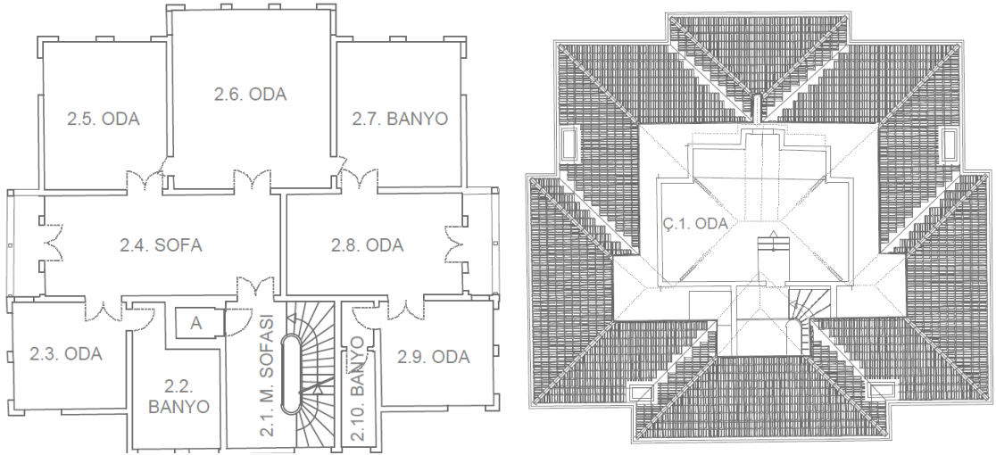
Şekil 5. 149: Baras Yalısı 2. kat restorasyon çizimi (Öztek Mimarlık Arşivi)
