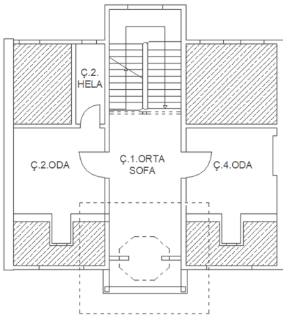
Şekil 5. 125: Dikranyan Yalısı özgün 2. kat planı (Restitüsyon raporları doğrultusunda çizilmiştir)
