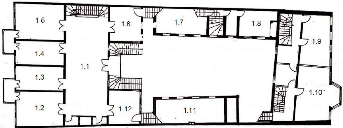
Şekil 5. 25: Fuad Paşa Yalısı rekonstrüksiyon öncesi 1. kat planı (Erdenen, 2006: 81)
