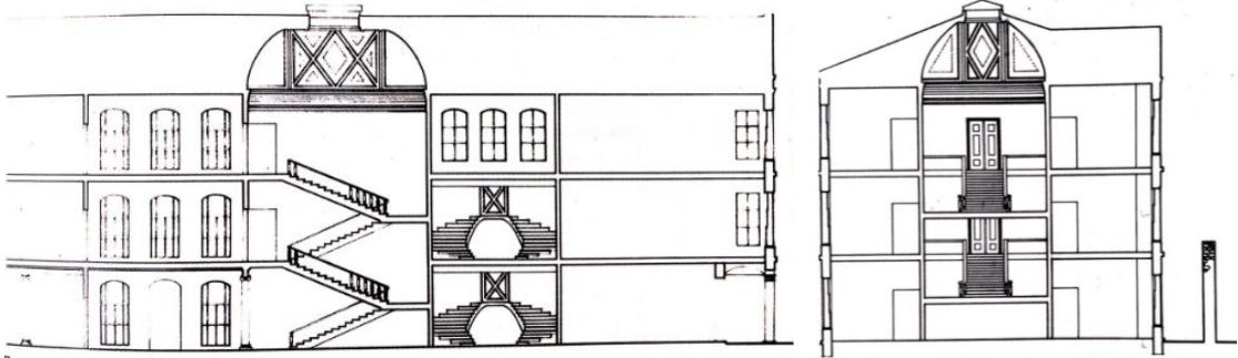
Şekil 5. 85: Esma Sultan Yalısı özgün kuzey-güney yönü kesiti (Erdenen, 2006: 427)
