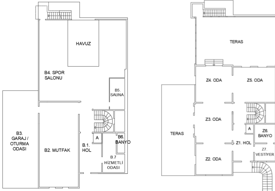
Şekil 5. 13: Kalkavan Yalısı bodrum kat planı (Rekonstrüksiyon sonrası plana göre çizilmiştir)
