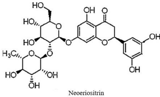
Şekil 2.4. Neoeriositrinin kimyasal yapısı
