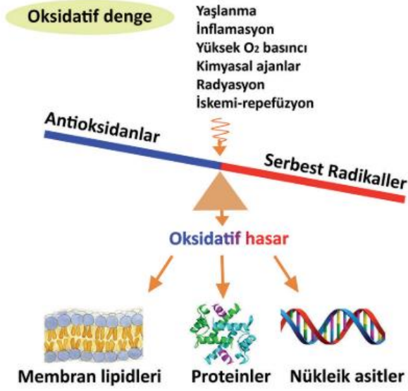
Şekil 2.1. Hücre içi oksidan-antioksidan dengesi [26]
