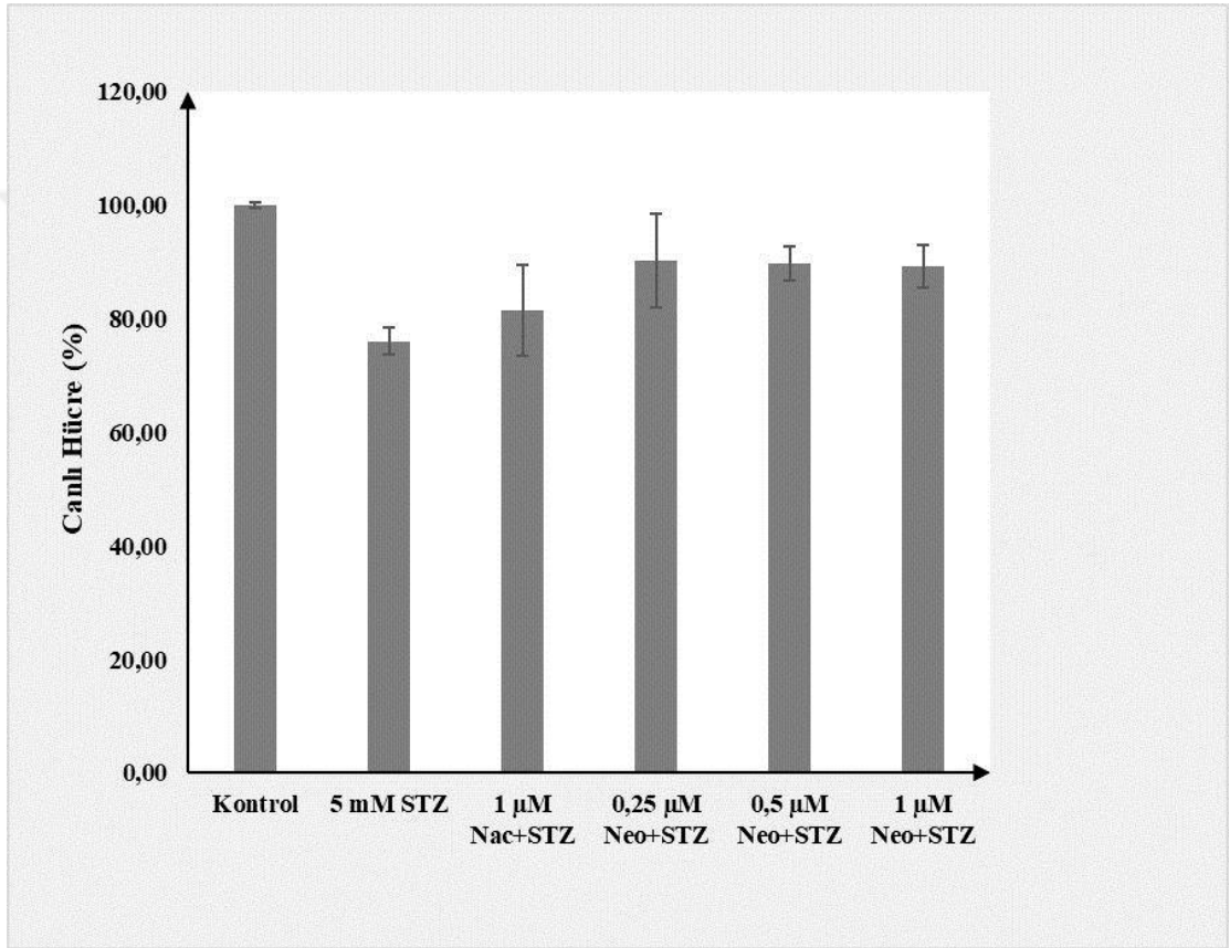
Şekil 4.5. INS-1E pankreas hücrelerinde tripan mavisi boyama testi ile hücre canlılık sonuçları.
