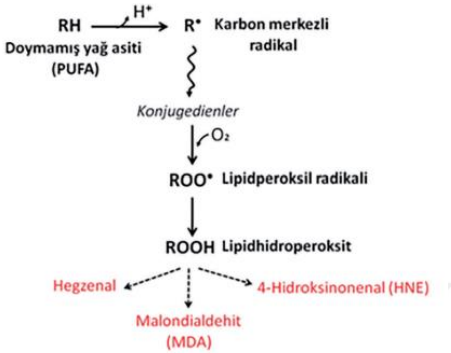
Şekil 2.8. Lipid peroksidasyon testi [26]
