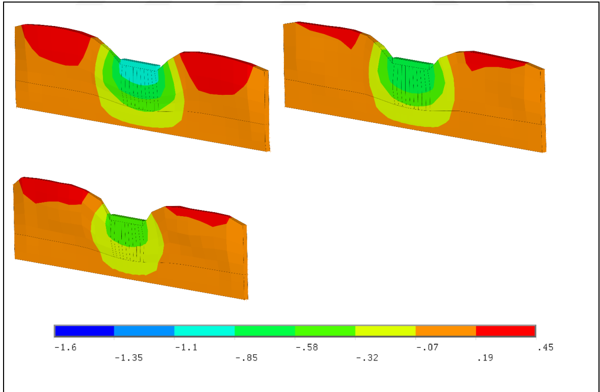
Şekil 7.8. A-A kesiti toplam yer değiştirme değerleri (m) a) Kobe b) İzmit c) El Centro
