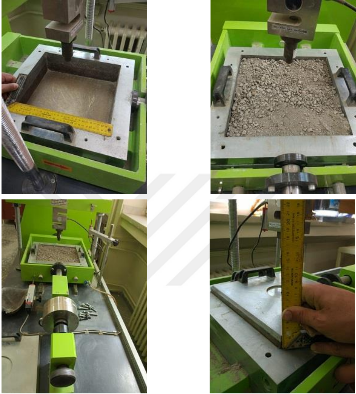
Resim 6.2. Büyük ölçekli kesme deneyi için ölçülerin alınması ve deney numunesinin hazırlanması
