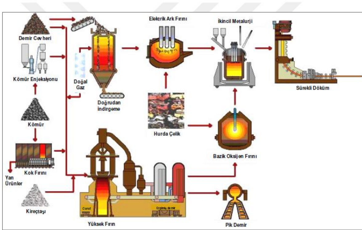
Şekil 4.2. Demir-çelik üretimi akış şeması [44]
