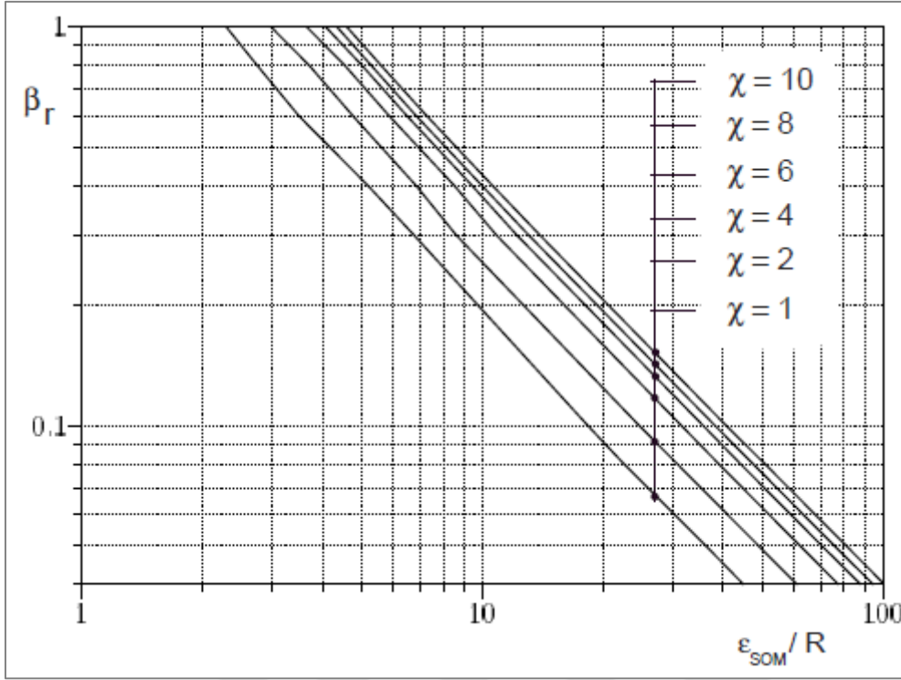
Şekil 5.12. Farklı \chi değerleri için \beta_r vs. \epsilon_{SOM}/R korelasyonu [64]
