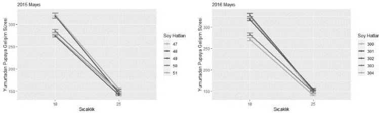
Şekil 4.10. 2015 ve 2016 yıllarına ait Mayıs ayı soy hatlarının 18°C ve 25°C'deki yumurtadan pupaya gelişim sürelerine ait reaksiyon normları.
