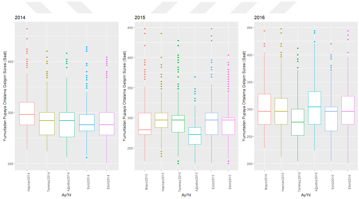
Şekil 4.1. 18°C'de yumurtadan pupaya ortalama gelişim süresinin yıllara göre standart hata çubuklarıyla gösterimi.
