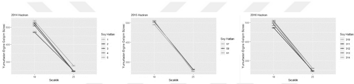
Şekil 4.23. 2014, 2015 ve 2016 yıllarına ait Haziran ayı soy hatlarının 18°C ve 25°C'deki yumurtadan ergine gelişim sürelerinin reaksiyon normları.
