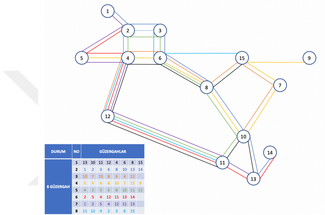
Şekil 4.3: ToTaRO modeli ile Mandl ağında elde edilmiş en iyi rota kümesi.
