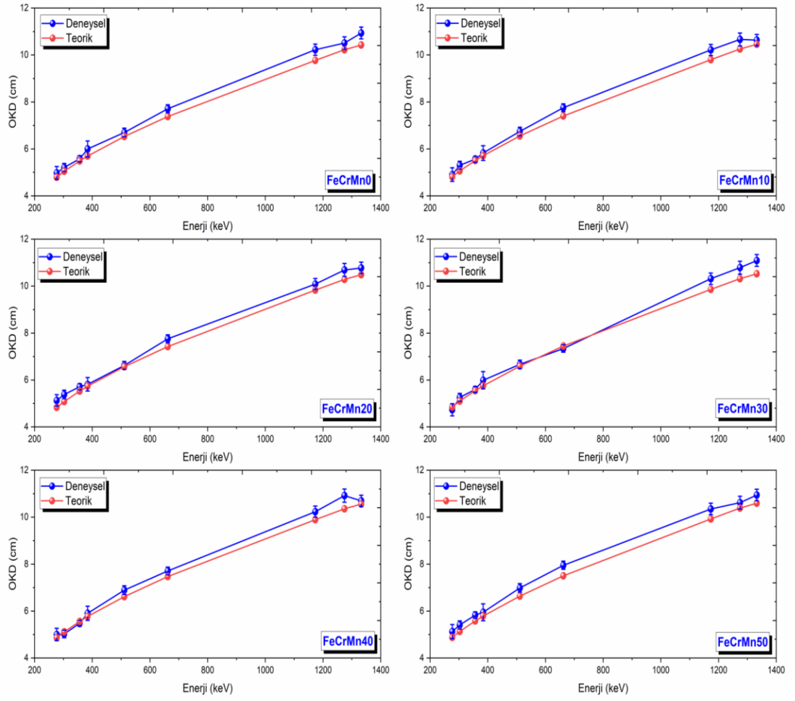
Şekil 5.17. FeCrMn kodlu üçlü kompozitlere ait onda-bir kalınlık değeri sonuçlarının enerji ile değişimi
