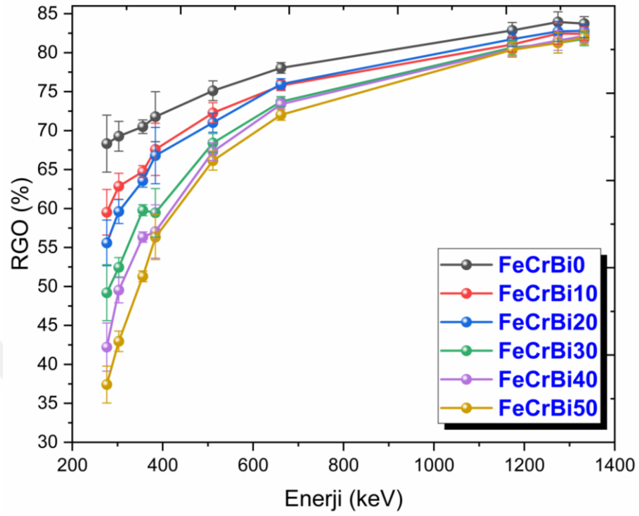
Şekil 5.4. FeCrBi kodlu üçlü kompozitlere ait radyasyon geçirir oranı sonuçlarının enerji ile değişimi
