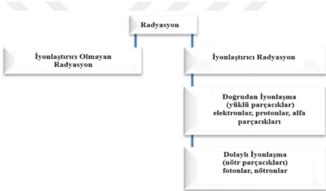
Şekil 3.1. Radyasyonun sınıflandırılması
