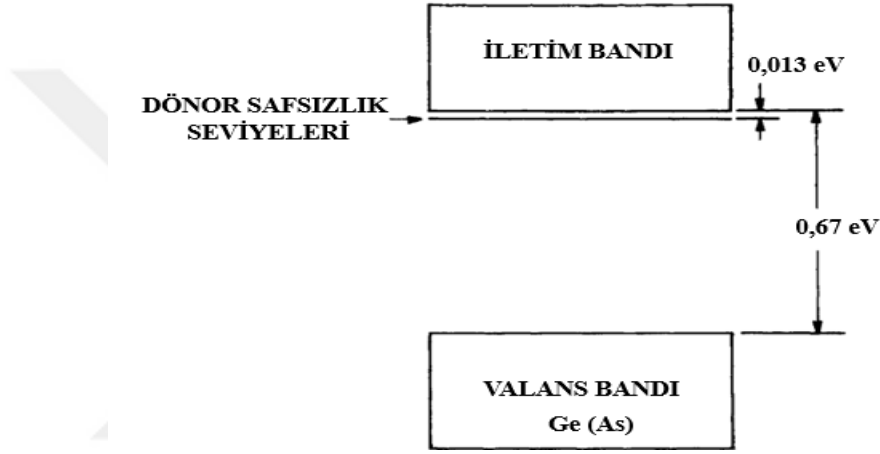
Şekil 3.19. Arsenik (As) dönör atomları içeren germanyum (Ge) kristali için enerji seviyesi diyagramı
