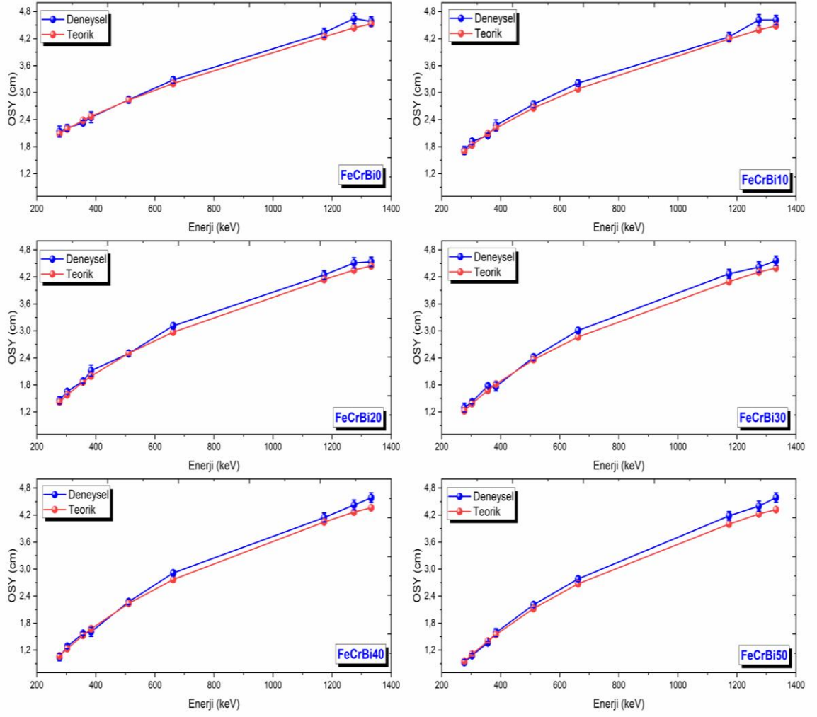
Şekil 5.19. FeCrBi kodlu üçlü kompozitlere ait ortalama serbest yol sonuçlarının enerji ile değişimi
