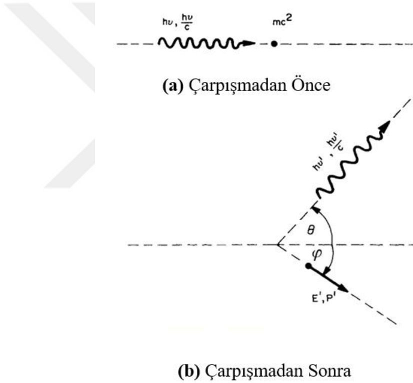
Şekil 3.5. Compton saçılmasının (a) çarpışmadan önceki ve (b) çarpışmadan sonraki gösterimi
