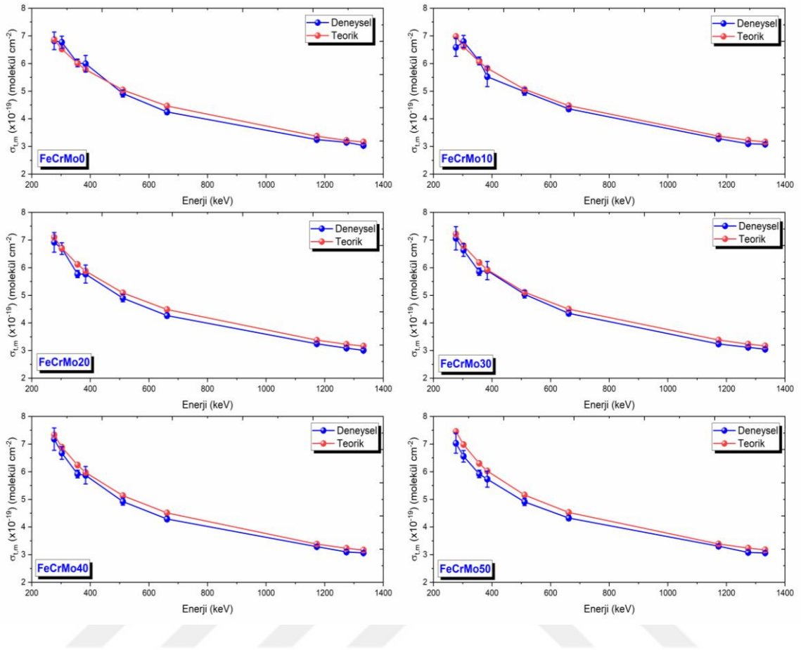
Şekil 5.24. FeCrMo kodlu üçlü kompozitlere ait moleküler tesir kesiti sonuçlarının enerji ile değişimi
