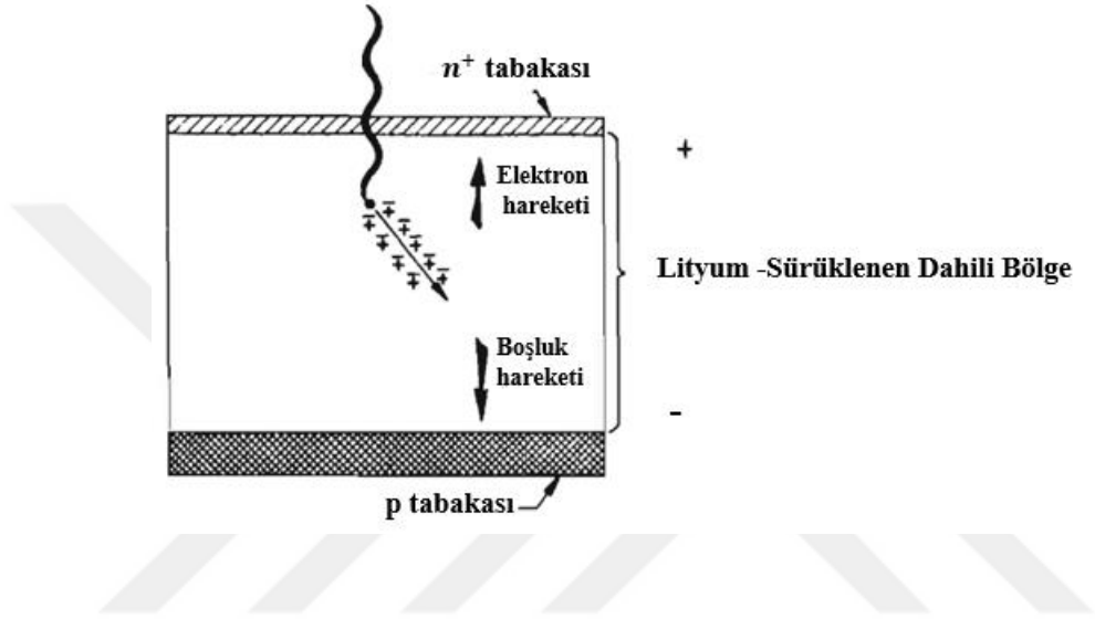
Şekil 3.23. Bir Ge (Li) detektörünün işleyişinin gösterimi
