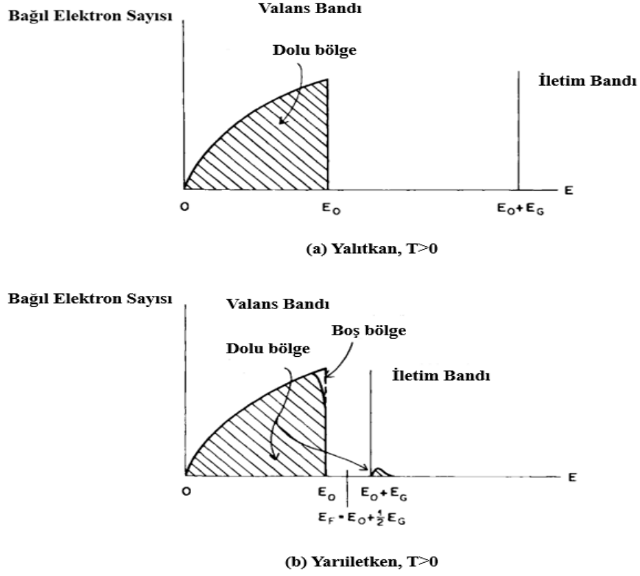
Şekil 3.16. Valans ve iletkenlik bantlarının bağlı elektron sayısı (a) Yalıtkan T > 0 ve (b) Yarıiletken T > 0
