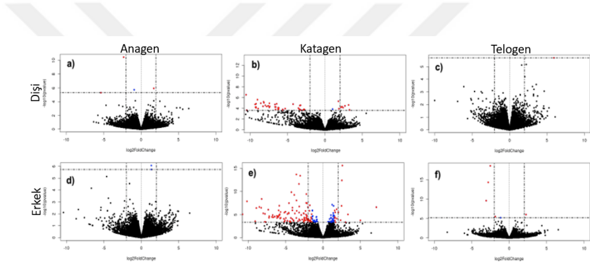
Şekil 4.6 Eskişehir ve Lalahan Ankara keçisi varyetelerinin dişi-dişi ve erkek-erkek gruplarının her bir faz için karşılaştırılması sonucu elde edilen DEG’lere ait volcano plot görüntüleri (a) Eskişehir ve Lalahan varyetesindeki dişi keçilerin anagen fazı bakımından karşılaştırılması sonucu elde edilen volcano plot, (b) Eskişehir ve Lalahan varyetesindeki dişi keçilerin katagen fazı bakımından karşılaştırılması sonucu elde edilen volcano plot, (c) Eskişehir ve Lalahan varyetesindeki dişi keçilerin telogen fazı bakımından karşılaştırılması sonucu elde edilen volcano plot, (d) Eskişehir ve Lalahan varyetesindeki erkek keçilerin anagen fazı bakımından karşılaştırılması sonucu elde edilen volcano plot, (e) Eskişehir ve Lalahan varyetesindeki erkek keçilerin katagen fazı bakımından karşılaştırılması sonucu elde edilen volcano plot, (f) Eskişehir ve Lalahan varyetesindeki erkek keçilerin telogen fazı bakımından karşılaştırılması sonucu elde edilen volcano plot
