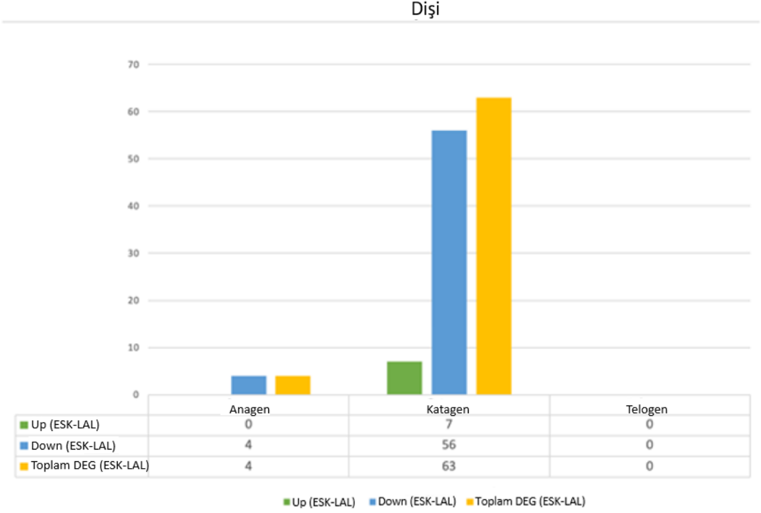
Şekil 4.7 Eskişehir ve Lalahan varyetesindeki dişilerin birbiriyle dişilerde anagen, katagen ve telogen fazı bakımından ayrı ayrı karşılaştırılması sonucu elde edilen DEG'lerin sayısını gösteren sütun grafiği ('ESK' Eskişehir varyetesini, 'LAL' Lalahan varyetesini ifade etmektedir.)
