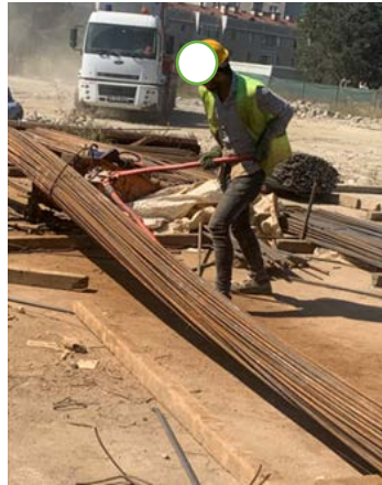
Şekil 13. Sabitlenmiş demir makası ile demirlerin bağ tellerinin kesilmesi
