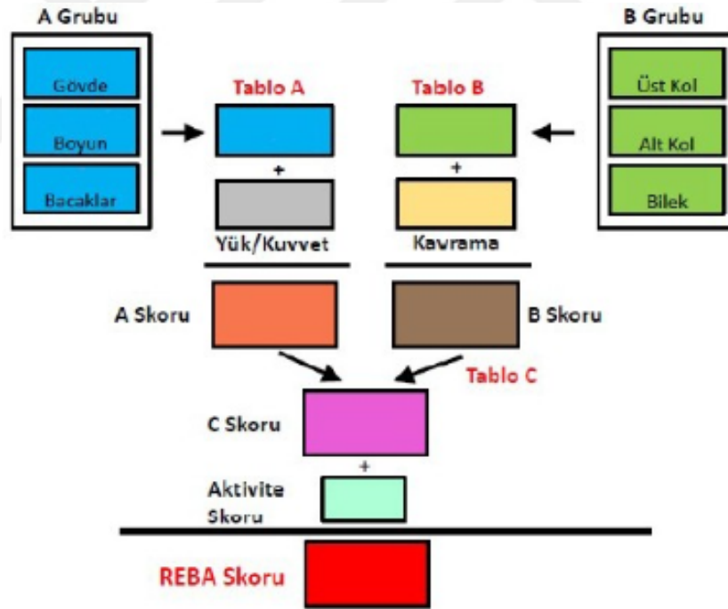
Şekil 8. Reba skoru
