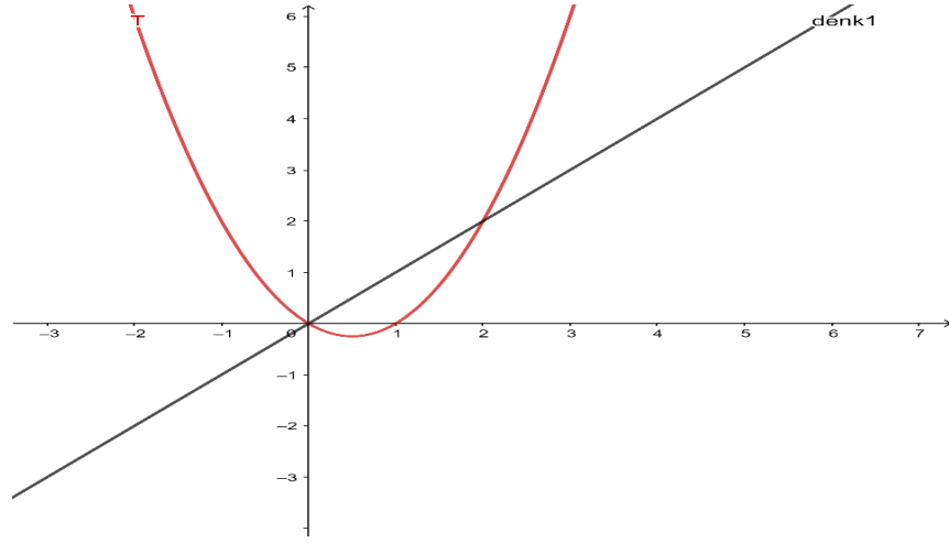
Şekil 1.1. T(\mu) = \mu^2 - \mu fonksiyonunun sabit noktalarının grafiği
