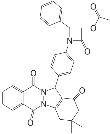
Şekil 3.1. 1-(4-(3,3-dimetil-1,6-dioxo-2,3,4,6,11,13-hekzahidro-1H-indazolo[1,2-b]ftalazin-13-yl)fenil)-2-fenilazetidin-3-yl asetat'ın kimyasal yapısı
