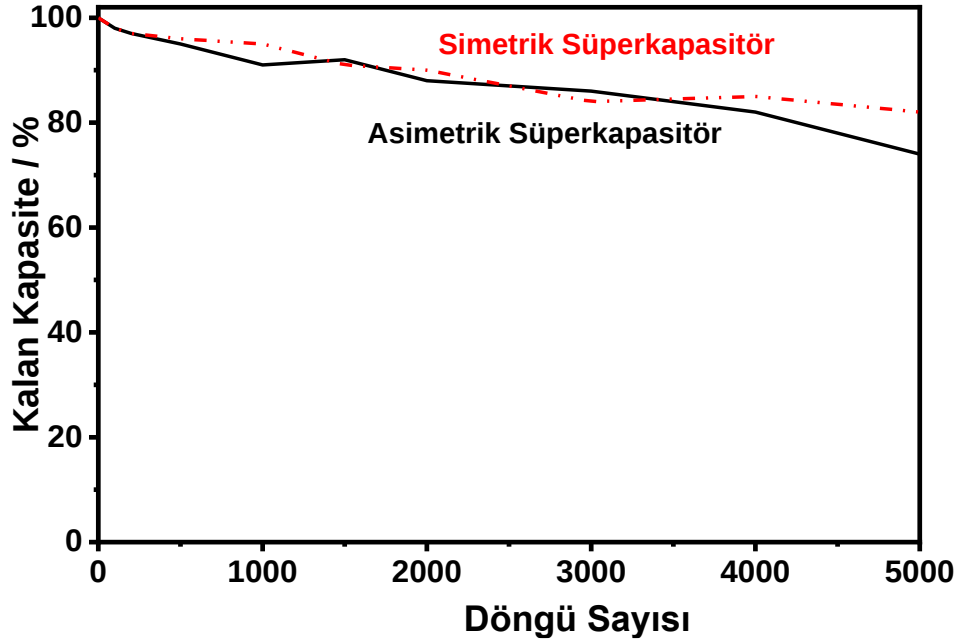
Şekil 4.24. V-int.GK/PPy/VO x /CMC elektrodu ( 10.0 mg cm -2 kütle yüklemesinde) kullanılarak hazırlanan hücre konfigürasyonları için 100 mM HBF 4 /TBABF 4 içeren asetonitril/adiponitril içinde akım yoğunluğunda simetrik ve asimetrik süperkapasitörün döngü kararlılığı ( 2.5Ag -1 ).
