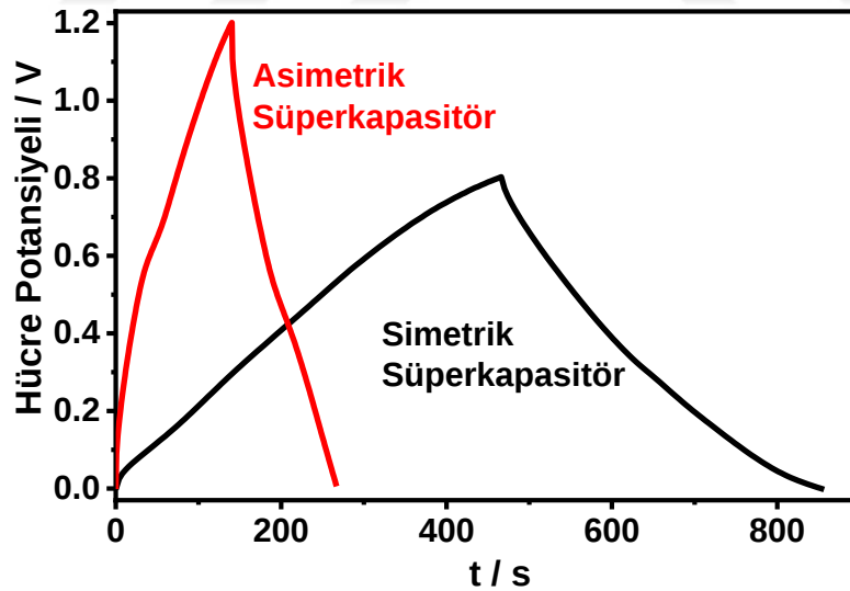
Şekil 4.20. Pb-int.GK/PPy/PbO x /CMC elektrodunun ( 10 mg cm -2 kütle yüklemesinde, 0.2 cm 2 ) iki hücre konfigürasyonu için PVA/H 2 SO 4 jel elektroliti içinde hücre voltajlarının zamana göre değişimi ( 0.5 A g -1 ).
