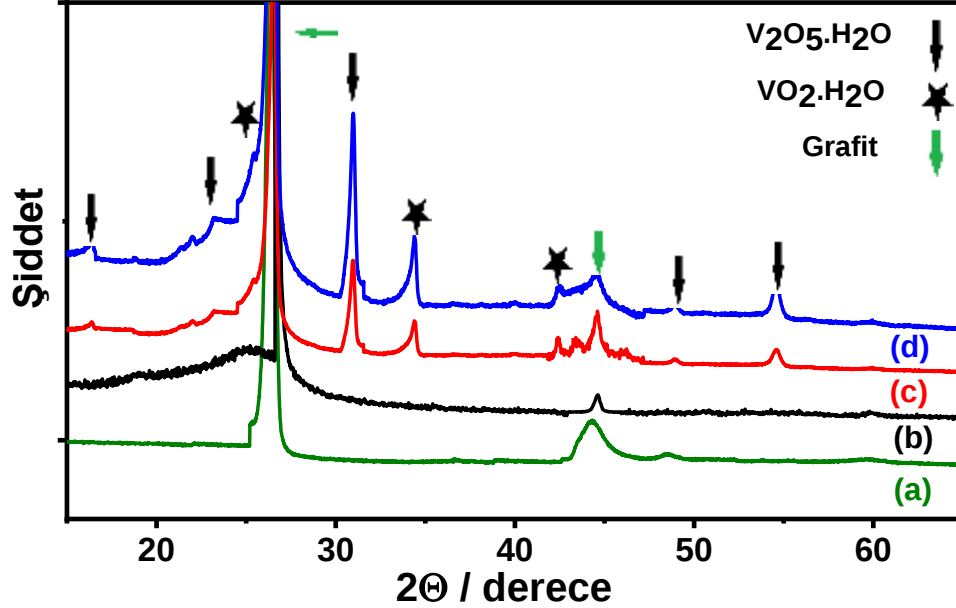
Şekil 20. PPy/VO x /CMC kaplamanın XRD ile karakterizasyonu: (a) Kaplanmamış grafit levha elektrodun: grafit levha yüzeyinde (b) PPy ve (c) PPy/VO x /CMC kaplamaların, (d) V-int.grafit levha/PPy/VO x /CMC kompozitinin XRD spektrumları.
