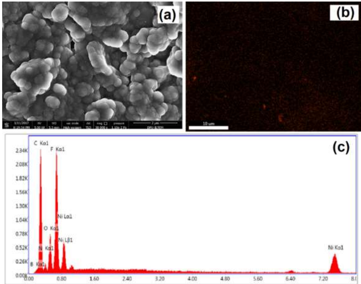
Şekil 34. Ni-int.KG yüzeyindeki PPy/NiO x /CMC kaplamanın (a) SEM görüntüsü, (b) Ni-EDX haritalaması ve (c) EDX alan spektrumu
