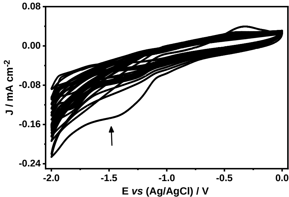
Şekil 6. Grafit Elektrodun Gümüş ile İnterkalasyonu: Polimerizasyon çözeltisinde 0.0 \text{ V} ve -2.0 \text{ V} arasında 50 döngü tarama ile KG yüzeyinin interkalasyonu esnasında kaydedilen çok döngülü voltamogram, v=100 \text{ mV s}^{-1} . (Sentez çözeltisi: C_{\text{Py}} = 125 \text{ mM} , C_{\text{TBABF}_4} = 125 \text{ mM} , C_{\text{HBF}_4} = 125 \text{ mM} , C_{\text{Ag}(\text{BF}_4)_2} = 50 \text{ mM} , C_{\text{CMC}} = 0.5 \text{ mg mL}^{-1} , C_{\text{H}_2\text{O}} = 50 \text{ mM} )
