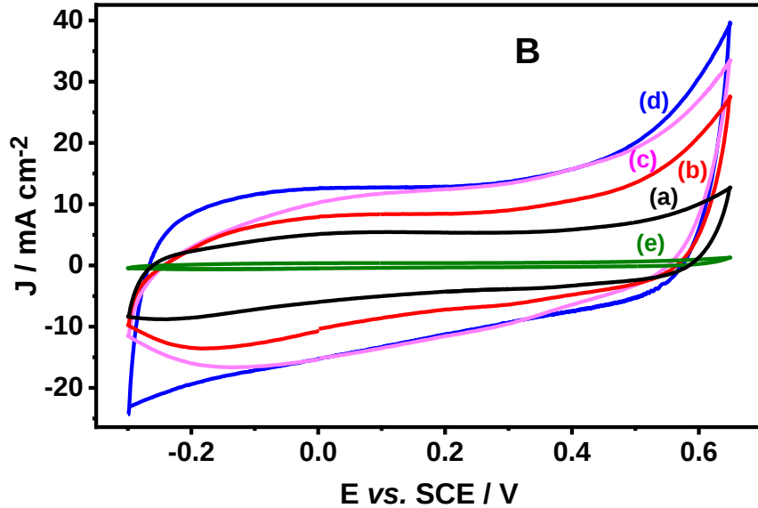
Şekil 4.2.B. Şekil 4.2.A da gösterilen sırasıyla (a-d) kaplamaların (0.19 mg cm -2 kütle yüklemesinde) ve (e) kaplanmamış KG nin 100 mM \text{H}_2\text{SO}_4 çözeltisinde alınan dönüşümlü voltamogramları, v = 100 mV s -1 .
