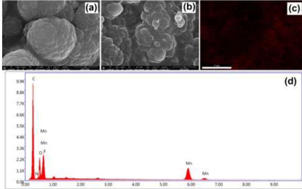
Şekil 4.13. (a) KG yüzeyinde PPy; Mn-int.KG yüzeyinde PPy/MnO x /CMC kaplamanın (b) SEM görüntüsü (c) Mn-EDX haritalaması (d) EDX alan spektrumu.
