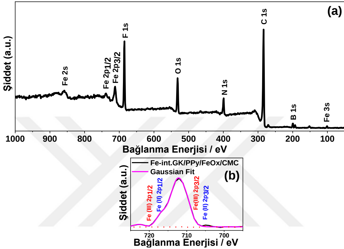
Şekil 28. PPy/FeO x /CMC kaplamanın XPS ile karakterizasyonu: Fe-int.GK yüzeyindeki PPy/FeO x /CMC kaplamanın (a) tam taraması (b) Fe 2p kısmi taraması.
