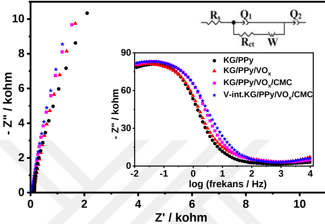
Şekil 4.7. KG/PPy, KG/PPy/VO x , KG/PPy/VO x /CMC ve V-int.KG/PPy/VO x /CMC (0.19 mg cm -2 kütle yüklemesinde) elektrotlarının 100 mM H 2 SO 4 çözeltisinde kaydedilen Nyquist eğrileri (Bode eğrileri ve eşdeğer devre ( R_s(Q_1(R_{ct}W))Q_2 ) şekil içinde verilmiştir).
