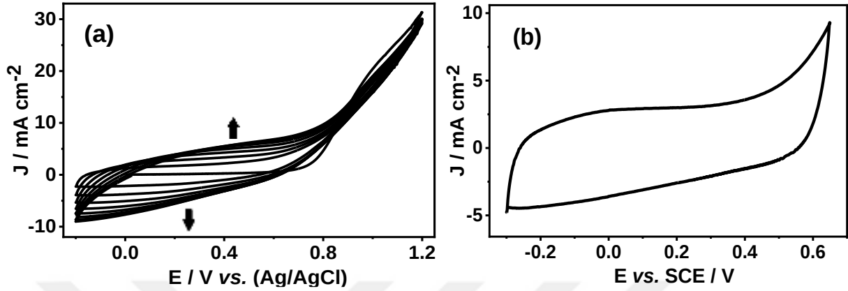
Şekil 4.1.(a) Py, TBABF 4 , HBF 4 , H 2 O ve VO(BF 4 ) 2 içeren asetonitril çözeltisinde KG yüzeyine PPY/VO x kompozitin sentezi boyunca kaydedilen çok döngülü voltamogram, (b) Şekil 4.1.(a) deki bu kaplamanın (0.19 mg cm -2 kütle yüklemesinde) 100 mM H 2 SO 4 çözeltisinde elde edilen dönüşümlü voltamogramı, \nu = 100 \text{ mV s}^{-1} .
