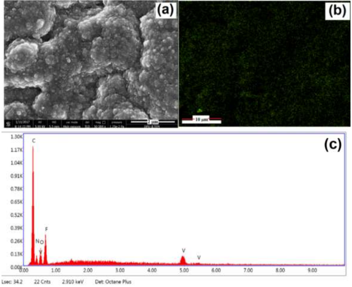
Şekil 32. V-int.KG yüzeyindeki PPy/VO x /CMC kaplamanın (a) SEM görüntüsü, (b) V-EDX haritalaması ve (c) EDX alan spektrumu
