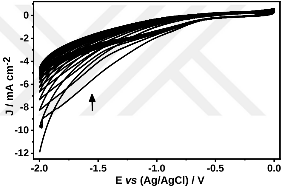
Şekil 4.4. Sentez çözeltisinde 0.0 V ve -2.0 V arasında 50 döngü tarama ile KG yüzeyinin interkalasyonu esnasında kaydedilen çok döngülü voltamogram, v=100 \text{ mV s}^{-1} . (Sentez çözeltisi: c_{Py} = 25 \text{ mM} , c_{TBABF_4} = 25 \text{ mM} , c_{HBF_4} = 25 \text{ mM} , c_{VO(BF_4)_2} = 10 \text{ mM} , c_{CMC} = 0.5 \text{ mg mL}^{-1} , c_{H_2O} = 100 \text{ mM} ).
