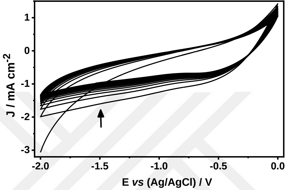
Şekil 2. Grafit Elektrodun Kurşun ile İnterkalasyonu: Polimerizasyon çözeltisinde 0.0 ve -2.0 V arasında 50 döngü tarama esnasında kaydedilen çok döngülü voltamogram, v=100 \text{ mV s}^{-1} . (Sentez çözeltisi: c_{\text{Py}} = 25 \text{ mM} , c_{\text{TBABF}_4} = 25 \text{ mM} , c_{\text{HBF}_4} = 25 \text{ mM} , c_{\text{Pb}(\text{BF}_4)_2} = 10 \text{ mM} , c_{\text{CMC}} = 0.5 \text{ mg mL}^{-1} , c_{\text{H}_2\text{O}} = 50 \text{ mM} )
