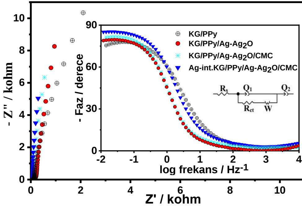
Şekil 8. KG/PPy/Ag-Ag 2 O/CMC sentezine katkılarının ve interkalasyonun etkisinin Elektrokimyasal Empedans Spektroskopisi ile incelenmesi: KG/PPy, KG/PPy/Ag-Ag 2 O, KG/PPy/Ag-Ag 2 O/CMC ve Ag-int.KG/PPy/Ag-Ag 2 O/CMC elektrotlarının (4.0 mg cm -2 kütle yüklemesinde) 100 mM H 2 SO 4 çözeltisinde kaydedilen Nyquist eğrileri. (Bode eğrileri ve eşdeğer devre (R s (Q 1 (R ct W))Q 2 ) şekil içinde gösterilmiştir).
