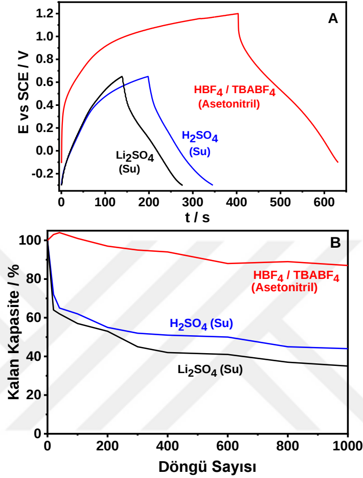
Şekil 4.16. V-int.KG/PPy/VO x /CMC elektrodun ( 0.19 \text{ mg cm}^{-2} kütle yüklemesinde) sulu 100 mM H 2 SO 4 ve 100 mM Li 2 SO 4 çözeltilerinde ve 100 mM HBF 4 /TBABF 4 asetonitril çözeltilisinde (A) 1 \text{ mA cm}^{-2} kaydedilen galvanostatik şarj-deşarj eğrileri ve (B) döngü ömürleri ( 15 \text{ mA cm}^{-2} de) ( A_{\text{KG}} = 0.0244 \text{ cm}^2 ).
