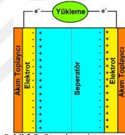
Şekil 2.2. Süperkapasitörün şematik gösterimi
