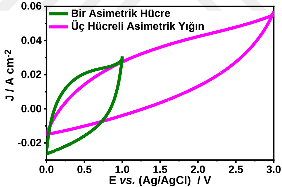
Şekil 4.39. 1.0 \text{ cm}^2 ( 1 \text{ cm} \times 1 \text{ cm} ) lik Pb-int.GK/PPy/PbO x /CMC ( 10.0 \text{ mg cm}^{-2} ) elektrotları kullanılarak hazırlanan bir hücre ve üç hücreli asimetrik yığının PVA:H 2 SO 4 jel elektrolit çözeltisinde alınan dönüşümlü voltamogramları, v = 10 \text{ mV s}^{-1} .
