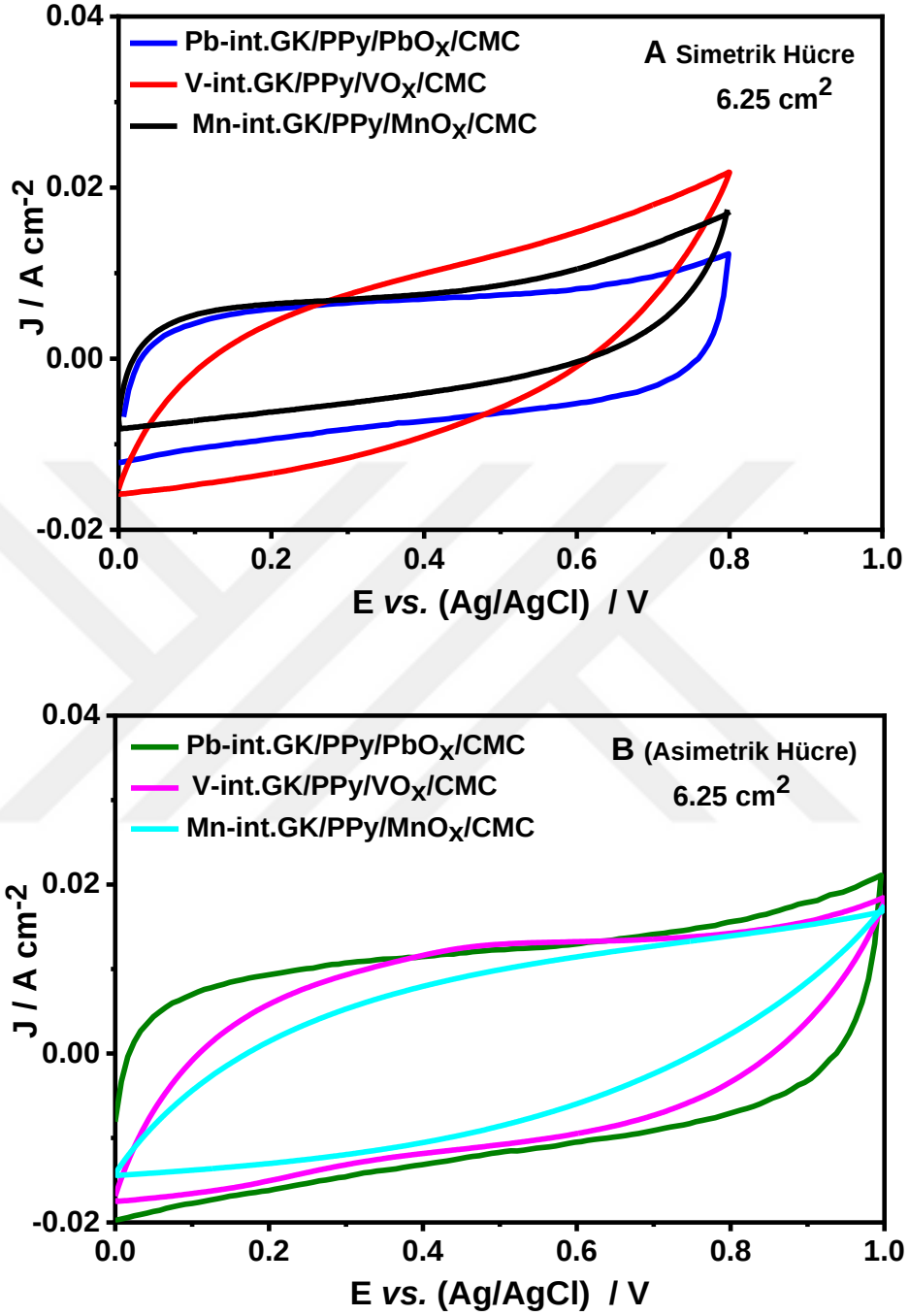
Şekil 4.32. 6.25 cm 2 (2.5 cm x 2.5 cm) lik kendi metalleri ile int.GK yüzeylerindeki PPy/MO x /CMC (10.0 mg cm -2 ) kompozit kaplanmış elektrotlar kullanılarak hazırlanan A. simetrik, B. asimetrik hücrelerin PVA:H 2 SO 4 jel elektrolit çözeltisinde alınan dönüşümlü voltamogramları, v = 10 \text{ mV s}^{-1} (M: metal).
