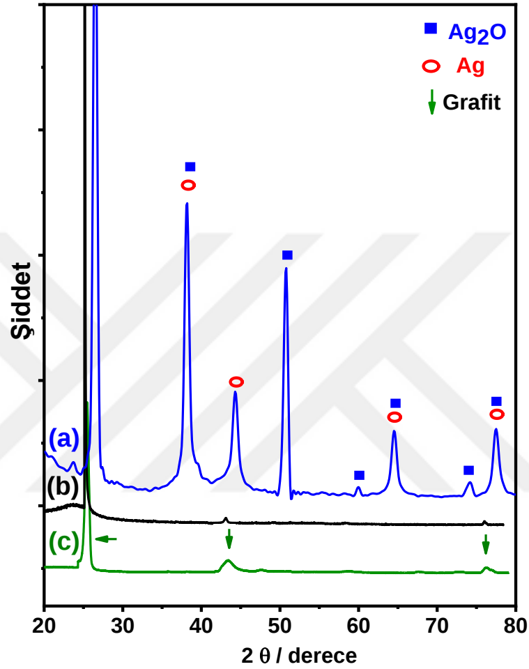
Şekil 22. PPy/Ag-Ag 2 O/CMC kaplamanın XRD ile karakterizasyonu: (a) Kaplanmamış grafit levha elektrodun, (b) grafit levha/PPy ve (c) Ag-int.grafit levha/PPy/Ag-Ag 2 O/CMC kaplamaların XRD spektrumları.
