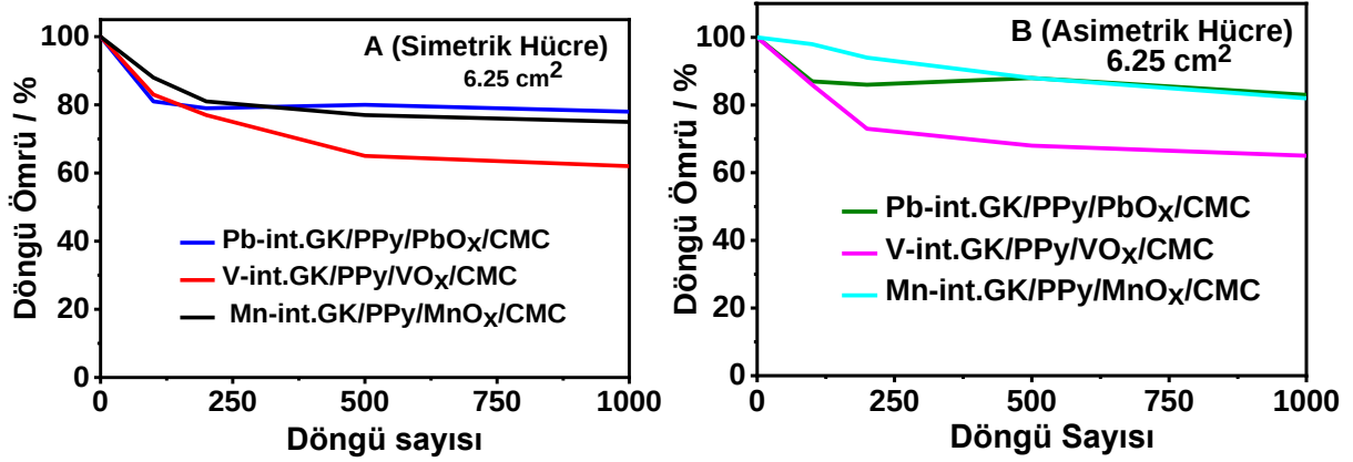
Şekil 4.36. 6.25 cm 2 (2.5 cm x 2.5 cm) lik kendi metalleri ile int. GK yüzeyindeki PPy/MO x /CMC (10.0 mg cm -2 ) kompozit kaplanmış elektrotlar kullanılarak hazırlanan A. simetrik, B. asimetrik hücrelerin PVA:H 2 SO 4 jel elektrolit çözeltisinde 2.0 A g -1 akım yoğunluğunda elde edilen galvanostatik şarj-deşarj eğrilerinden hesaplanan döngü ömürleri (M: metal)
