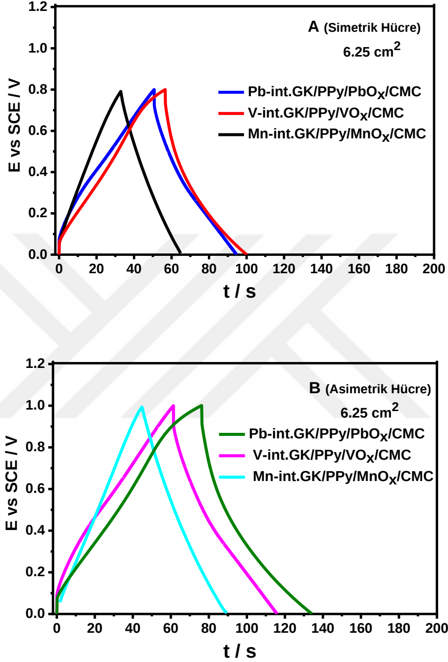
Şekil 4.34. 6.25 cm 2 (2.5 cm x 2.5 cm) lik kendi metalleri ile int. GK yüzeyindeki PPy/MO x /CMC (10.0 mg cm -2 ) kompozit kaplanmış elektrotlar kullanılarak hazırlanan A. simetrik, B. asimetrik hücrelerin PVA:H 2 SO 4 jel elektrolit çözeltisinde 2.0 A g -1 akım yoğunluğunda elde edilen galvanostatik şarj-deşarj eğrileri (M: metal)
