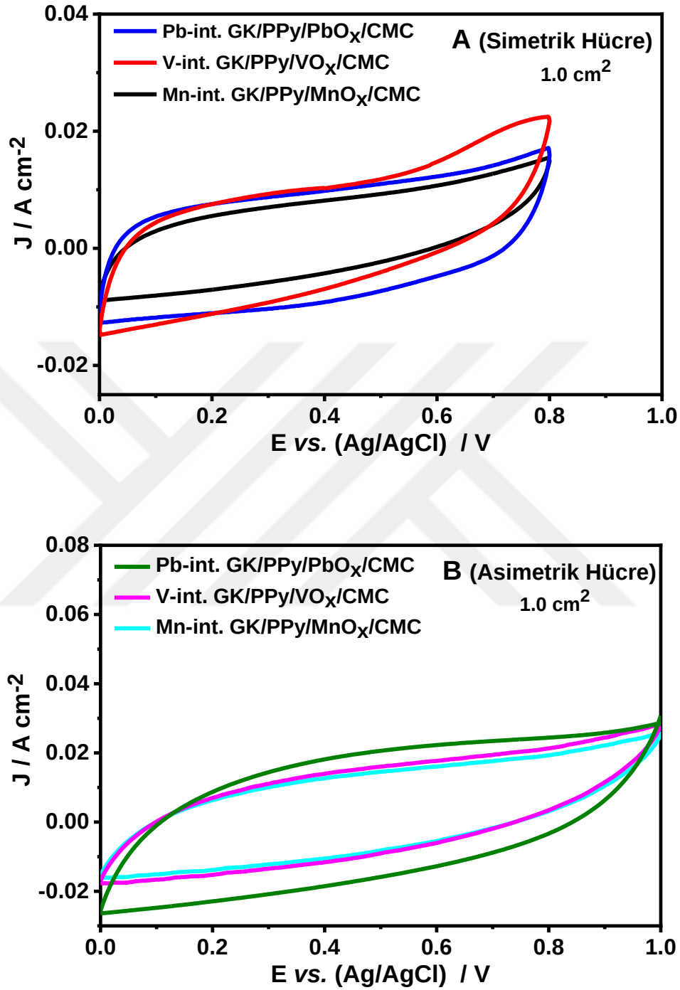
Şekil 4.31. 1 cm 2 (1 cm x 1 cm) lik kendi metalleri ile int. GK yüzeylerindeki PPy/MO x /CMC (10.0 mg cm -2 ) kompozit kaplanmış elektrotlar kullanılarak hazırlanan A. simetrik, B. asimetrik hücrelerin PVA:H 2 SO 4 jel elektrolit çözeltisinde alınan dönüşümlü voltamogramları, v = 10 \text{ mV s}^{-1} (M: metal).
