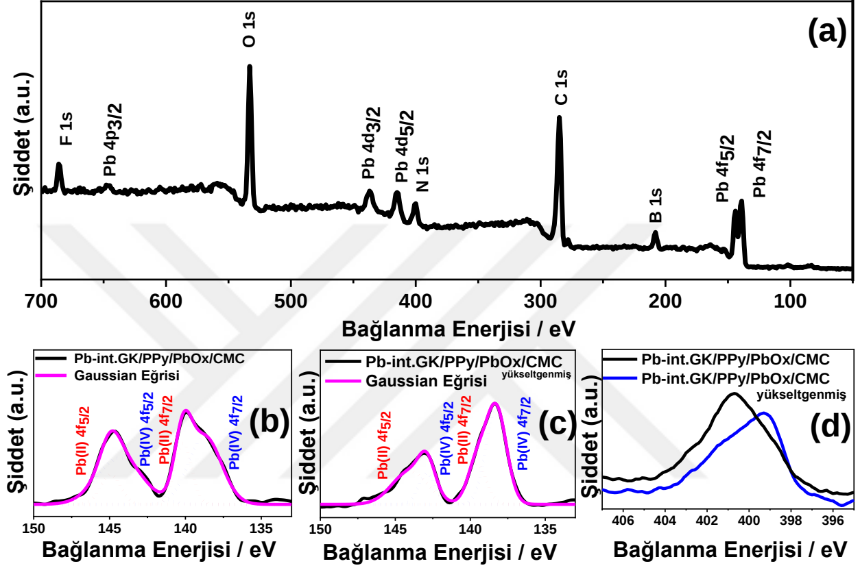
Şekil 24. PPy/PbO x /CMC kaplamanın XPS ile karakterizasyonu: Pb-int. GK yüzeyindeki PPy/PbO x /CMC kompozitinin (a) tam taraması (b) Pb 4f kısmi taraması ve yükseltgenmiş kompozitin (c) Pb 4f ve (d) N 1s kısmi taraması
