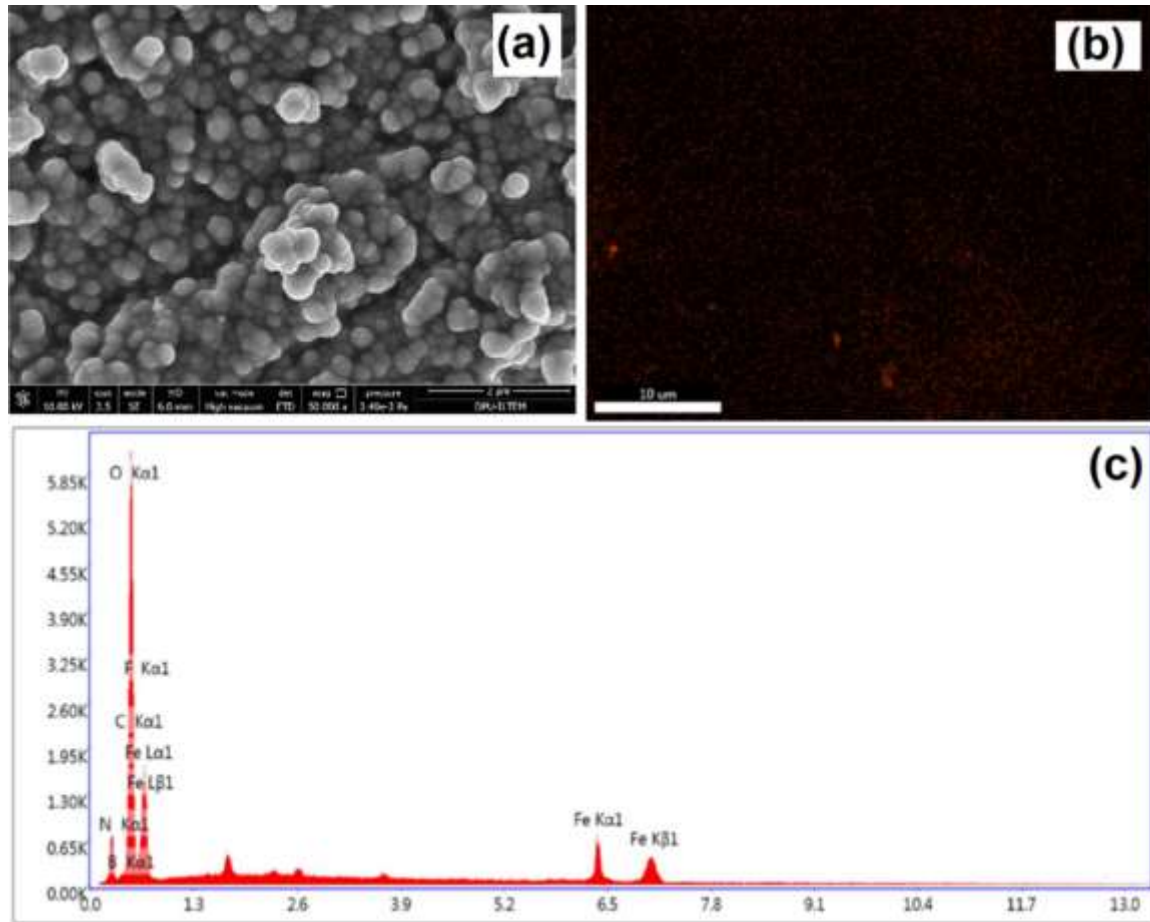
Şekil 35. Fe-int.KG yüzeyindeki PPy/FeO x /CMC kaplamanın (a) SEM görüntüsü, (b) Fe-EDX haritalaması ve (c) EDX alan spektrumu
