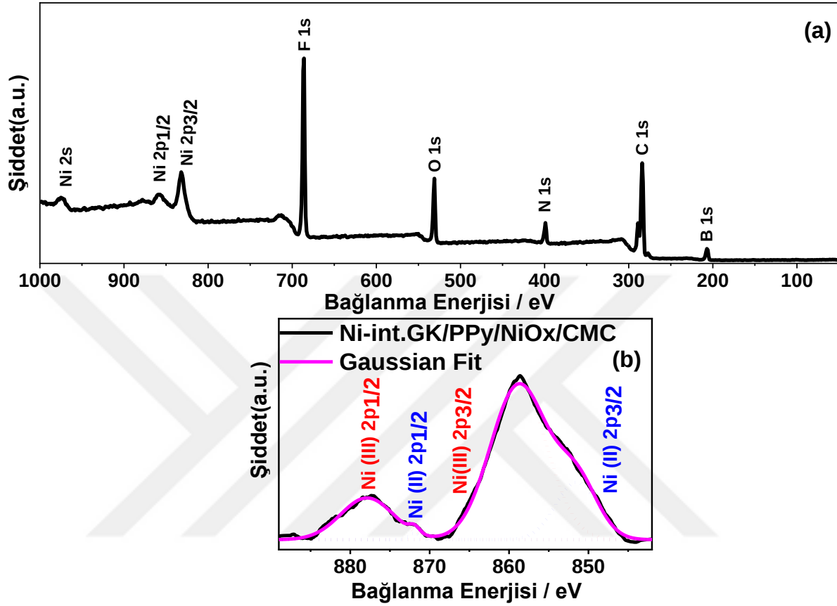
Şekil 27. PPy/NiO x /CMC kaplamanın XPS ile karakterizasyonu: Ni-int.GK yüzeyindeki PPy/NiO x /CMC kaplamanın (a) tam taraması (b) Ni 2p kısmi taraması.
