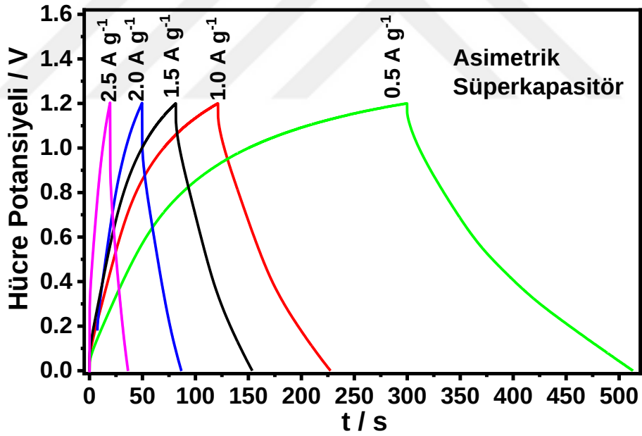
Şekil 4.25. V-int.GK/PPy/VO x /CMC elektrodu ( 10.0 mg cm -2 kütle yüklemesinde) kullanılarak hazırlanan hücre konfigürasyonları için 100 mM HBF 4 /TBABF 4 içeren asetonitril/adiponitril içinde çeşitli akım yoğunluklarında elde edilen simetrik ve asimetrik süperkapasitörün galvanostatik şarj-deşarj eğrileri.
