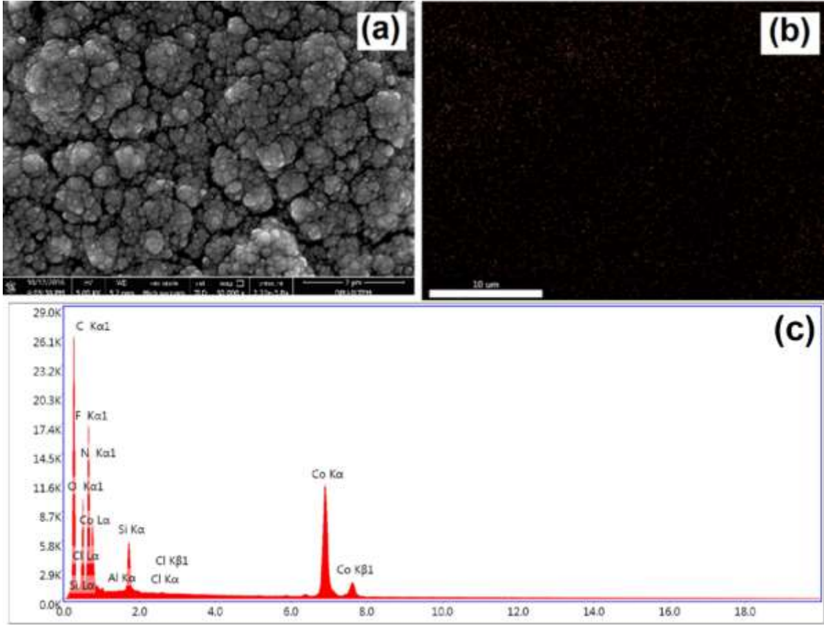
Şekil 33. Co-int.KG yüzeyindeki PPy/CoO x /CMC kaplamanının (a) SEM görüntüsü, (b) Co-EDX haritalaması ve (c) EDX alan spektrumu
