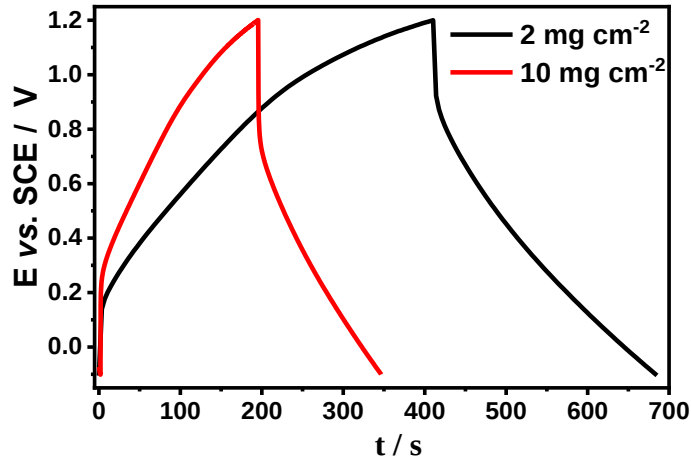
Şekil 4.17. (a) 2 \text{ mg cm}^{-2} ve (b) 10.0 \text{ mg cm}^{-2} kütle yüklemesiyle sentezlenen V-int. KG/PPy/VO x /CMC elektrodun 100 mM HBF 4 /TBABF 4 çözeltilisinde 2 \text{ A g}^{-1} 'da alınan galvanostatik şarj-deşarj eğrileri, ( A_{\text{KG}} = 0.0244 \text{ cm}^2 ).
