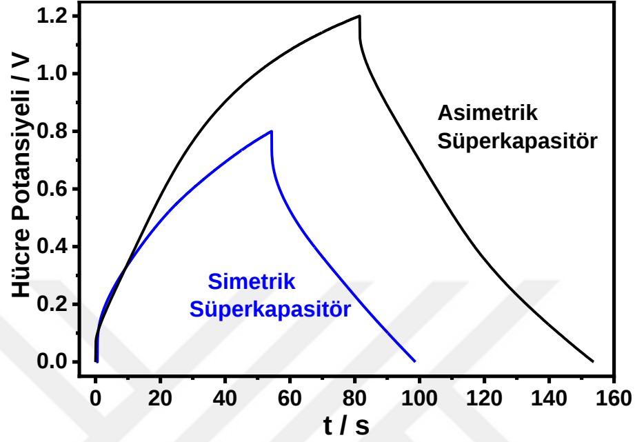
Şekil 4.23. V-int.GK/PPy/VO x /CMC ( 10.0 mg cm -2 kütle yüklemesinde) elektrodu kullanılarak hazırlanan iki hücre konfigürasyonu için 100 mM HBF 4 /TBABF 4 içeren asetonitril/adiponitril elektrolitinde hücre voltajlarının zamana göre değişimi ( 1.5 A g -1 ).
