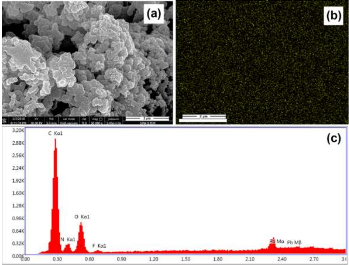
Şekil 30. Pb-int.KG yüzeyindeki PPy/PbO x /CMC kaplamanın (a) SEM görüntüsü, (b) Pb-EDX haritalaması ve (c) EDX alan spektrumu
