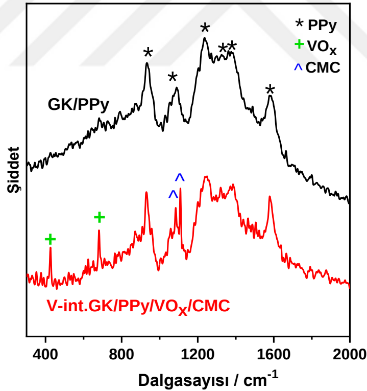
Şekil 4.3. Grafit kağıt (GK) yüzeyinde (a) PPy homopolimerinin (b) V-int.GK/PPy/VO x /CMC kompozitinin (300-2000 cm -1 ) Raman spektrumu.
