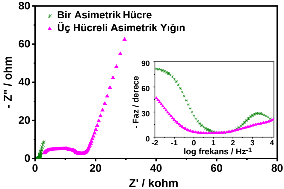
Şekil 4.38. 1.0 cm 2 (1 cm x 1 cm) lik Pb-int.GK/PPy/PbO x /CMC (10.0 mg cm -2 ) elektrotları kullanılarak hazırlanan bir hücre ve üç hücreli asimetrik yığının PVA:H 2 SO 4 jel elektrolit çözeltisinde alınan Nyquist eğrileri (Eşdeğer devre ve Bode eğrileri şekil içinde gösterilmiştir)
