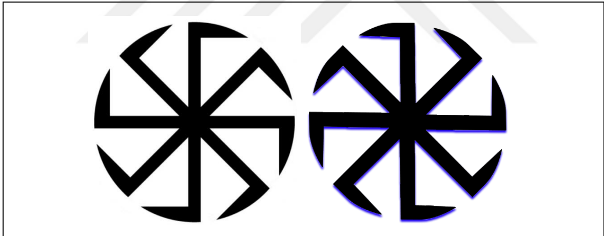
Şekil 3.9. Kalavrot ve Solntsevorot
