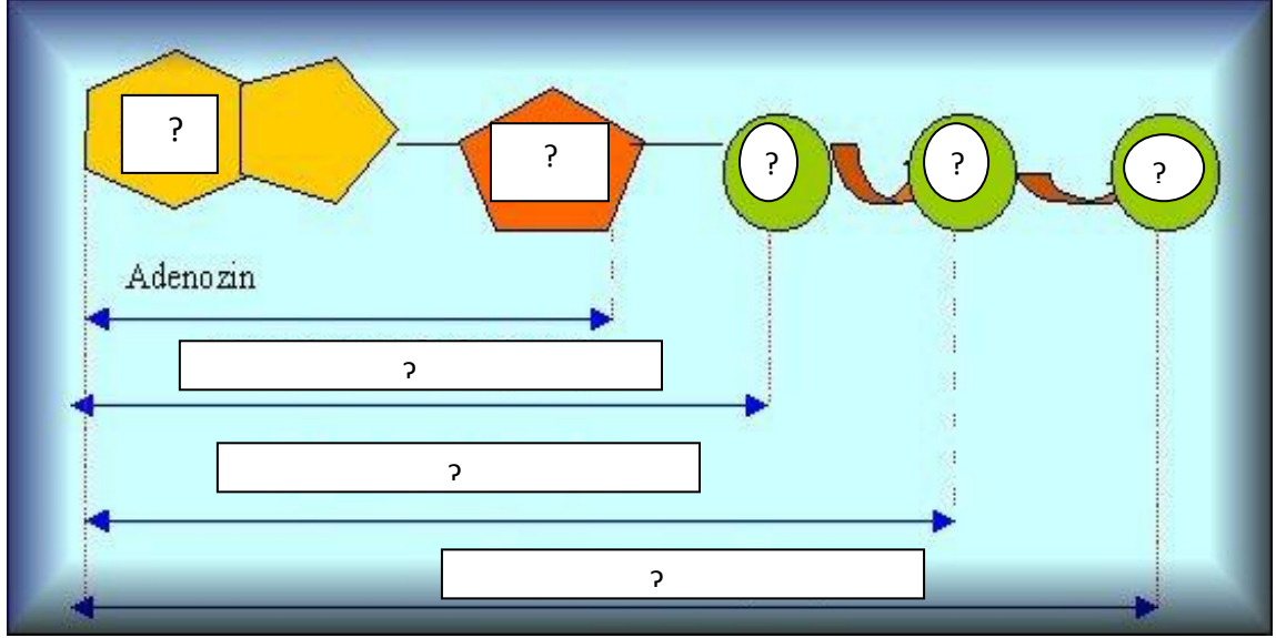
ATP MOLEKÜLÜ
