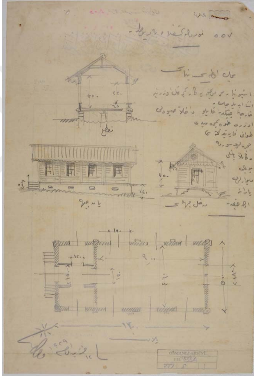
Şekil 88: "Yemek odası binası" başlıklı, R.12 Haziran 1329/25 Haziran 1913 tarihli ve Vedad imzalı cephe ve plan çizimleri. (BOA.HH.EBA.779-5-1)
