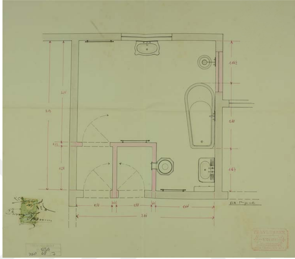
Şekil 85: Zincirlikuyu Kasrı'nda yaptırılan banyonun R.14 Teşrinisani 1329/M.27 Ekim 1913 tarihli ve Franz Thamm imzalı planı. (BOA.HH.EBA.760-45-7)
