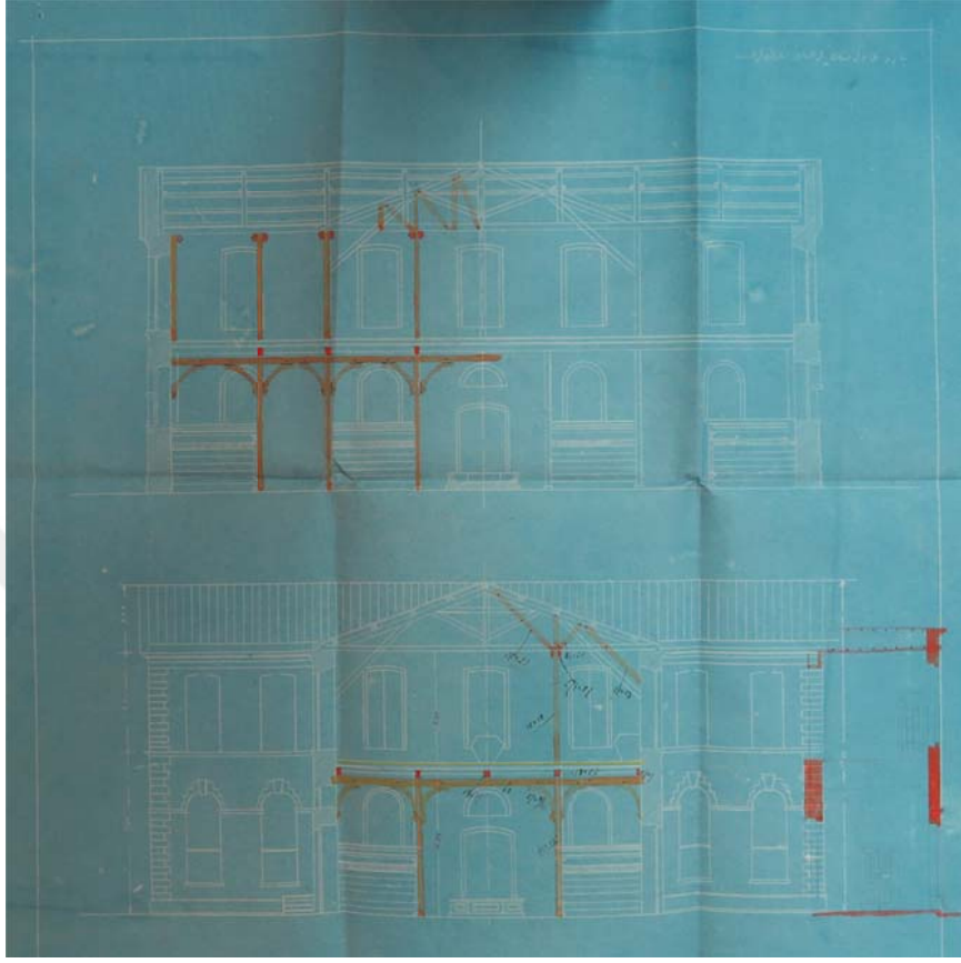
Şekil 60: Tarihsiz ve imzasız "Tiyatro Tavilesi arzani makta'aları" başlıklı yatay kesit çizimi. (BOA-HH-EBA-706-1)
