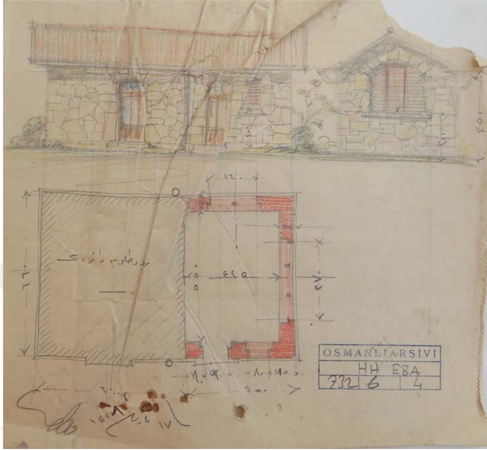
Şekil 72: R.17 Mart 1328/30 Mart 1912 tarihli ve Vedad imzalı cephe ve plan. Planın içinde "Mevcut tulumba dairesi" yazıyor. Yanındaki kırmızı ile renklendirilmiş plan ise eklenecek yapıya ait. (BOA.HH.EBA.732-6-4.)
