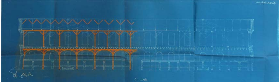
Şekil 62: R.Haziran 1325/Haziran-Temmuz 1909 tarihli, "Tiyatro tavilesinin tûlânî makta'ı" başlıklı ve Vedad imzalı düşey kesit çizimi. (BOA-HH-EBA-706-3)
