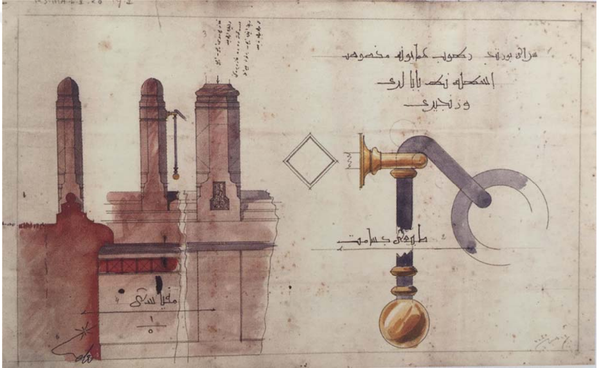
Görsel 74: "Sarayburnu'nda rükub-u hümayuna mahsus iskelenin babaları ve zincirleri" başlıklı ve Vedad imzalı çizim. (Afife Batur, "Sermimar-ı Hazret-i Şehriyari: Mehmed Vedad", 150. Yılında Dolmabahçe Sarayı Sempozyumu Bildirileri, TBMM Matbaası, Ankara, 2007, s.103)
