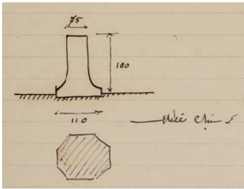
Şekil 35: 30 numaralı keşif defterinde yer alan kaide çizimi. (BOA.HH.D.27125)
