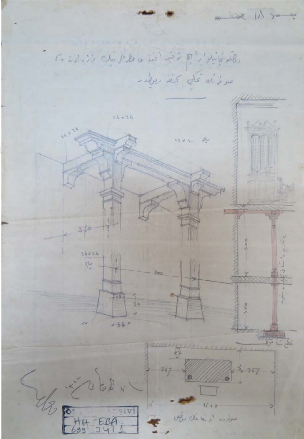
Şekil 77: "Devletli necâbetli İbrahim Tevfik Efendi hazretlerinin dairelerindeki sofanın tahkîmi keşfine merbuttur" başlıklı, R.7 Kanunusani 1327/20 Ocak 1912 tarihli ve Vedad imzalı çizim. (BOA. HH-EBA.699-34-2)
