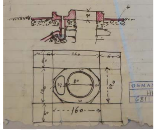
Şekil 22: "Beşiktaş Saray-ı Hümayunu kuyularının bilezikleri" başlıklı keşif defterine ait çizim. (BOA.HH.EBA.681-32)
