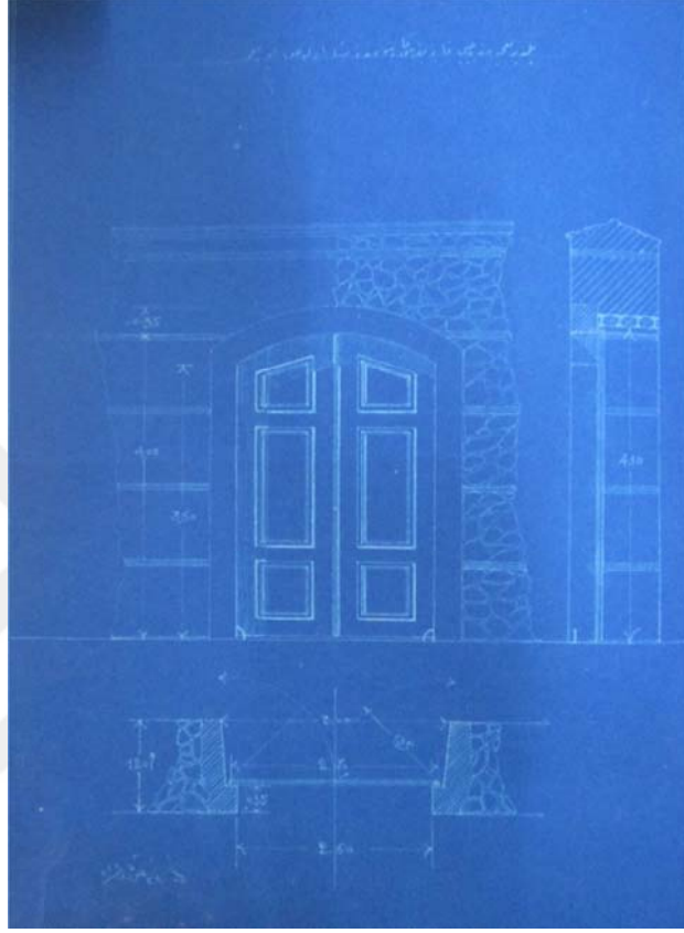
Şekil 67: "Yıldız bahçesinde Çini Fabrikası karşısında inşa olunacak kapı" başlıklı, R.24 Kanunusani 1325/6 Şubat 1910 tarihli ve Vedad imzalı çizim. (BOA.HH.EBA.679.12)
