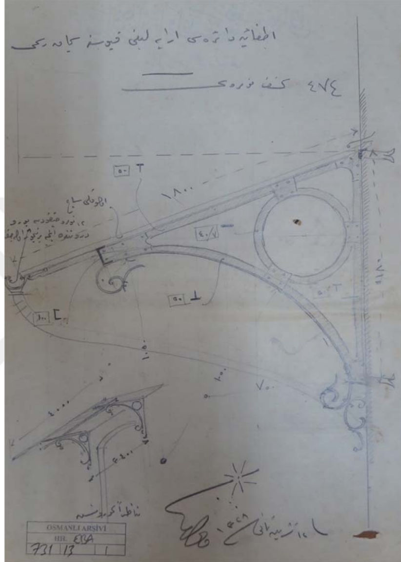
Şekil 40: Vedad Bey tarafından İtfaiye Dairesi için hazırlanmış daha ileri tarihli bir çalışma: "İtfaiye dairesi arabalığı kapısına saçak inşası" başlıklı ve R.13 Teşrinisani 1328/26 Kasım 1912 tarihli keşif defterinin ekindeki Vedad imzalı çizim. (BOA.HH.EBA.731-13-3)
