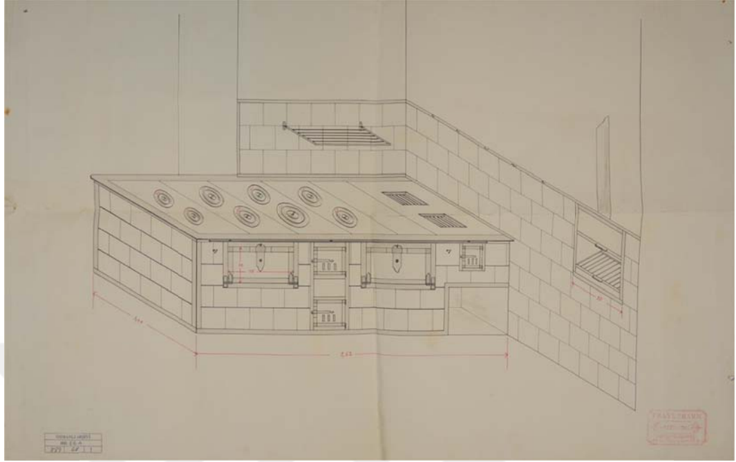
Şekil 86: Zincirlikuyu Kasrı için sipariş edilen mutfak sobasının çizimi. (BOA.HH.EBA.789-47-
