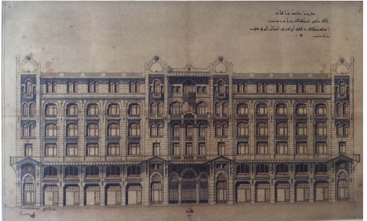
Şekil 94: Vedad Bey'in Emlâk-ı Hakani Mimarı imzasıyla hazırladığı R.1330/1914 tarihli cephe rölövesi. (Afife Batur, "Sermimar-ı Hazret-i Şehriyari: Mehmed Vedad", 150. Yılında Dolmabahçe Sarayı Sempozyumu Bildirileri, TBMM Matbaası, Ankara, 2007, s.103)
