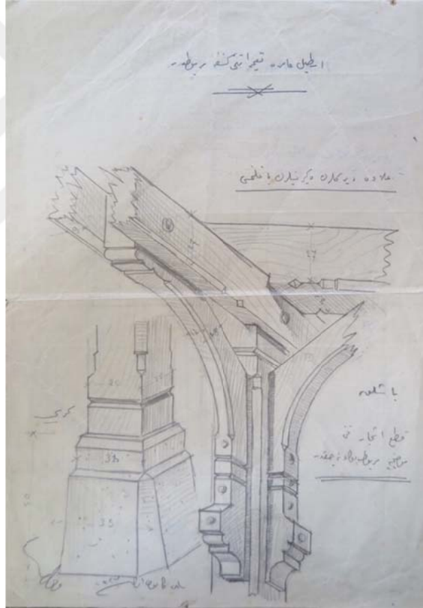
Şekil 63: "İstabl-ı Âmire tamirâtı keşfine merbuttur. İlave direklerin ve kirişlerin bağlanması" başlıklı R.28 Kanunuevvel 1327/10 Ocak 1912 tarihli ve Vedad imzalı çizim. (Bodrum Mimarlık Kitaplığı, Vedad Tek Arşivi, Süha Özkan ve Pelin Derviş Koleksiyonu.)
