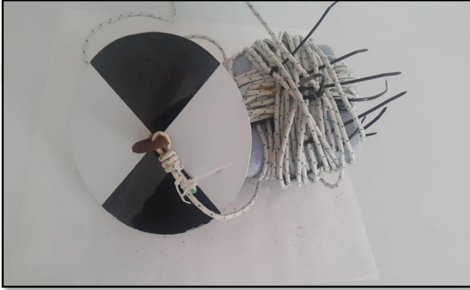
Şekil 3.9. Arazide kullanılan seki disk
