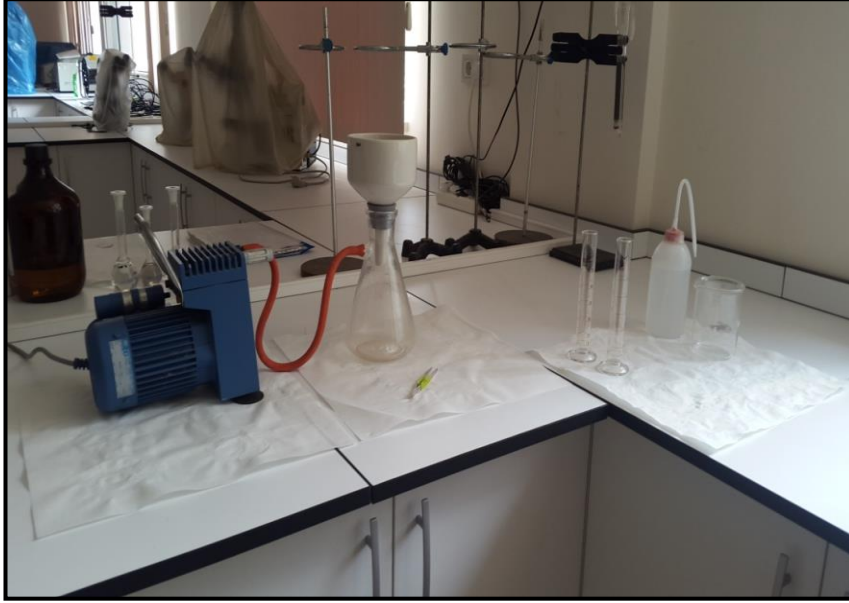
Şekil 3.11. AKM tayini düzeneği
