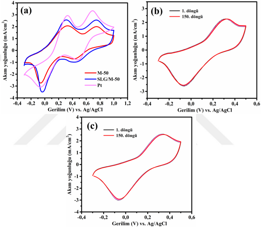
Şekil 4.26. (a) M-50, SLG/M-50 ve Pt nin CV eğrileri, (b) M-50 ve (c) SLG/M-50 filmlerinin çoklu CV eğrileri
