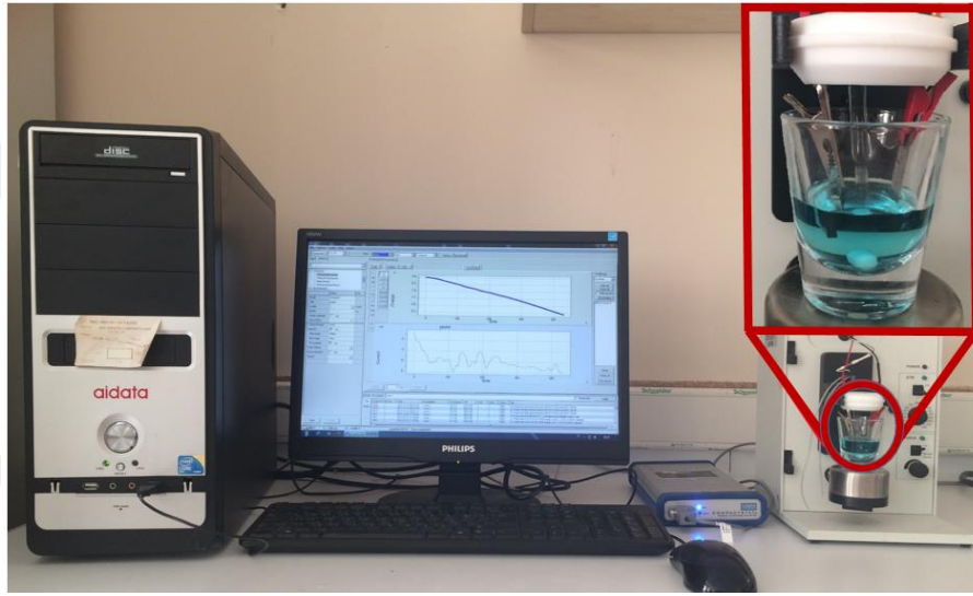
Şekil 3.1. Elektro-polimerizasyon işleminde kullanılan sistemin dijital fotoğrafı ve hücrenin yakından görünümü (iç resim)
