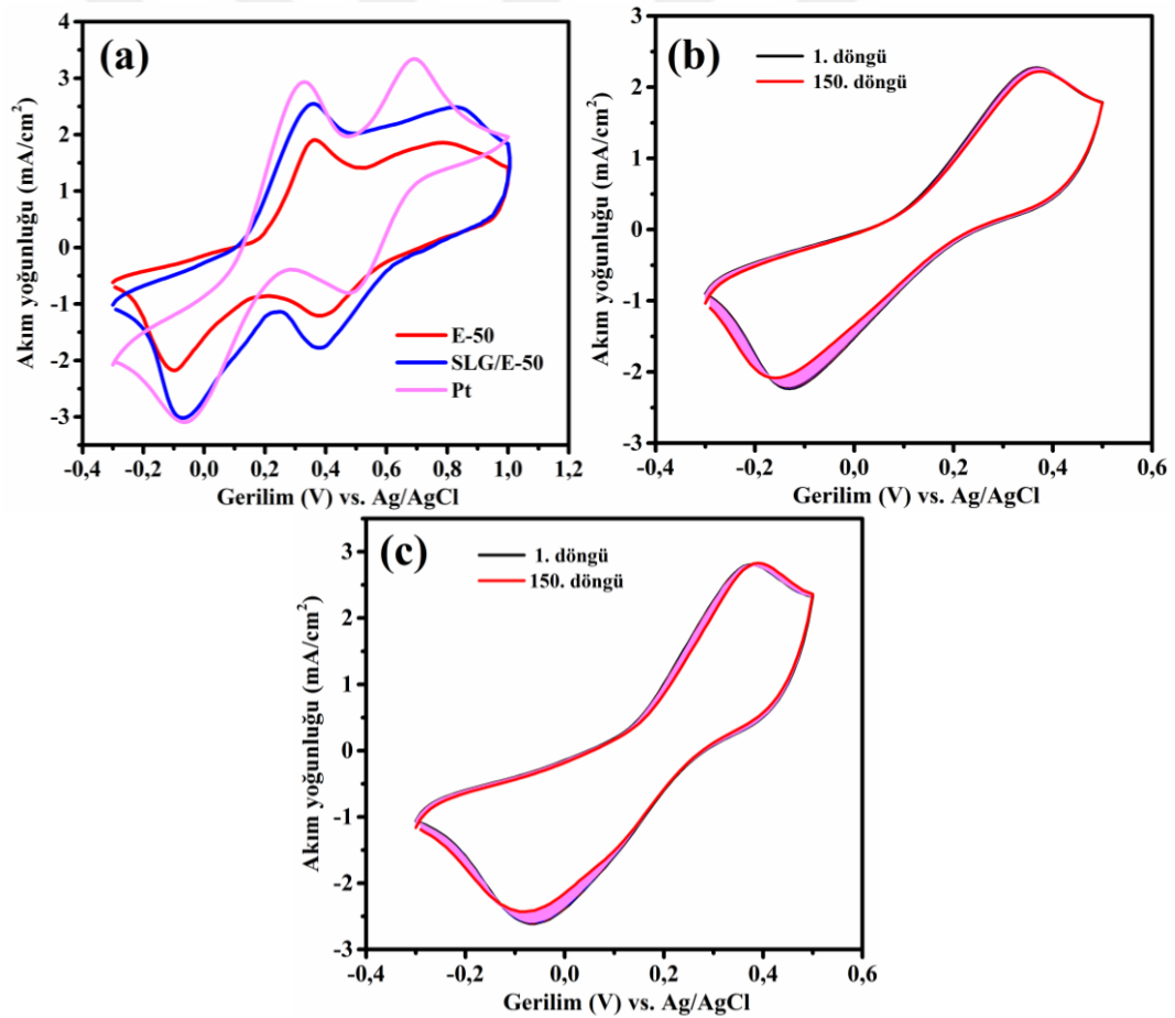
Şekil 4.25. (a) E-50, SLG/E-50 ve Pt nin CV eğrileri, (b) E-50 ve (c) SLG/E-50 filmlerinin çoklu CV eğrileri
