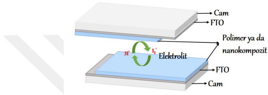
Şekil 3.6. Karşıt elektrotlarla hazırlanan simetrik hücreler
