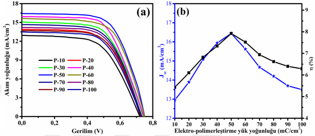
Şekil 4.6. (a) PProDOT temelli hücrelerin kalınlığa bağlı J-V eğrileri ve (b) akım yoğunluğu-dönüşüm verimliliği değişimi
