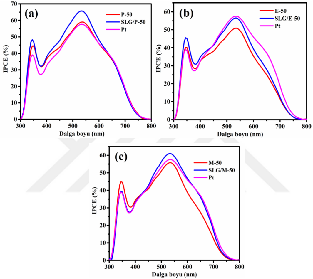
Şekil 4.30. (a) P-50, SLG/P-50 ve Pt, (b) E-50, SLG/E-50 ve Pt, (c) M-50, SLG/M-50 ve Pt filmleri üretilen BDH'lerin kuantum verimliliği eğrileri
