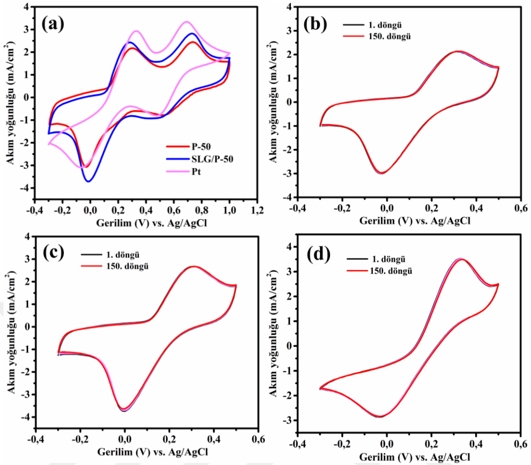
Şekil 4.24. (a) P-50, SLG/P-50 ve Pt nin CV eğrileri, (b) P-50, (c) SLG/P-50 ve (d) Pt filmlerinin çoklu CV eğrileri
