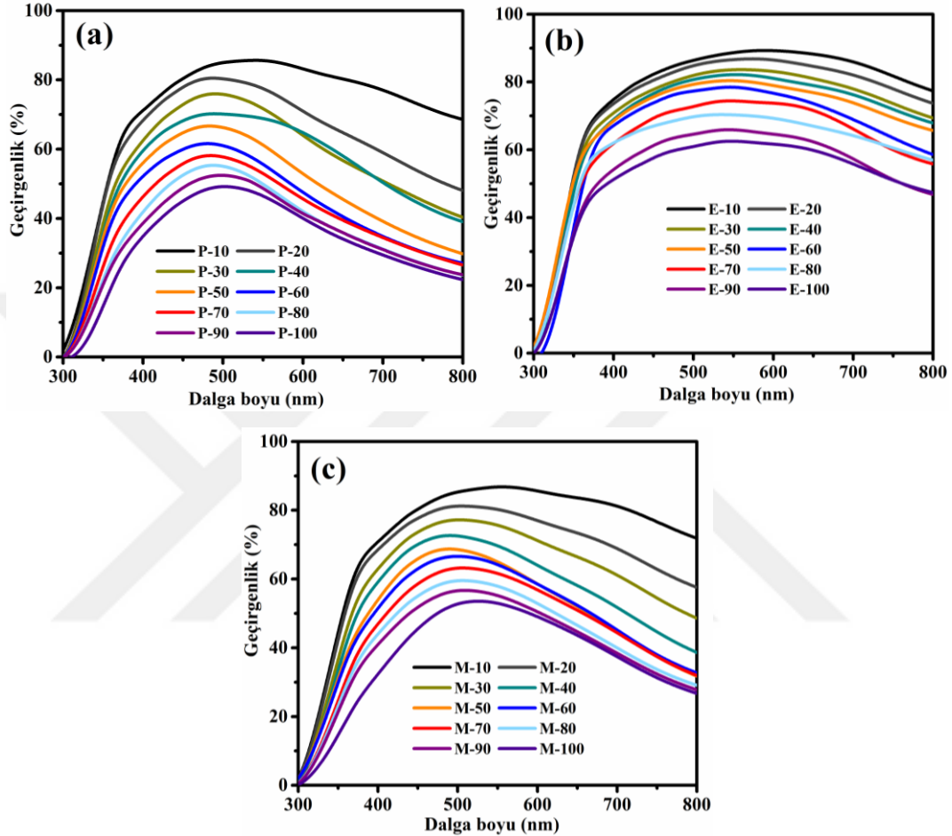
Şekil 4.3. Farklı kalınlıklarda elde edilen (a) PProDOT, (b) PProDOT-Et 2 ve (c) PProDOT-Me 2 polimerlerinin ışık geçirgenliği grafikleri
