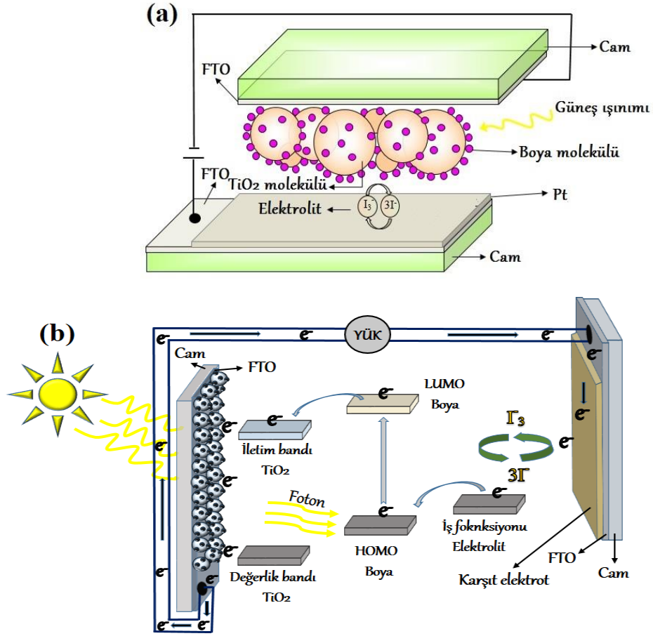
Şekil 1.1 (a) Boya duyarlı güneş hücresinin yapısı ve (b) çalışma prensini gösteren şemalar
