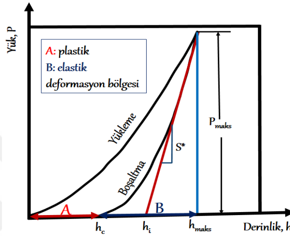
Şekil 4.17. Tipik bir yük (P) batma derinliği (h) eğrisini gösteren grafik
