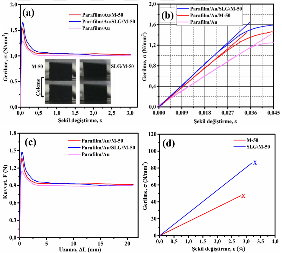
Şekil 4.21. (a) Parafilm/Au/M-50, Parafilm/Au/SLG/M-50 ve Parafilm/Au filmlerinin gerilme-şekil değiştirme eğrileri, (b) karşılık gelen çekme-şekil değiştirme eğrilerinin lineer bölgedeki fitleri, (c) Parafilm/Au/M-50, Parafilm/Au/SLG/M-50 ve Parafilm/Au filmlerinin kuvvet-uzama eğrileri ve (d) M-50 ve SLG/M-50 filmlerinin hesaplanan gerilme-şekil değiştirme eğrileri
