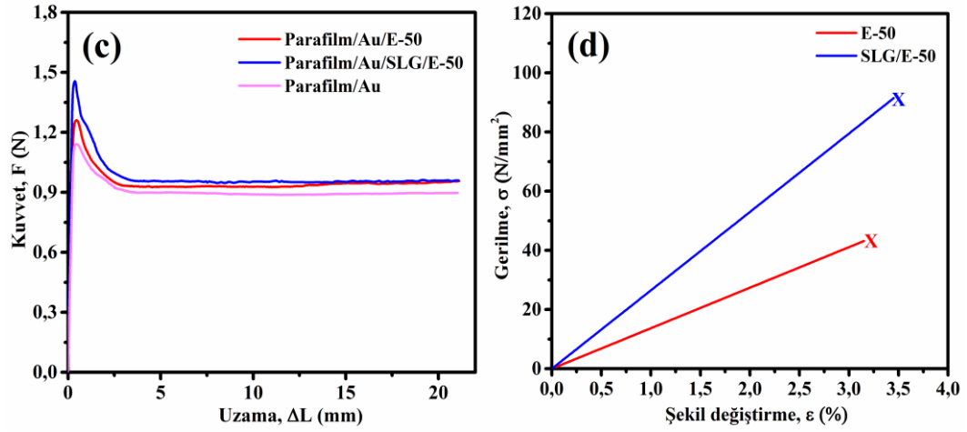
Şekil 4.20. (a) Parafilm/Au/E-50, Parafilm/Au/SLG/E-50 ve Parafilm/Au filmlerinin gerilme-şekil değiştirme eğrileri, (b) karşılık gelen çekme-şekil değiştirme eğrilerinin lineer bölgedeki fitleri, (c) Parafilm/Au/E-50, Parafilm/Au/SLG/E-50 ve Parafilm/Au filmlerinin kuvvet-uzama eğrileri ve (d) E-50 ve SLG/E-50 filmlerinin hesaplanan gerilme-şekil değiştirme eğrileri
