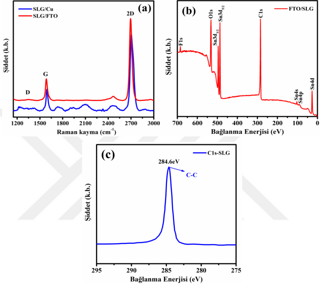
Şekil 4.10. (a) Bakır üzerindeki ve FTO alttaş üzerine aktarılan SLG yapısının Raman spektroskopisi, FTO/SLG yapısının (b) genel ve (c) C1s orbital XPS spektrumu
