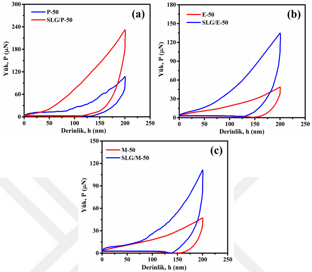
Şkil 4.18. Nano-çentikleme ölçümlerinden elde edilen (a) P-50, SLG/P-50, (b) E-50, SLG/E-50 ve (c) M-50, SLG-M-50 filmlerine ait yük-derinlik eğrileri
