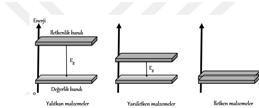
Şekil 1.5. Yalıtkan, yarıiletken ve iletken malzemelerde band aralıkları
