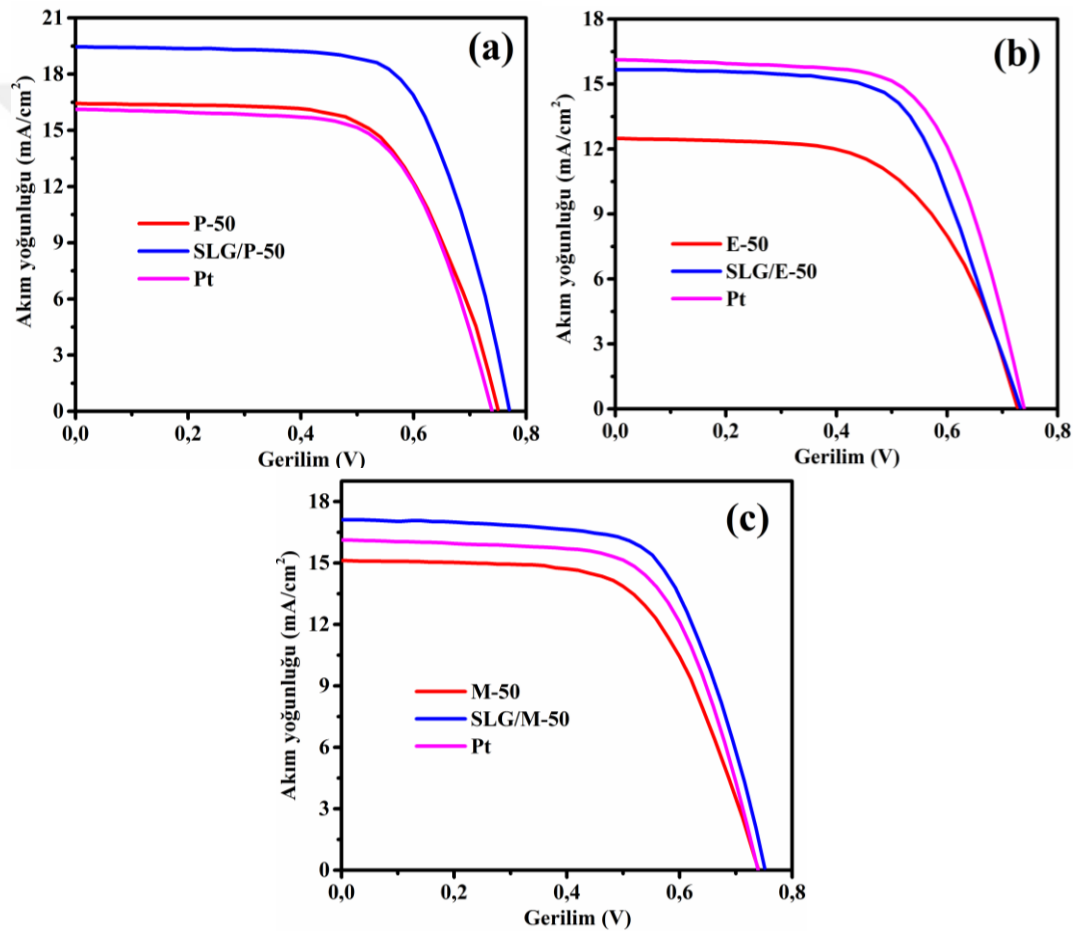
Şekil 4.29. (a) P-50, SLG/P-50 ve Pt, (b) E-50, SLG/E-50 ve Pt, (c) M-50, SLG/M-50 ve Pt filmleri üretilen BDGH'lerin J-V eğrileri
