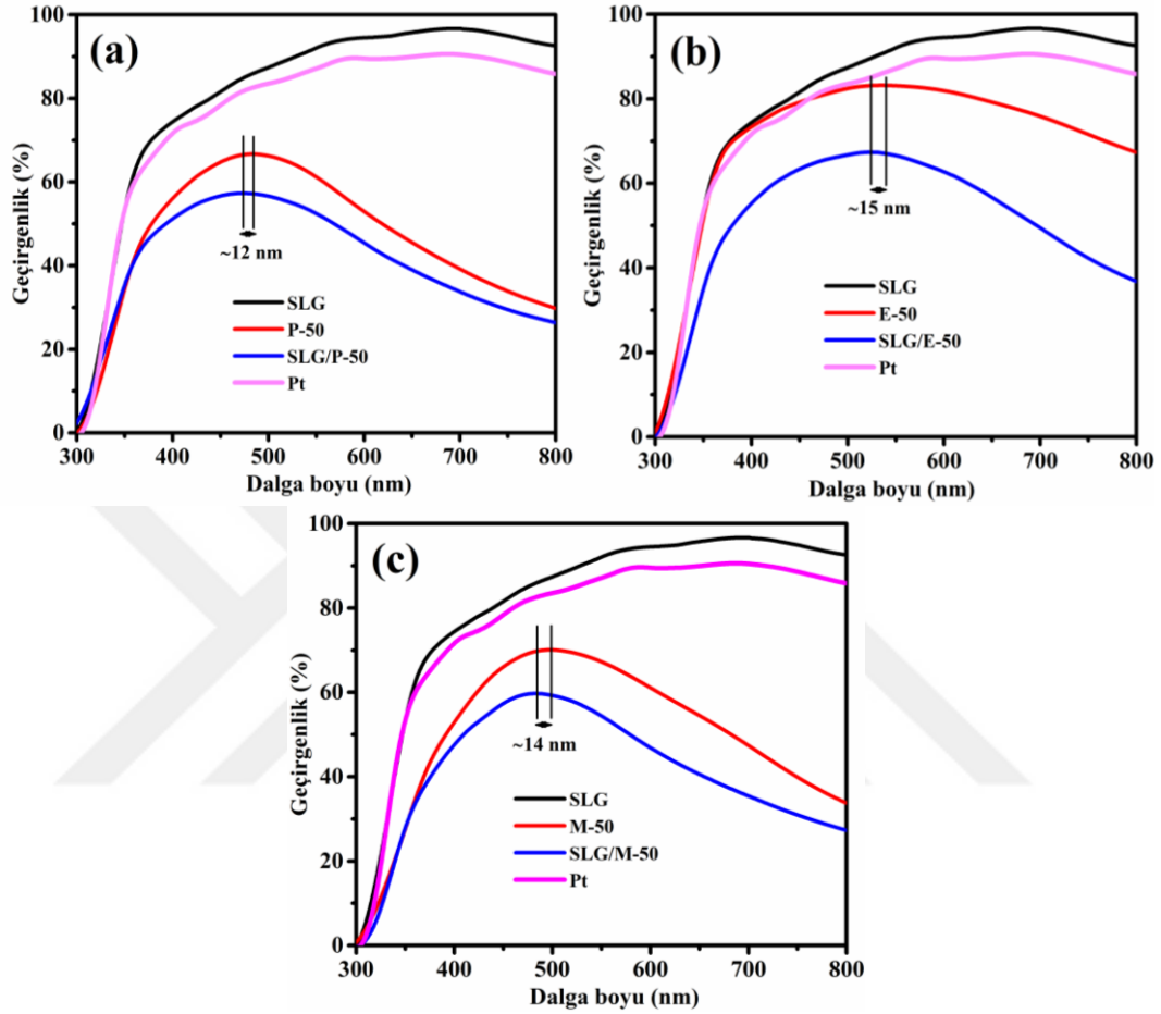
Şekil 4.14. (a) PProDOT, (b) PProDOT-Et 2 ve (c) PProDOT-Me 2 polimer tabanlı ince filmlerin geçirgenlik grafikleri
