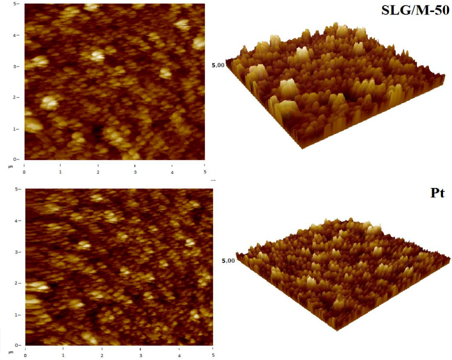
Şekil 4.16. Sentezlenen P-50, SLG/P-50, E-50, SLG/E-50, M-50, SLG/M-50 ve Pt yapıları filmlerin AFM görüntüleri (sol: 2-boyutlu ve sağ: 3-boyutlu)
