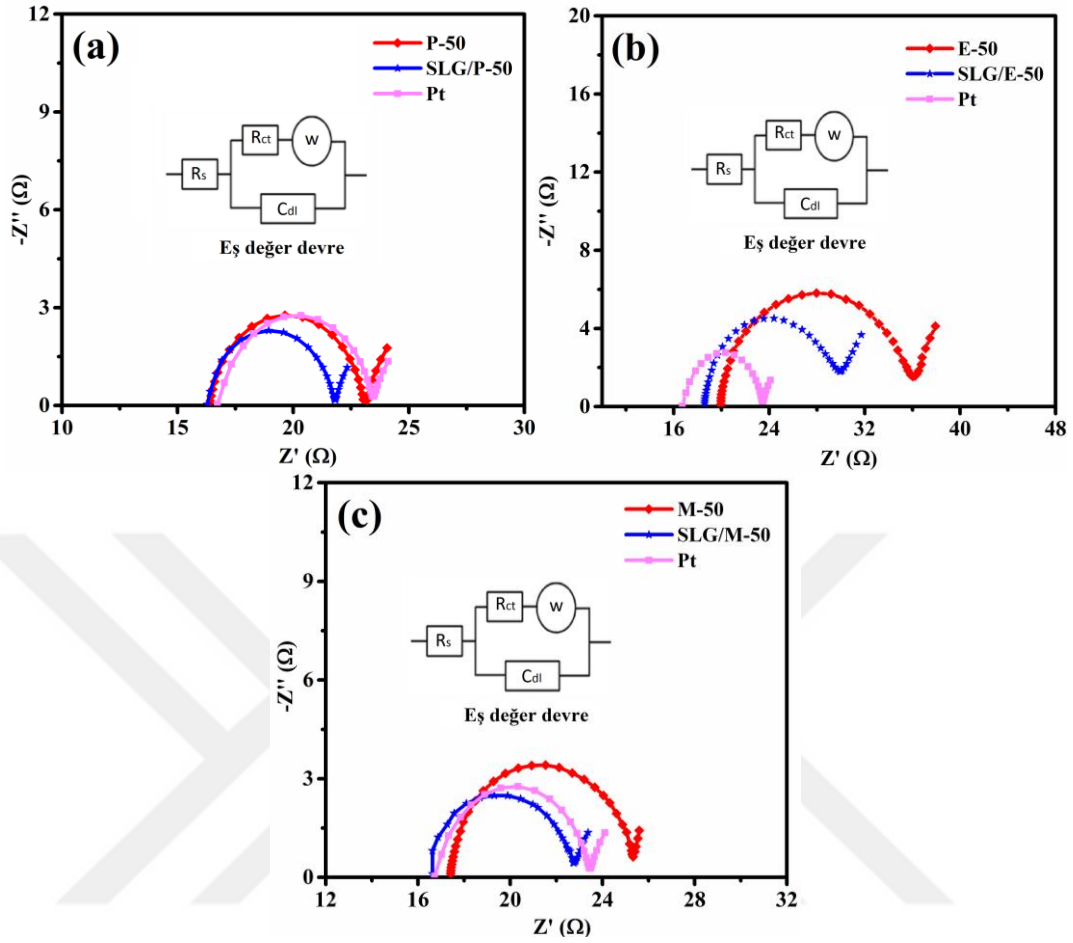
Şekil 4.27. (a) P-50, SLG/P-50 ve Pt, (b) E-50, SLG/E-50 ve Pt, (c) M-50, SLG/M-50 ve Pt filmleri ile oluşturulan simetrik hücrelerinin Nyquist eğrileri
