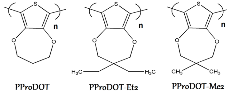
Şekil 1.9. PProDOT–X polimerlerinin moleküler yapıları
