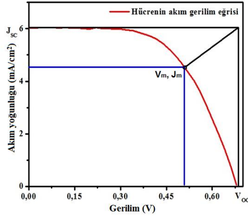
Şekil 4.5. BDGH'nin fotovoltaiik parametrelerinin belirlenmesi için örnek bir J-V eğrisi
