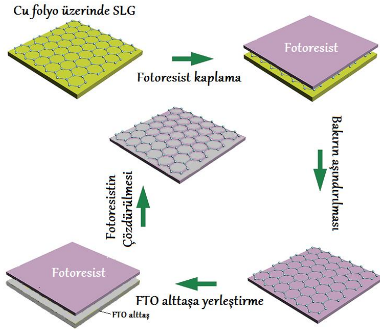
Şekil 3.4. Bakır plakalar üzerindeki SLG yapılarının FTO alttaşlara aktarımı için izelenen prosesin şematik gösterimi
