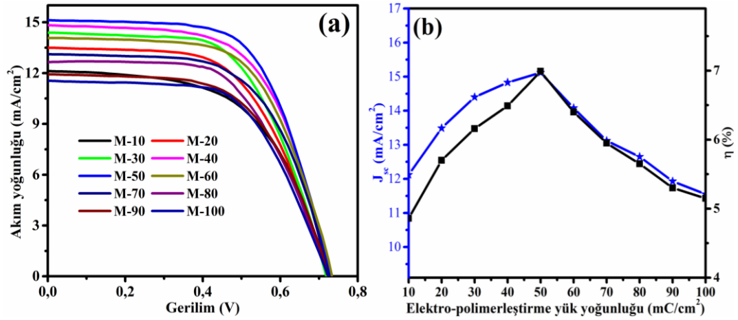
Şekil 4.8. (a) PProDOT–Me 2 temelli hücrelerin kalınlığa bağlı J-V eğrileri ve (b) akım yoğunluğu-dönüşüm verimliliği değişimi
