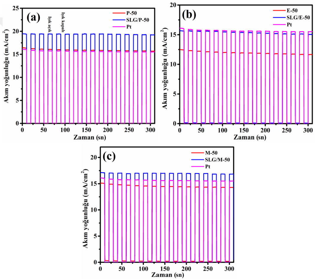
Şekil 4.31. (a) P-50, SLG/P-50 ve Pt, (b) E-50, SLG/E-50 ve Pt, (c) M-50, SLG/M-50 ve Pt filmleri üretilen BDGH'lerin başlat/durdur döngüleri
