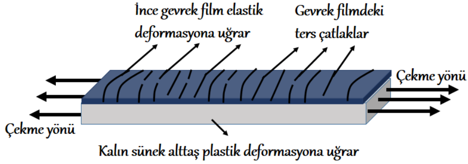
Şekil 4.22. Gevrek filmlerin sünek alttaşlar üzerindeki kırılma mekanizmaları
