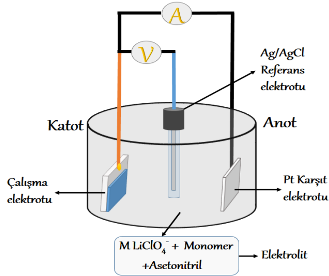
Şekil 1.10. Elektro-polimerizasyon işleminde kullanılan hücrenin şeması
