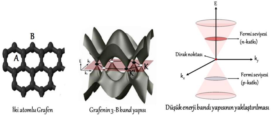
Şekil 1.13. Grafen yapısının elektronik bant yapısı
