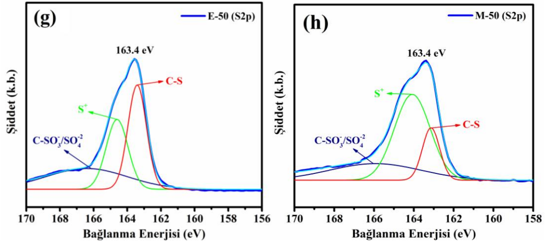
Şekil 4.1. (a) PProDOT-X polimerlerinin genel XPS haritaları, (b) P-150, (c) E-50 ve (d) M-150 polimerlerinin C1s orbitallerinin spektrumları, (e) PProDOT-X polimerlerinin O1s orbital spektrumları ve (f) P-150, (g) E-50 ve (h) M-50 polimerlerinin S2p orbitallerine ait spektrum haritaları
