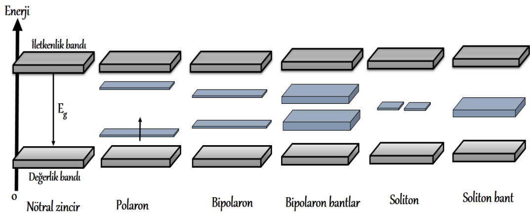
Şekil 1.7. İletken polimerlerde oluşan elektronik bandların şematik gösterimi
