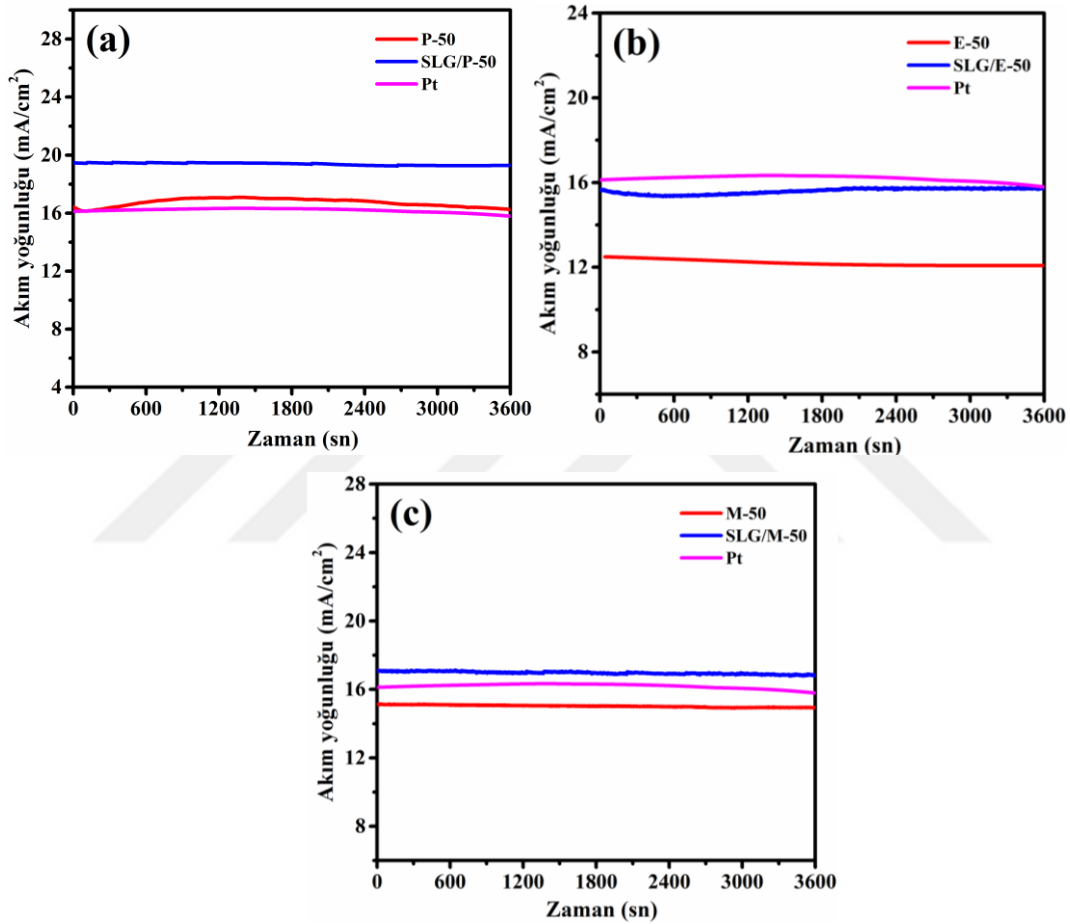
Şekil 4.32. (a) P-50, SLG/P-50 ve Pt, (b) E-50, SLG/E-50 ve Pt, (c) M-50, SLG/M-50 ve Pt filmleri üretilen BDGH'lerin zamana bağlı J_{sc} kararlılık profilleri
