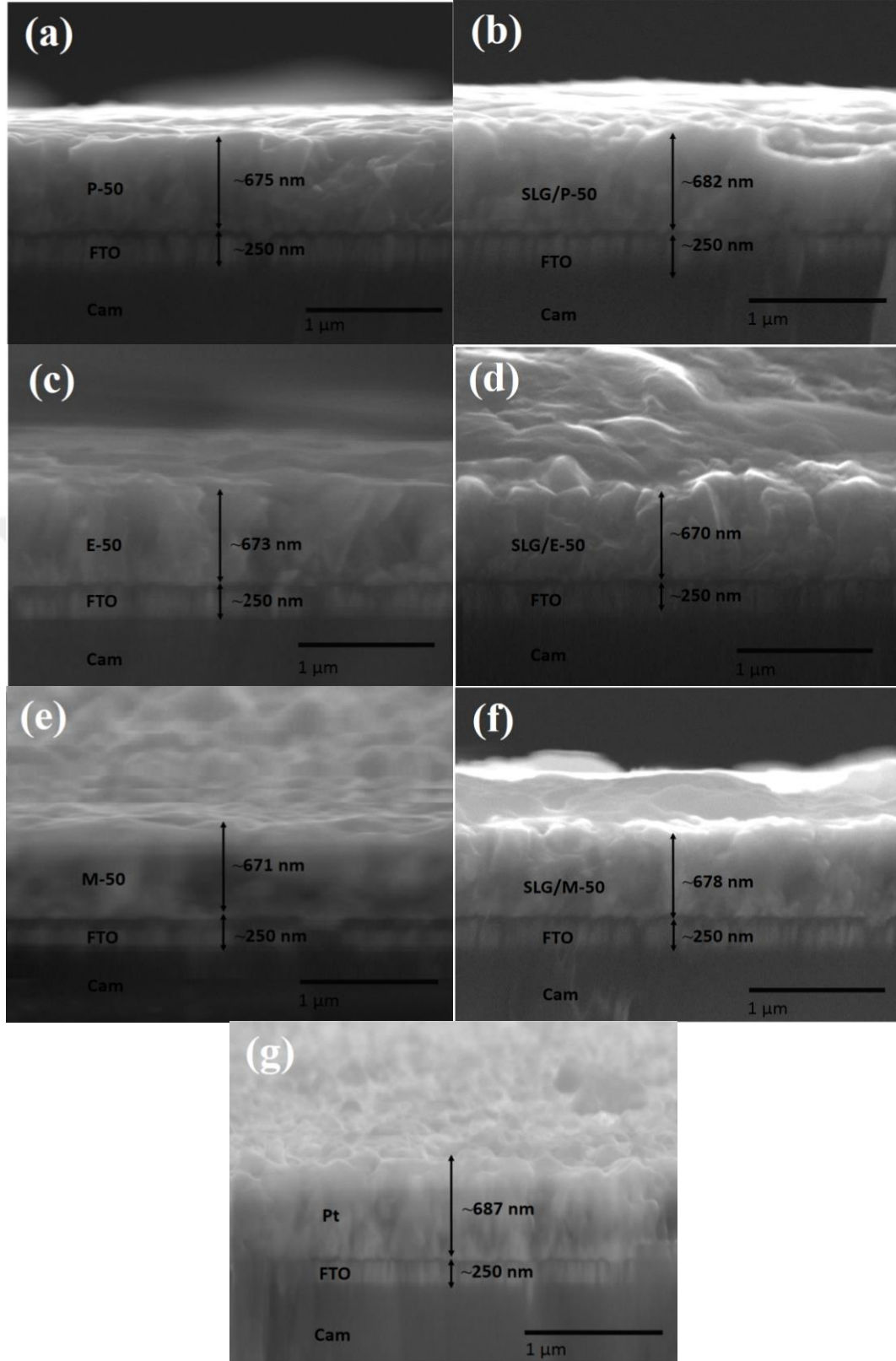
Şekil 4.13. (a) P-50, (b) SLG/P-50, (c) E-50, (d) SLG/E-50, (e) M-50, (f) SLG/M-50, (g) Pt yapılı karşıt elektrotların kesit alanları
