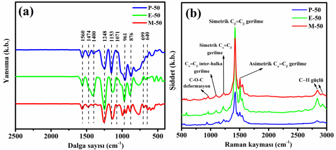
Şekil 4.2. PProDOT-X filmlerine ait (a) FT-IR ve (b) Raman spektroskopileri
