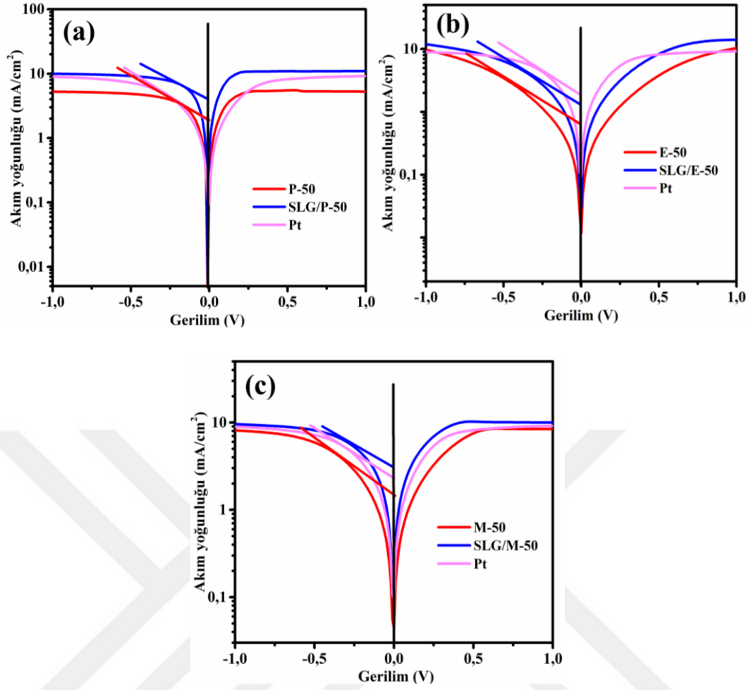
Şekil 4.28. (a) P-50, SLG/P-50 ve Pt, (b) E-50, SLG/E-50 ve Pt, (c) M-50, SLG/M-50 ve Pt filmleri ile oluşturulan simetrik hücrelerin Tafel polarizasyonları
