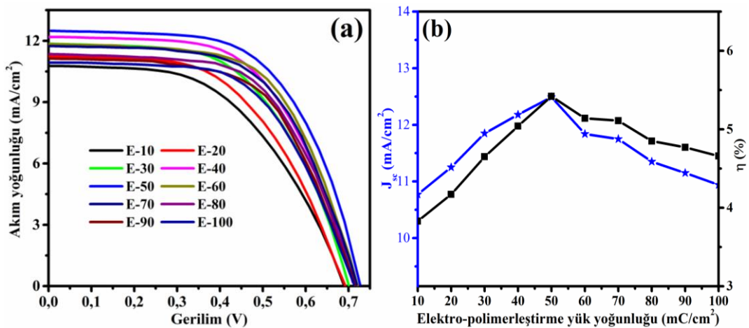
Şekil 4.7. (a) PProDOT–Et 2 temelli hücrelerin kalınlığa bağlı J-V eğrileri ve (b) akım yoğunluğu-dönüşüm verimliliği değişimi
