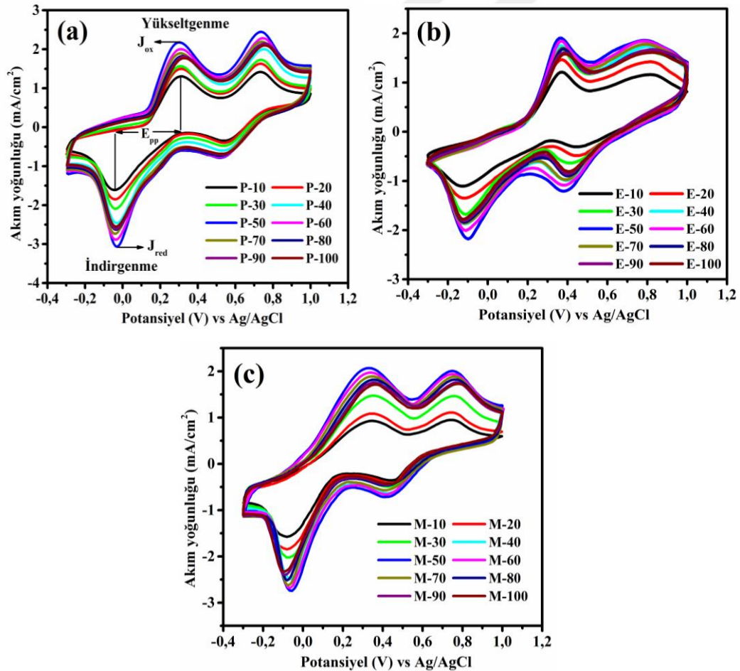
Şekil 4.4. Farklı kalınlıklarda elde edilen (a) PProDOT, (b) PProDOT–Et 2 ve (c) PProDOT–Me 2 polimerlerinin CV eğrileri
