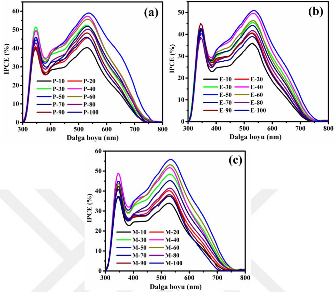
Şekil 4.9. Değişen PProDOT-X polimer kalınlıklarına bağlı BDGH'lerin kuantum verimlilik grafikleri
