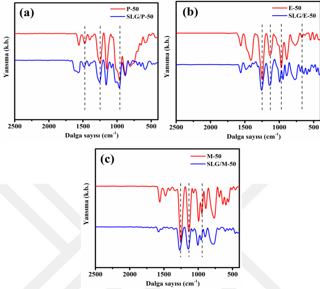
Şekil 4.12. (a) P-50, SLG/P-50, (b) E-50, SLG/E-50 ve (c) M-50, SLG/M-50 filmlerinin FT-IR spektrumları
