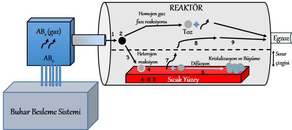
Şekil 1.14. CVD sisteminde içerisinde gerçekleşen reaksiyonların şematik gösterimi
