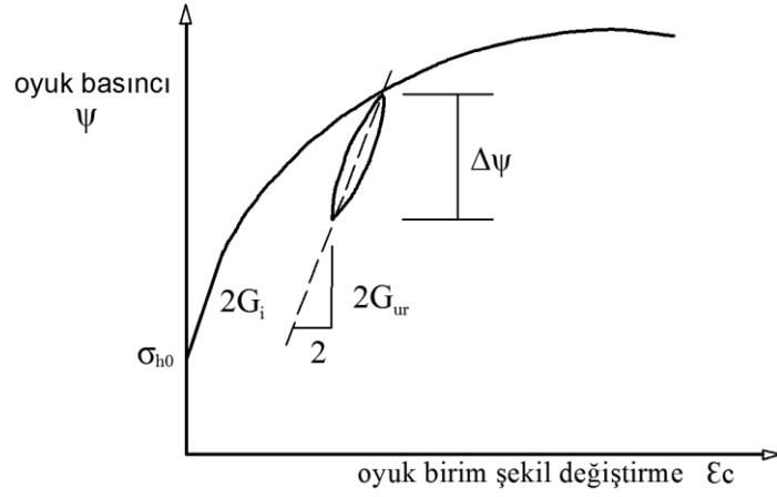
Şekil 3.2: Presiyometre eğrisinden kayma modülü (Yu, 2000).
