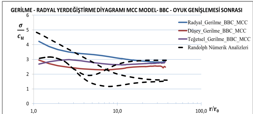
Şekil 6.5 : MCC modeli için oyuk genişlemesi sonrasında meydana gelen gerilme radyal yer değiştirme diyagramı.
