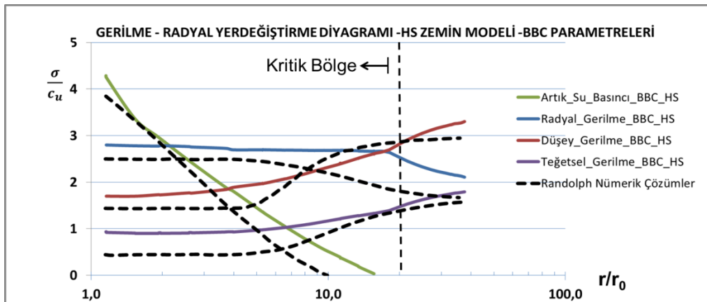
Şekil 6.4 : HS modeli için oyuk çevresinde meydana gelen c_u ile normalize edilmiş gerilme radyal yer değiştirme diyagramı.
