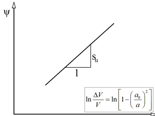
Şekil 3.3 : Gibson ve Anderson (1961) analizi ile grafik metodu.
