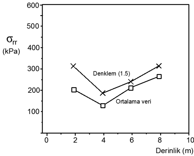
Şekil 3.6 : Normal konsolide Huntspill killeri için kazık gövde normal gerilmesini tahmini (Data verileri Coop ve Wrot, 1989).
