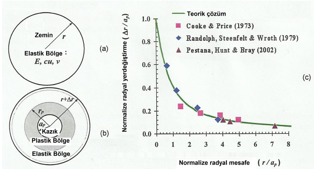
Şekil 5.8 : a) Oyuk genişlemesi öncesi zemin elementi b) Oyuk genişlemesi durumu c) Teorik ve ölçüme dayalı radyal doğrultudaki zemin deformasyonları karşılaştırılması (Biringen, 2005).
