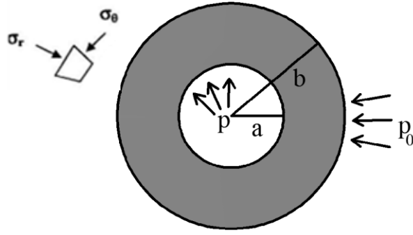
Şekil 2.1 : Uniform iç ve dış basınç etkisi altında silindirik oyuk.
