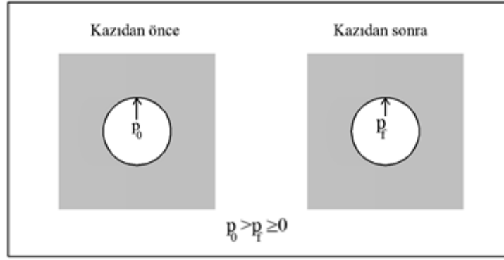
Şekil 3.11 : Tünel ya da yeraltı kazısı sırasında gerilme durumu.
