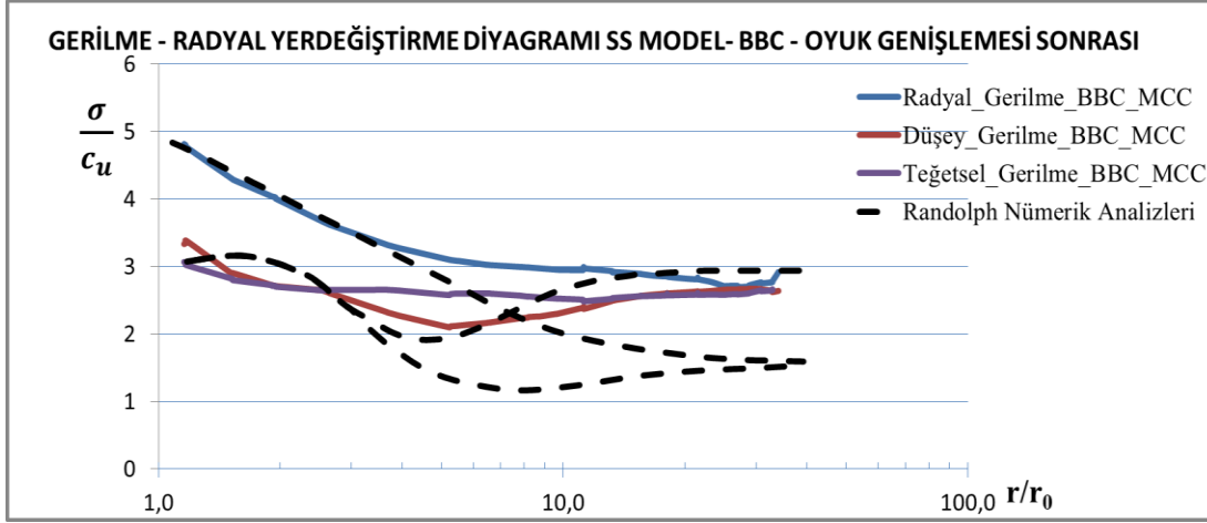
Şekil 6.6 : SS modeli için oyuk genişlemesi sonrasında meydana gelen gerilme radyal yer değiştirme diyagramı.
