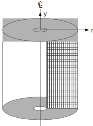
Şekil 5.3 : Bir eksenel simetrik problem (IGE, ETH Zurich).
