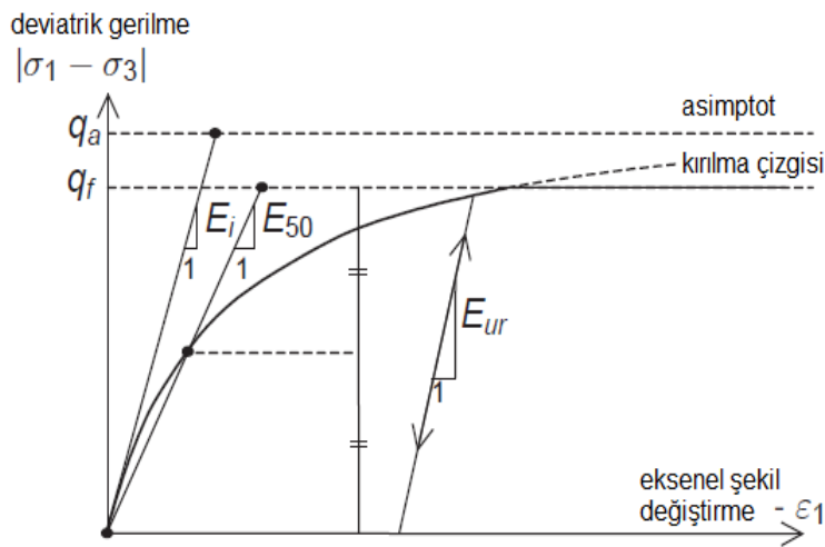
Şekil 4.5 : Hiperbolik gerilme-şekil değiştirme ilişkisi (Plaxis Manual 2D 2011).
