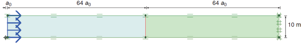
Şekil 5.10 : Silindirik oyuk genişlemesi modelleme geometrisi.
