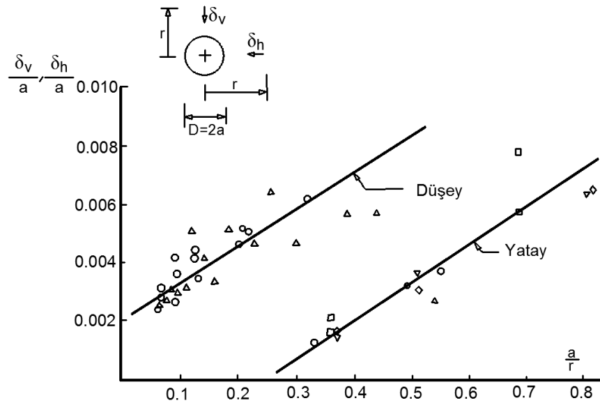
Şekil 3.13 : Tünel civari Londra kilinde düşey ve yatay yer hareketleri (Mair ve Taylor, 1993).
