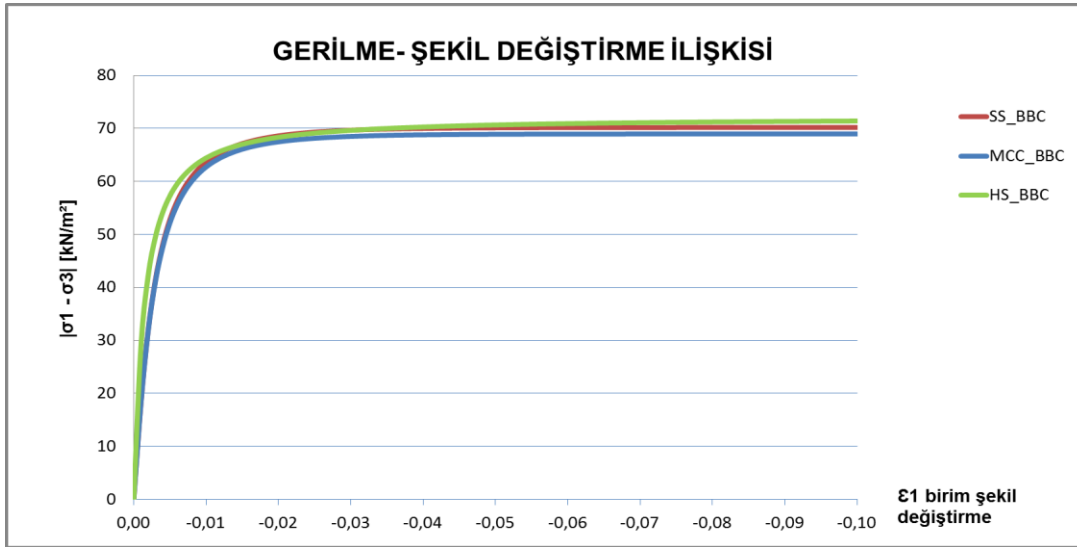
Şekil 5.15 : MCC, SS ve HS modellerden elde edilen gerilme şekil değiştirme ilişkisi.
