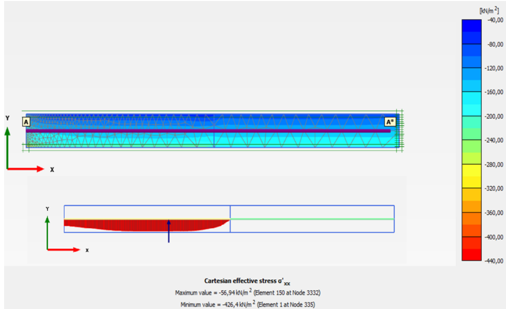
Şekil 5.19 : Sayısal modelleme için oyuk orta derinliğinde gerilme dağılımı.
