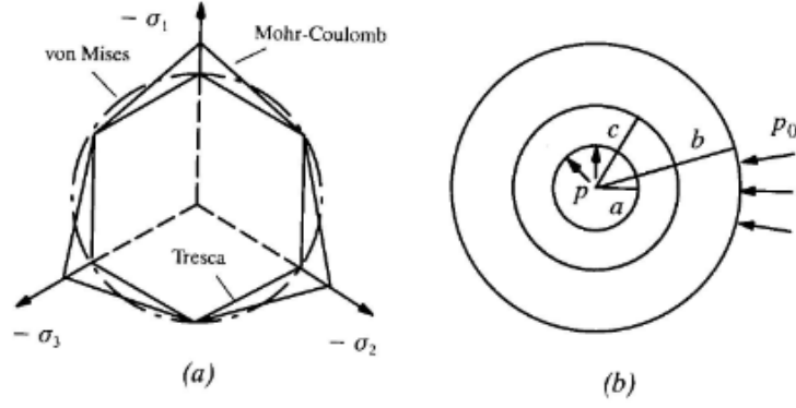
Şekil 2.2: Akma yüzeyleri ve silindirik bir oyukun genişlemesi
