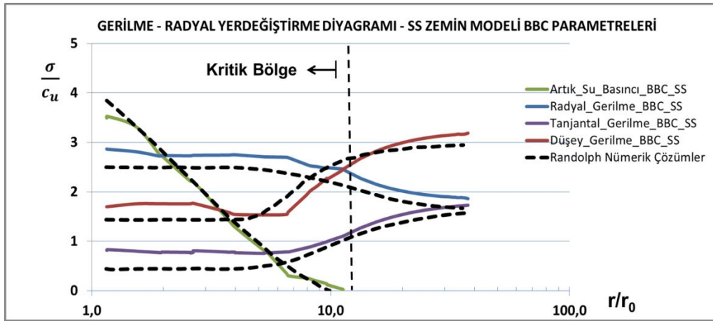
Şekil 6.3 : SS modeli için oyuk çevresinde meydana gelen c_u ile normalize edilmiş gerilme –radyal yer değiştirme diyagramı.
