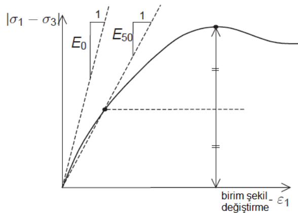
Şekil 4.1: Üç eksenli deney sonucu elde edilen E_0 ve E_{50} rijitlik modülleri (Plaxis 2011 2D Material Models Manual).
