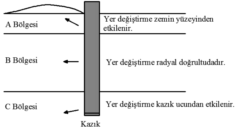
řekil 3.5 : Kazık klemeđi sonrasında zemin yerdeęiřtirmeđi.
