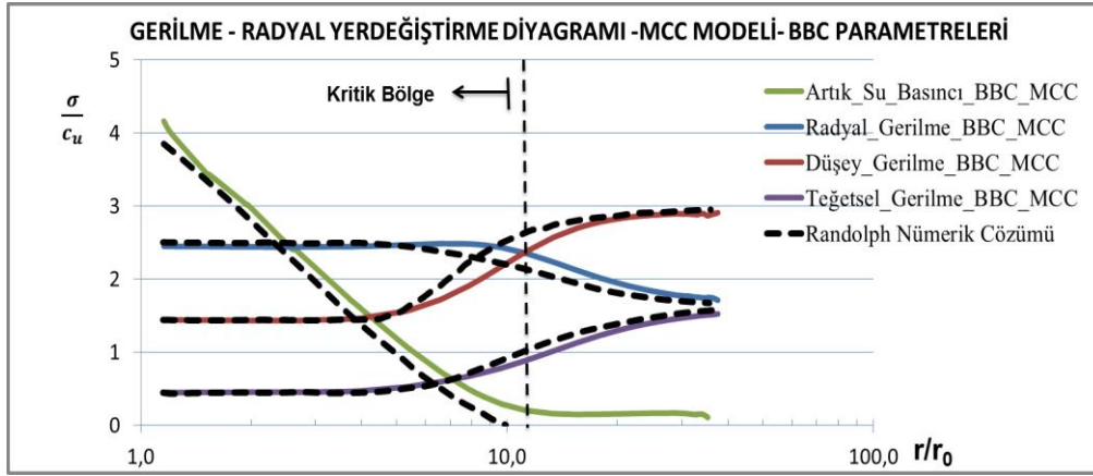
Şekil 6.2 :MCC modeli için oyuk çevresindeki c_u ile normalize edilmiş gerilme radyal yer değiştirme diyagramı.
