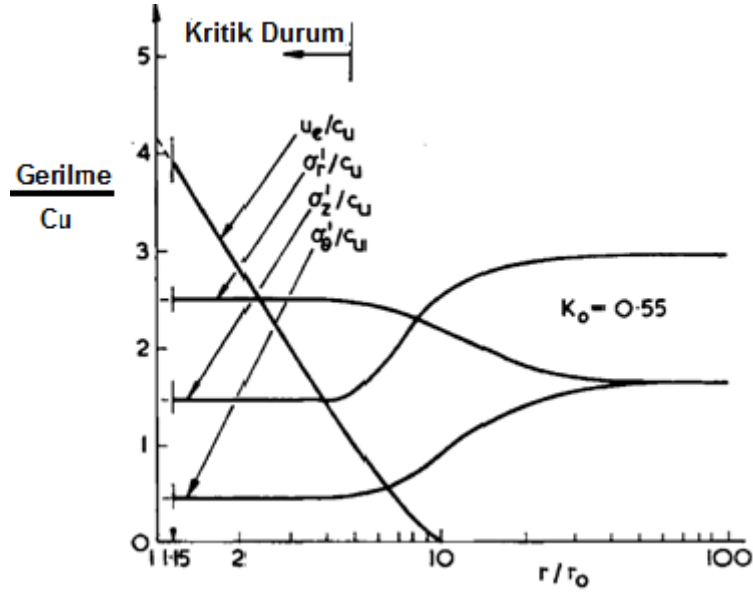
Şekil 5.5 : Kazık yükleme sonrası zemin çevresindeki gerilme dağılımı (AKO=1, Ko=0.55)- Carter vd. (1979).
