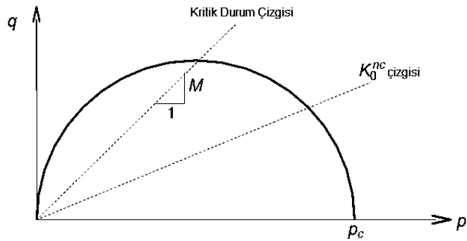
Şekil 4.3: p'-q akma yüzeyinde Modified Cam Clay akma yüzeyi (Plaxis Manual 2D 2011).
