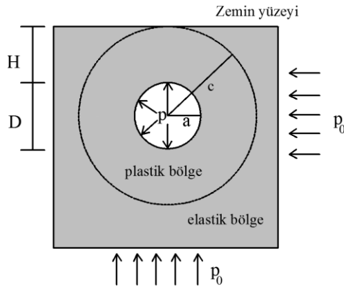
Şekil 3.15 : Tünelde göçme meydana gelme durumu.
