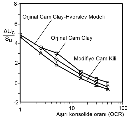
Şekil 5.7 : Oyuk duvarındaki artık boşluk suyu basıncı - OCR değişimi (Collins ve Yu 1996).
