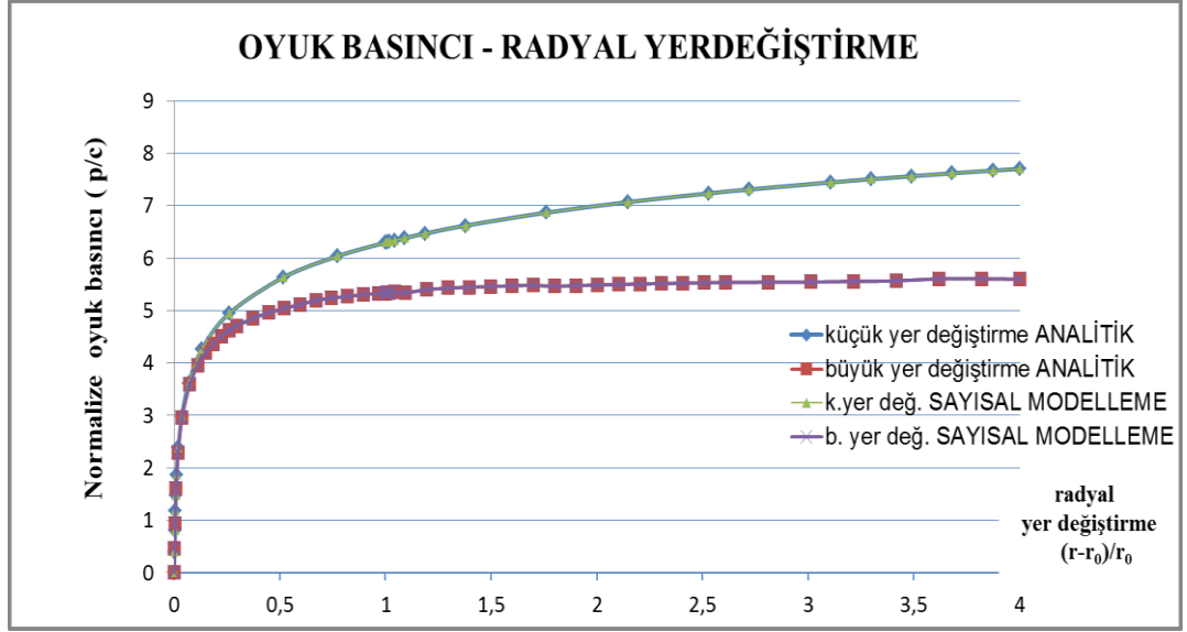
Şekil 5.13 : Oyuk basıncı radyal yerdeğiştirme ilişkisi.
