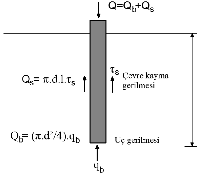
Şekil 3.4 : Zemin içerisinde eksenel yüklü çakma kazığı
