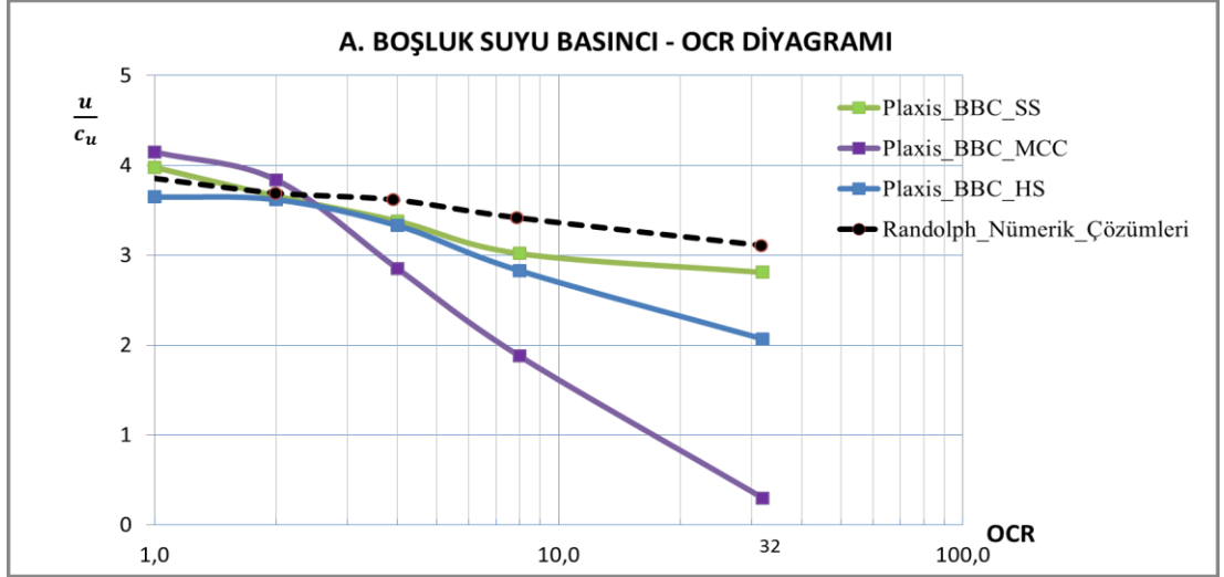
Şekil 6.8 : Oyuk yanındaki artık boşluk suyu basıncı ( c_u ile normalize edilen) AKO ilişkisi.
