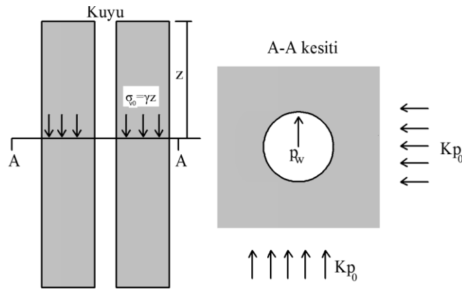
Şekil 3.17 : Düşey bir kuyu görünümü.
