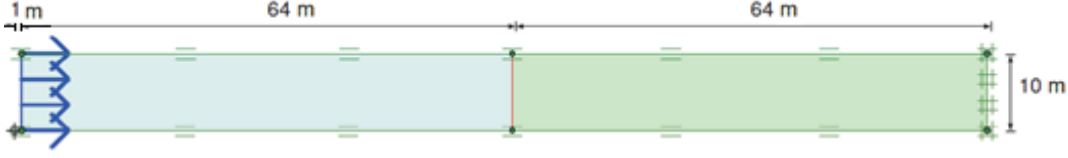
Şekil 5.18 : Oyuk genişlemesi problemi için model geometri özellikleri.
