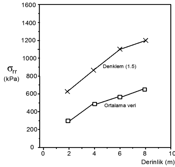
Şekil 3.7 : Aşırı konsolide Madingley killeri için kazık gövde normal gerilmesinin tahmini (Data verileri Coop ve Wrot, 1989).
