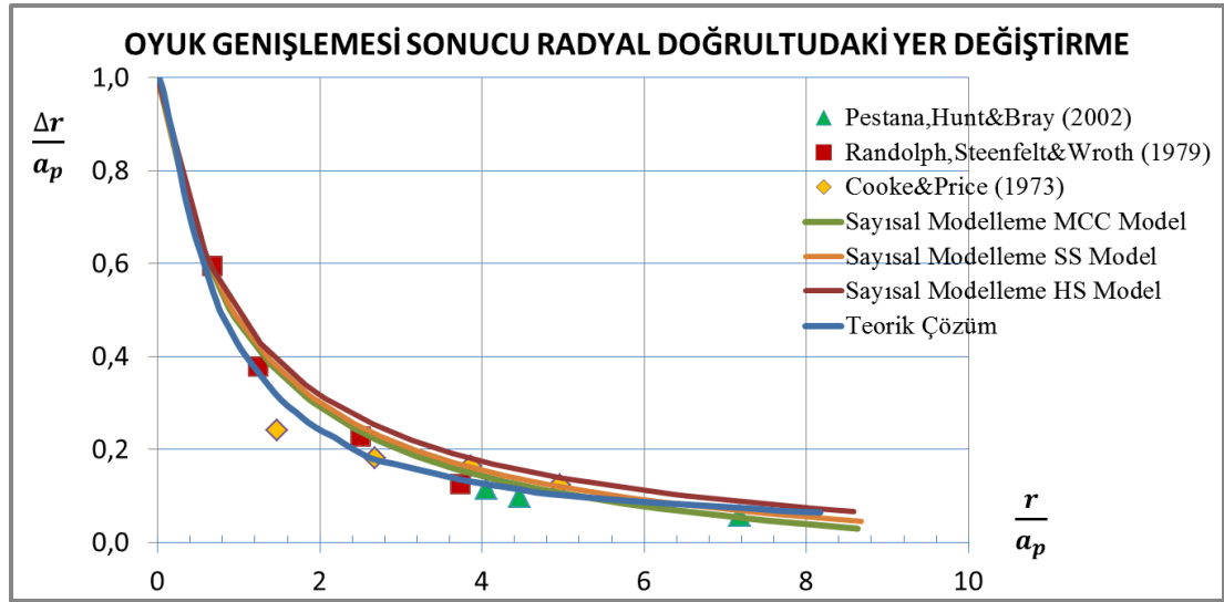
Şekil 6.1 : Sayısal modelleme sonuçları ile teorik ve ölçüme dayalı radyal doğrultudaki zemin deformasyonları karşılaştırmaları.
