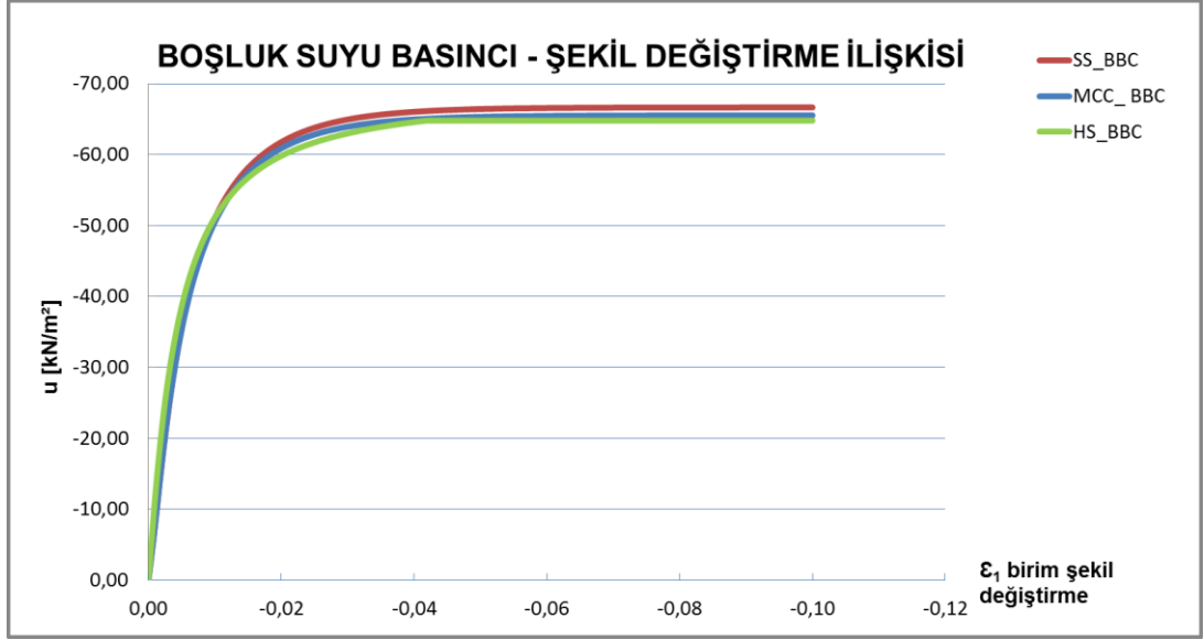
Şekil 5.16 : MCC, SS ve HS modellerden elde edilen boşluk suyu basıncı şekil değiştirme ilişkisi.
