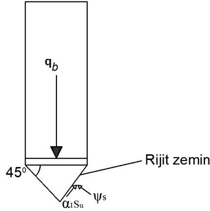
Şekil 3.8 : Drenajsız killerde küresel limit basıncı ile uç kapasite arasındaki ilişki.
