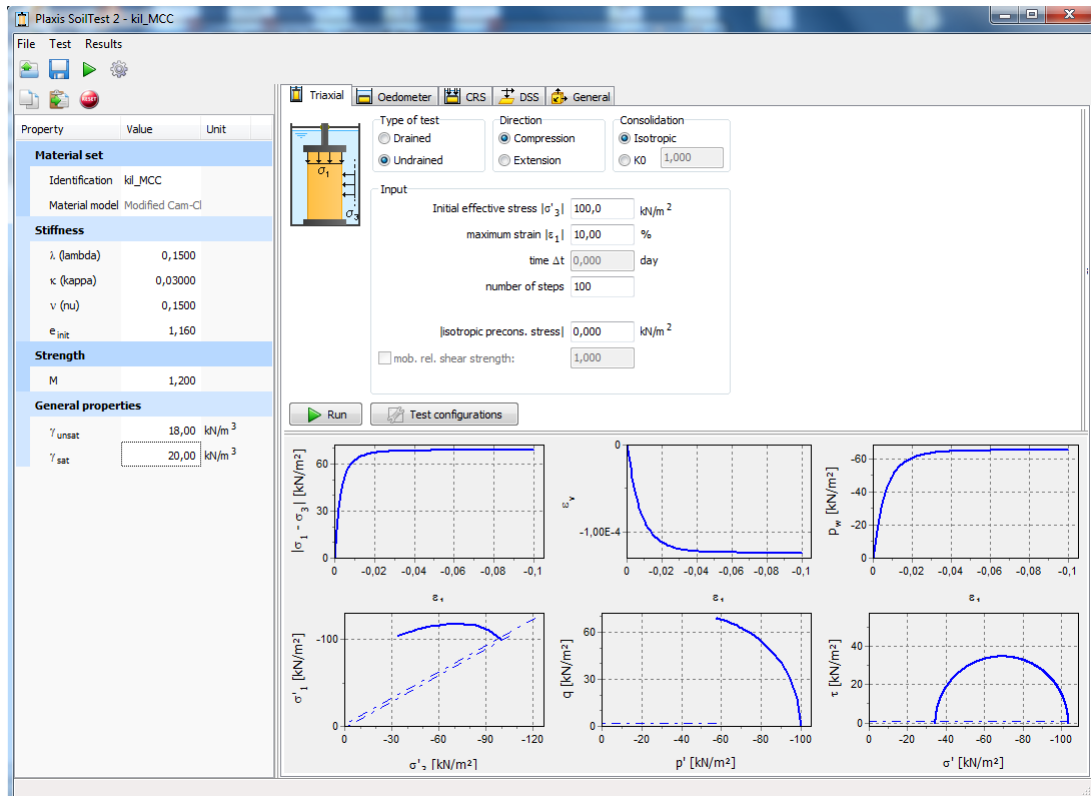
Şekil 5.14 : Boston Mavi Kili için MCC modelde Zemin Deneyi Modülü (Plaxis-Soil Test Module).
