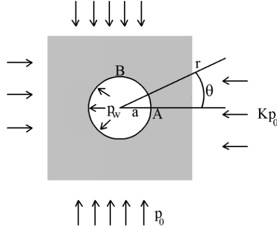
Şekil 3.18 : Hidrostatik olmayan arazi gerilmeleri altında kuyu problemi geometrisi.
