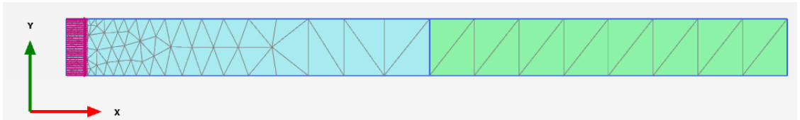
Şekil 5.11 : Oyuk genişlemesi problemi sonlu elemanlar ağı.
