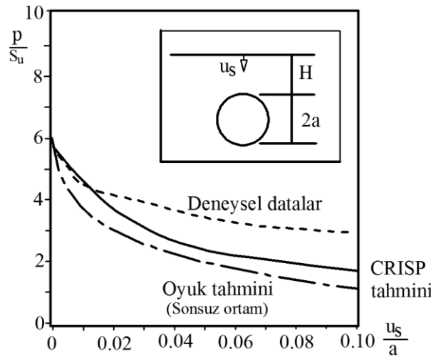
Şekil 3.14 : Tünel iç basıncının azalmasından dolayı tahmin edilen ve ölçülen yerdeğiştirmeler.
