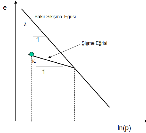
Şekil 4.2: Konsolidasyon karakterinin e - \ln (p) diyagramında gösterimi (Das, 2005).
