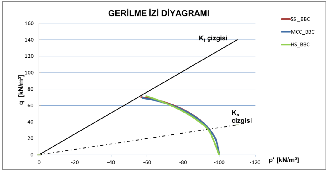
Şekil 5.17 : MCC, SS ve HS modellerden elde edilen gerilme izi diyagramı.
