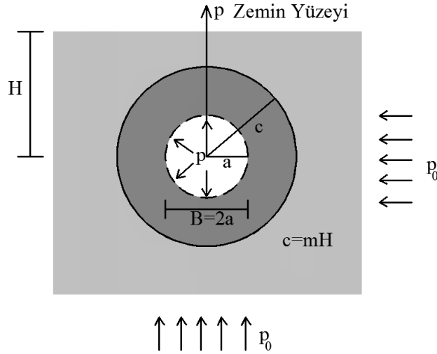
Şekil 3.9 : Ankraj plakasının geometrisi ve kırılma koşulları (Yu, 2000).
