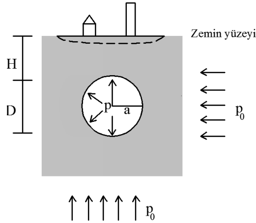
Şekil 3.12 : Zemin içerisindeki sıg tünel görünümü.
