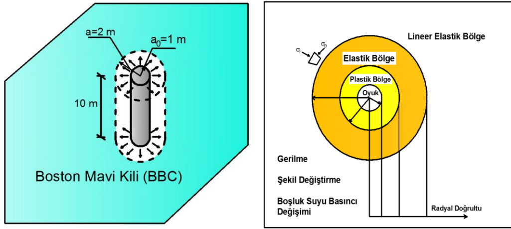
Şekil 5.1: Oyuk genişlemesi problemi geometrisi ve tanımı.
