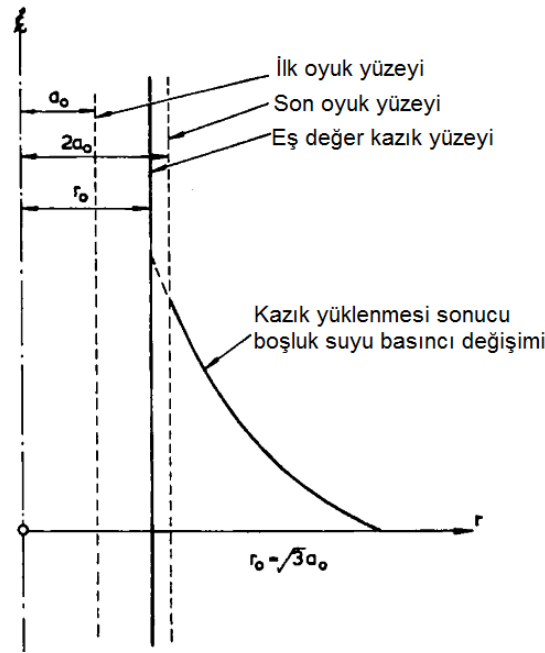
Şekil 5.4 : Kazık yüklemesinin oyuk genişlemesi problemi olarak modellenmesi (Carter vd. 1979).
