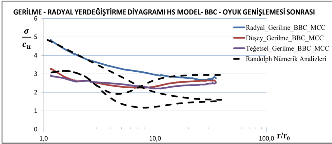
Şekil 6.7 : HS modeli için oyuk genişlemesi sonrasında meydana gelen gerilme radyal yer değiştirme diyagramı.
