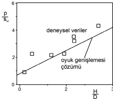
Şekil 3.16 : Deneysel ve teorik elde edilen tünel stabilite sonuçlarının karşılaştırılması (Yu, 2000).
