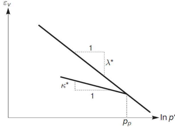
Şekil 4.4: Hacimsel birim şekil değiştirme-ortalama efektif gerilme logaritmik ilişkisi (Plaxis Manual 2D 2011).
