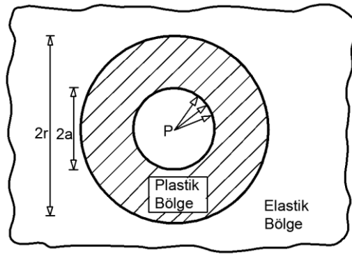
Şekil 5.9 : Silindirik oyuk genişlemesi.
