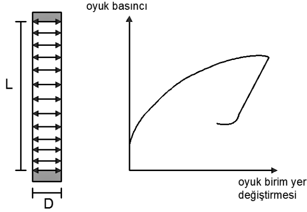
Şekil 3.1: Presiyometre çalışma mekanizması ve deney eğrisi (Yu, 2000).
