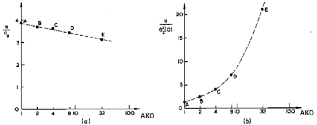
Şekil 5.6 : Kazık yüzü yanındaki artık boşluk suyu basıncı- Randolph vd. (1979a).
