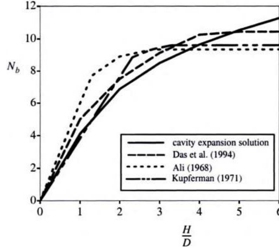
Şekil 3.10 : Yuvarlak ankrajlar için deneysel veriler ile karşılaştırma (Yu, 2000).
