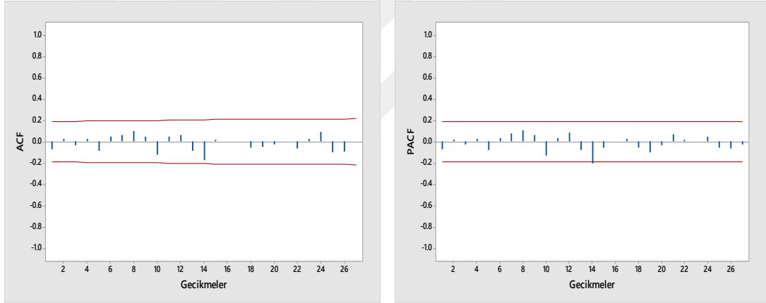
Şekil 4.5. ARIMA (5, 1, 3) modeli için artıkların ACF ve PACF grafiği
