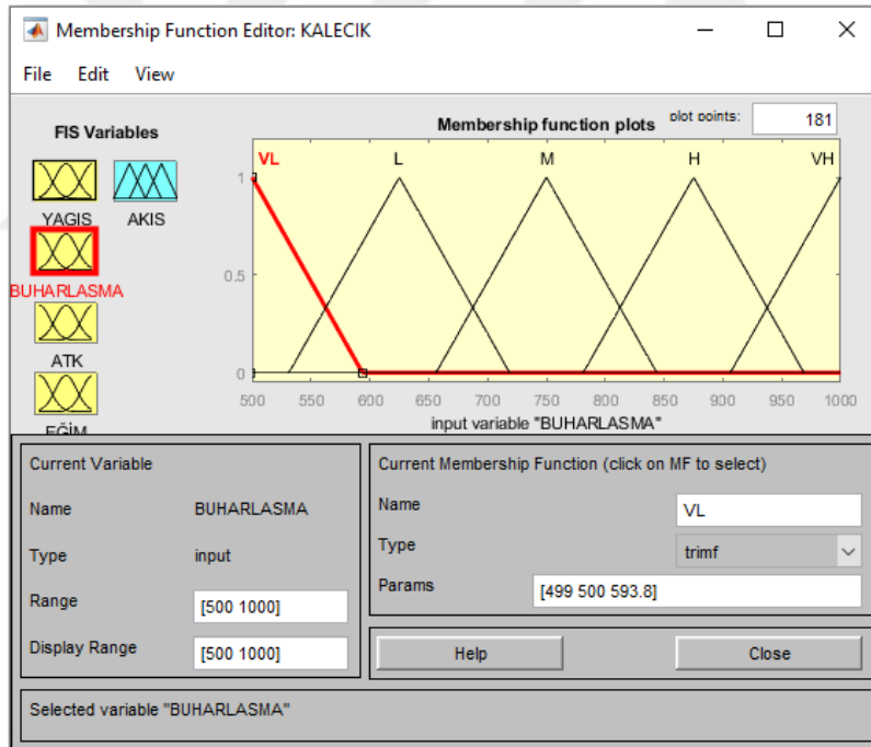
Şekil 4.5. Buharlaşma girdisine ait bulanık kümelerin görünümü
