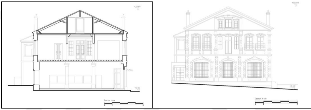
a-Kesit
