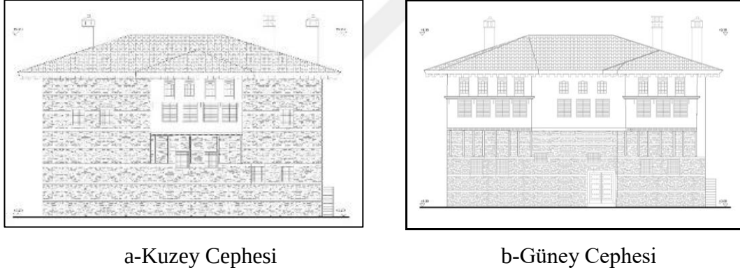
Şekil 4. 136. Poulkos Konağı Cephe Görünümleri
