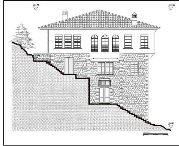
b- Güney Cephesi
