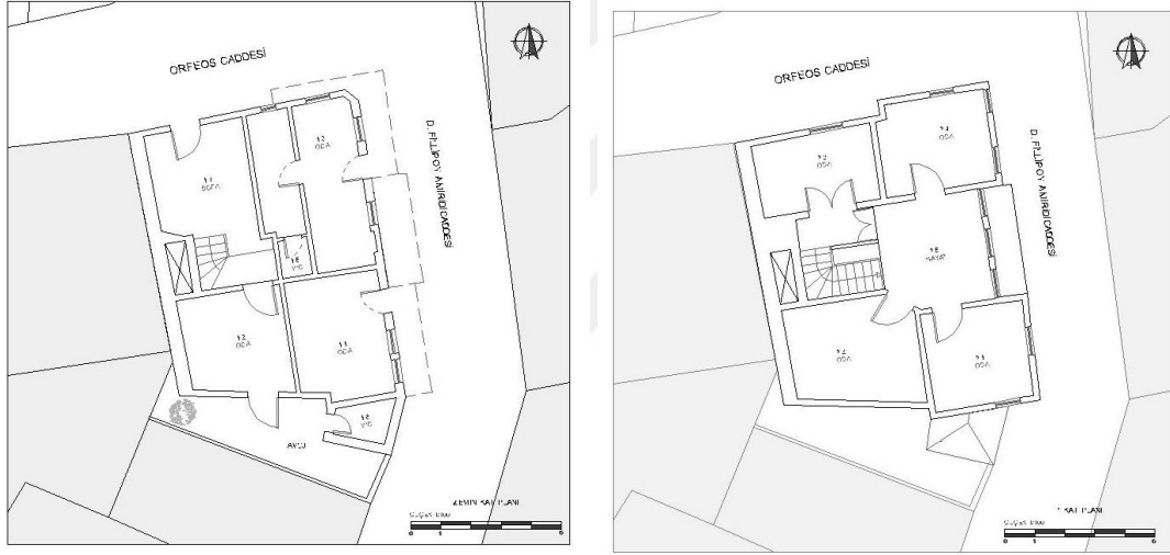
a-Zemin Kat Planı
