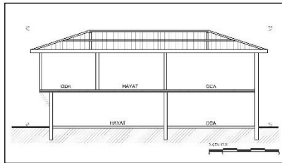
a-Kesit
