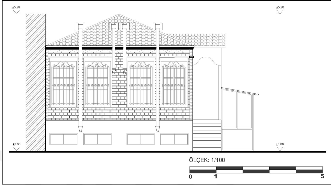
c- Güneydoğu Cephesi
