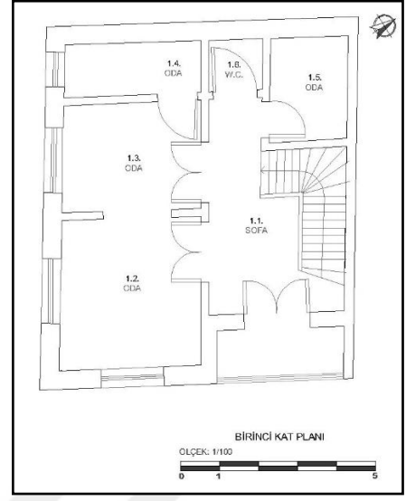
b- Birinci Kat Planı
