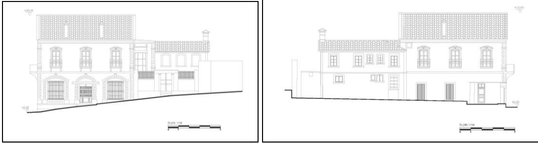
c-Kuzeydoęu Cephesi
