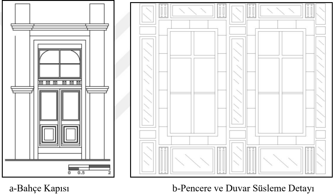
Şekil 3. 61. Anna Kaloudi Evi Detay Çizimleri
