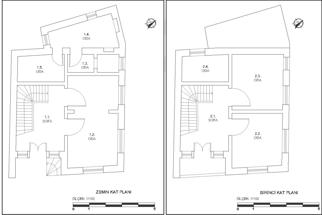
a-Zemin Kat Planı
