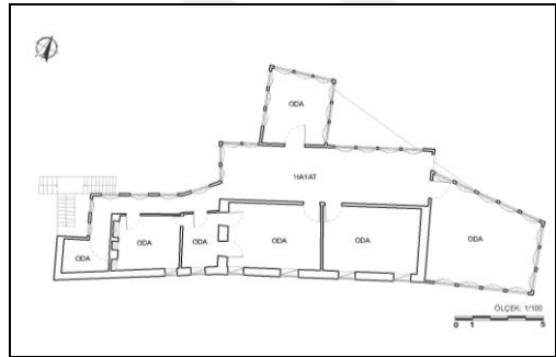
c-Birinci Kat Planı
