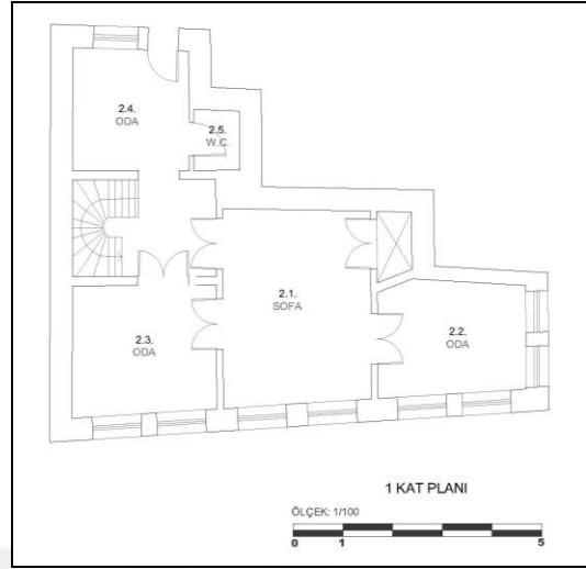
b-Birinci Kat Planı
