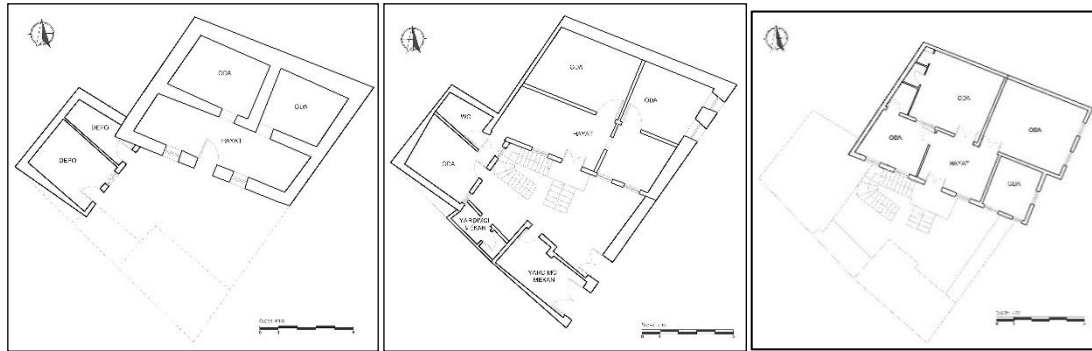
a- Bodrum Kat Planı
