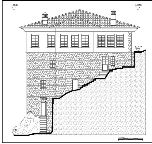
a- Kuzey Cephesi
