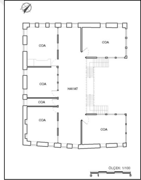
b- Birinci Kat Planı
