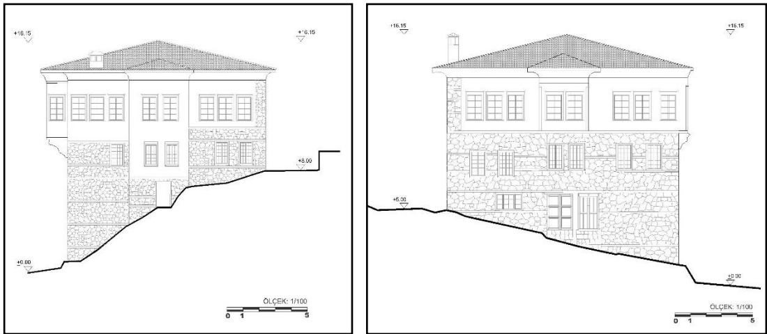
a-Doğu Cephesi
