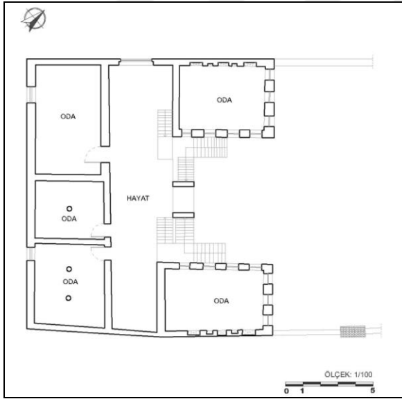
a-Zemin Kat Planı
