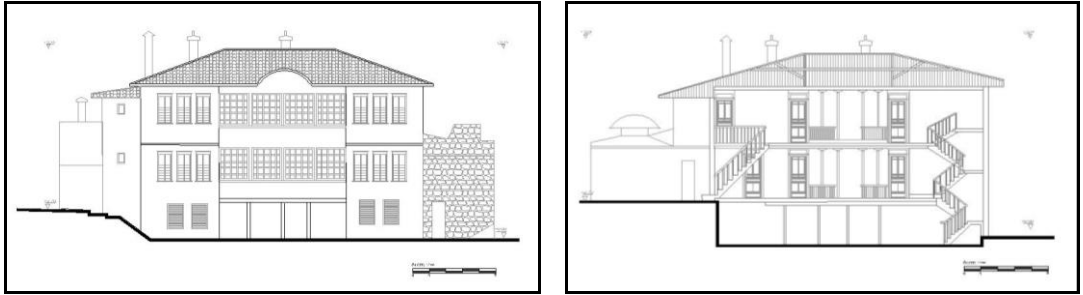
Şekil 3. 31. Salihoğlu Konağı Güney Cephesi 11 Şekil 3. 32. Salihoğlu Konağı Kesiti 12
