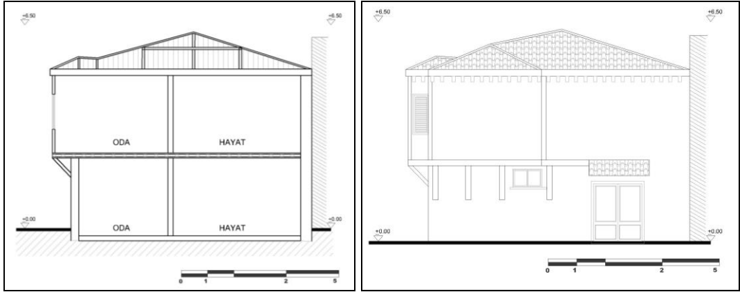
a-Kesit
