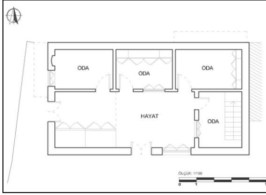
a-Zemin Kat Planı
