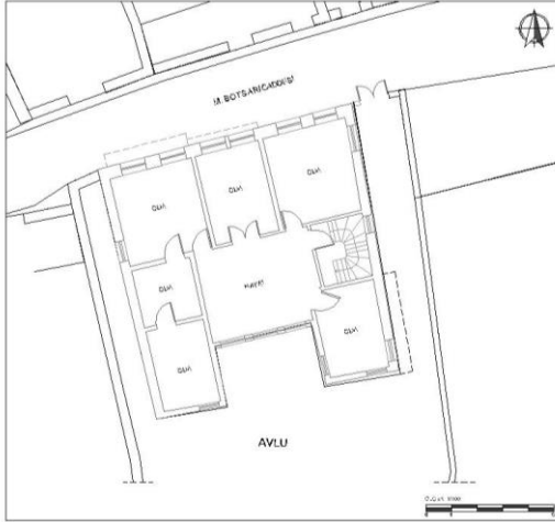
a-Zemin Kat Planı
