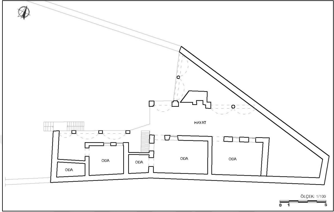
a-Zemin Kat Planı
