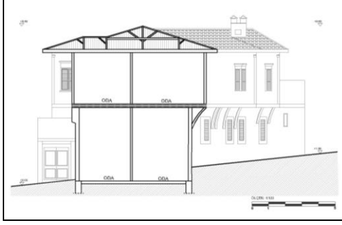
a- Kesit
