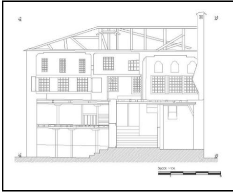
a-A-A Kesiti
