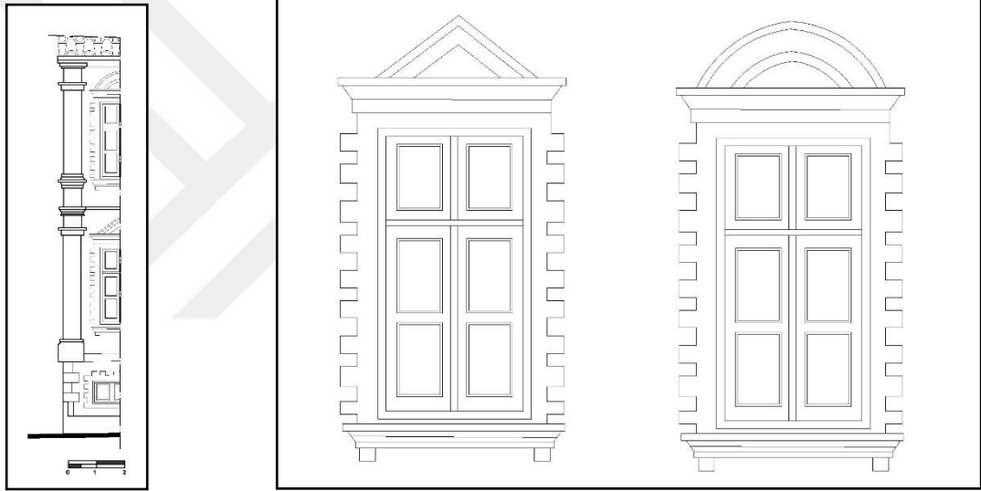
Şekil 3. 71. Kuyumcuoğlu (Kougioumtzoglou) Evi Pencere ve Cephe Detayları
