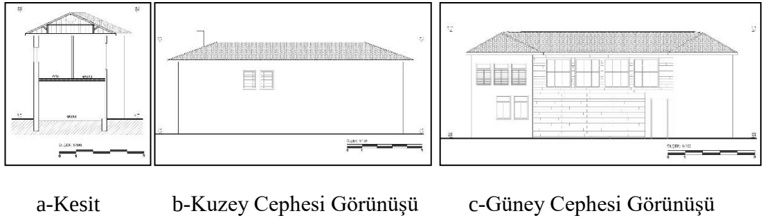
Şekil 3. 133. Yunus Ağa Evi Kesit ve Görünüşleri
