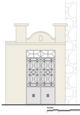
a-Ana Giriş Kapısı ve Detay Çizimi
