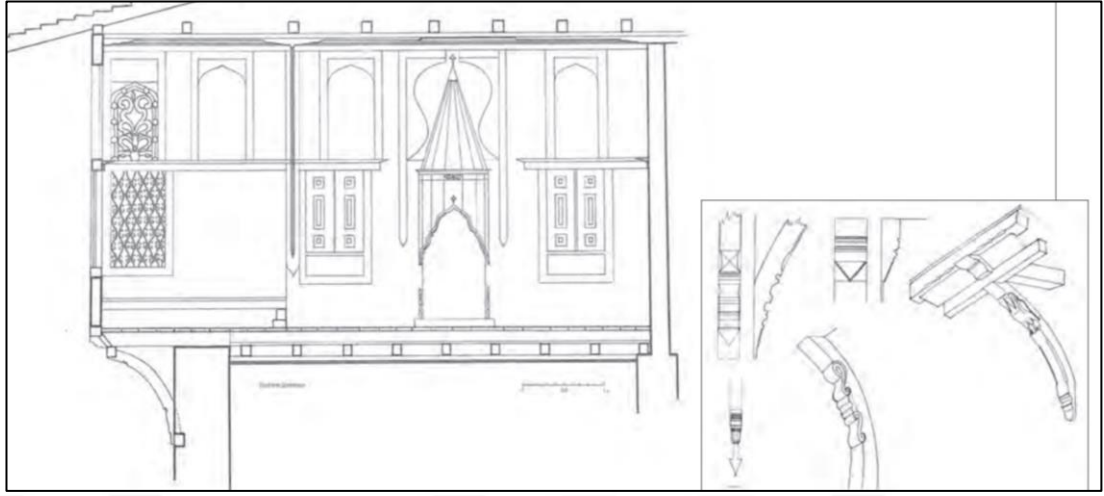
Şekil 5. 75. Vourkas Konağı Ocak ve Detaylar (Pasxalidou-Moreti) 106
