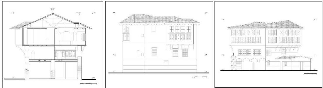
a-Kesit
