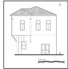
c- Kuzey Cephesi Görünümü
