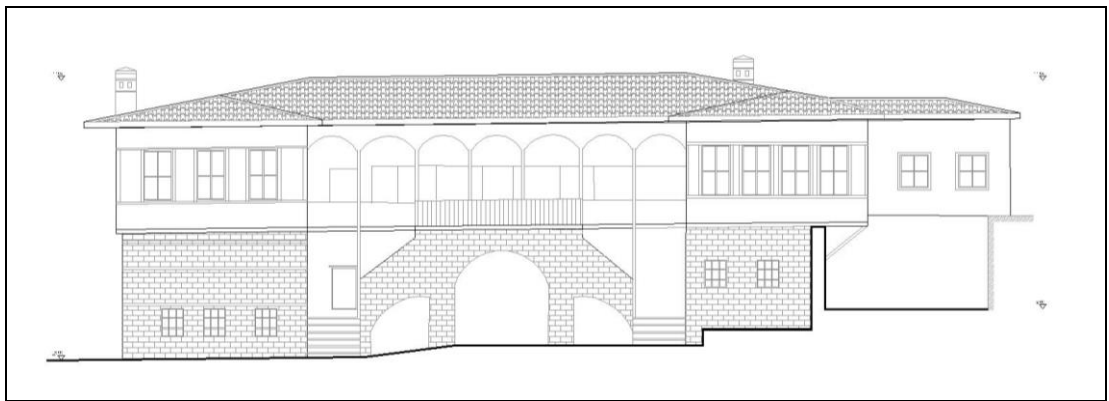
Şekil 5. 15. Hayrettin Paşa Evi Görünüşü 88
