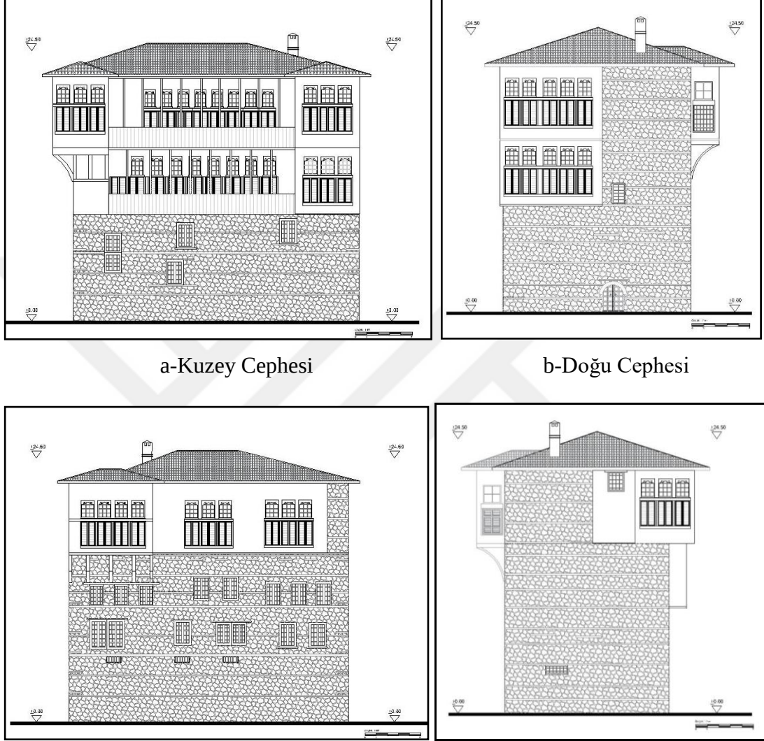
c-Güney Cephesi
