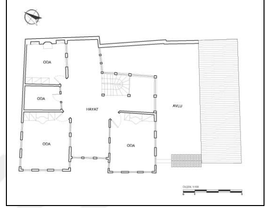
b-Birinci Kat Planı
