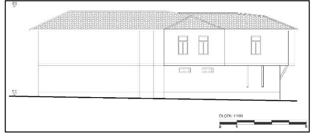
b-Kuzeybatı Cephesi
