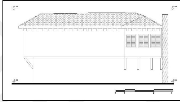
c- Kuzey Görünüşü
