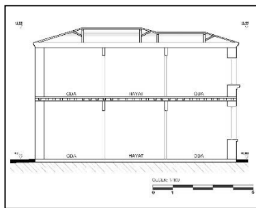
a-Kesit
