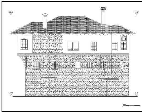
d-Batı Cephesi
