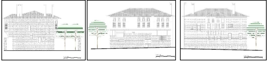
a-Doğu Cephesi
