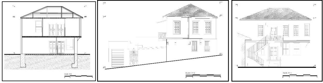
a-Kesit
