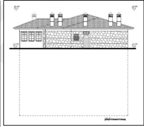
d-Doğu Cephesi
