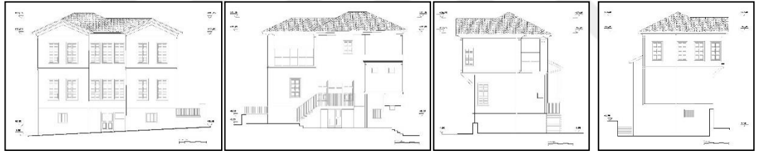
a-Güneydoğu Cephesi b-Kuzeybatı Cephesi c-Kuzeydoğu Cephesi d-Güneybatı Cephesi
