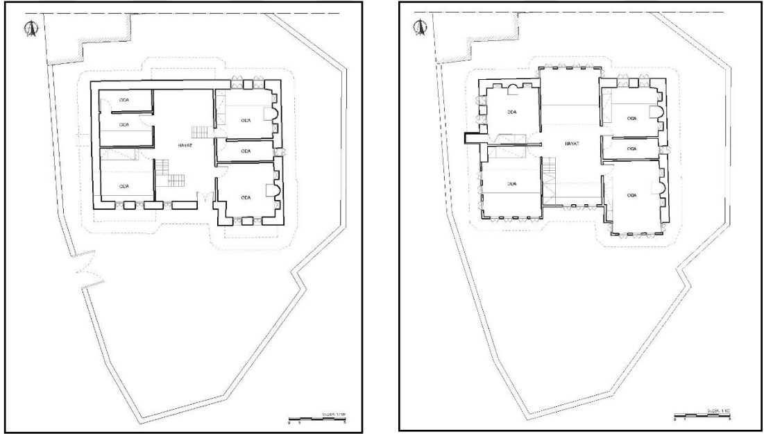
a-Zemin Kat Planı
