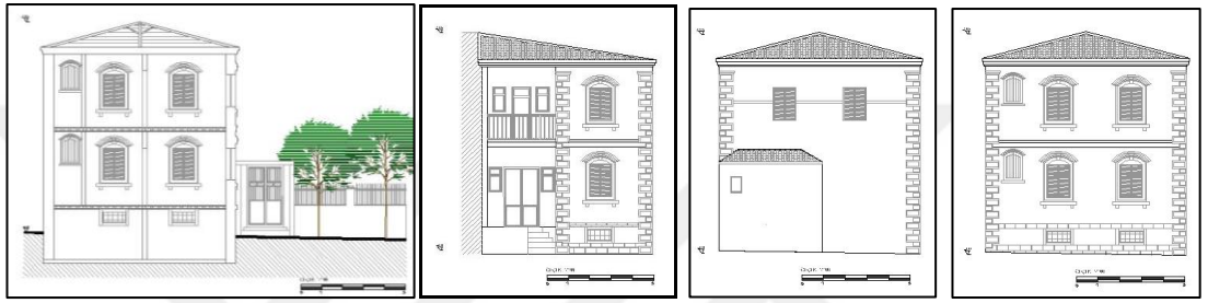
a-Kesit b-Güneydoğu Cephesi c-Kuzeybatı Cephesi d-Kuzeydoğu Cephesi
