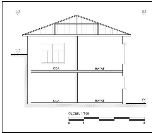
a-Kesit
