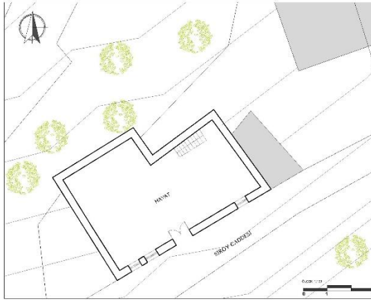
a-Zemin Kat Planı
