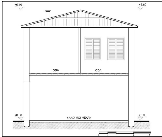
a-Kesit
