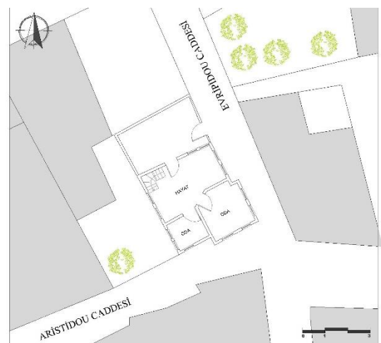
b-Birinci Kat Planı
