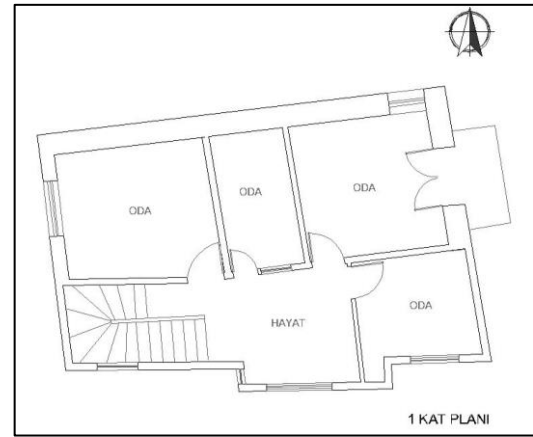
b-Birinci Kat Planı
