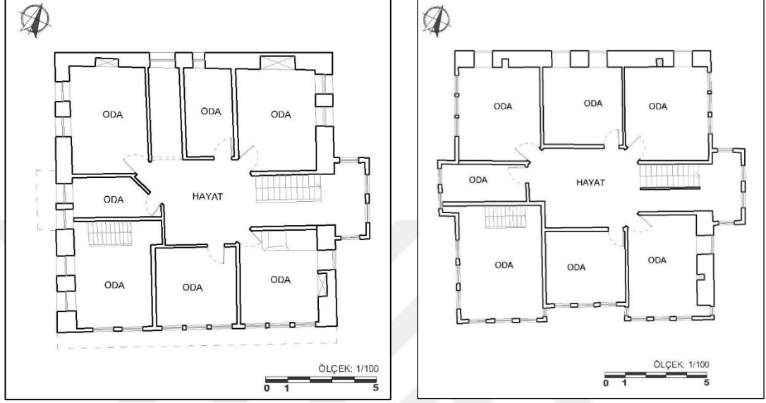
a--Birinci Kat Planı
