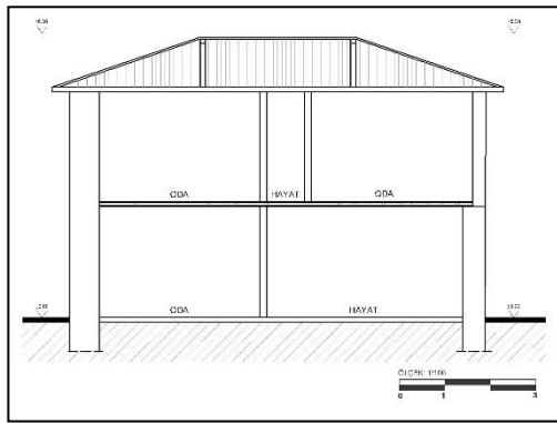
a-Kesit
