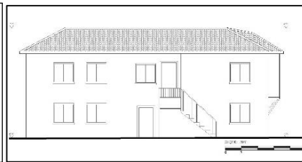
b-Batı Cephesi
