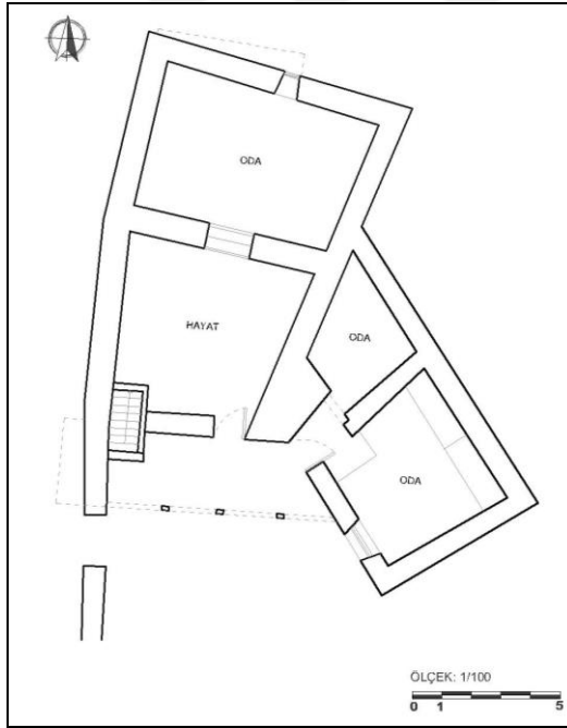
a-Zemin Kat Planı
