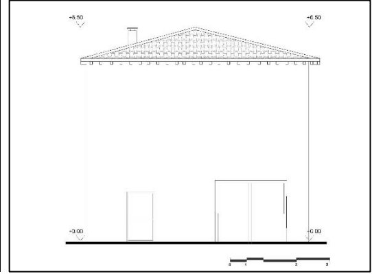
d- Batı Cephesi
