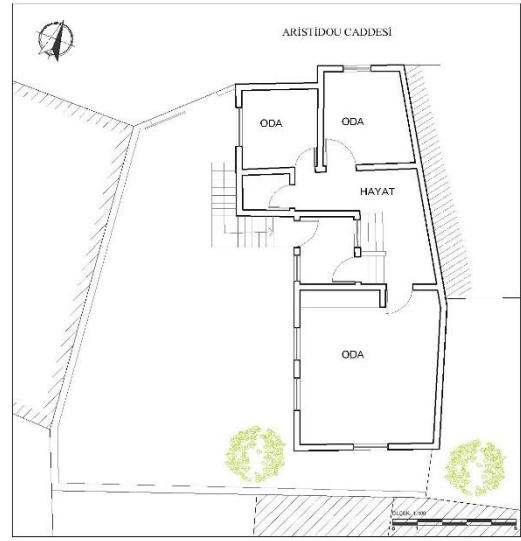
b-Birinci Kat Planı
