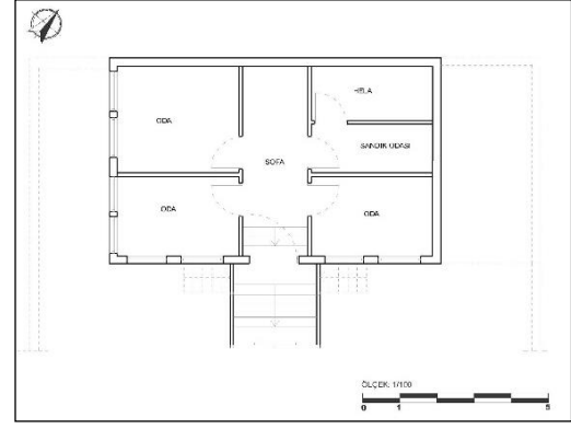
b-Bodrum Kat Planı
