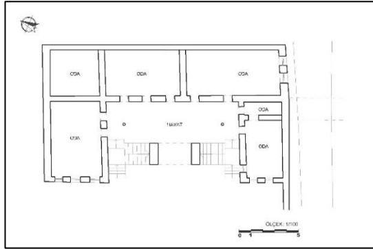
a-Zemin Kat Planı
