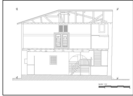
b-B-B Kesiti
