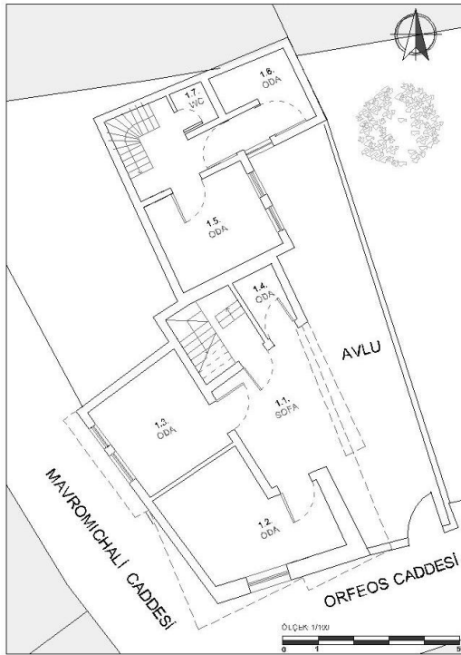
a- Zemin Kat Planı
