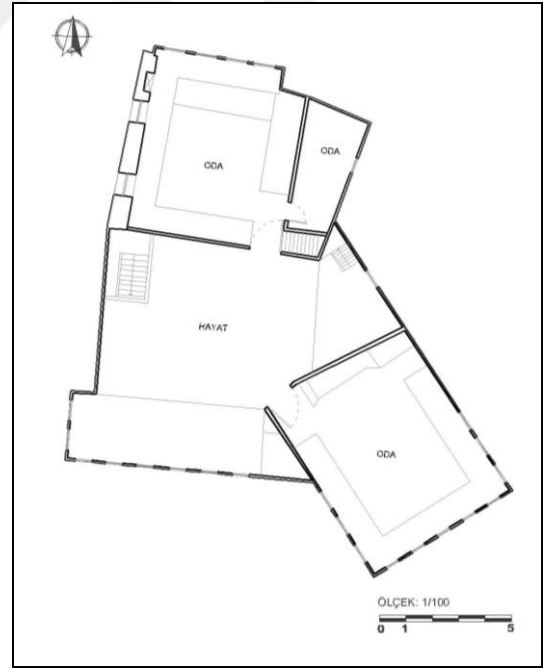
b-Birinci Kat Planı
