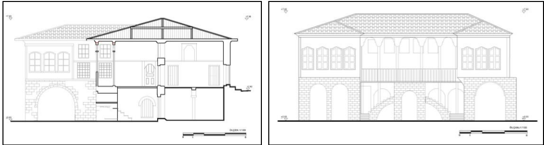
Şekil 5.6. Hüseyin Bey Evi Görünüş ve Kesiti 84 (Loukanis, 1977)
