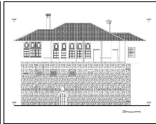
e-Doğu Cephesi
