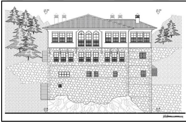
c- Batı Cephesi
