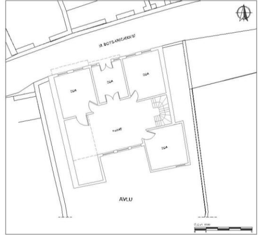
b- Birinci Kat Planı
