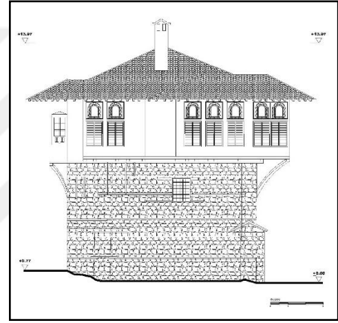
d-Güney Cephesi
