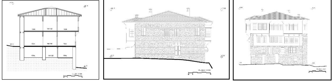
a-Kesiti
