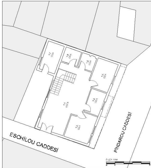
a-Zemin Kat Planı
