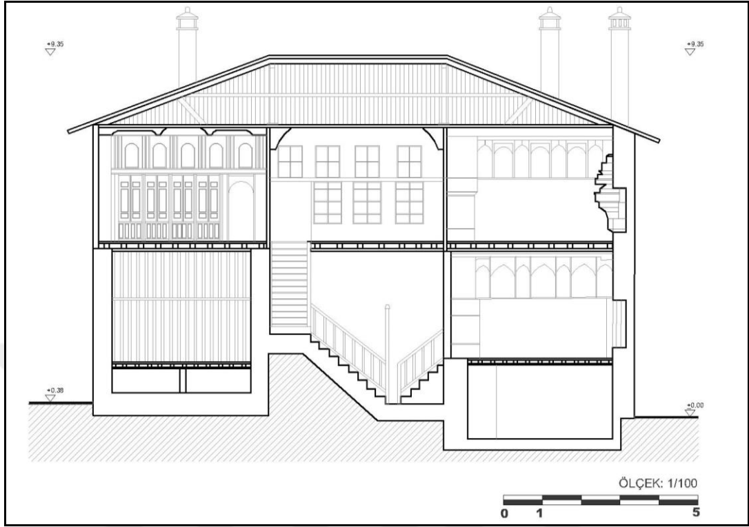
Şekil 4. 120. Poulkos Konağı Kesiti
