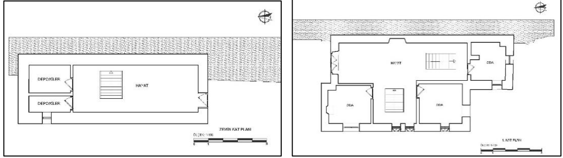
a-Zemin Kat Planı 46
