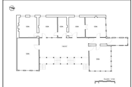
b-Birinci Kat Planı
