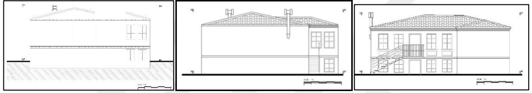
a-Kesit
