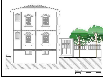
a-Kesit
