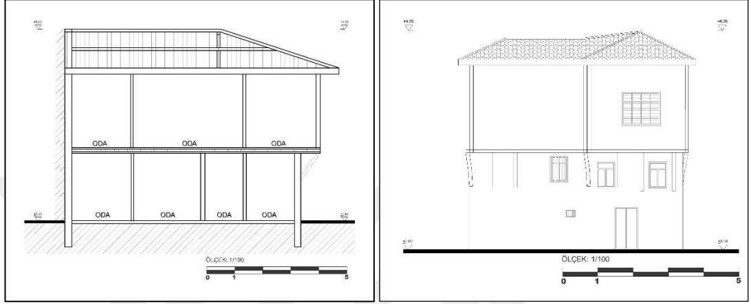
a-Kesit
