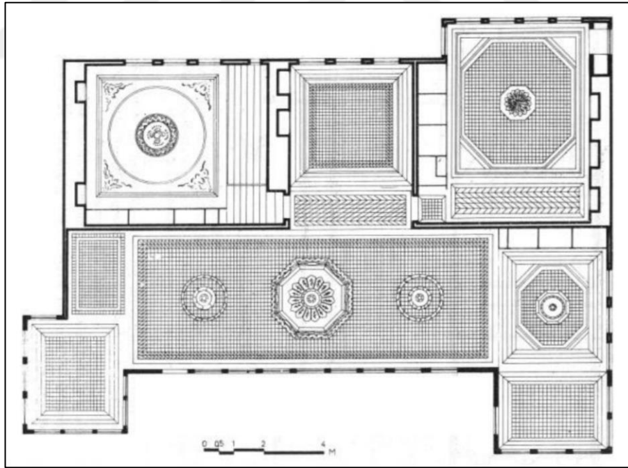
Şekil 4. 50. Tsatsapa Konağı İkinci Kat Tavan Planı (Moutsopoulou,1966)
