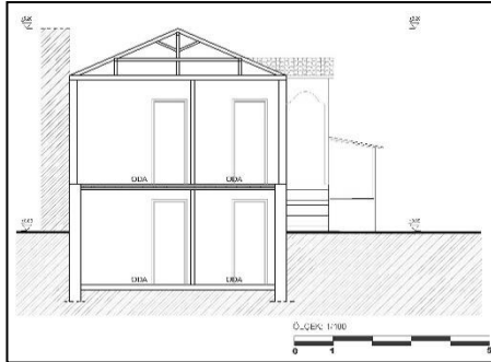
a-Kesit
