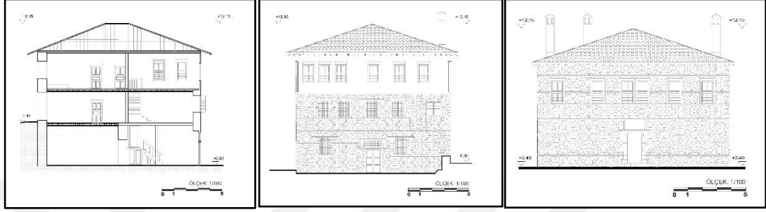
a-Kesit
