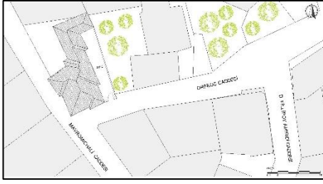
Şekil 3. 46. Mavromichali Cad. Evi Vaziyet Planı 14
