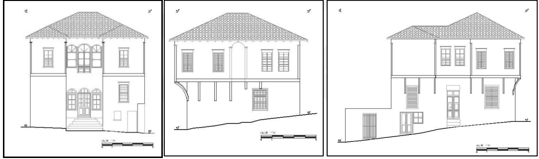
a-Güneydoğu Cephesi
