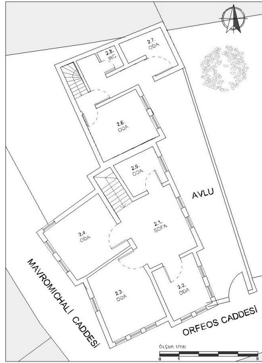
b- Birinci Kat Planı
