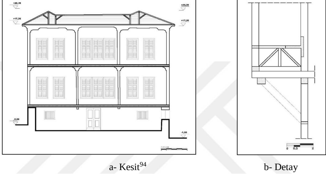
Şekil 5. 47. Atatürk Evi Kesit ve Detay
