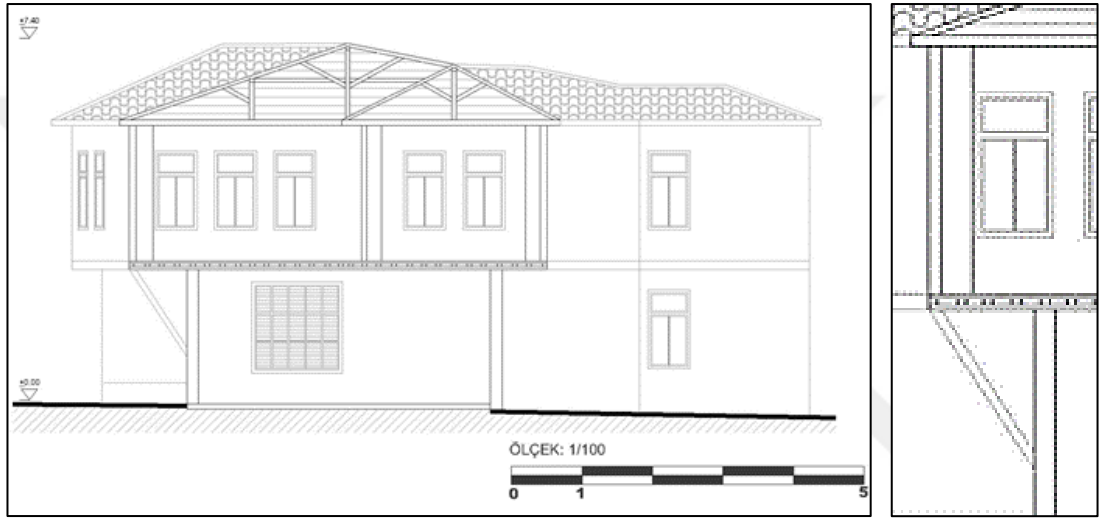
a- A-A Kesiti
