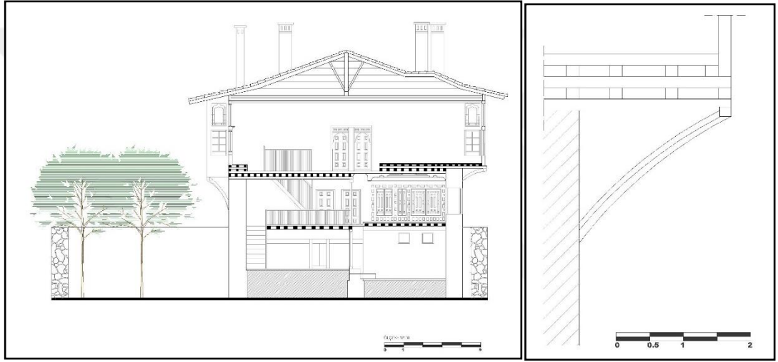
a-A-A Kesiti
