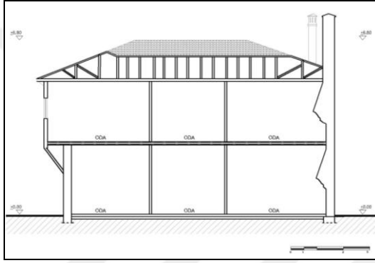
a-Kesit
