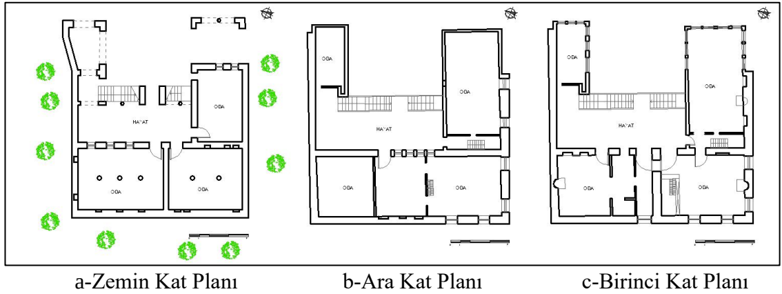
Şekil 5. 5. Hüseyin Bey Evi Kat Planları 83
