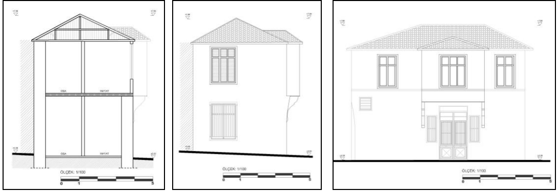
a-Kesit
