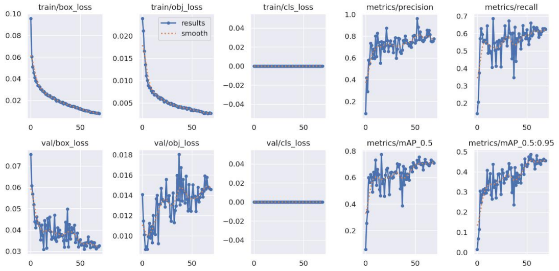
Şekil 9.1. Eğitim aşamanın loss ve doğruluk grafikleri.
