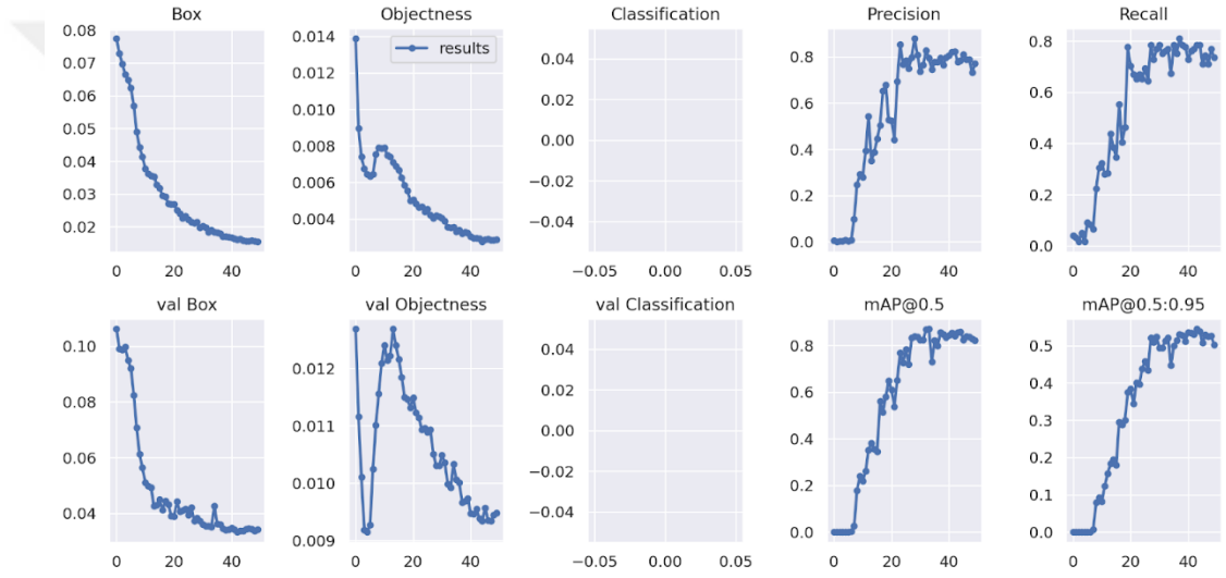
Şekil 9.8. Eğitim aşamanın loss ve doğruluk grafikleri.
