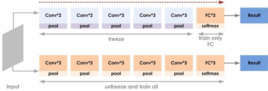
Şekil 8.11. Ön eğitilmiş modelden öğrenme aktarması işlemi sırasında tüm konvolüsyon katmanlarının dondurulması ve yalnızca üst katmanların eğitimi gerçekleşmektedir [179].
