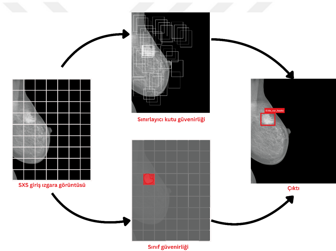
Şekil 8.3. YOLO’nun çalışma prensibi.
