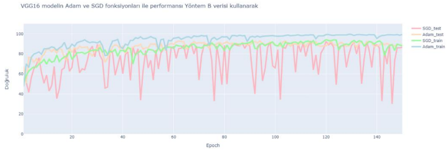
Şekil 10.6. VGG16’nın Yöntem A ve Yöntem B veri setleri üzerinde SGD ve Adam optimizier’larla eğitim ve test doğruluk grafikleri. a) Yöntem A, b) Yöntem B.
