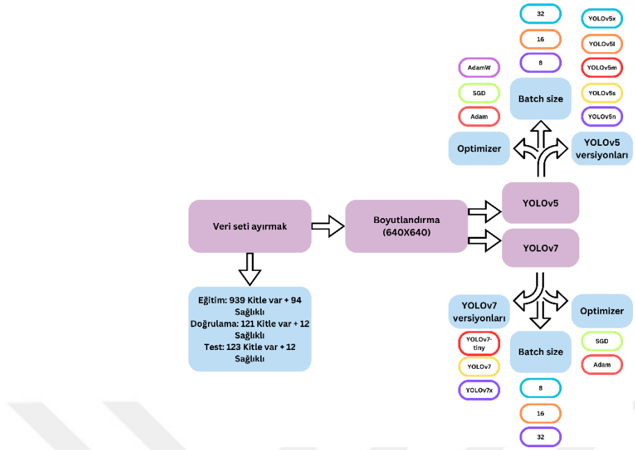
Şekil 8.7. YOLO uygulamasının akış diyagramı.
