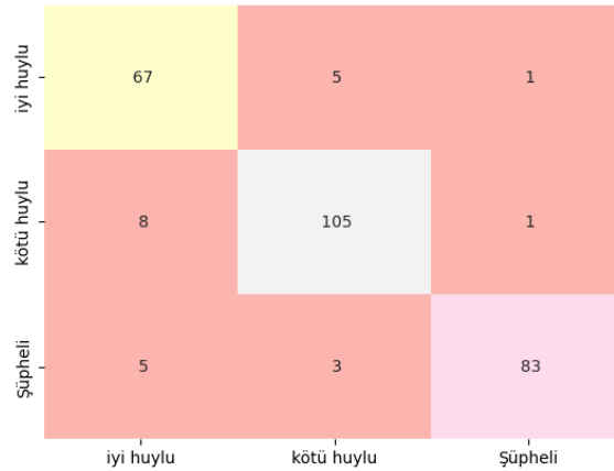
Şekil 9.32. Karışıklık matrisi.
