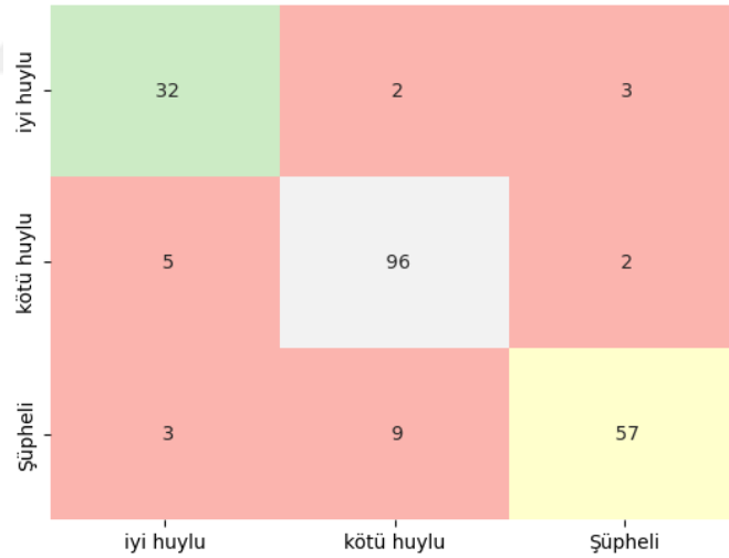
Şekil 9.30. Karışıklık matrisi.
