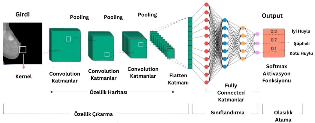
Şekil 8.10. CNN mimarisi [178].
