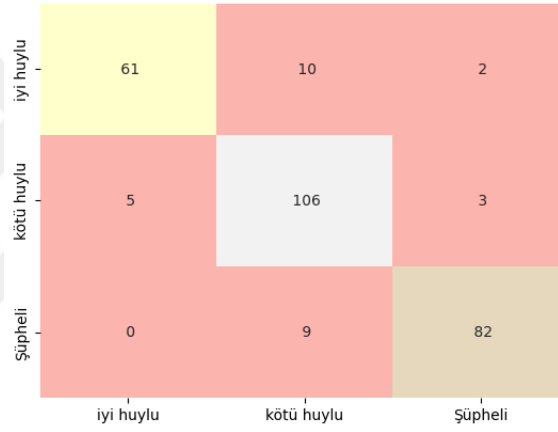
Şekil 9.28. Karışıklık matrisi.
