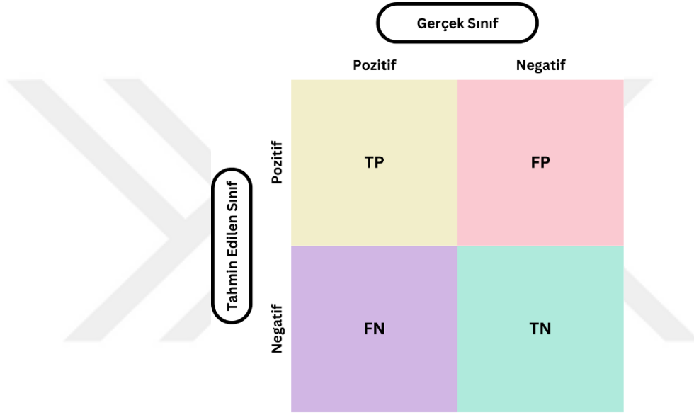
Şekil 8.17. Karışıklık matrisi.
