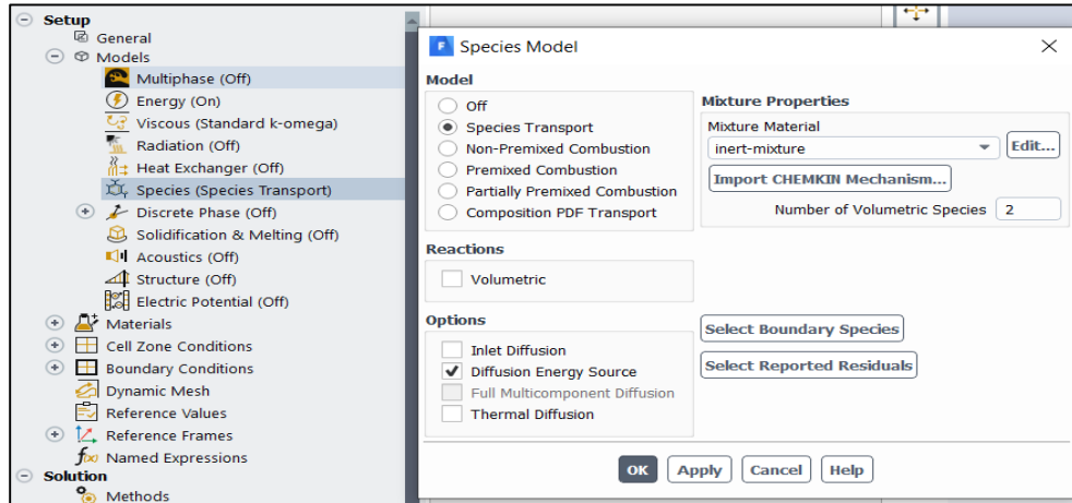
Şekil 3. 9. Analizin gaz karışımı tipinin seçilmesi
