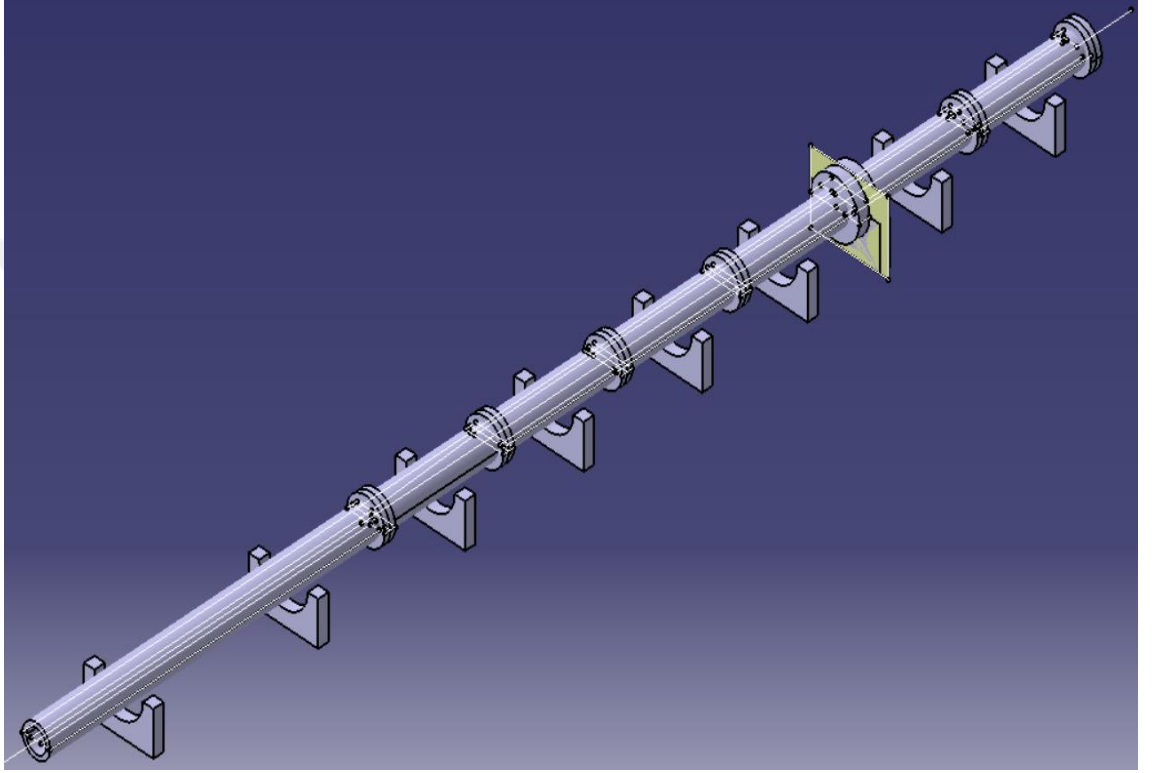
Şekil 3. 1. CFD analizlerini doğrulamak için kullanılan deneysel verilerin ait olduğu şok tüpünün CAD görüntüsü
