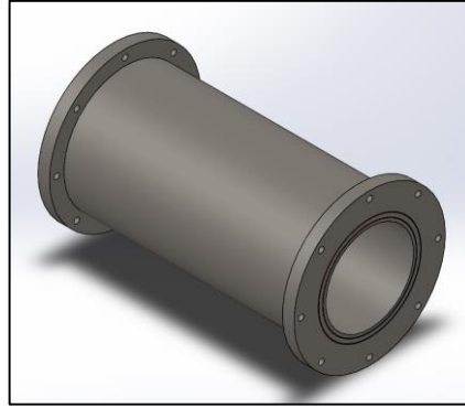
Şekil 3. 35. Şok tüpü ön basınç bölgesi tasarımı
