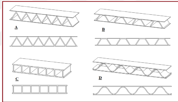
Şekil 2. 9. Farklı geometrilerde oluklu çekirdek yapıya sahip sandviçler
