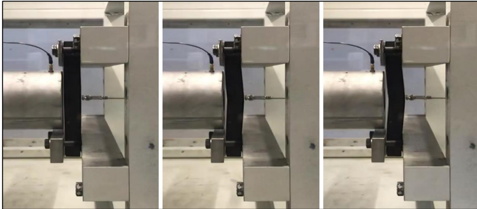
Şekil 4. 3. EPP köpük çekirdek yapıli sandviçin şok tüpü testindeki zamana bağıli deęişim görüntüsü
