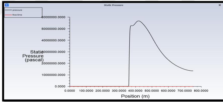
Şekil 3. 23. Analiz sonucunda elde edilen basınç grafiği
