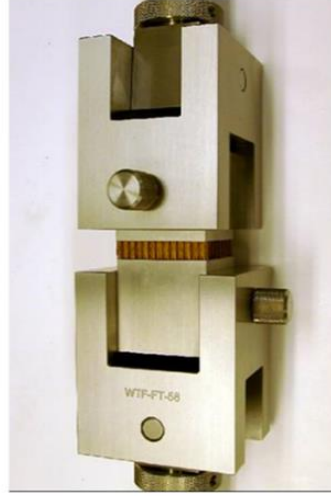
Şekil 2. 16. Çekme testi (ASTM C297)
