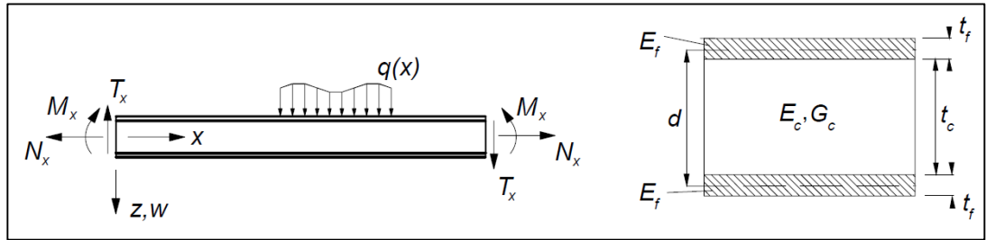
Şekil 2. 20. Sandviç kiriş için işaretlerin belirlenmesi (Zenkert 1995)
