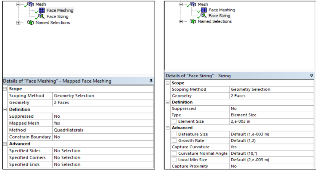
Şekil 3. 4. Mesh özellikleri
