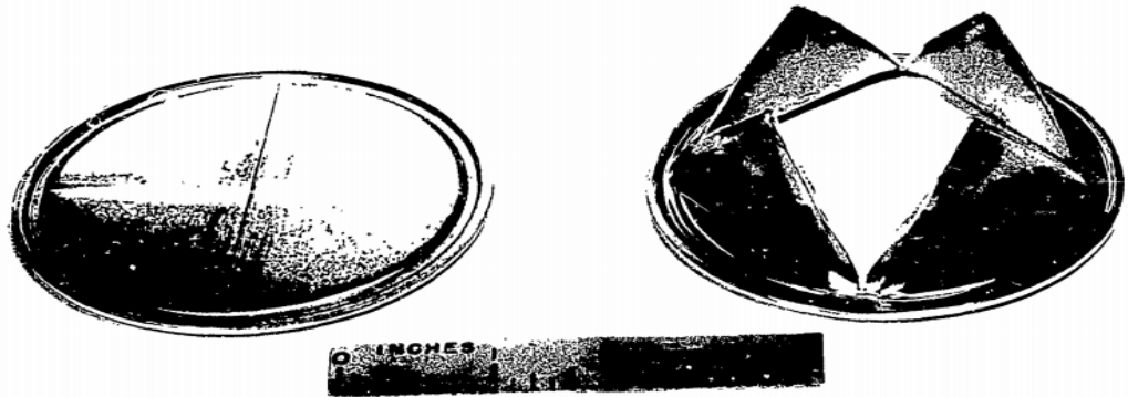
Şekil 2. 33. Patlamadan önce ve sonra diyafram örneği (Wright 1961).
