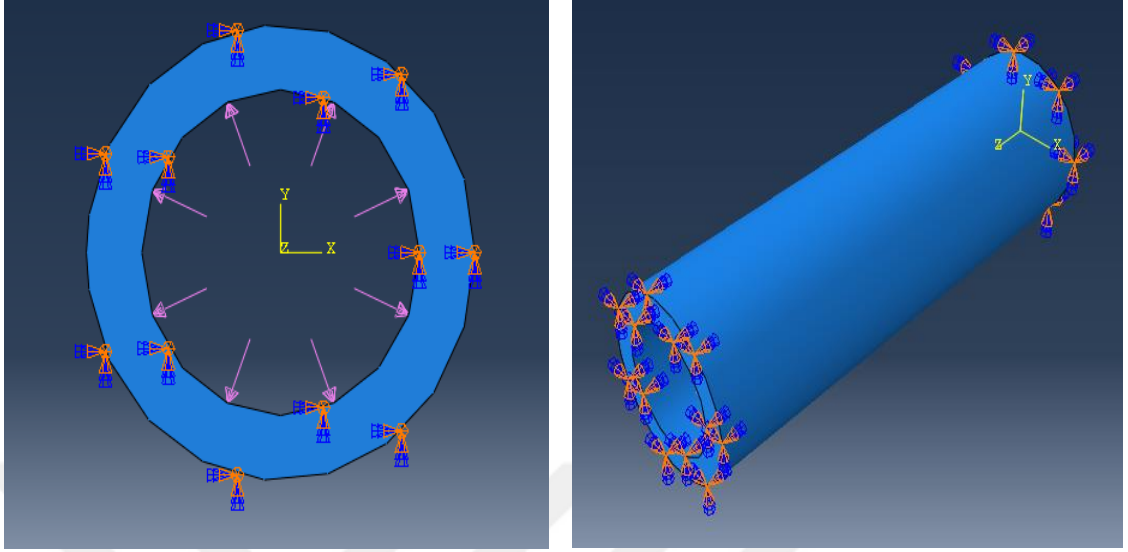
Şekil 3. 28. Parça 2'nin analiz başlangıç şartlarının gösterimi
