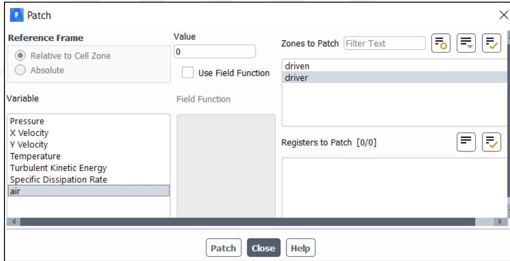
Şekil 3. 19. Analizin başlangıç şartlarının girilmesi 3
