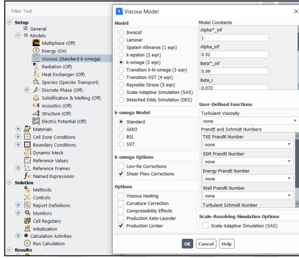
Şekil 3. 8. Analizin akış tipinin seçilmesi
