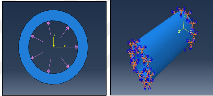
Şekil 3. 26. Parça 1'in analiz başlangıç şartlarının gösterimi
