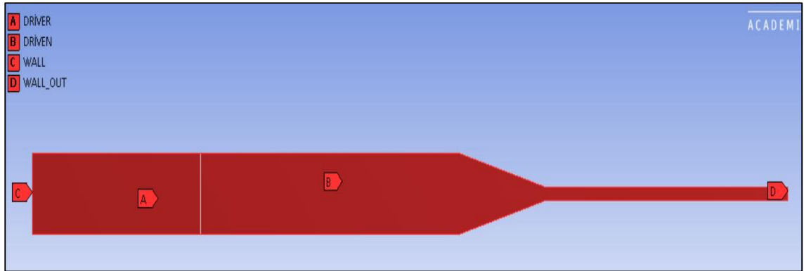
Şekil 3. 5. 2D modelin bölgeleştirilmesi
