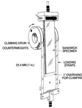
Şekil 2. 17. Yapışma testi (soyma uygulaması) (ASTM D1781)
