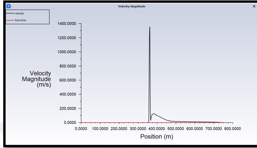
Şekil 3. 24. Analiz sonucunda elde edilen hız grafiği
