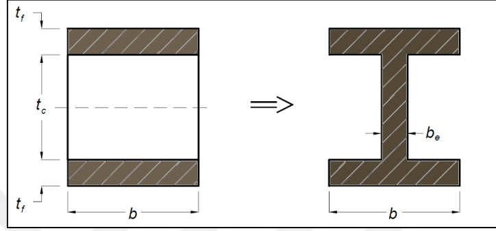
Şekil 2. 24. Sandviç yapı ve I-kirişin eşdeğer ağ genişliği (Zenkert 1995)
