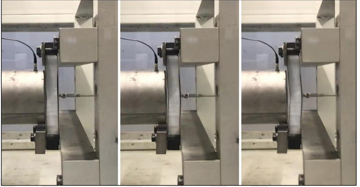
Şekil 4. 6. XPS köpük çekirdek yapılı sandviçin şok tüpü testindeki zamana bağlı değişim görüntüsü
