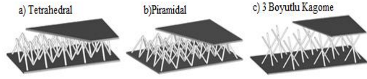
Şekil 2. 11. Farklı geometrilere kafes kiriş çekirdek yapılar
