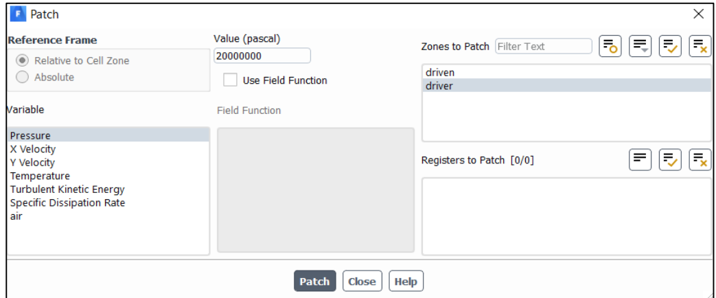
Şekil 3. 17. Analizin başlangıç şartlarının girilmesi 1
