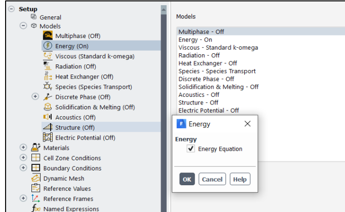
Şekil 3. 7. Analiz enerji modülünün aktif edilmesi
