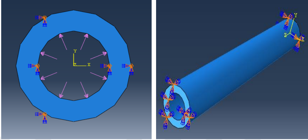
Şekil 3. 32. Parça 4'ün analiz başlangıç şartlarının gösterimi
