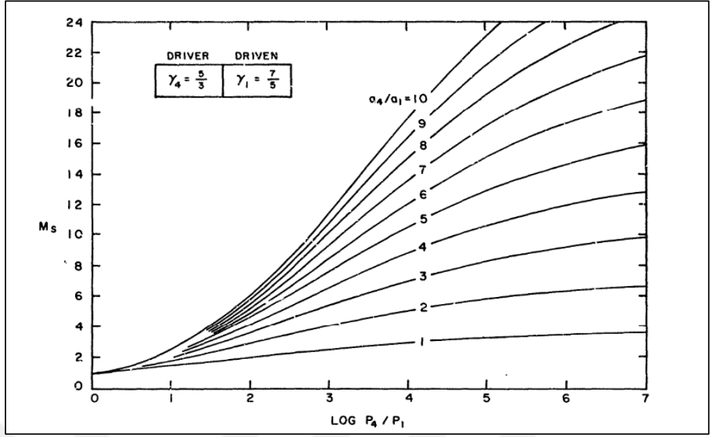
Şekil 2. 32. Çeşitli Basıncı Oranlarından Elde Edilen Mach Sayısı(Russo, A.L. and Hertzberg, A. 1958)
