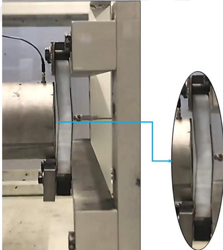
Şekil 4. 7. Şok testi sırasında malzemede oluşan deplasman (XPS köpük)
