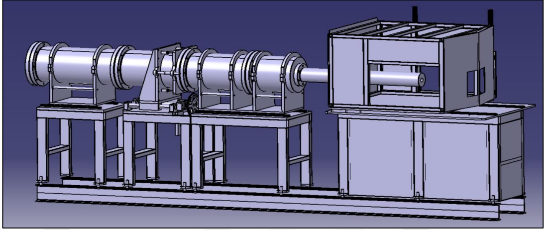
Şekil 3. 39. Şok tüpü son tasarımı
