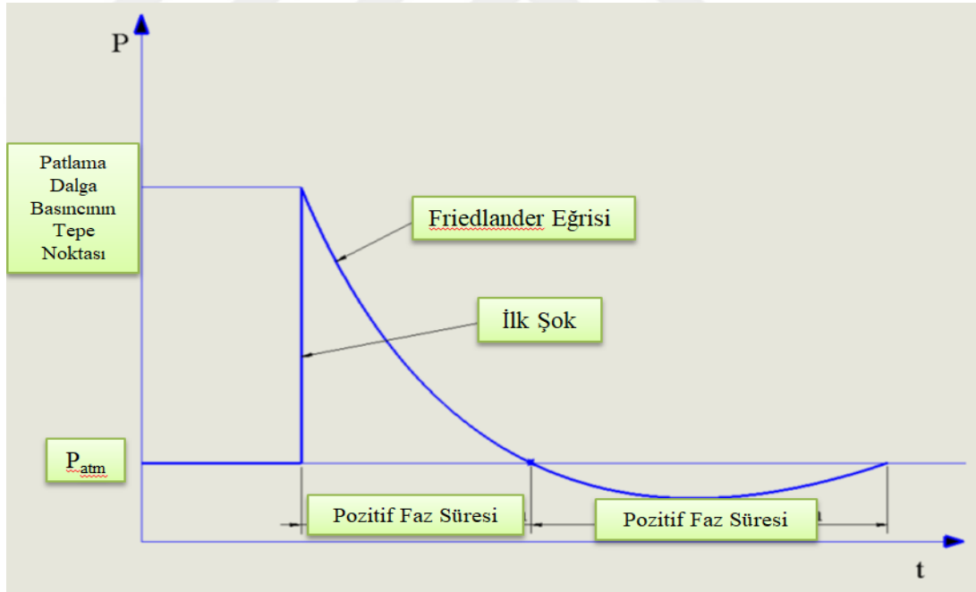
Şekil 2. 27. Friedlander ya da ideal patlama dalgaları (Saad 1993)
