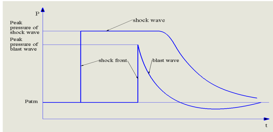
Şekil 2. 31. Şok dalgasının ve patlama dalgasının karşılaştırılması (Russo, A.L. and Hertzberg, A. 1958)
