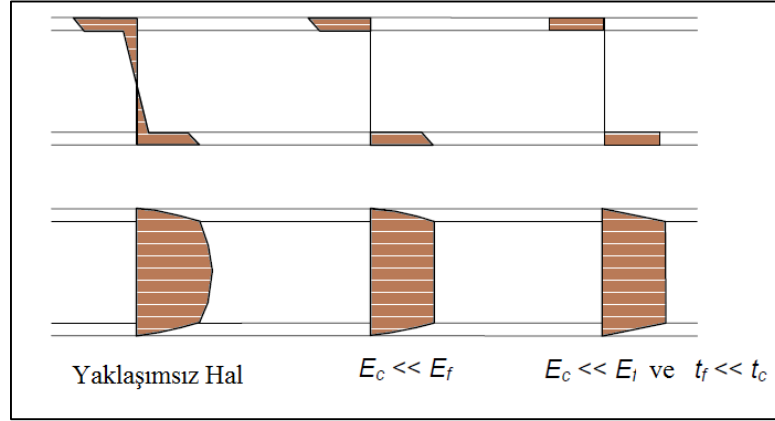
Şekil 2. 22. Farklı yaklaşım seviyeleri için normal ve kayma gerilmeleri (Zenkert 1995)
