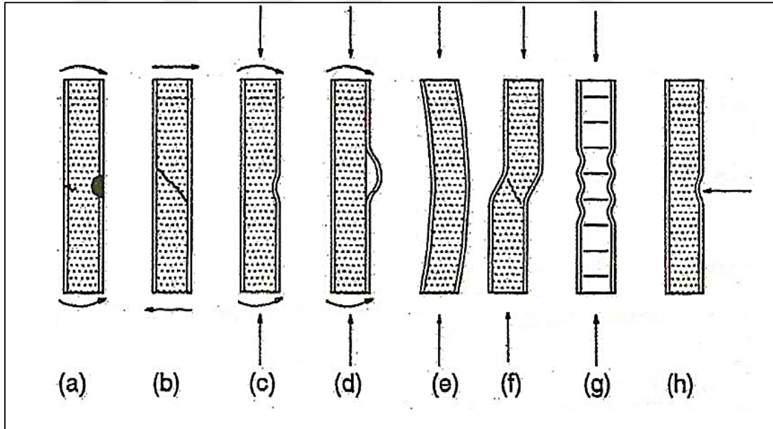
Şekil 2. 18. Sandviç kirişlerin en yaygın hasar modları
