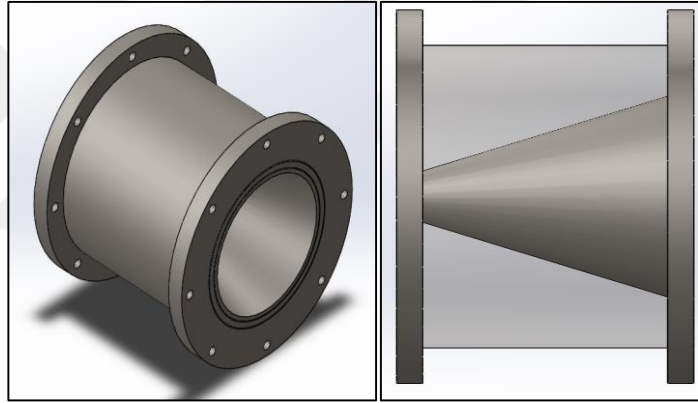
Şekil 3. 37. Şok tüpü akış bölgesi konik kısım tasarımı
