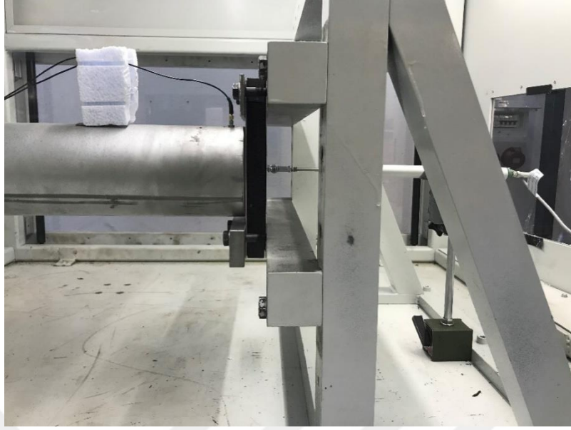
Şekil 3. 45. EPP köpük malzeme çekirdek yapısına sahip sandviç yapı test düzeneğine bağlanması
