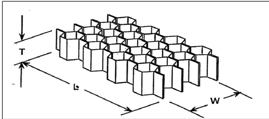
Şekil 2. 7. Balpeteği çekirdek yapının şerit yönleri (Türkoğlu 2020)
