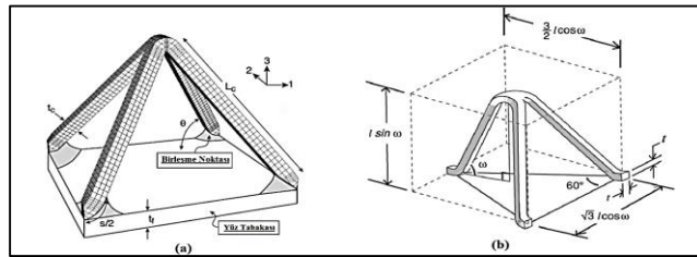
Şekil 2. 12. Tek hücreli kafes kiriş yapıların geometrileri
