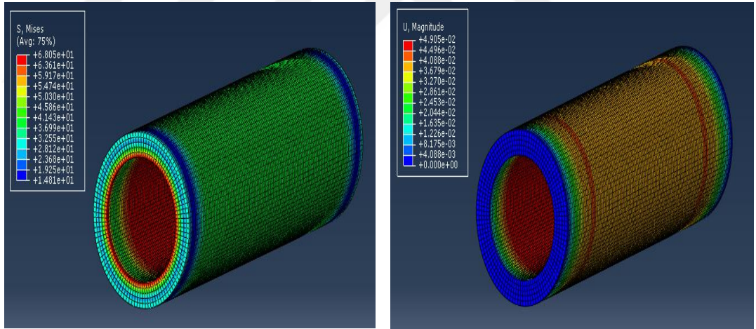
Şekil 3. 29. Parça 2'nin analiz sonuçları
