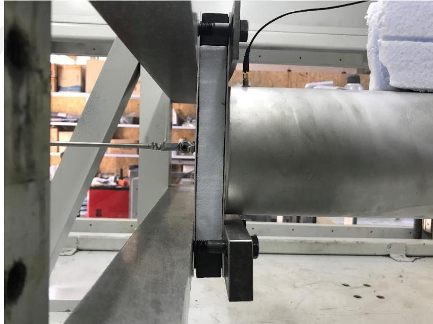
Şekil 3. 46. XPS köpük malzeme çekirdek yapısına sahip sandviç yapı test düzeneğine bağlanması
