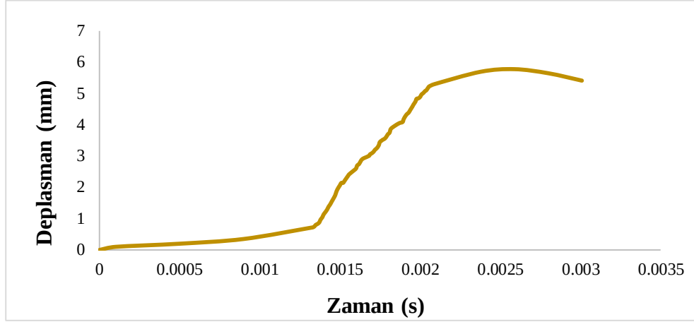
Şekil 4. 8. XPS köpük çekirdek yapısına sahip sandviç yapının arka plakasının şok testi sonucunda oluşan deplasman-zaman grafiği
