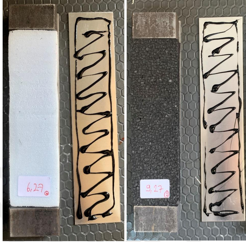
Şekil 3. 42. Yapıştırıcı sürülen yüzey plakaları
