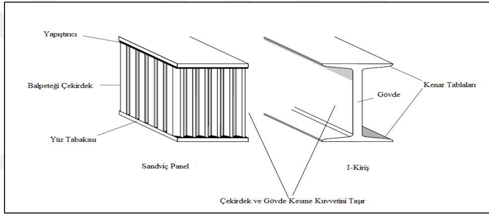
Şekil 2. 4. Temel prensip olarak sandviç yapı ve I kiriş (Türkoğlu 2020)
