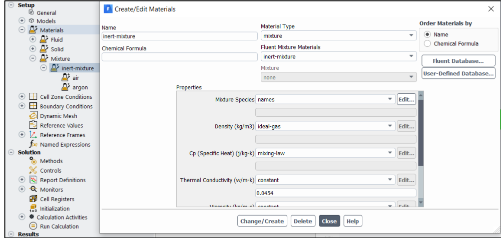
Şekil 3. 12. Analizde kullanılan materyallerin değerlerinin seçilmesi 2
