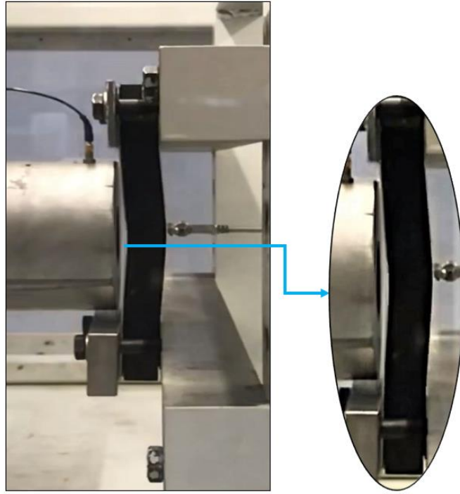
Şekil 4. 4. Şok testi sırasında malzemede oluşan deplasman (EPP köpük)
