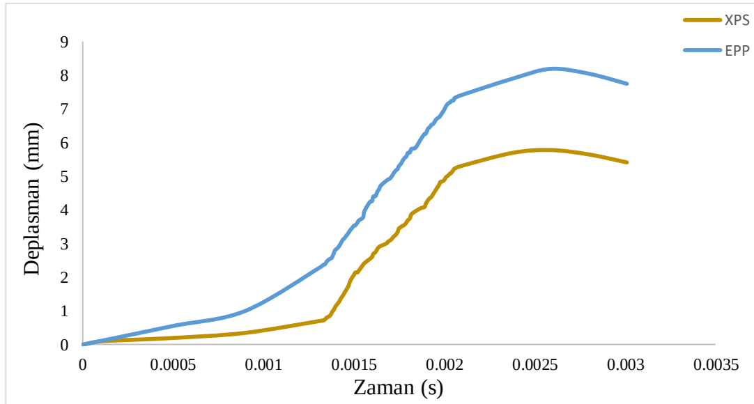
Şekil 4. 9. XPS ve EPP köpük çekirdek yapısına sahip sandviç yapıların arka plakalarında şok testi sonucunda oluşan deplasman-zaman grafiklerinin karşılaştırılması
