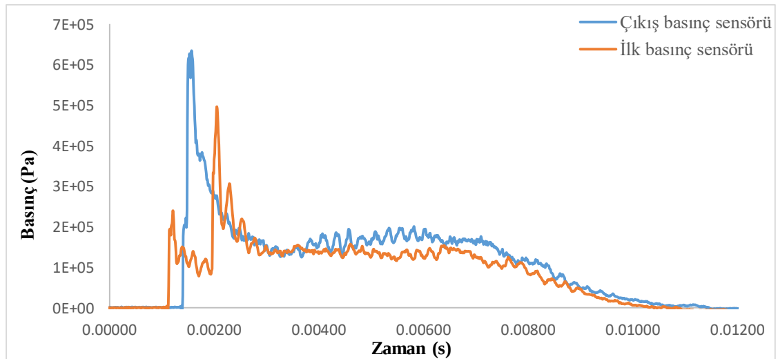
Şekil 4. 1. Şok testlerinde patlama sonucu oluşan basınç- zaman grafiği
