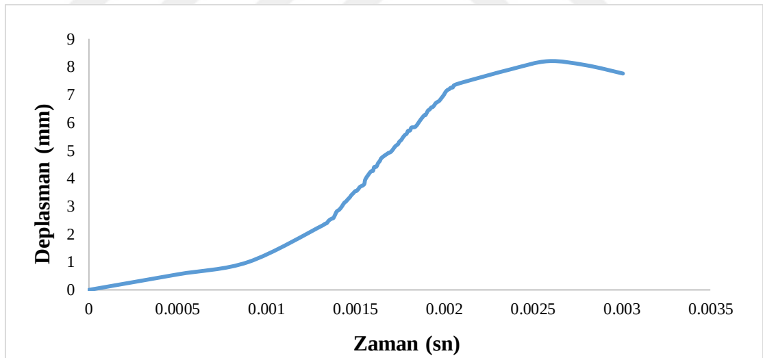
Şekil 4. 5. EPP köpük çekirdek yapısına sahip sandviç yapının arka plakasının şok testi sonucunda oluşan deplasman-zaman grafiği
