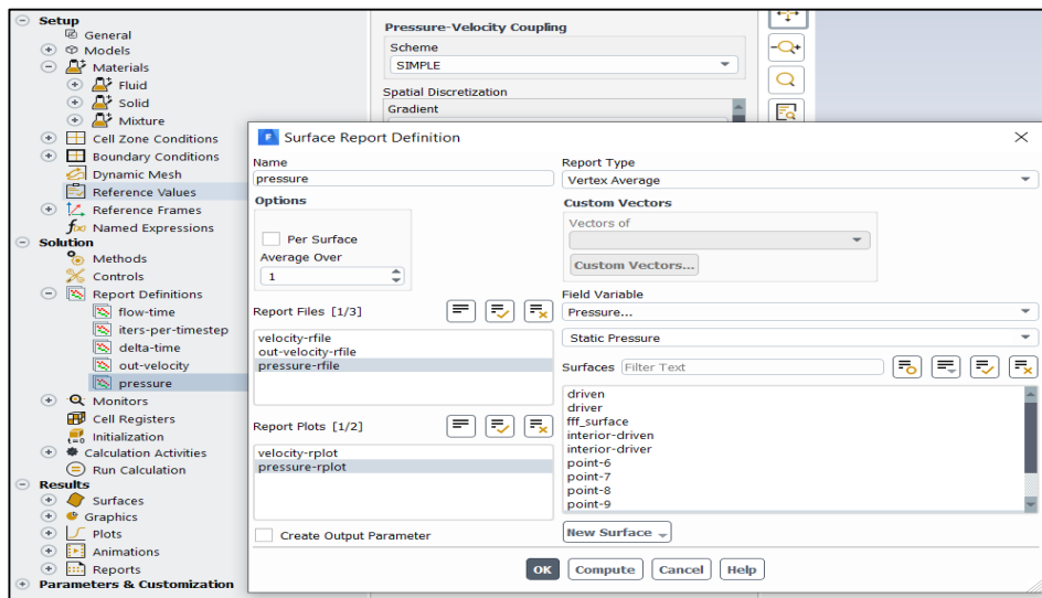
Şekil 3. 15. Analiz sonucu olarak istenilen grafiklerin seçilmesi
