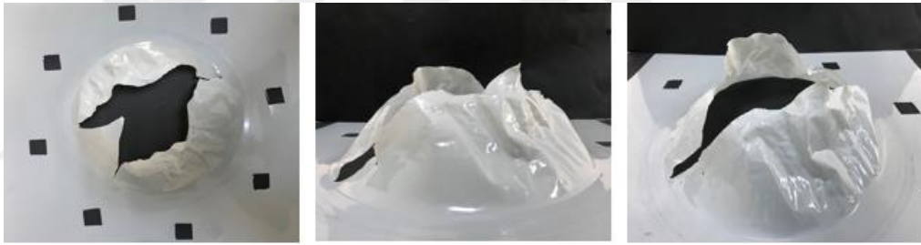
Şekil 4. 2. Şok testleri sonucunda oluşan diyafram görüntüsü
