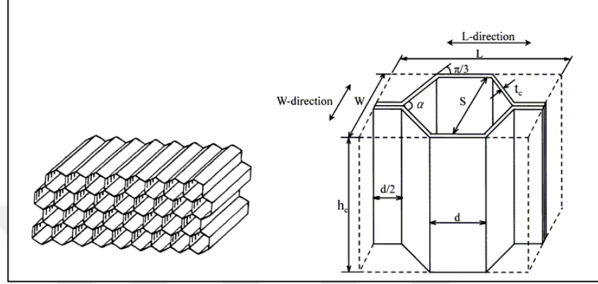
Şekil 2. 6. Balpeteği yapı geometrisi (Türkoğlu 2020)
