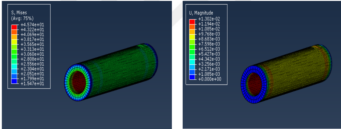
Şekil 3. 33. Parça 4'ün analiz sonuçları
