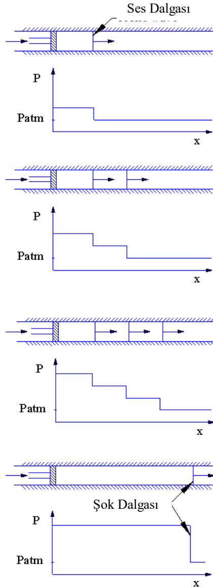
Şekil 2. 25. Şok dalgası meydana gelişi (Saad 1993)
