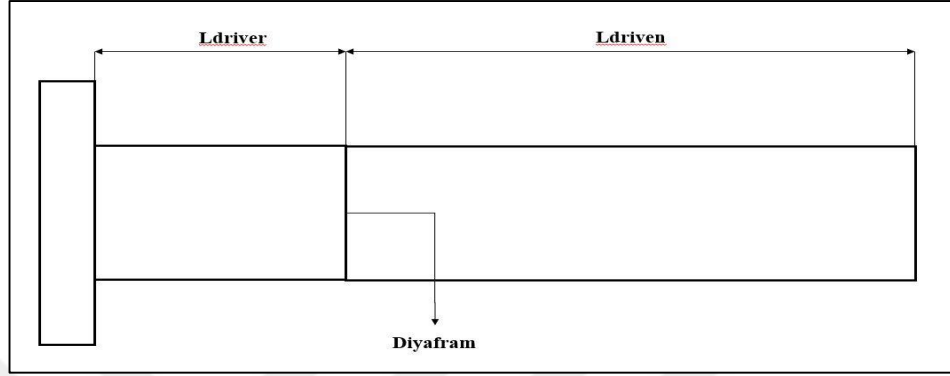
Şekil 2. 29. Teorik olarak şok tüpünün geometrisi
