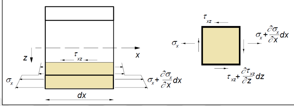
Şekil 2. 21. Bir alt alan için denge tanımlayan kiriş dx kesiti (Zenkert 1995)
