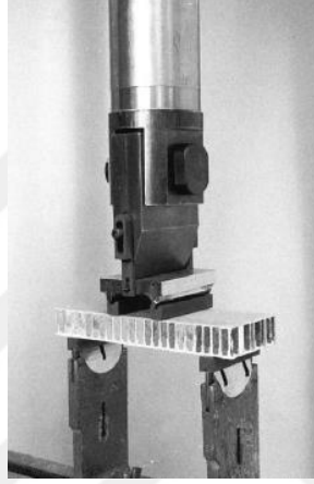
Şekil 2. 13. Sandviç yapı eğilme testi (ASTM C393)
