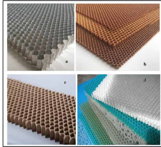
Şekil 2. 8. Farklı malzemelerden üretilmiş balpeteği çekirdek yapıları
