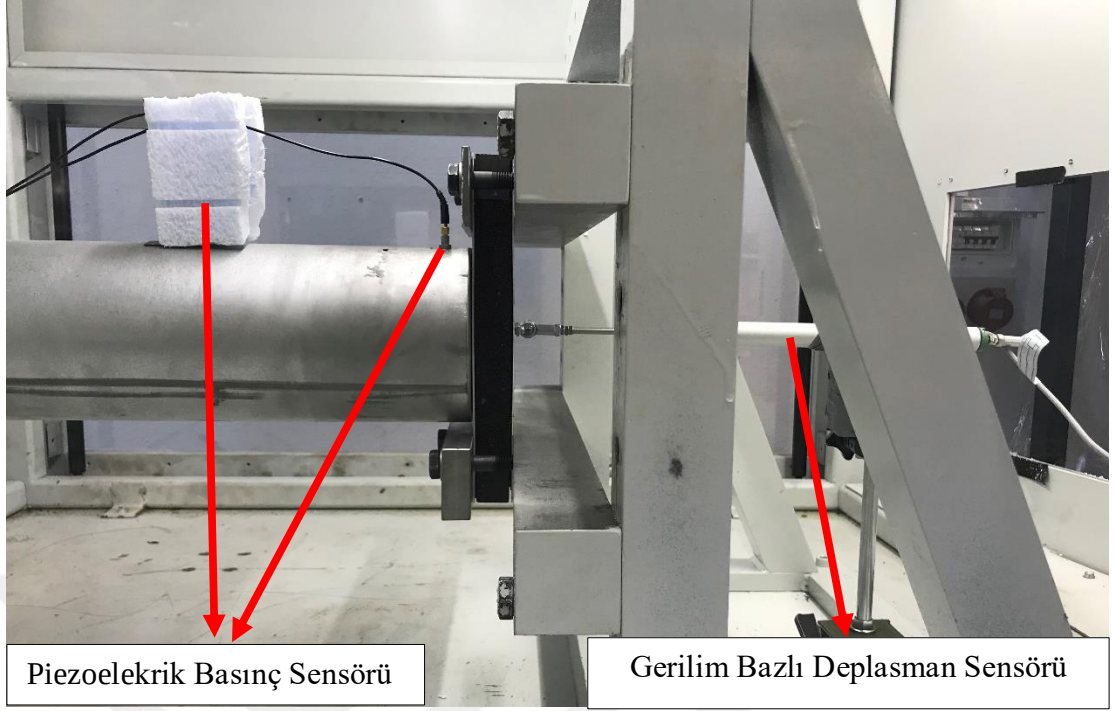
Şekil 3. 49. Deney düzeneğinde basınç ve deplasman sensörlerinin konumları
