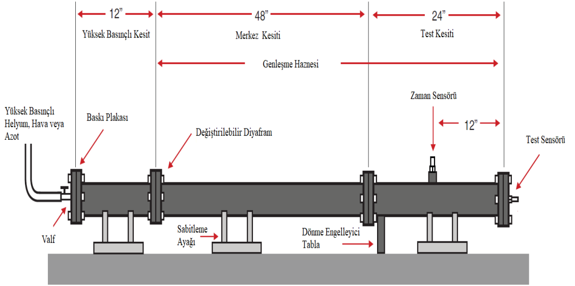
Şekil 2. 28. Örnek bir şok tüp tasarımı
