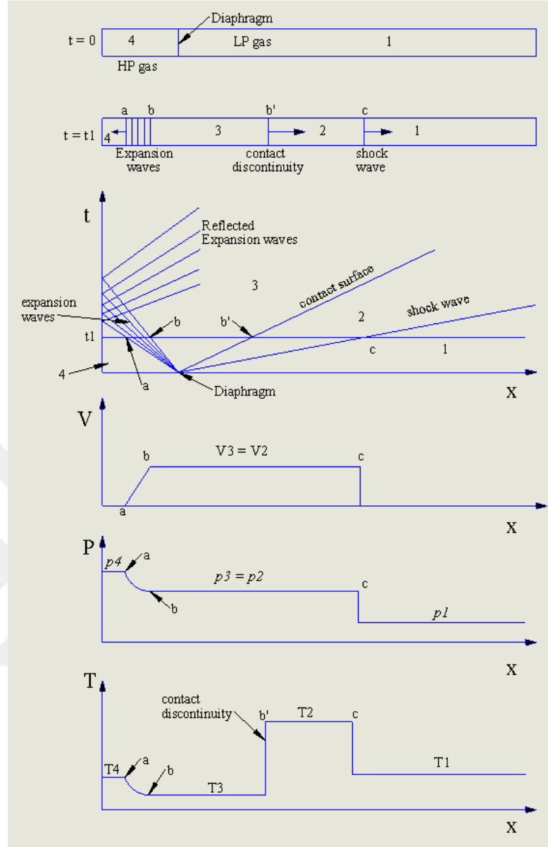
Şekil 2. 30. Şok tütünün çalışması (Russo, A.L. and Hertzberg, A. 1958)
