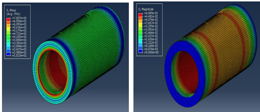
Şekil 3. 27. Parça 1'in analiz sonuçları
