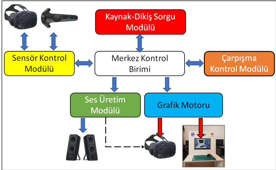
Şekil 3.3. Geliştirilen sanal kaynak simülatörünün yazılım mimarisi
