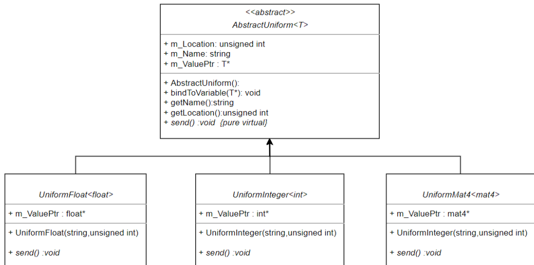
řekil 4.26. Genel deęiřken sınıfları UML diyagramı
