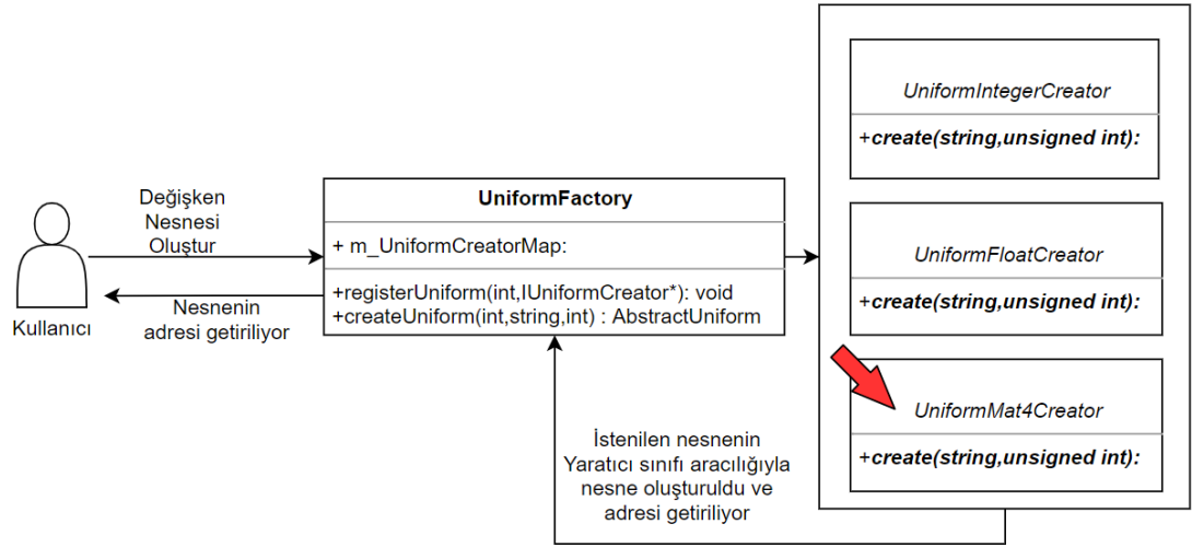
Şekil 4.28. Genel değişken nesnelerinin oluşturulması diyagramı
