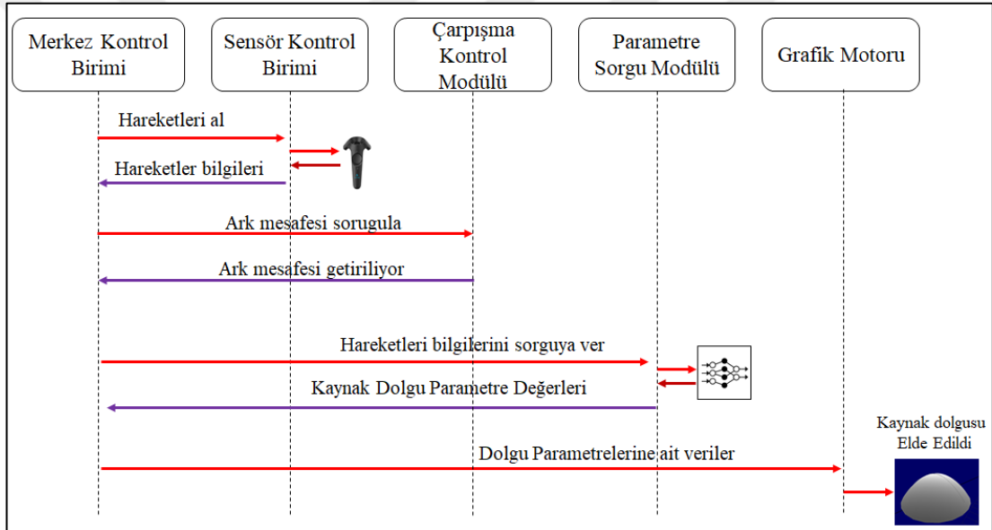
Şekil 5.18. Simülör modüllerinin kaynak dolgusunun elde edilmesindeki işlem sıra diyagramı
