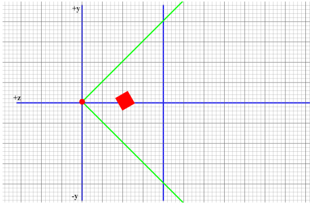
Şekil 4.50. Kamera dönüşümünün şekiller üzerine etkisi
