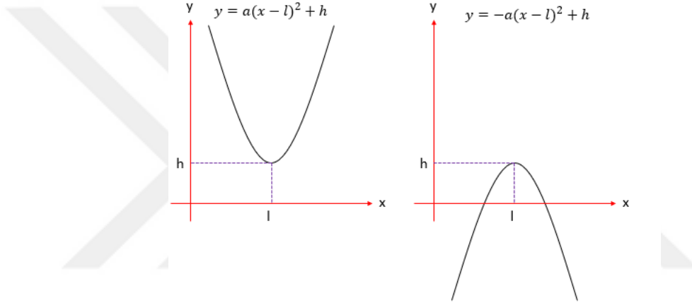
Şekil 5.5. Örnek parabol grafikleri
