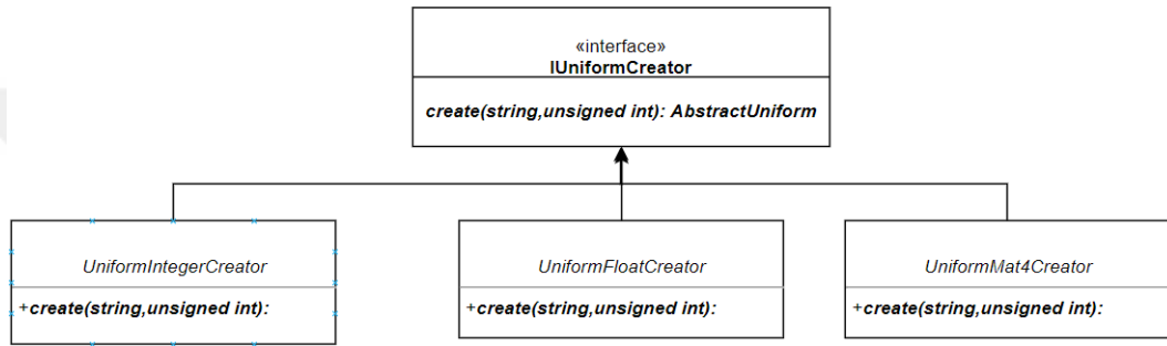
řekil 4.27. Yaratıcı fabrika sınıfları UML diyagramı
