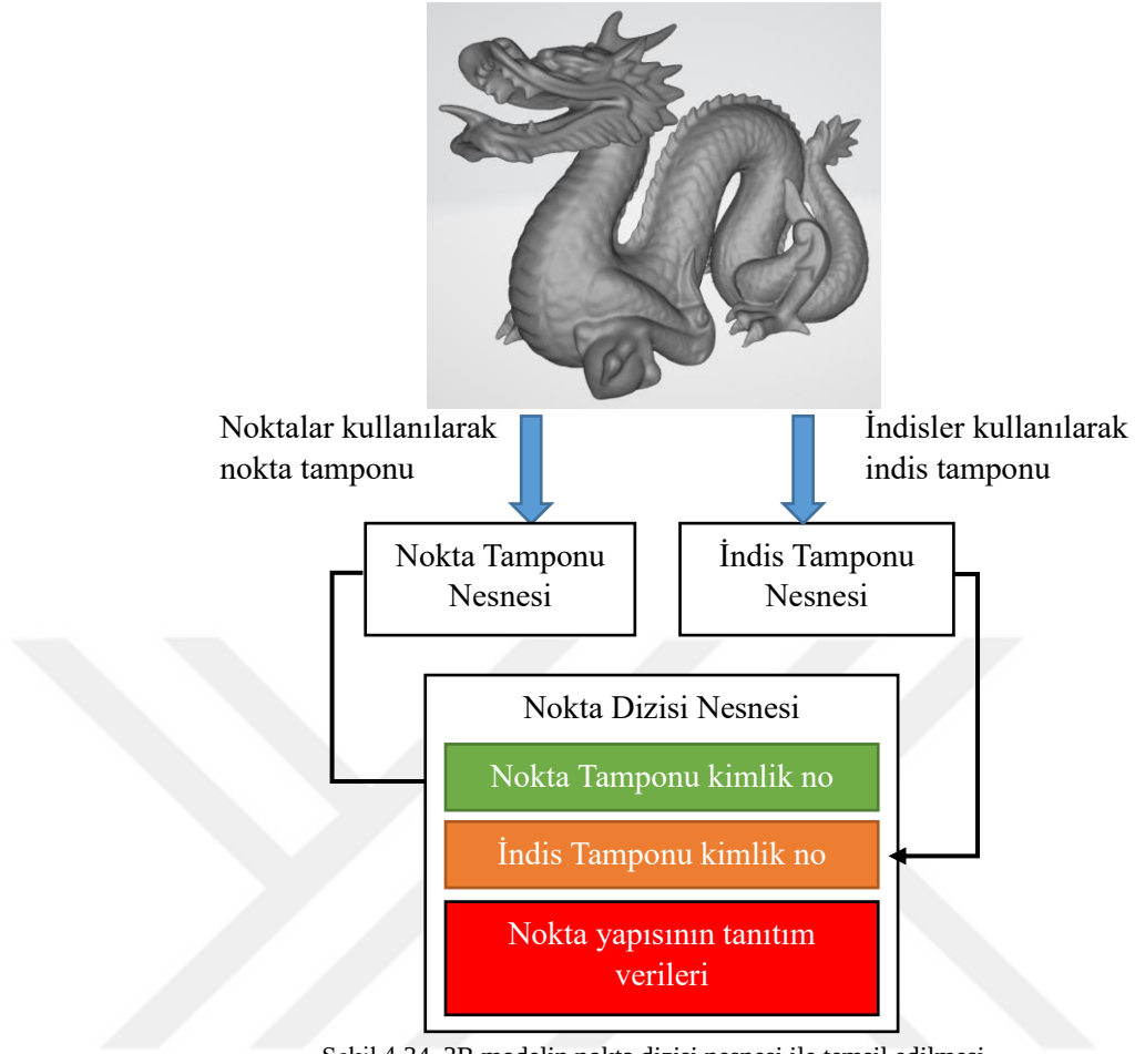
Şekil 4.34. 3B modelin nokta dizisi nesnesi ile temsil edilmesi
