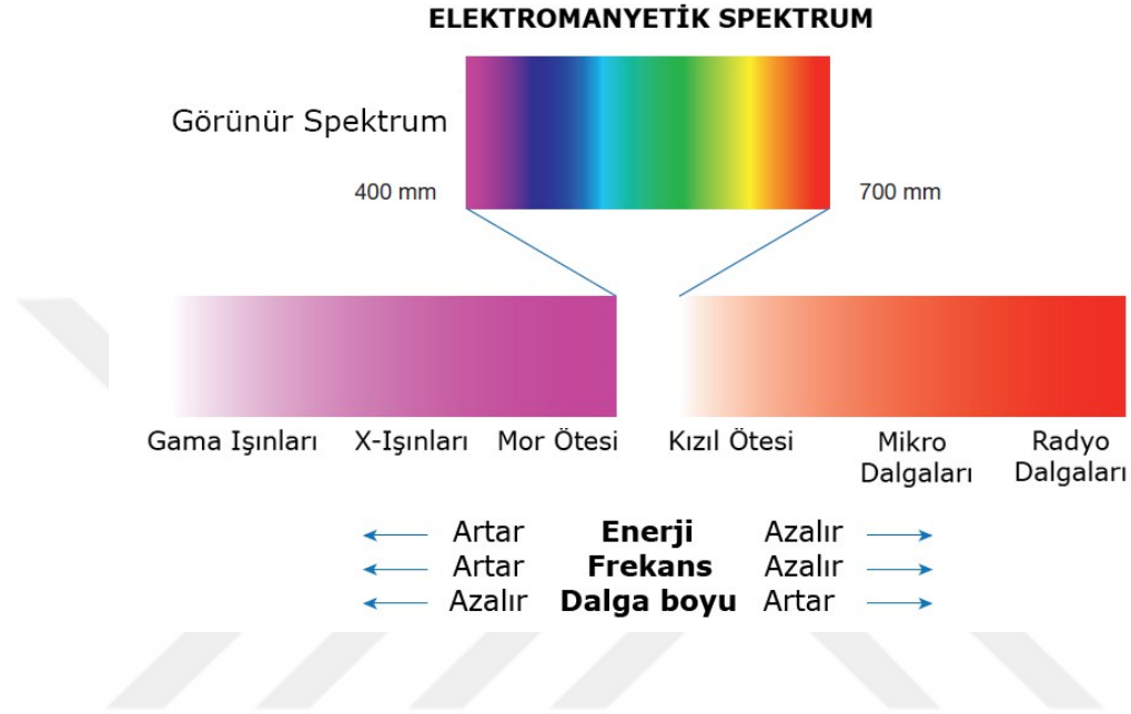
Şekil 1: Elektromanyetik Spektrum
