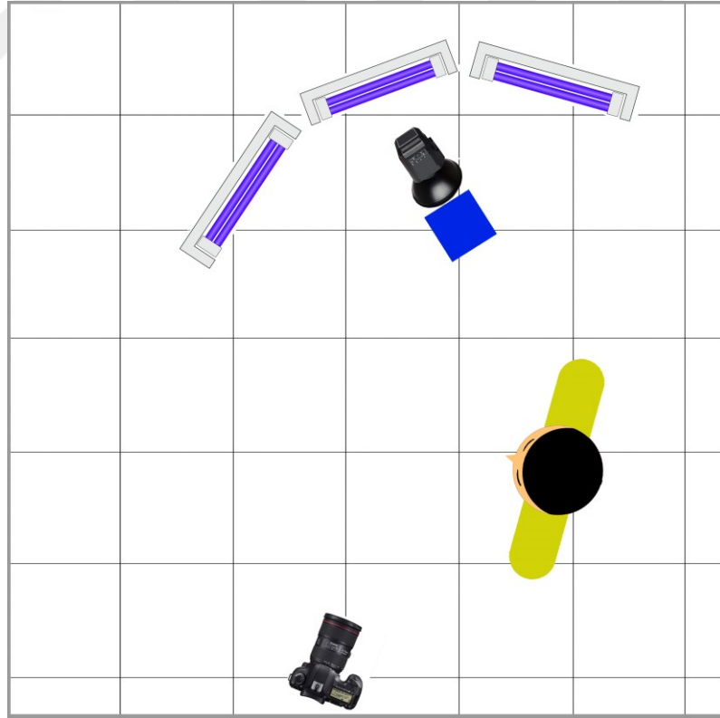
Şekil 45: Işık Şeması -3
