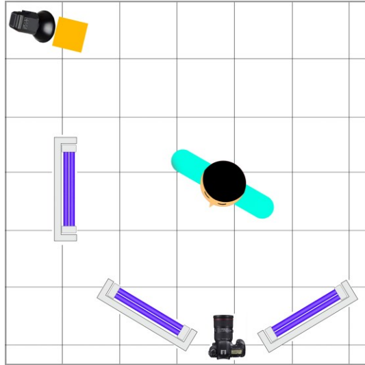
Şekil 43: Işık Şeması -1
