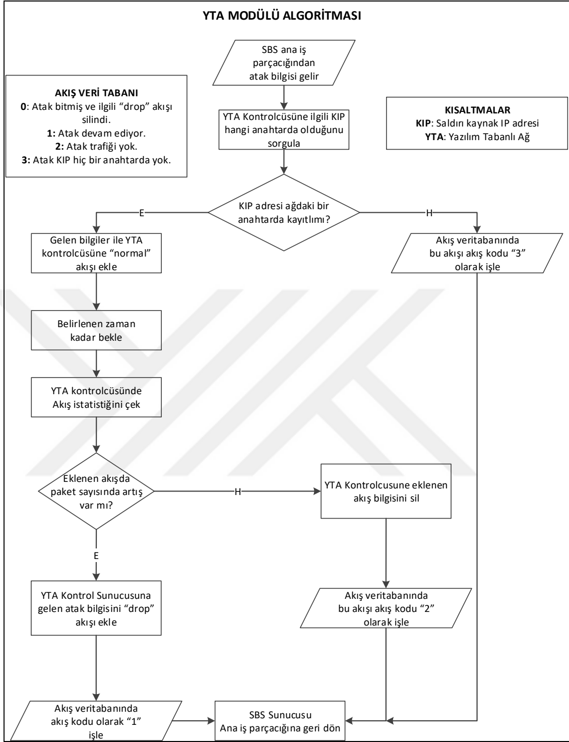
Şekil 4.12 YTA modülü algoritması.
