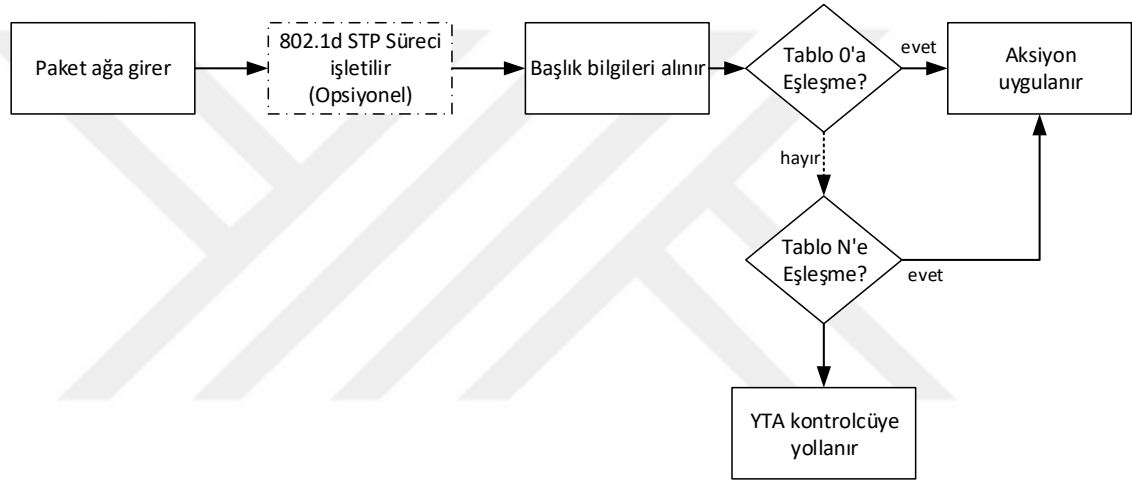
Şekil 2.7 YTA anahtar çalışma süreci.
