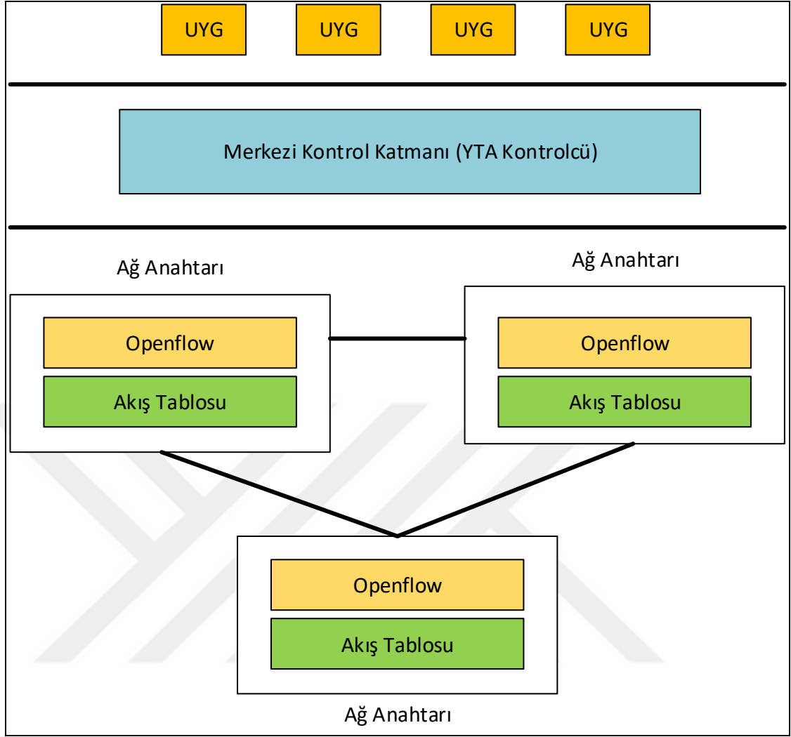
Şekil 2.6 Openflow destekli ağ anahtar yapısı.
