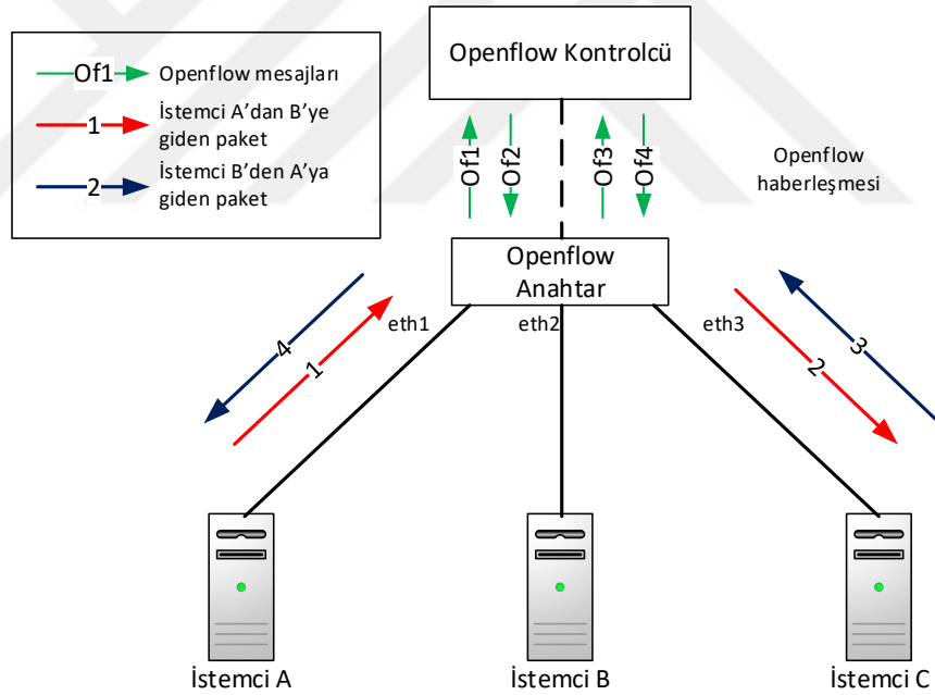
Şekil 2.9 Örnek YTA haberleşme süreci.
