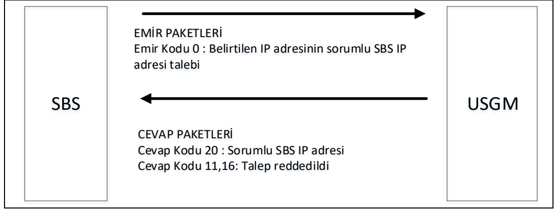
Şekil 4.7 SBS sunucusun atak kaynak IP adresini öğrenme süreci.
