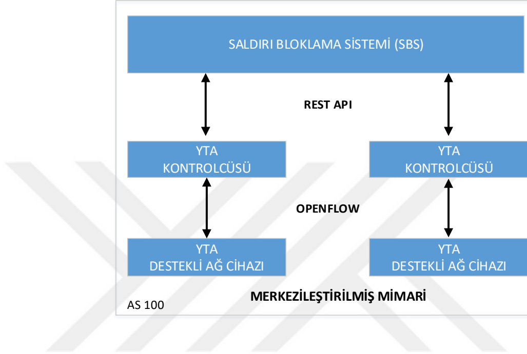
Şekil 3.1 Merkezi mimari.
