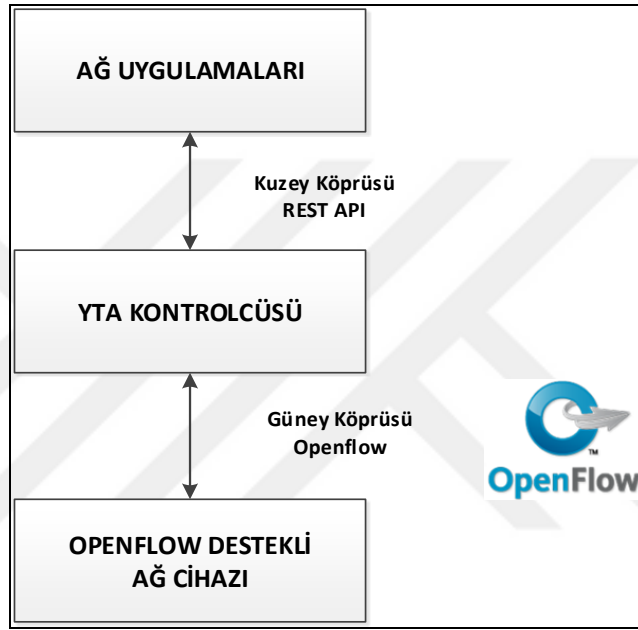
Şekil 2.4 YTA kuzey ve güney köprüsü.
