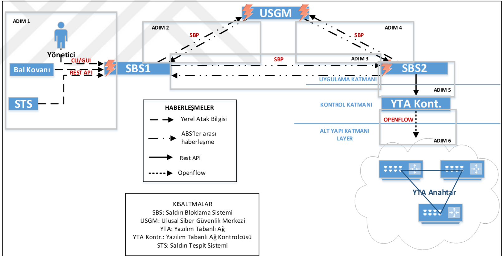
Şekil 3.8 Saldırı bloklama sistemi mimarisi.
