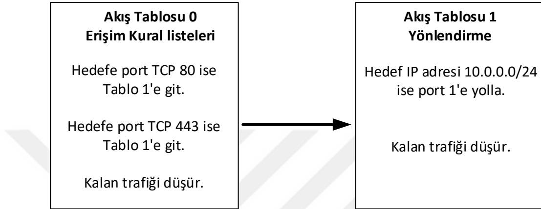
Şekil 2.8 Çoklu akış tablosu.
