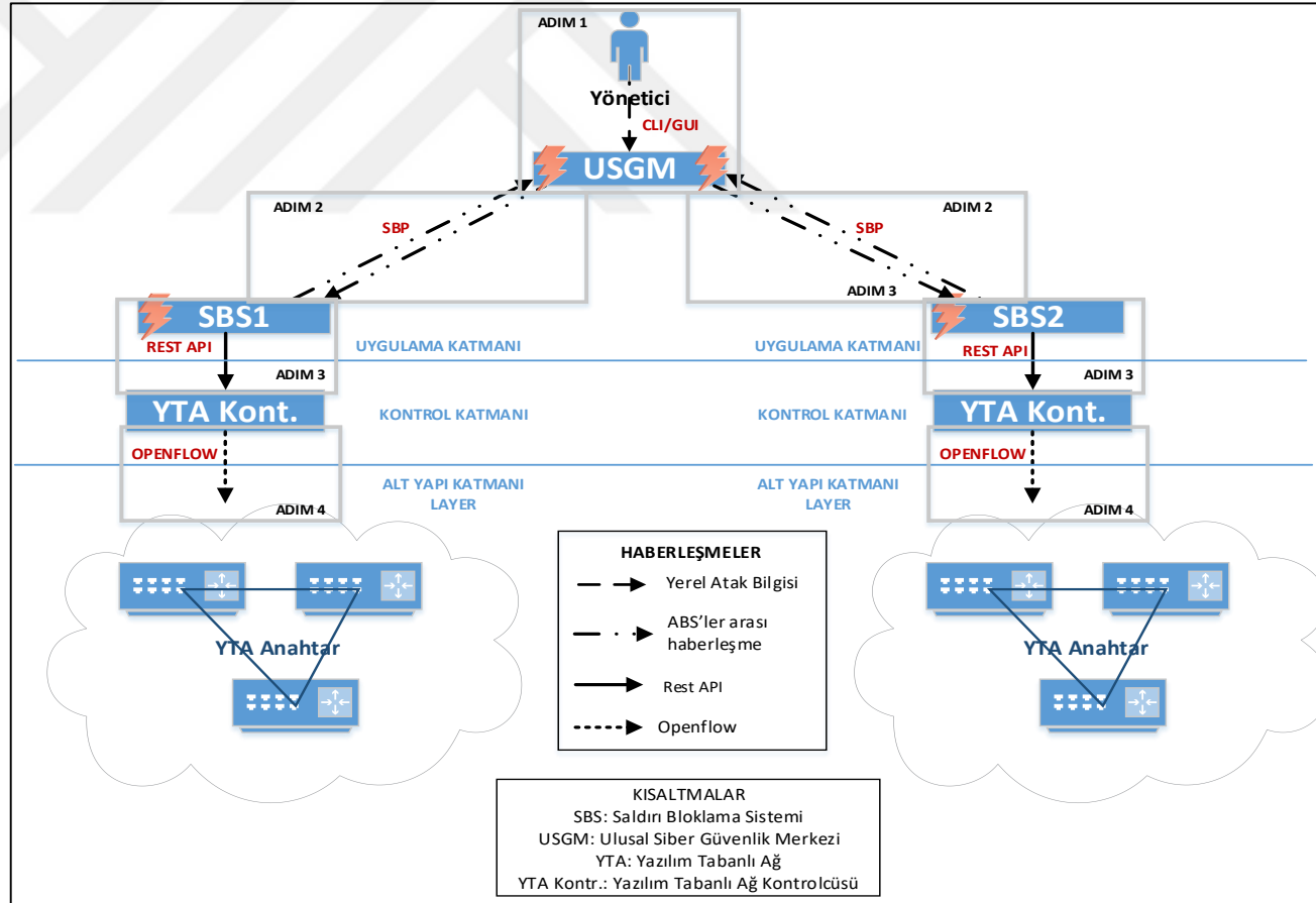
Şekil 3.10 Ulusal Saldırı Bloklama Sistemi mimarisi.
