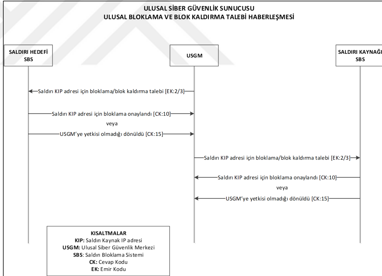
Şekil 4.19 USGM sunucusu ulusal bloklama ve blok kaldırma süreci.
