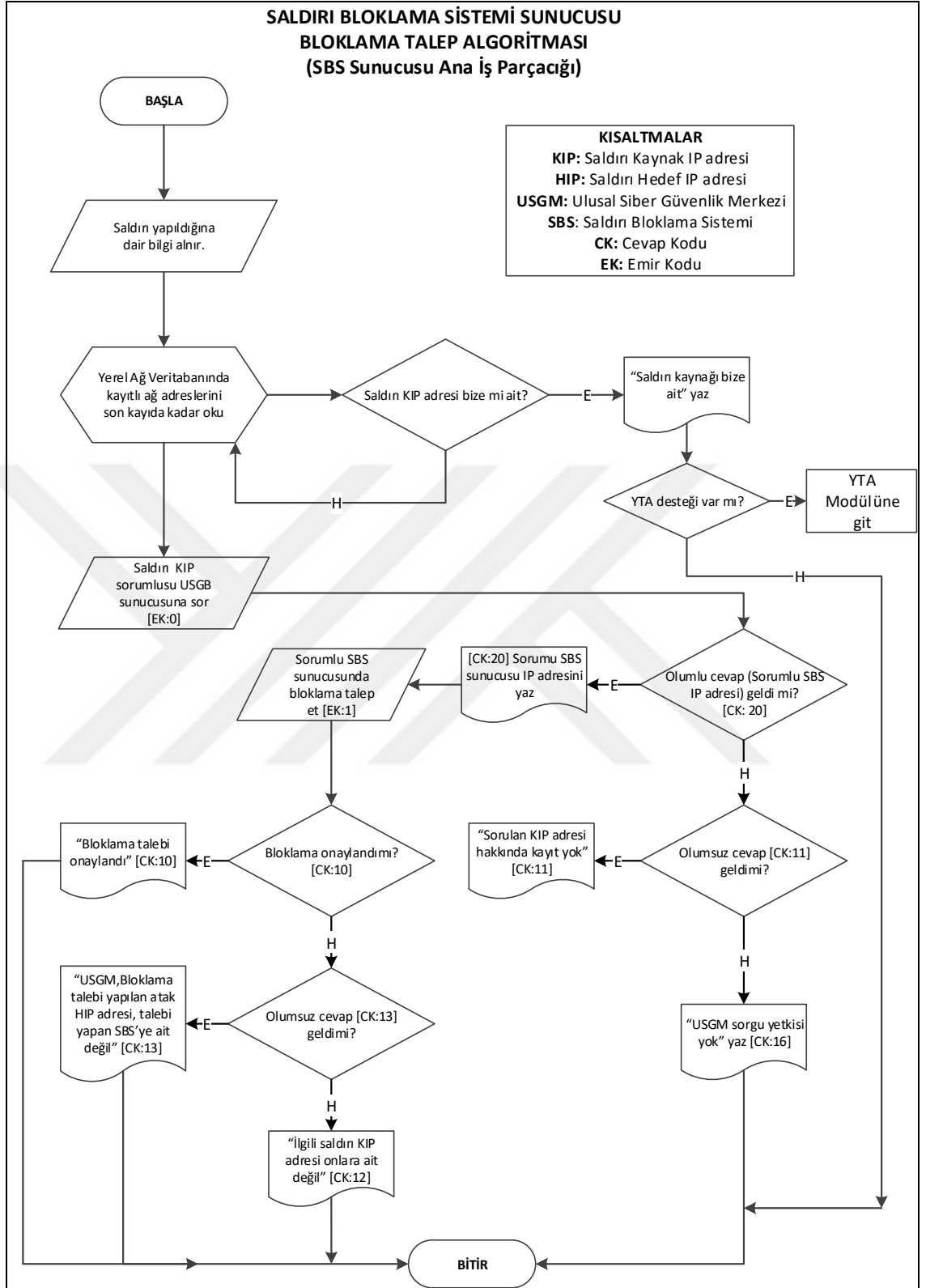
Şekil 4.9 Saldırı bloklama sistemi sunucusu bloklama talep algoritması.
