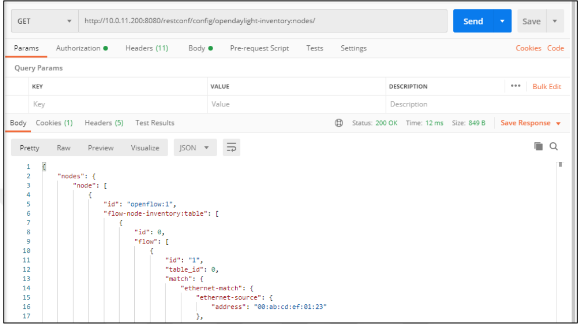
Şekil 5.12 Rest API ile sorgunun yapılması.
