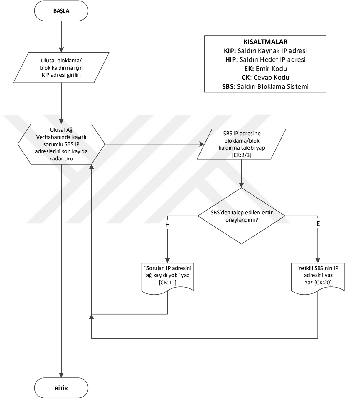
Şekil 4.20 USGM sunucusu ulusal bloklama ve blok kaldırma talep algoritması.
