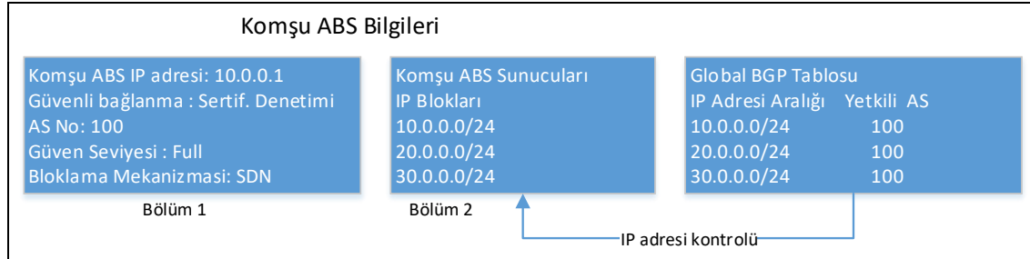
Şekil 3.5 Komşu ABS'nin tanımı ve ağ bilgilerinin kontrolü.
