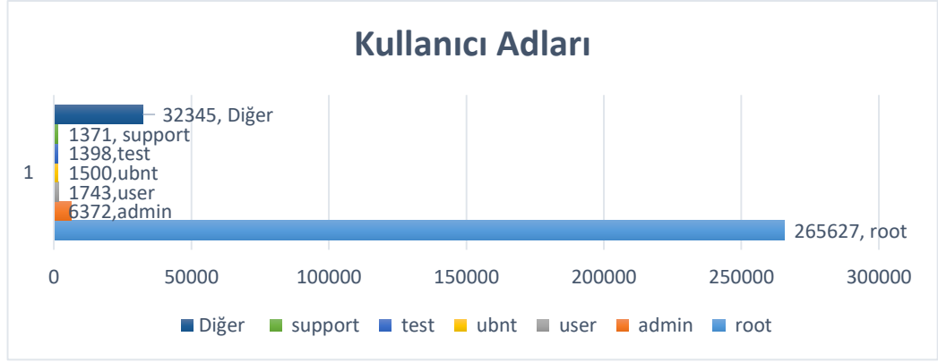
Şekil 1.2 Ataklarda kullanılan kullanıcı adları dağılımı.
