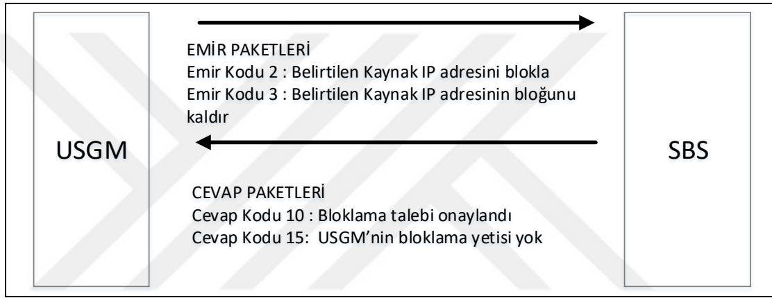
Şekil 4.18 USGM sunucusu ulusal bloklama ve blok kaldırma paketleri.
