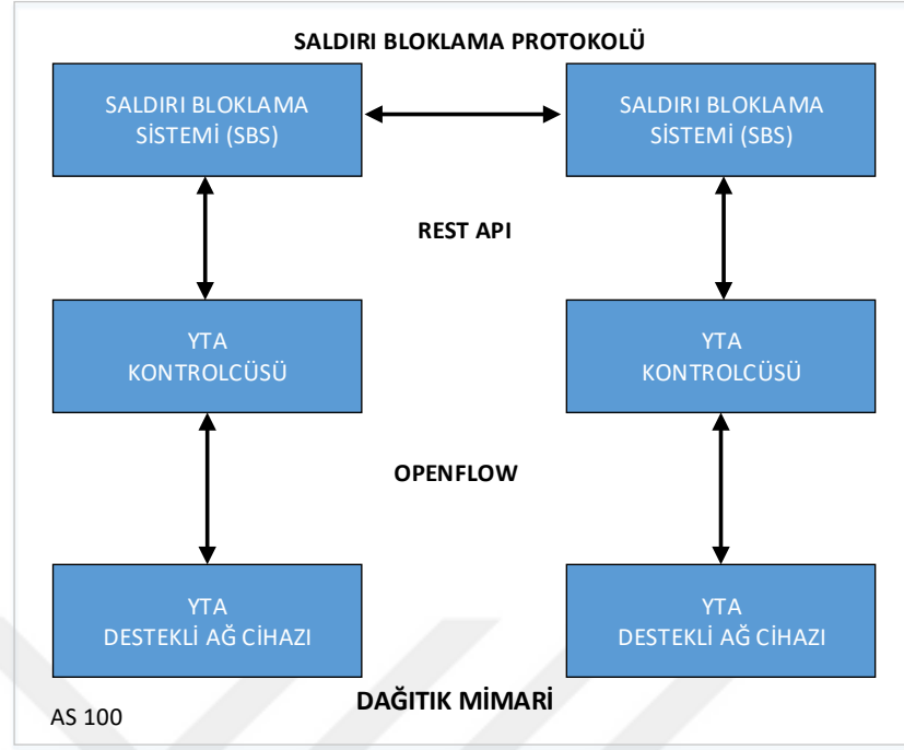
Şekil 3.2 Dağıtık mimari.
