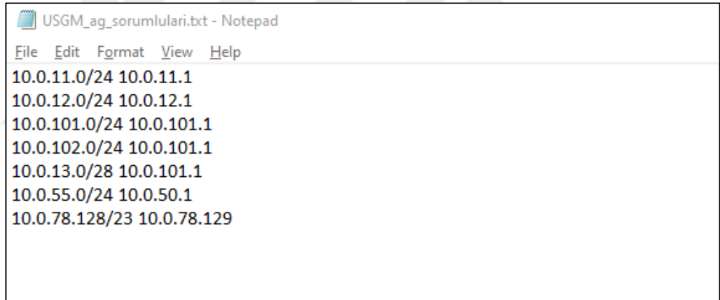
Şekil 4.15 USGM sunucusu yönetilen ağlar dosyası.
