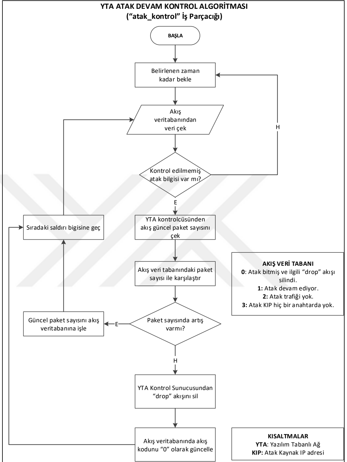
Şekil 4.13 YTA atak devam kontrol algoritması.
