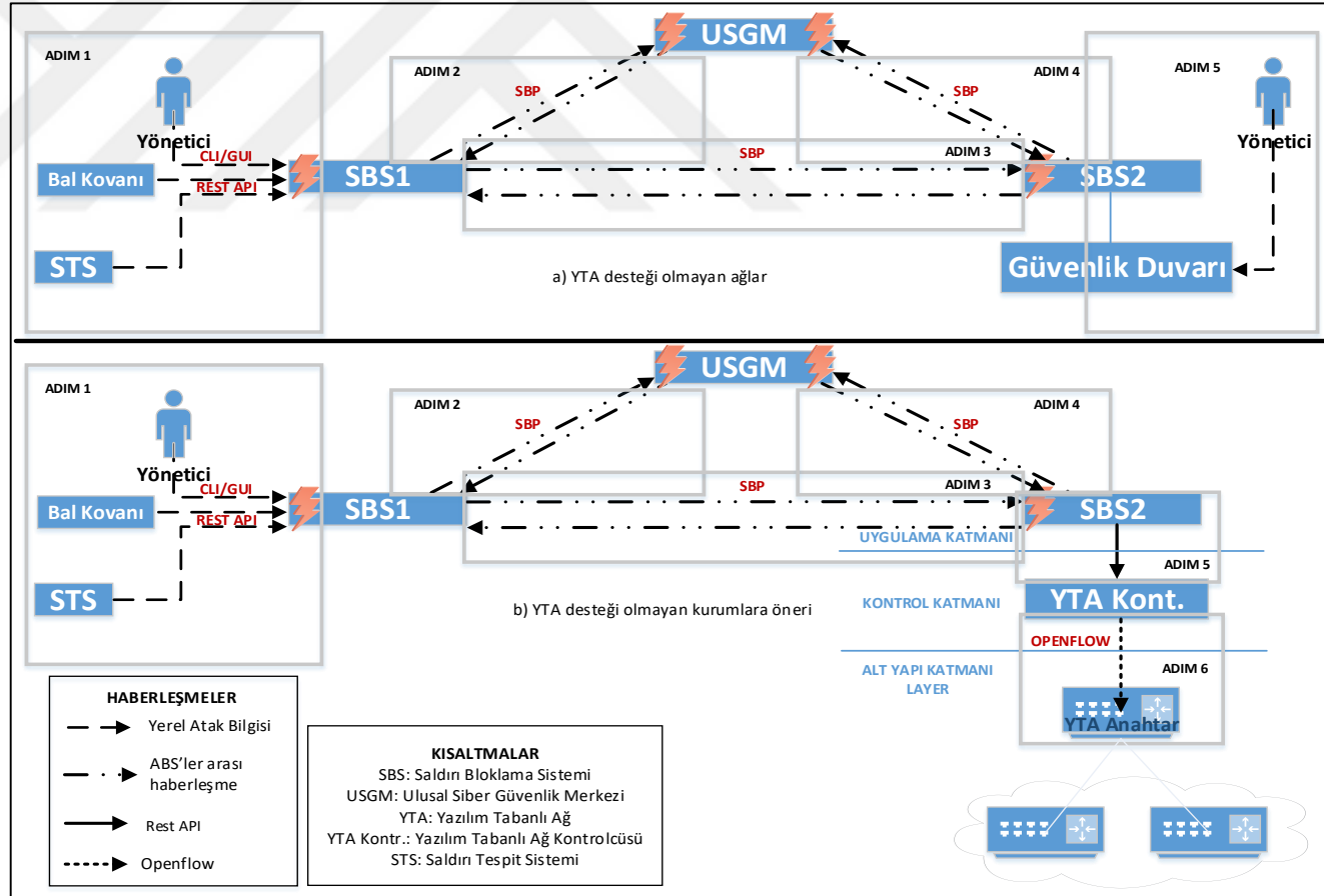
Şekil 3.9 a)YTA desteği olmayan ağlarda kullanım b) YTA desteği olmayan ağlarda tavsiye edilen kullanım.
