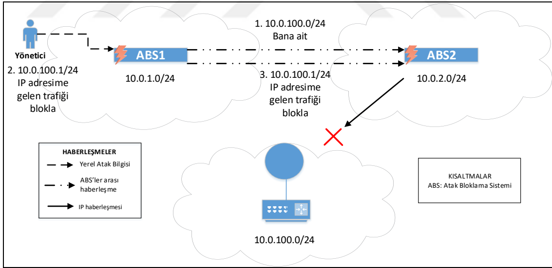
Şekil 3.4 Sistemin kötü amaçlı kullanımı.
