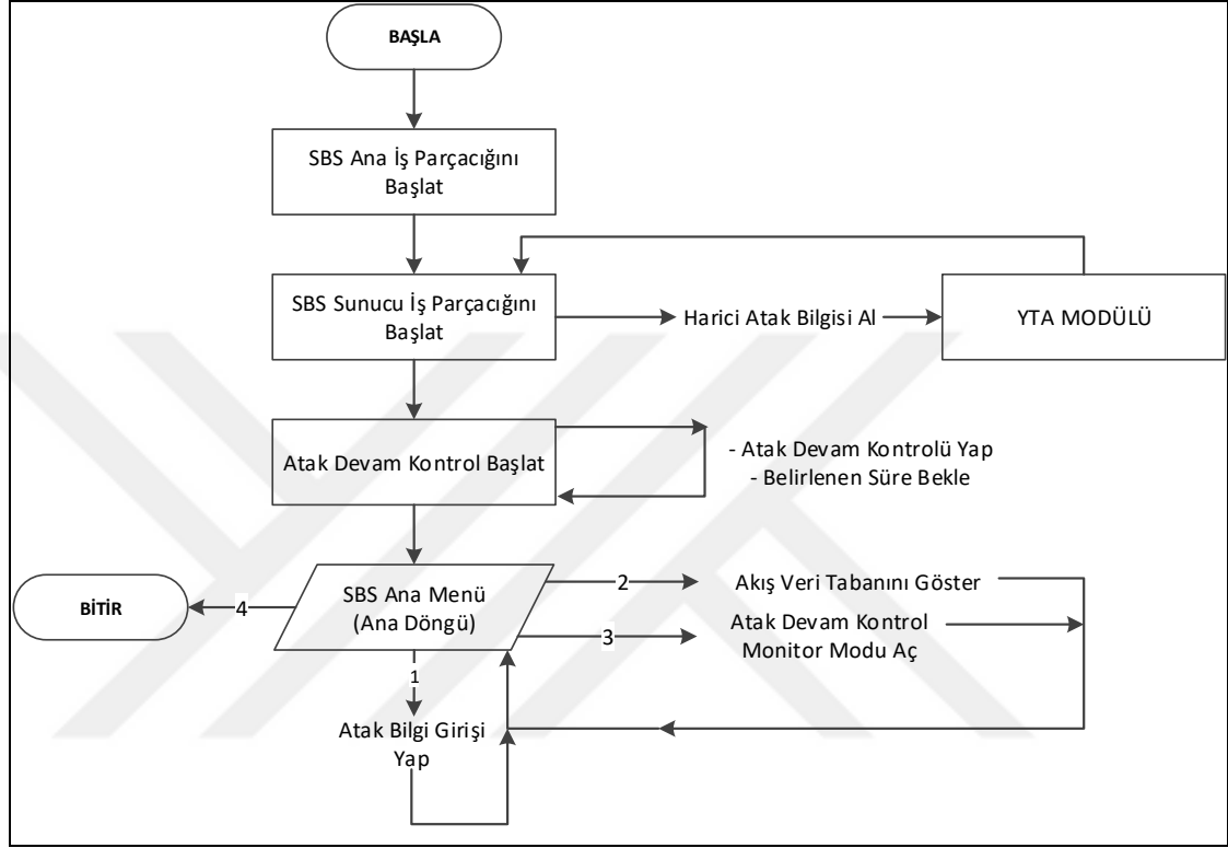
Şekil 4.1 SBS sunucusu iş parçacıkları çalışma süreci.
