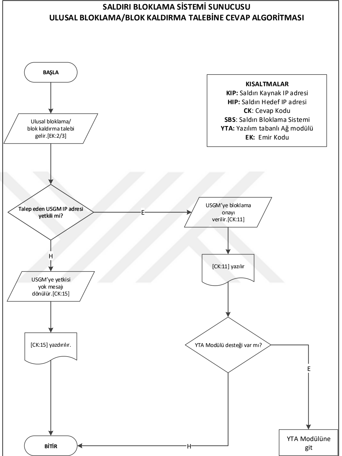
Şekil 4.21 USGM sunucusu ulusal bloklama ve blok kaldırma cevap algoritması.
