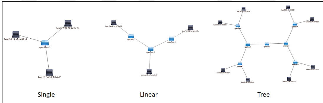
Şekil 5.3 Mininet hazır topoloji şablonları.
