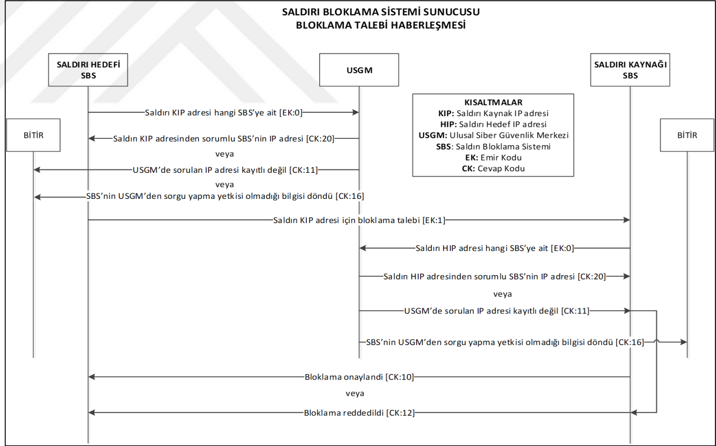
Şekil 4.6 USGM saldırı blokla ma süreci.
