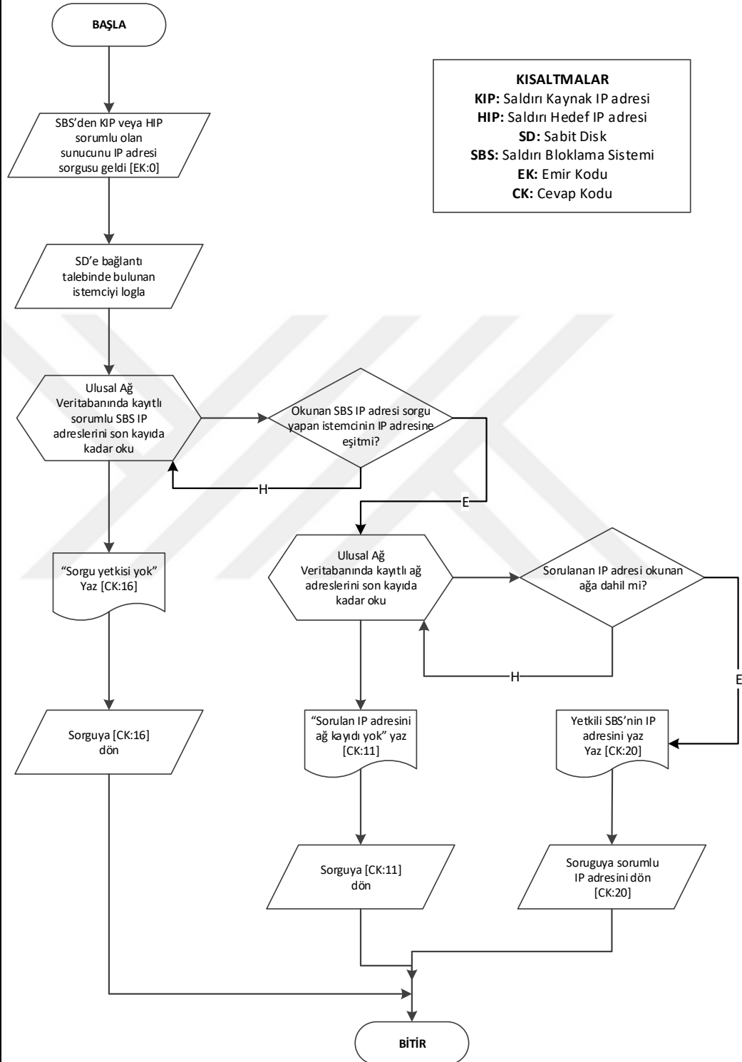
Şekil 4.11 USGM sunucusunun SBS sunucusunu bilgilendirme algoritması.
