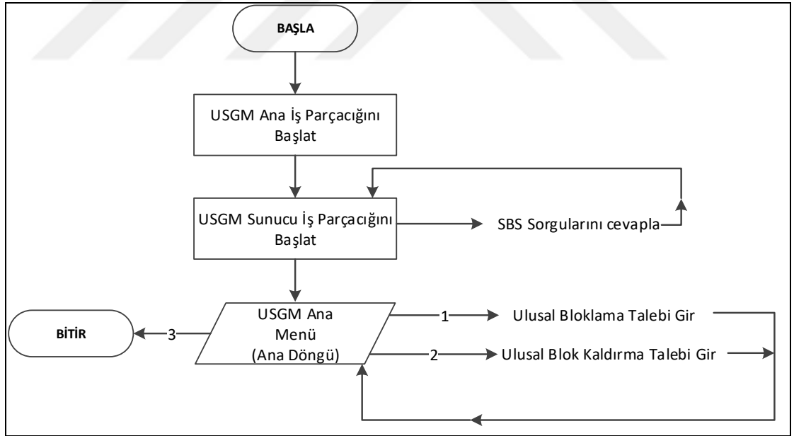
Şekil 4.14 USGM çalışma süreci.
