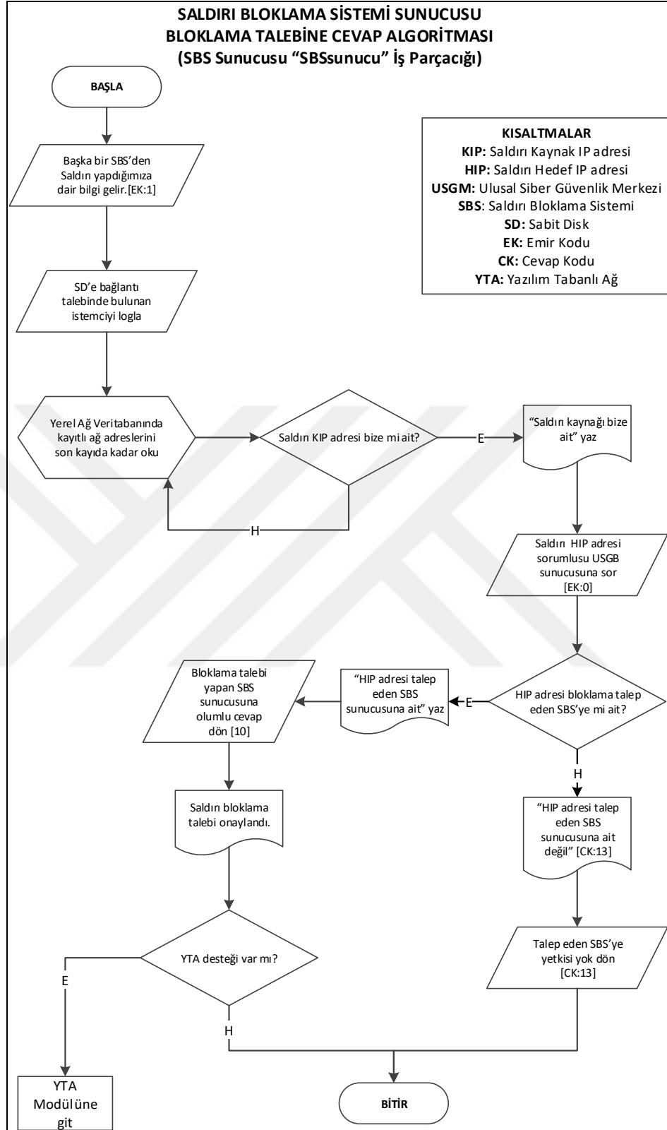
Şekil 4.10 Saldırı bloklaya sistemi sunucusu bloklaya talebine cevap algoritması.
