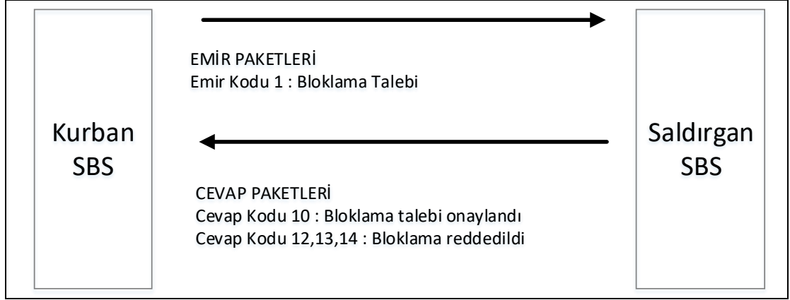
Şekil 4.8 SBS sunucusun atak kaynak IP'nin kontrolünü sağlayan SBS sunucusuna yaptığı bloklama talebi süreci.
