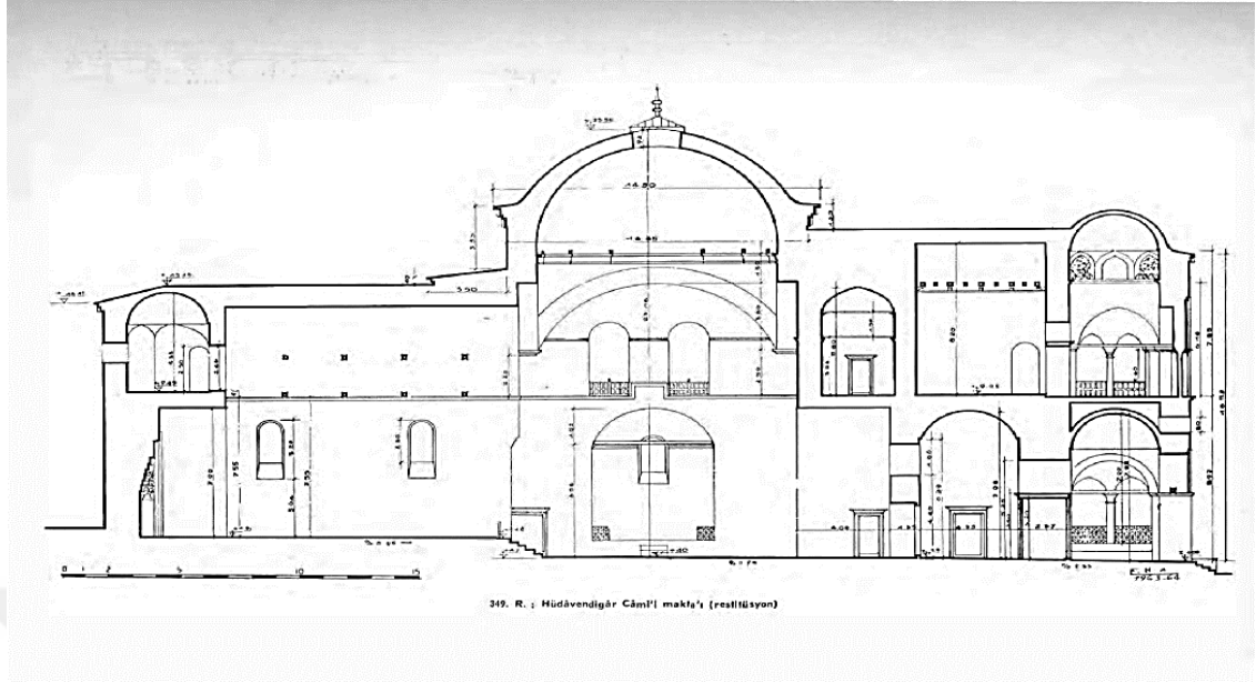
Şekil 2: Bursa Hudâvendigâr Külliyesi (Cami ve Medrese) Planı 151
