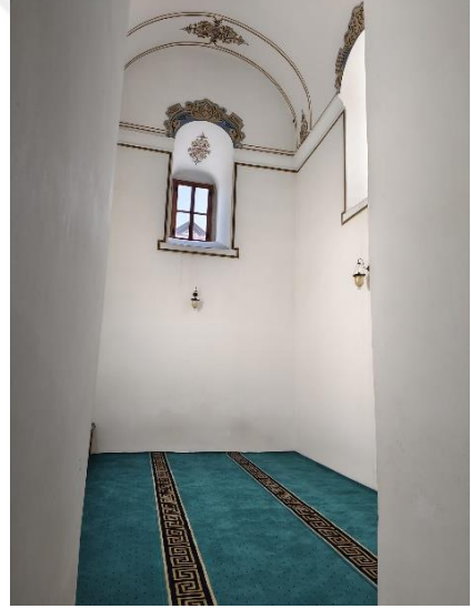
Resim 9: Tabhane İç Mekânı.
