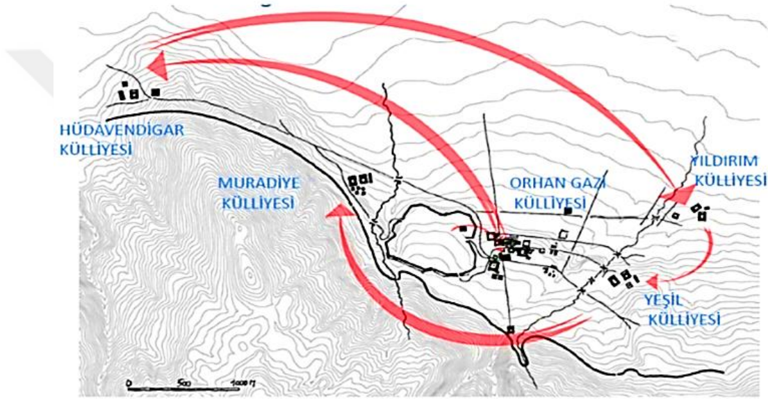
Şekil 1: Bursa Hudâvendigâr Külliyesi'nin Konumu 130
