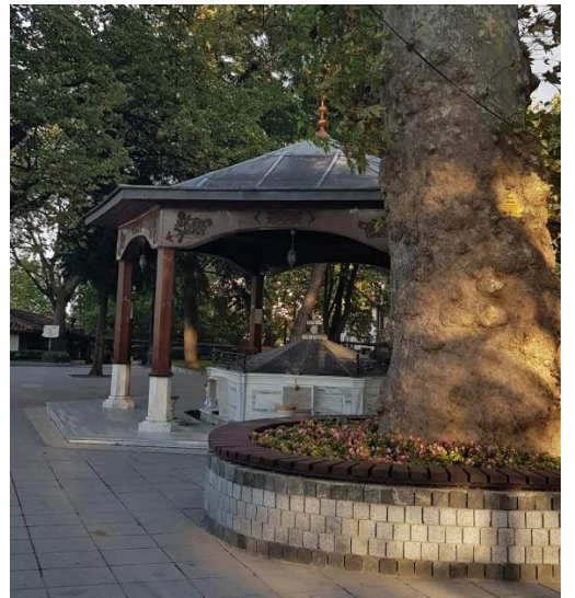
Resim 24: Caminin Dış Şadırvanı.
