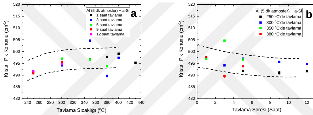
Şekil 5.5 Al (5 dk atmosfer) +a-Si:H örneklerin kristal pik konumlarının (a) tavlama sıcaklığı ve (b) tavlama süresi ile değişimi grafikleri. Kesikli çizgiler izleme kolaylığı içindir.
