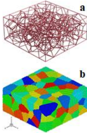
Şekil 2.4 pc-Si'un (a) tanecik sınırları ve (b) farklı kristal yönelimine sahip tanecikleri (altta) [54]
