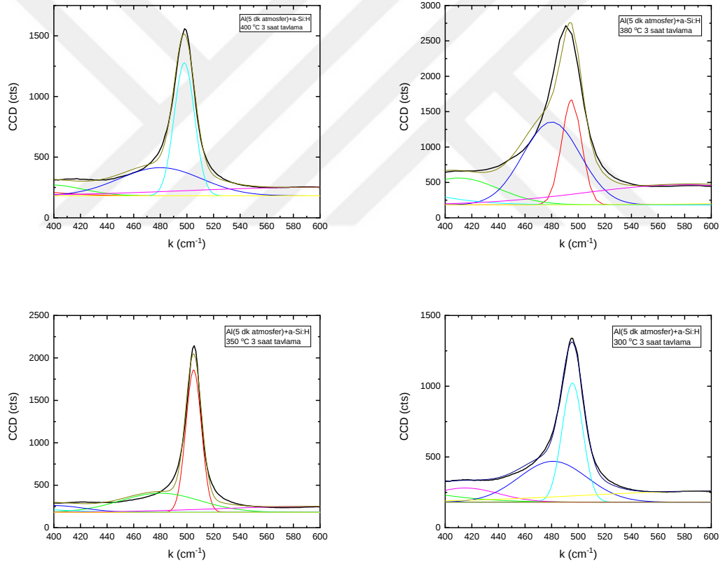
Şekil 5.1 3 saat süre ile farklı sıcaklıklarda tavllanmış örnekler için çoklu Gauss fonksiyonunun uygulanması
