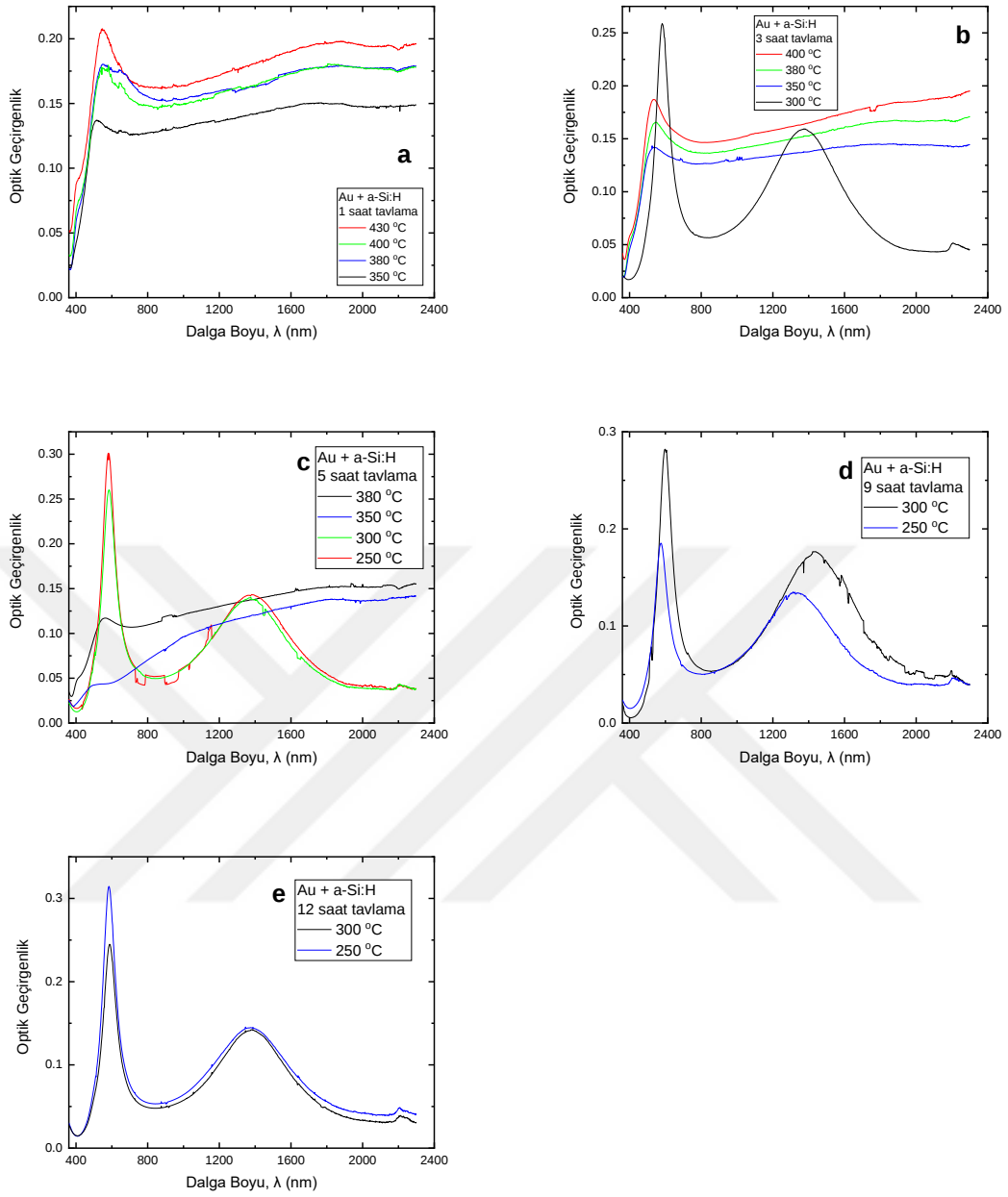
Şekil 5.13 Au + a-Si:H örneklerin optik geçirgenlik grafikleri
