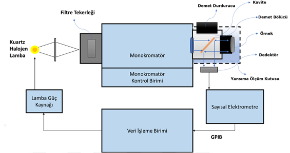
Şekil 3.7 Optik yansıtıcılık ölçüm düzeneği [98]
