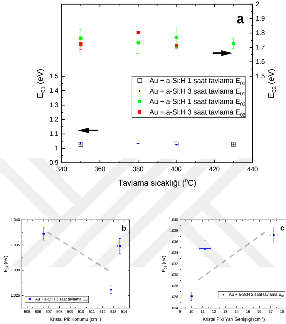
Şekil 5.22 AM05 örneklerin E_{01} ve E_{02} enerjilerinin sıcaklık (a), E_{01} enerjisinin kristal pik konumuna (b) ve kristal pik yarı genişliğine (c) bağlı grafikleri. Oklar izleme kolaylığı için verilmiştir.
