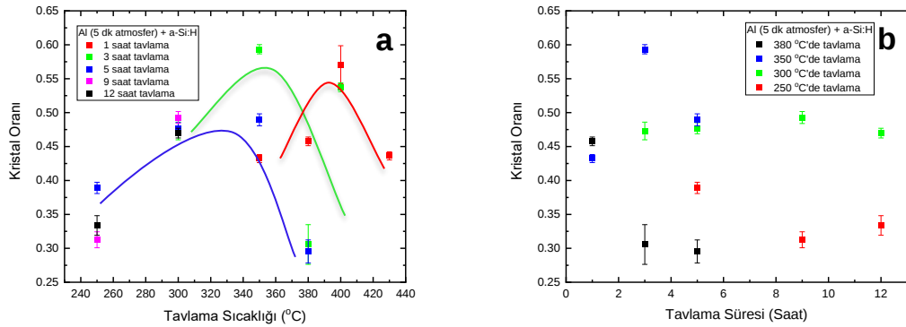
Şekil 5.2 Al (5 dk atmosfer) + a-Si:H örneklerin kristal oranlarının (a) tavlama sıcaklığı ve (b) tavlama süresi ile değişimi grafikleri. Eğriler izleme kolaylığı için eklenmiştir.
