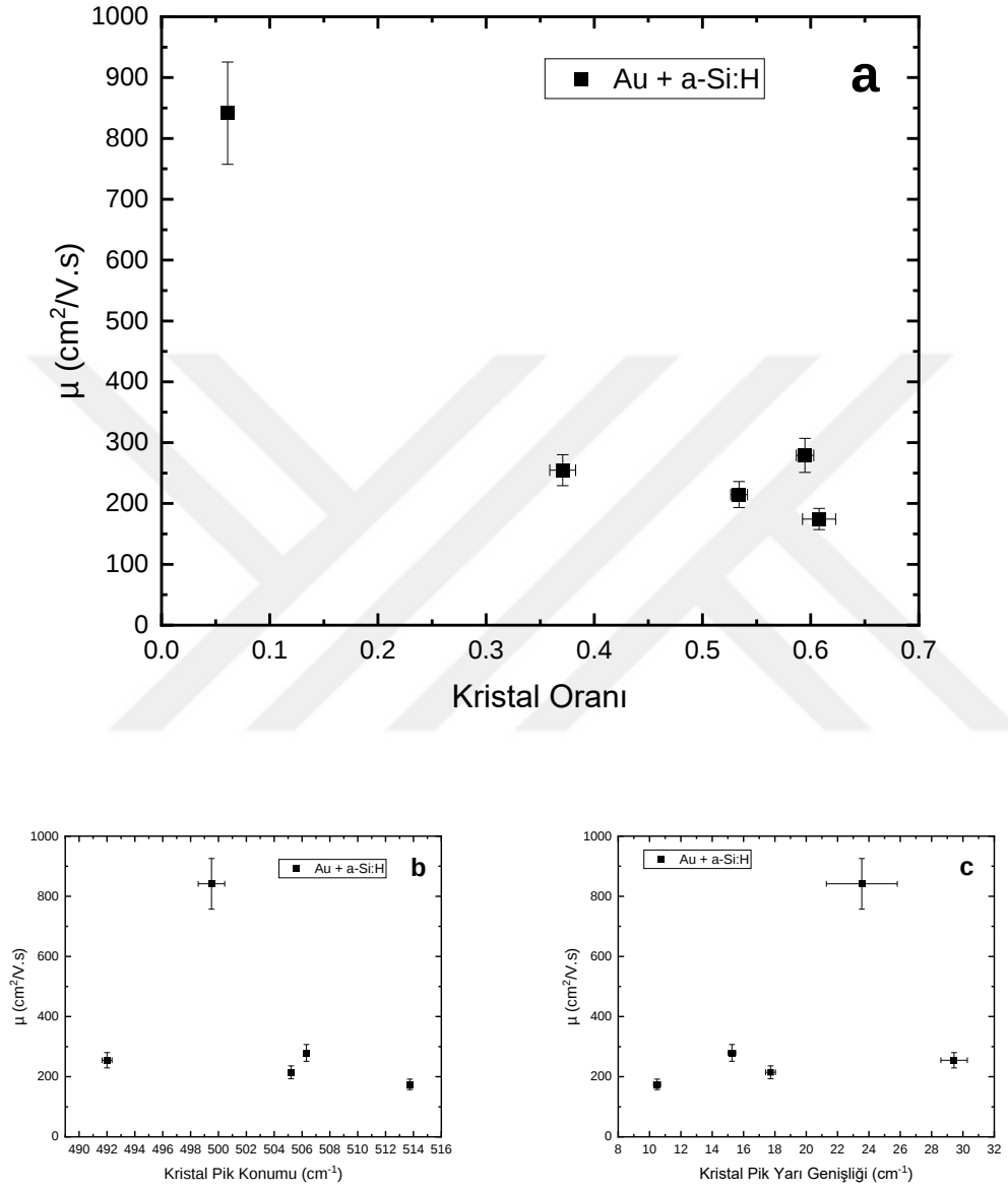
Şekil 5.28 Au + a-Si:H örneklerde taşıyıcı mobilitesinin kristal oranına (a), kristal pik konumuna (b) ve kristal pik yarı genişliğine (c) bağlı grafikleri. Oklar izleme kolaylığı için verilmiştir.
