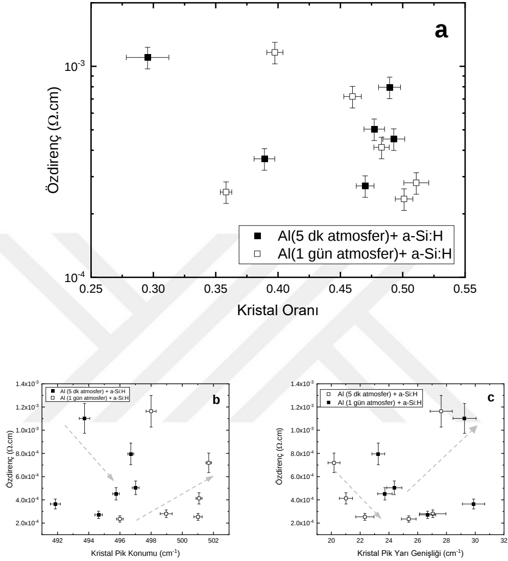
Şekil 5.23 Al (5 dakika atmosfer) + a-Si:H ve Al (1 gün atmosfer) + a-Si:H örneklerin öz direncinin kristal oranına (a), kristal pik konumuna (b) ve kristal pik yarı genişliğine (c) bağlı grafikleri. Oklar izleme kolaylığı için verilmiştir.
