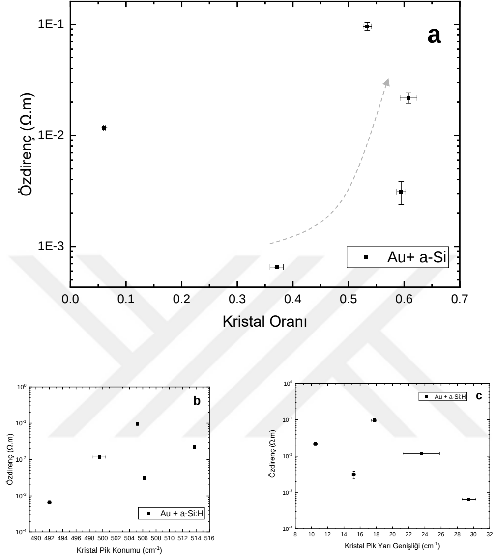
Şekil 5.24 Au + a-Si:H örneklerin öz direncinin kristal oranına (a), kristal pik konumuna (b) ve kristal pik yarı genişliğine (c) bağlı grafikleri. Oklar izleme kolaylığı için verilmiştir.
