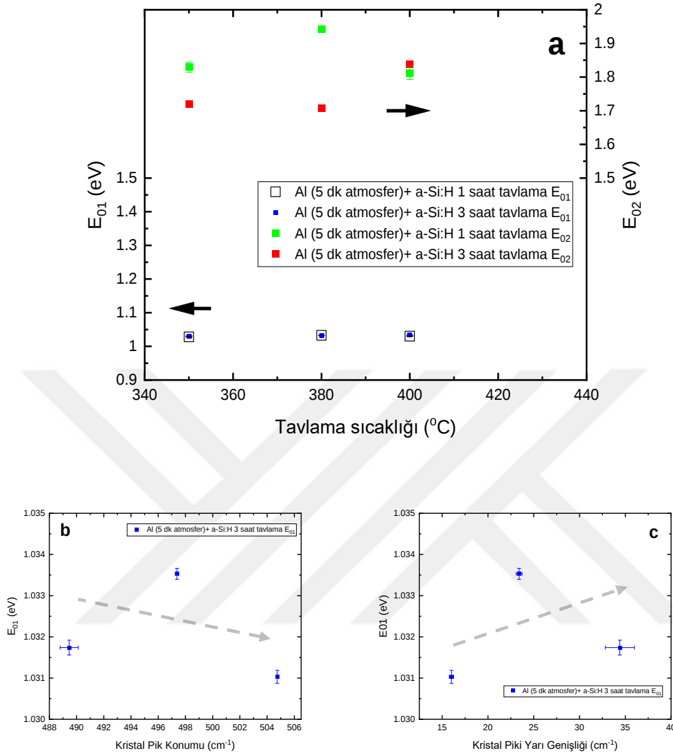
Şekil 5.21 AM03 örneklerin E_{01} ve E_{02} enerjilerinin sıcaklık (a), E_{01} enerjisinin kristal pik konumuna (b) ve kristal pik yarı genişliğine (c) bağlı grafikleri. Oklar izleme kolaylığı için verilmiştir.
