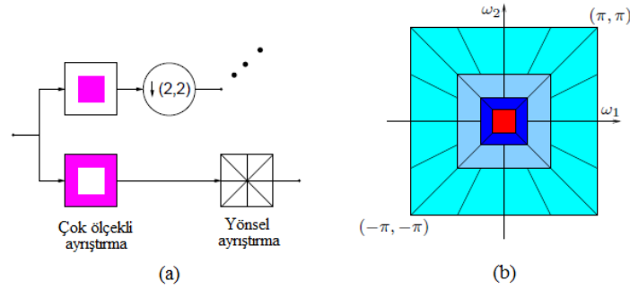
Şekil 2.15. Piramitsel yönsel filtre kümesi a) çok ölçekli ayrıştırma ve yönsel ayrıştırma ile piramitsel yönsel filtre kümesinin uygulanması b) sayı ve yönü değiştirilebilir frekans alt bölümleri (Do ve Vetterli, 2005)
