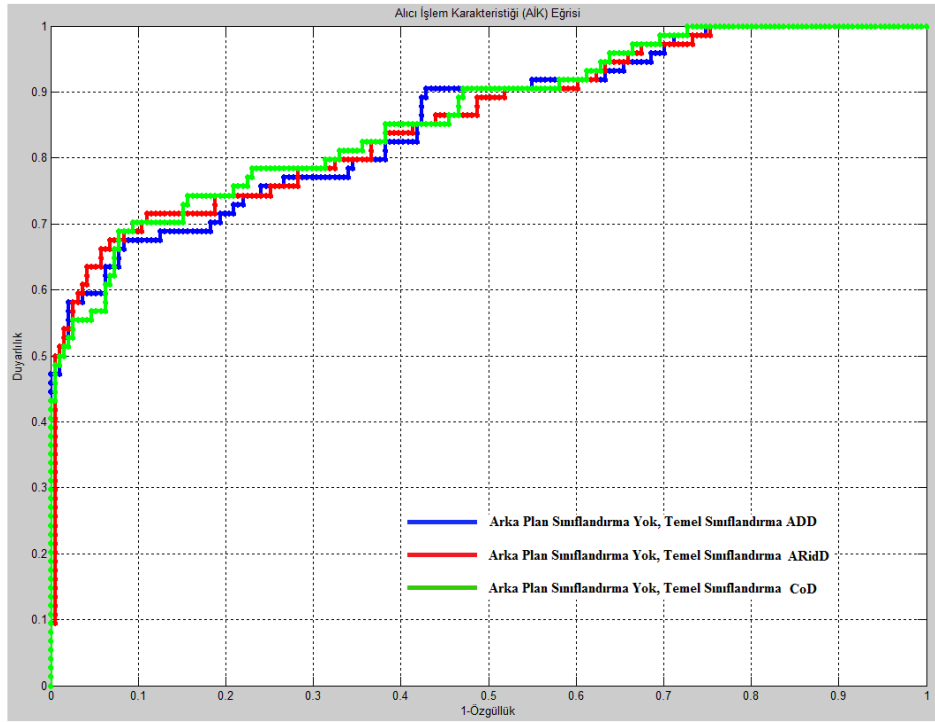
Şekil 4.9. Arka plan doku yoğunluk tipi dikkate alınmadan gerçekleştirilen temel sınıflandırma için AİK eğrileri
