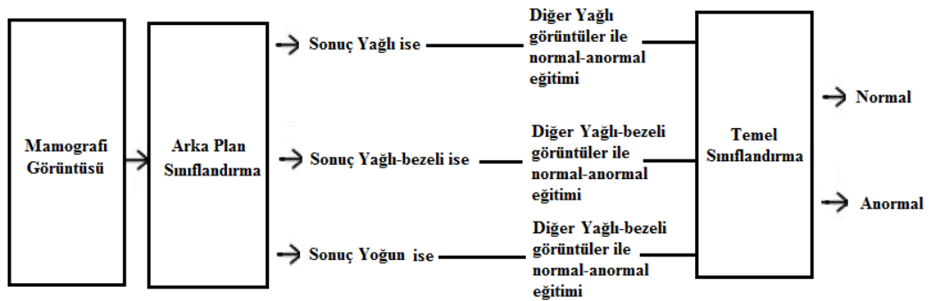
Şekil 4.7. Önerilen sınıflandırma sistemi
