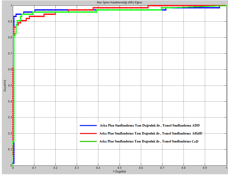
Şekil 4.14. Arka plan sınıflandırma tam doğrulukla yapılarak elde edilen temel sınıflandırma AİK eğrileri
