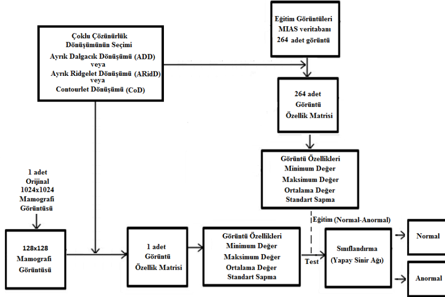
Şekil 4.8. Arka plan doku yoğunluk tipi dikkate alınmadan bir göğüs dokusunun normal-anormal olarak sınıflandırılması
