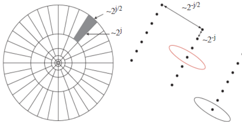
Şekil 2.11. HACuD iki boyutlu frekans düzlemi dilimleri (Candes ve ark., 2005)
