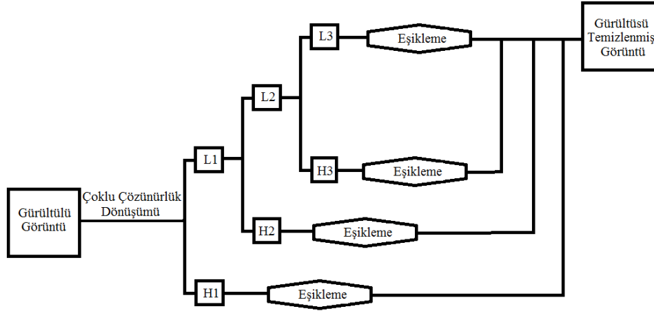
Şekil 4.1. Büzülmeli gürültü temizleme algoritmasının 3. seviye çoklu çözünürlük dönüşümü özellik katsayılarını kullanarak gürültü temizlemesi
