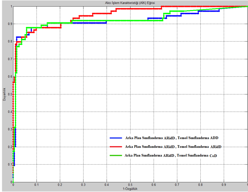
Şekil 4.12. Arka plan sınıflandırma için ARiD ile YSA kullanılarak elde edilen temel sınıflandırma AİK eğrileri
