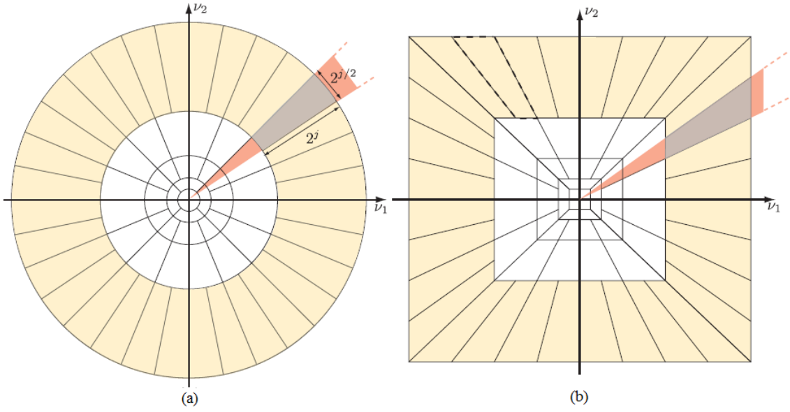
Şekil 2.10. 2NCuD a) sürekli versiyon (kutupsal koordinat sistemi) b) ayrık versiyon (kartezyen koordinat sistemi) radyal ve açısal frekans pencereleri (Donoho ve Duncan, 2000)
