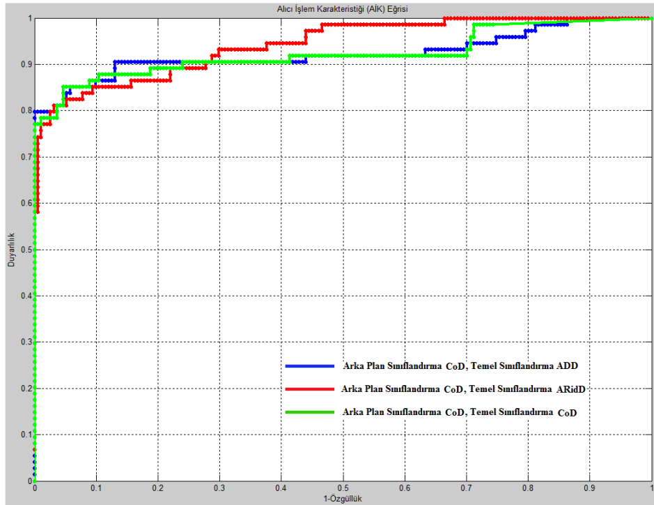
Şekil 4.13. Arka plan sınıflandırma için CoD ile YSA kullanılarak elde edilen temel sınıflandırma AİK eğrileri
