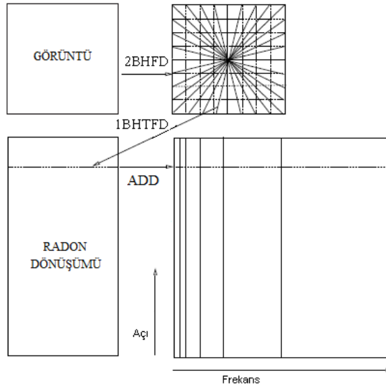
Şekil 2.5. ARidD akış şeması (Fadili ve Starck, 2012)
