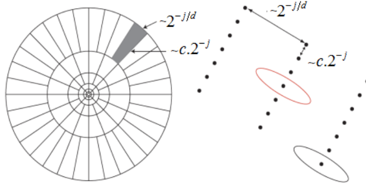
Şekil 2.17. HARip-1D iki boyutlu frekans düzlemi dilimleri
