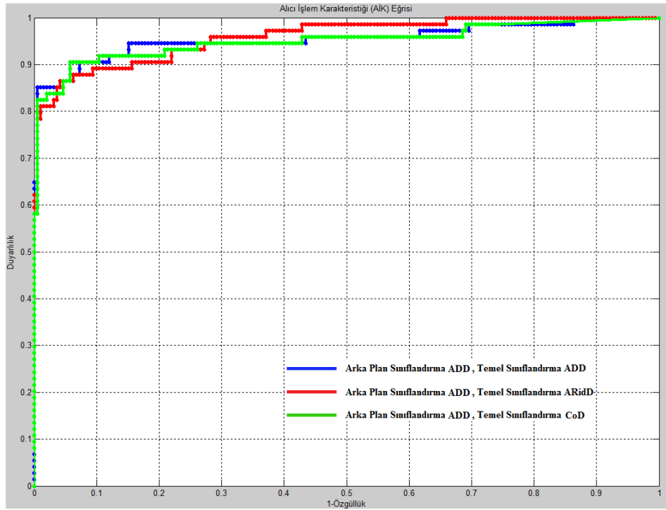
Şekil 4.11. Arka plan sınıflandırma için ADD ile YSA kullanılarak elde edilen temel sınıflandırma AİK eğrileri
