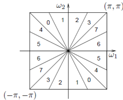
Şekil 2.14. Yönsel filtre kümesi ile frekans bölümlenme ( l=3 ve alt frekans bölümü sayısı 2^l=8 ) (Do ve Vetterli, 2005)
