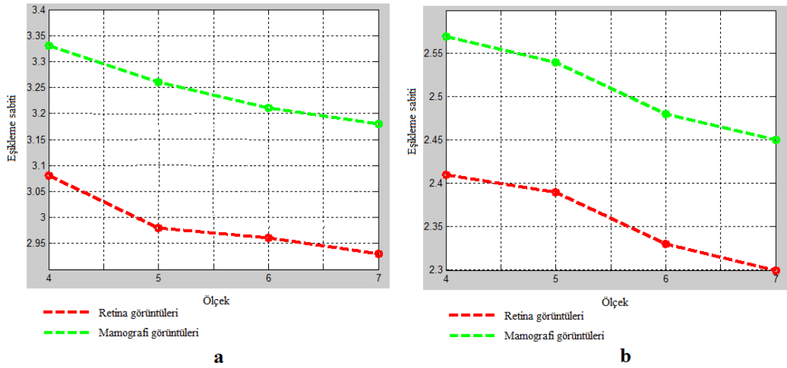
Şekil 5.1. Ölçek değerleri ile en iyi sonucun elde edildiği eşikleme sabiti değerlerinin birbirlerine göre değişimi a) RDHARip-1D özellik katsayıları ile gürültü temizleme b) KDHARip-1D özellik katsayıları ile gürültü temizleme
