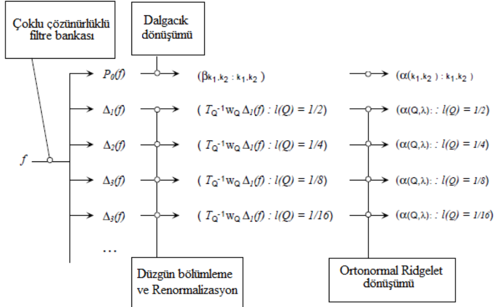
Şekil 2.8. 1NCuD alt basamakları (Donoho ve Duncan, 2000)
