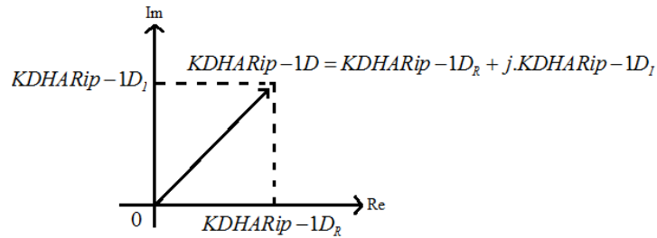
Şekil 2.18. KD HARip-1D özellik katsayılarının oluşumu
