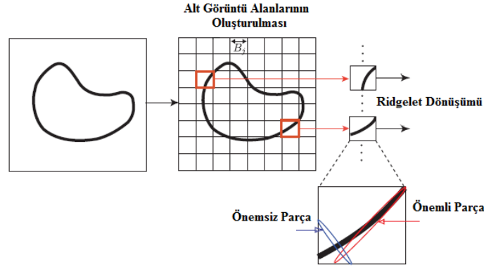
Şekil 2.6. Eğrisel çizgiselliklerin alt görüntü alanlarına bölünerek doğrusallaştırılması ve RidD ile işlenmesi (Candes ve Donoho, 2002)
