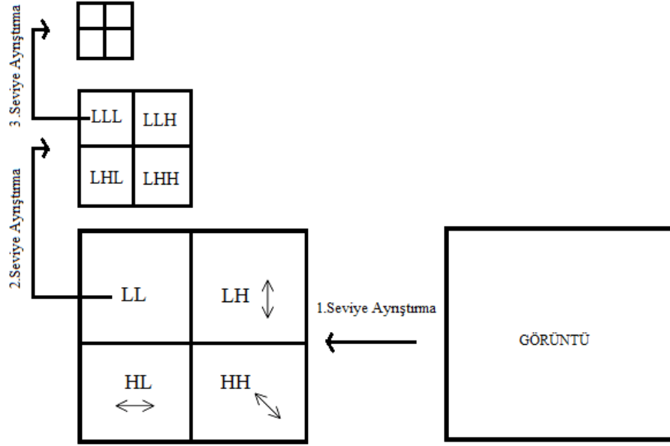
Şekil 2.2. 2BADD çoklu-seviyeli ayrıştırma hiyerarşisi (Ceylan, 2009)
