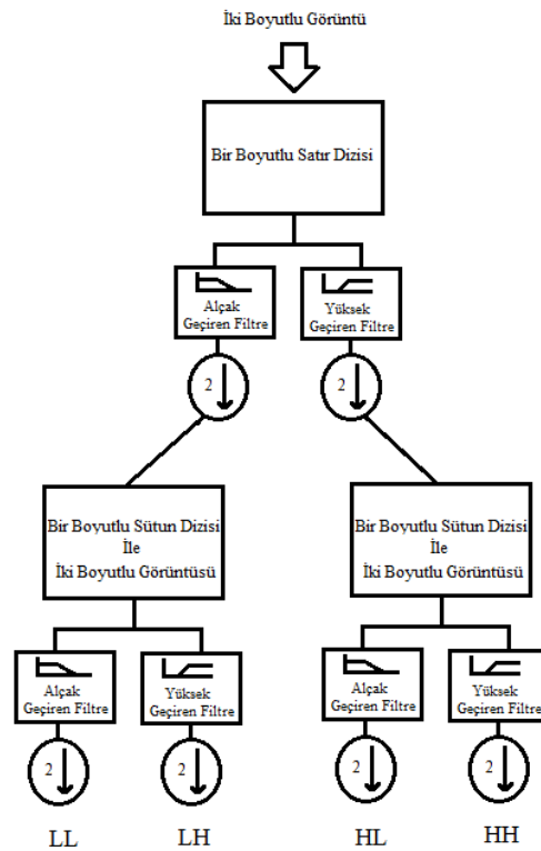
Şekil 2.1. 2BADD için bir seviyeli analiz filtre kümesi (Ceylan, 2009)
