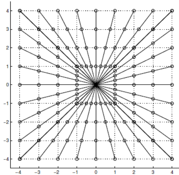
Şekil 2.4. 8×8 boyutlarında ve kartezyen koordinat sistemindeki görüntünün analiz yapılırken kullanılan kutupsal yönleri (Fadili ve Starck, 2012)
