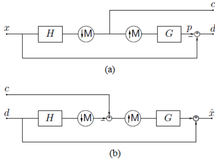
Şekil 2.13. Laplas piramidi şeması a) analiz b) sentez karşılaştırılması (Do ve Vetterli, 2005)
