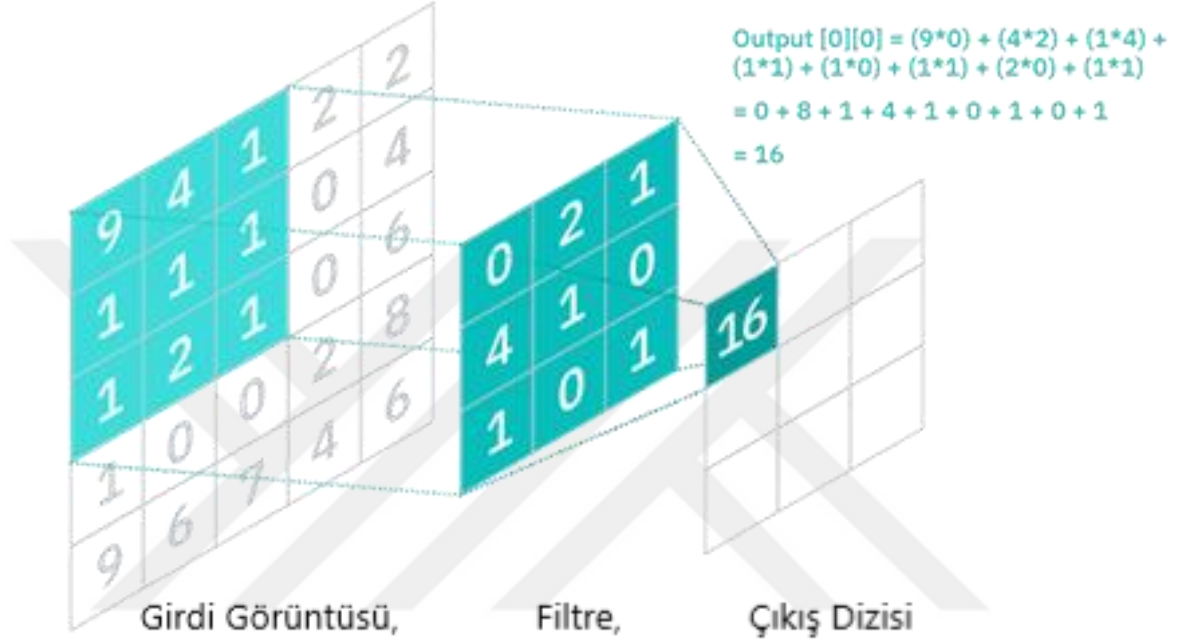
Şekil 3.3. Konvolüsyonel Sinir Ağı
