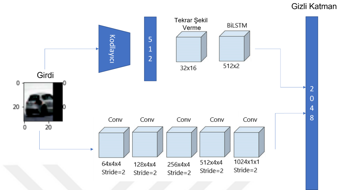
Şekil 3.5.5. Hibrit Model Part 1
