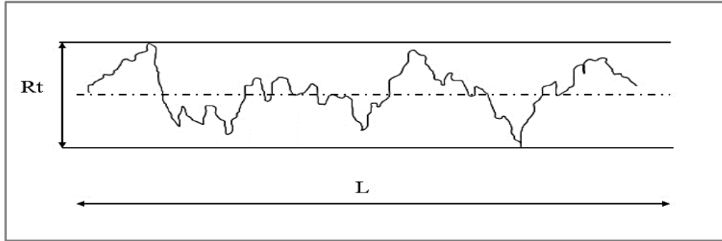
Şekil 3.4. Yüzey pürüzlülük en büyük değeri R_t [46].
