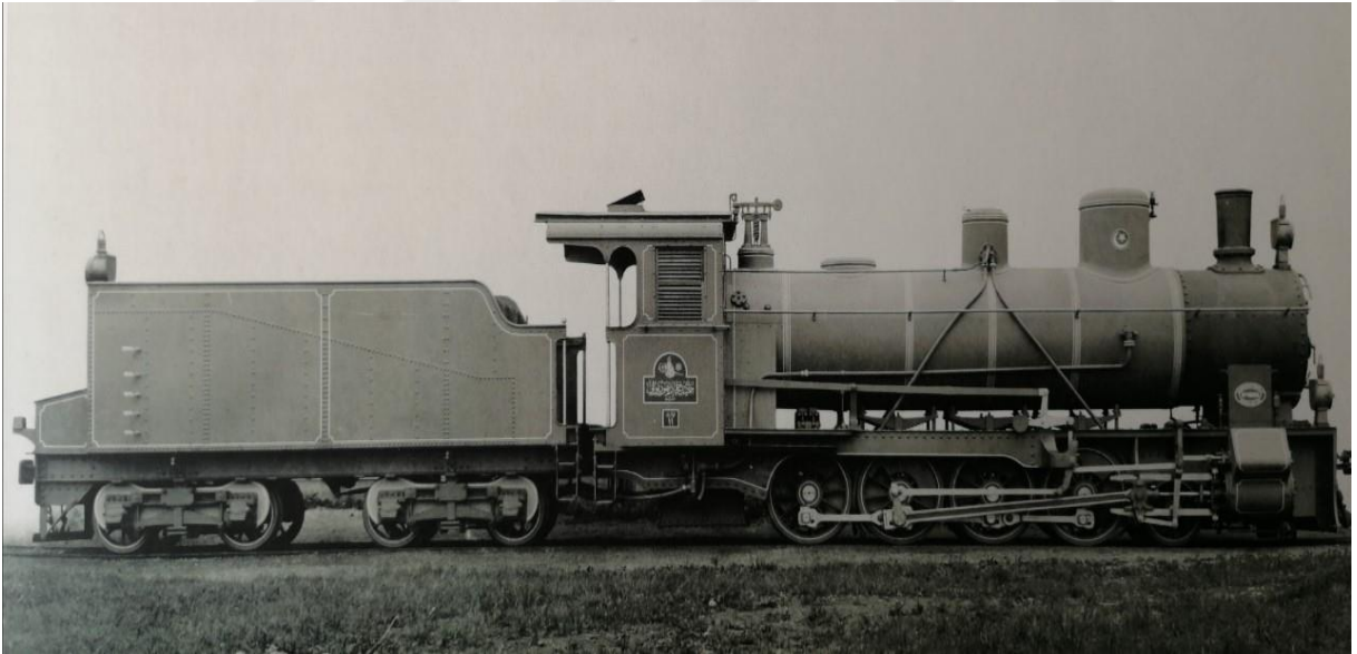
Ek XV – Hamidiye-Hicaz Demiryolu’nun 11 numaralı lokomotifi m. 1892-1893. (Yılmaz, a.g.e, s. 20-21.)
