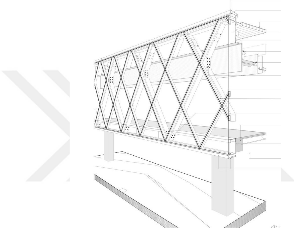
Şekil 1.2.2. Taşıyıcı Sistemli Cephe Örneği
