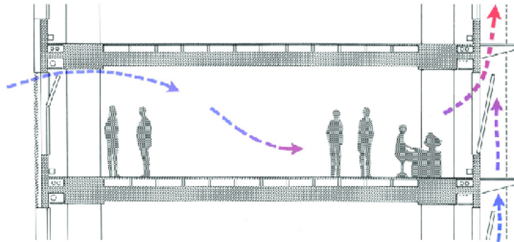
Şekil 5.11.2. GSW Headquarters Pasif Havalandırma Sistemi (url 57)
