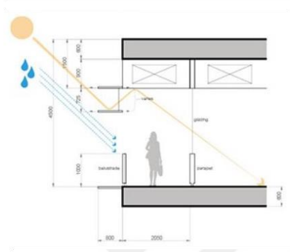
Şekil 3.1.2.3.Cephede Cam Korkuluk Etkisi Etkisi
