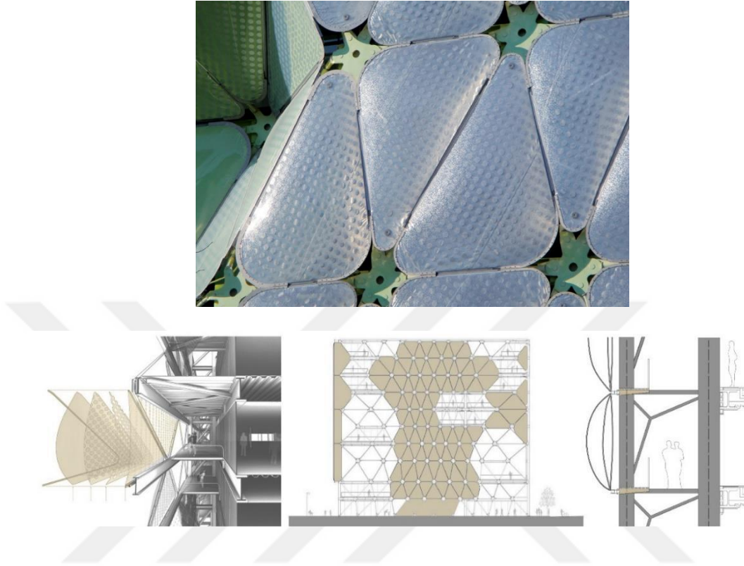
Şekil 5.14.3. Media-TIC Cephe Sistemi Diyagramları (url 17)
