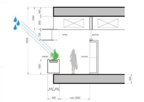
Şekil 3.1.2.5. Cephede Bitki Ögesi Etkisi Etkisi
