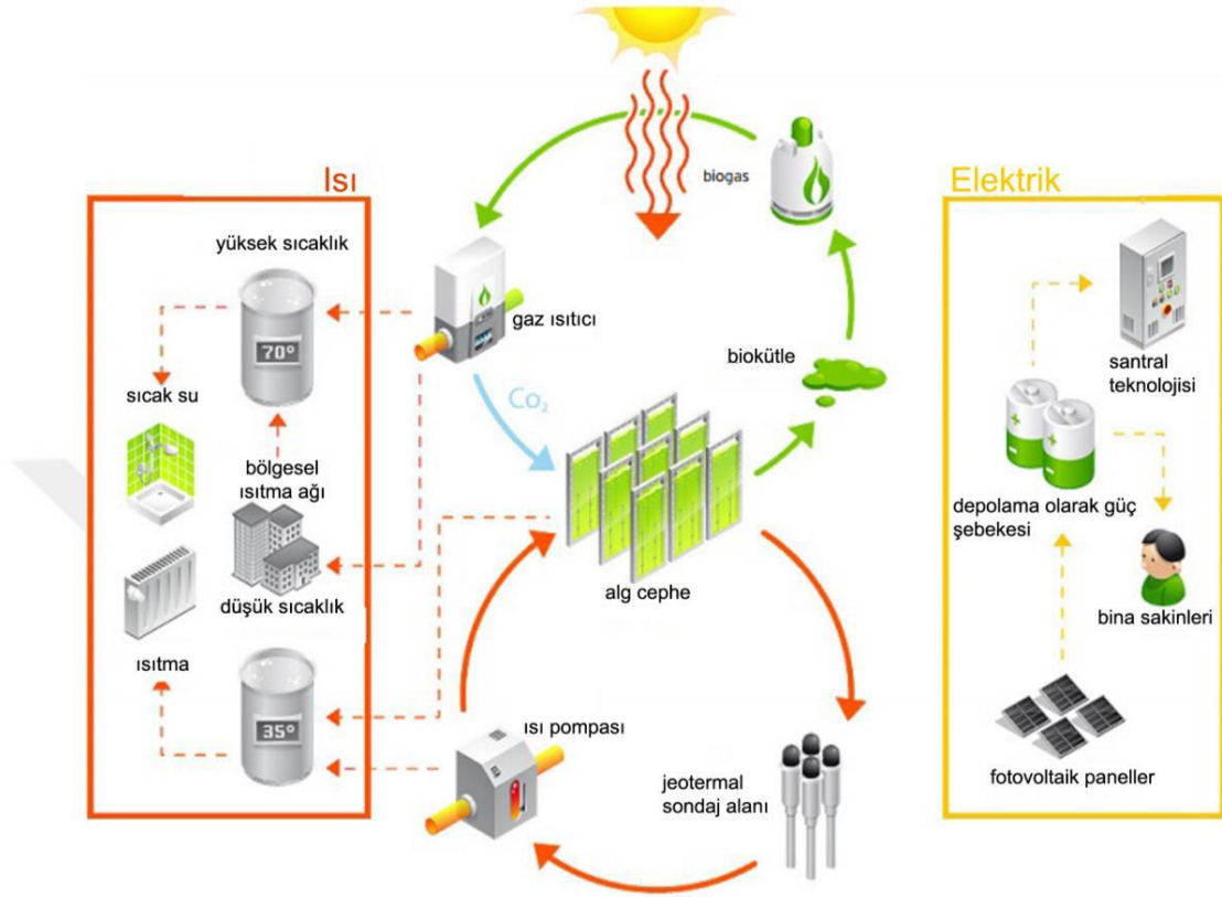
Şekil 4.3.1.4. Bio-Reaktör Cephe Sistem Şeması (url 47)
