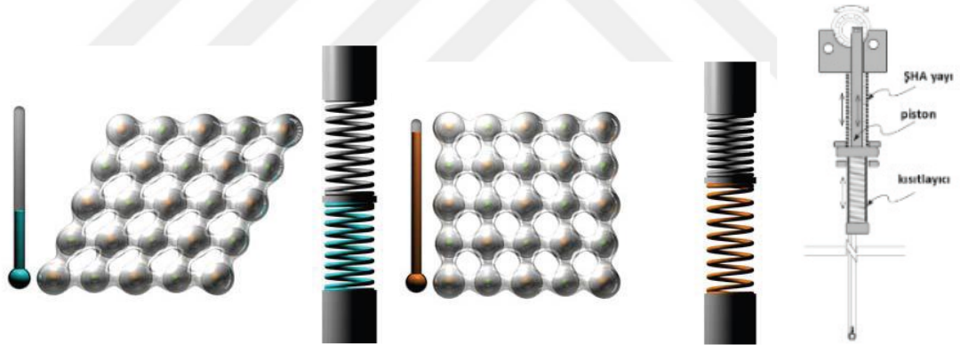
Şekil 4.3.1.7. Smartscreen Sisteminde R-Faz ŞHA, Sıcaklık Değişiminin Etkisi ve Sınırlayıcılar (Decker, Yeadon, 2008)
