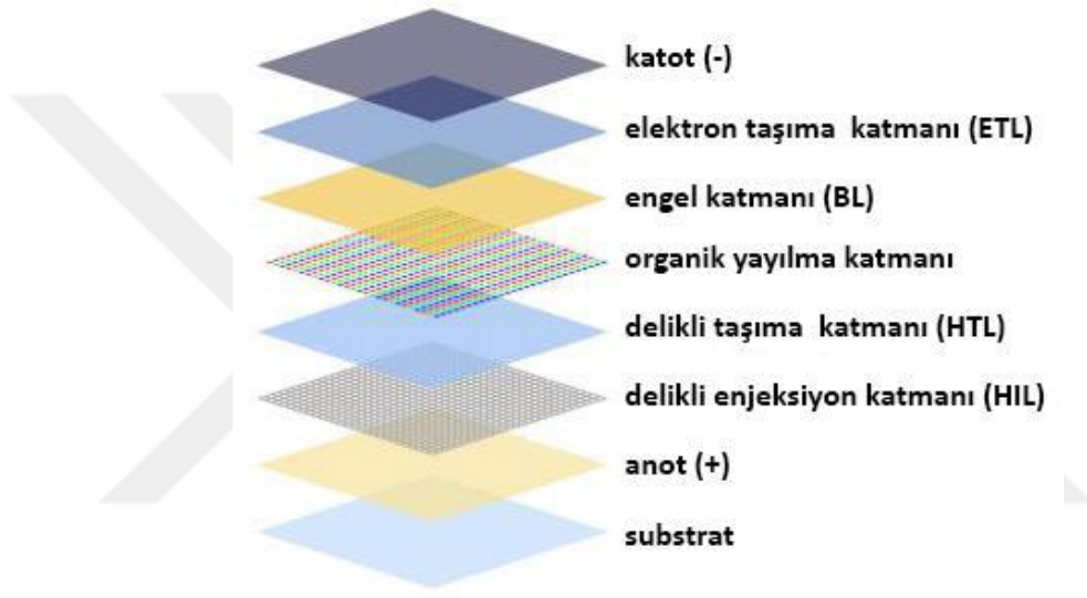
Şekil 3.3.13. OLED Katmanları (url 24)
