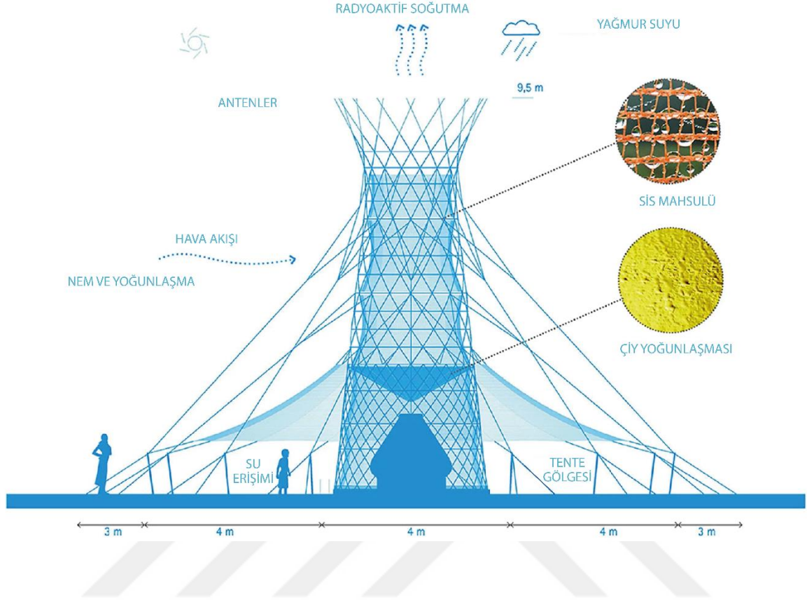
Şekil 3.4.2. Warka Kulesi Şematik Gösterim (url 32)
