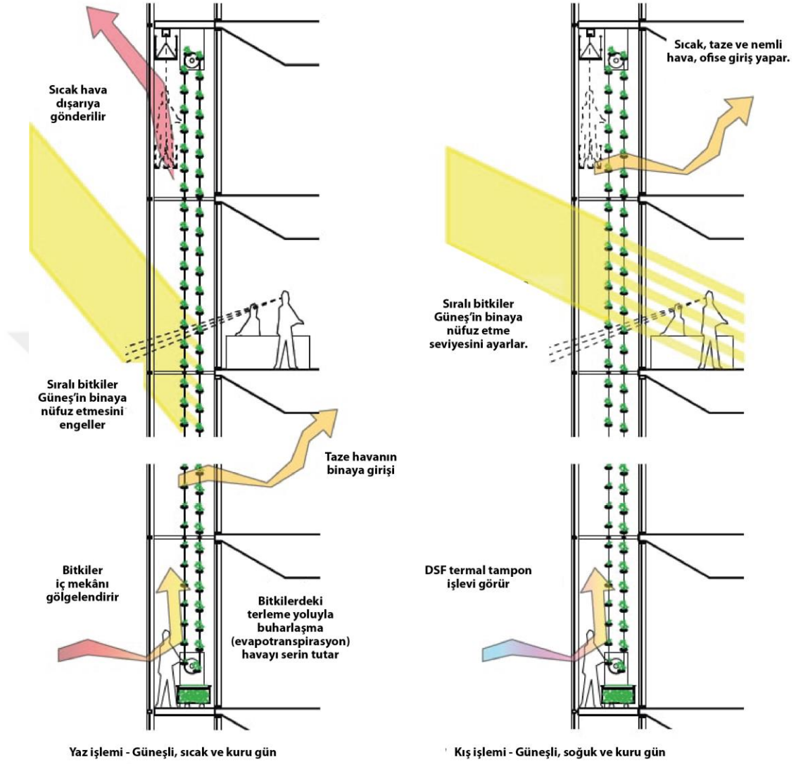
Şekil 4.3.2.1. Cephede Sera Uygulaması ve HVAC Sistemi Arasındaki İlişki (url 30)
