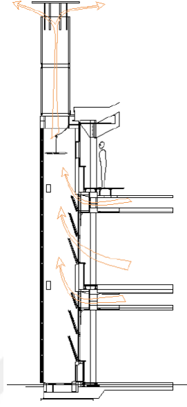
Şekil 3.3.5. BRE Ofis Binası Havalandırma Şeması (Arslantatar 2006, s. 66)
