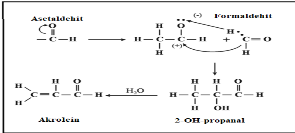
ekil 3.13. Basit aldehitlerin rekombinasyonu sonucu akrolein eldesi [60].
