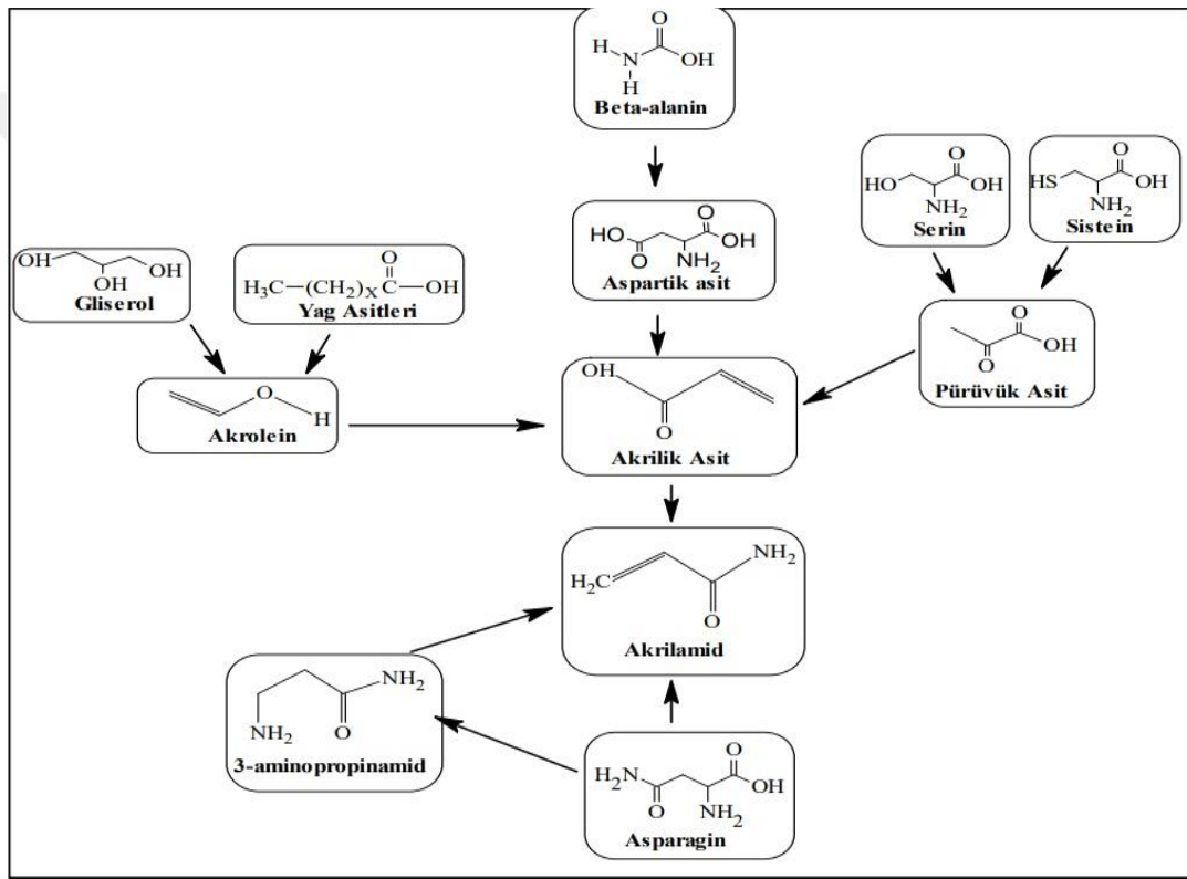
Şekil 3.2. Gıdalarda akrilamidin oluşum yolları [59].
