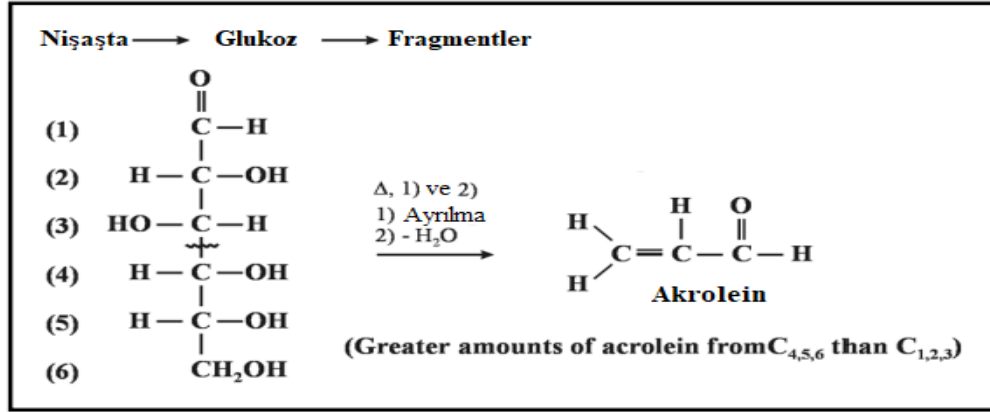
ekil 3.12. Niatanın paralanması ile akrolein eldesi [60].
