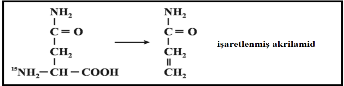
Şekil 3.6. Basamak 2: \alpha -amino grubunun akrilamid oluşumuna katılmadığını gösteren tepkime [61].
