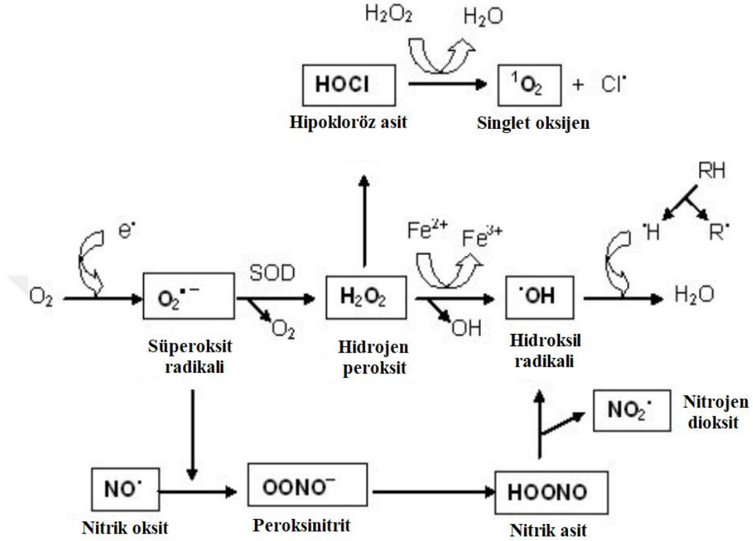
Şekil 5.1. Başlıca ROT ve RNT’ler [138].
