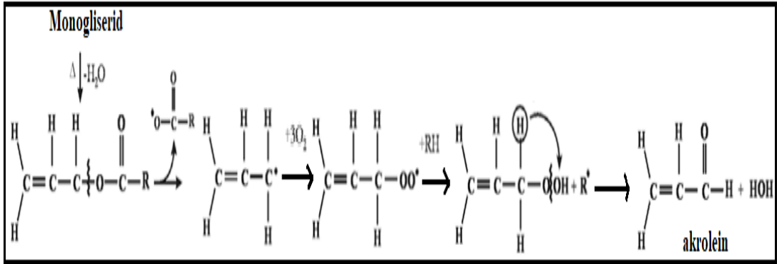
Şekil 3.11. Monoglisericidün oksidasyonu ile akrolein oluşumu [60].
