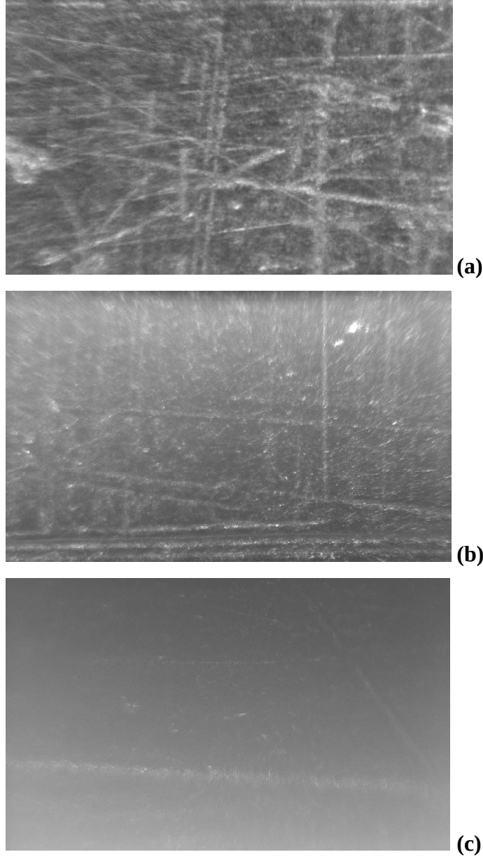
Şekil 6.3 : Üç aşamalı parlatılmış alüminyum yüzeyi görüntüleri. (a) başlangıç, (b) ilk parlatma, (c) pasta işlemi sonrası.
