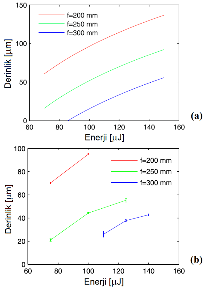
Şekil 7.15 : Farklı odaklamalar için ilerleme derinliği değişimi
