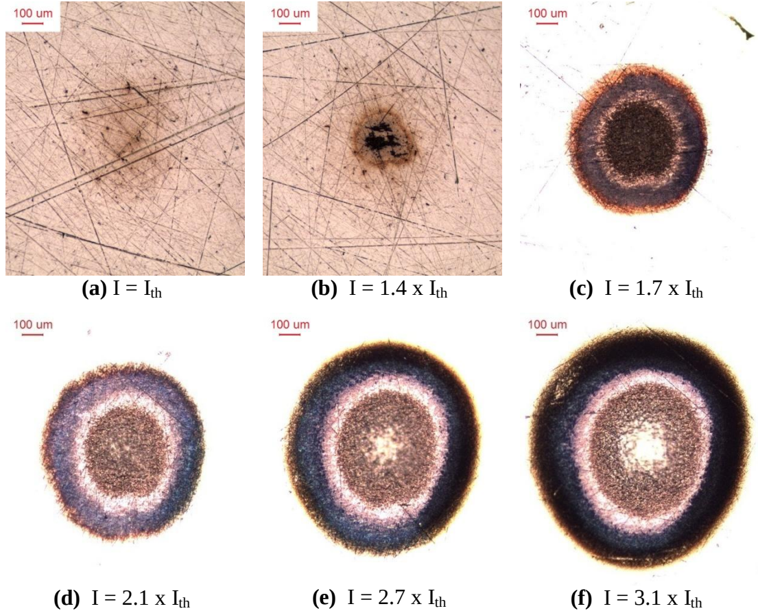
Şekil 7.9 : Bakırda farklı şiddetlerde açılan deliklerin mikroskop görüntüleri.
