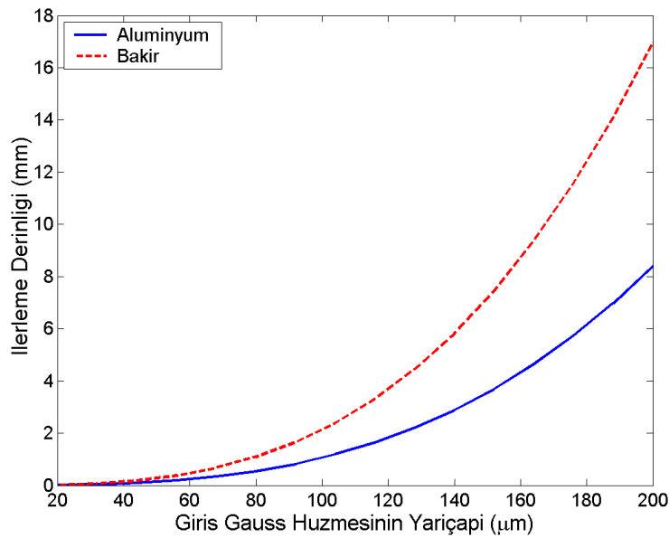
Şekil 5.9 : Farklı eğrilik çaplı huzmelerin ilerleme hesaplamaları ( I=1.5 \times I_{th} ).
