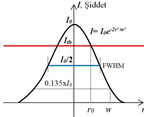
Şekil 5.1 : Gauss huzmeleri için dağılama yarıçapının huzme şiddetine bağımlılığı.
