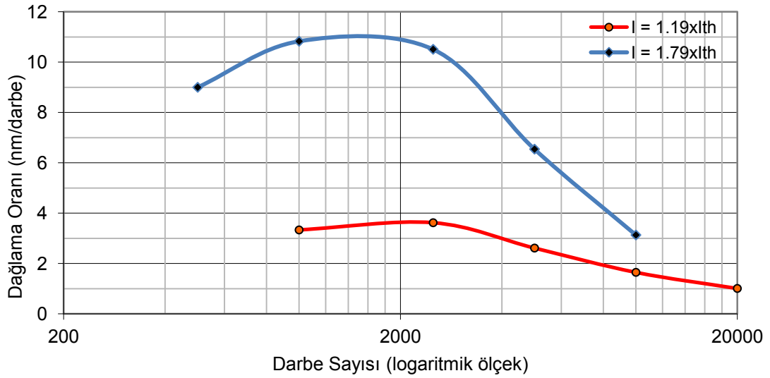
Şekil 6.18 : Bakırda dağlama oranının darbe sayısına göre değişimi.
