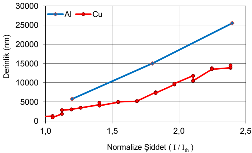
Şekil 7.10 : 250 mm odaklı Gauss huzmesinin bakır ve alüminyumda ilerlemesi.
