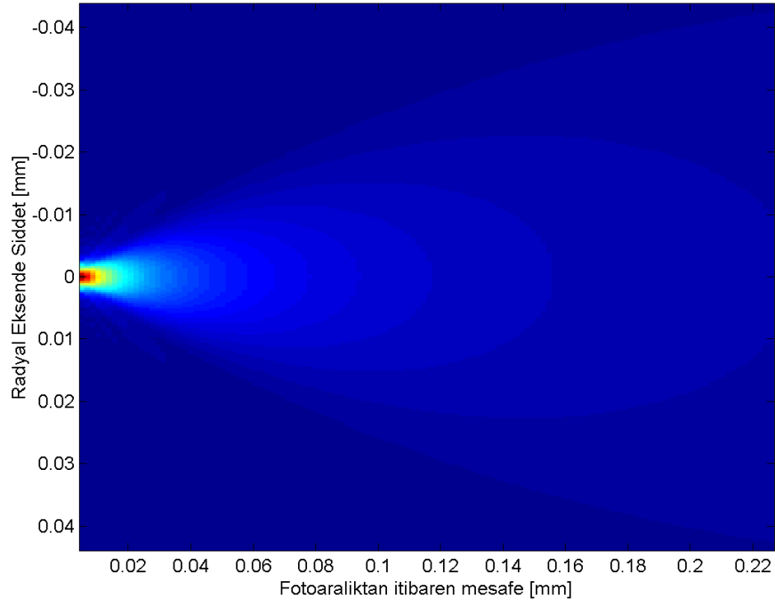
Şekil 4.9 : Fotoaralık sonrası açılma.
