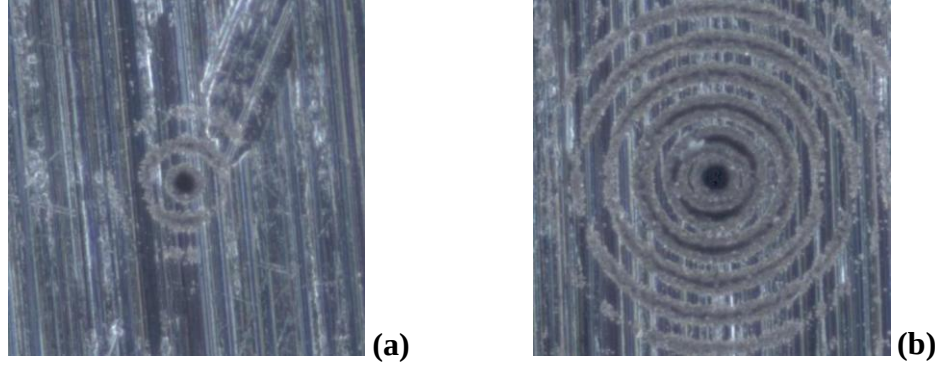
Şekil 6.24 : Alüminyumda konik mercek dağlaması (#1000 darbe). (a) 25 mW, (b) 100 mW.
