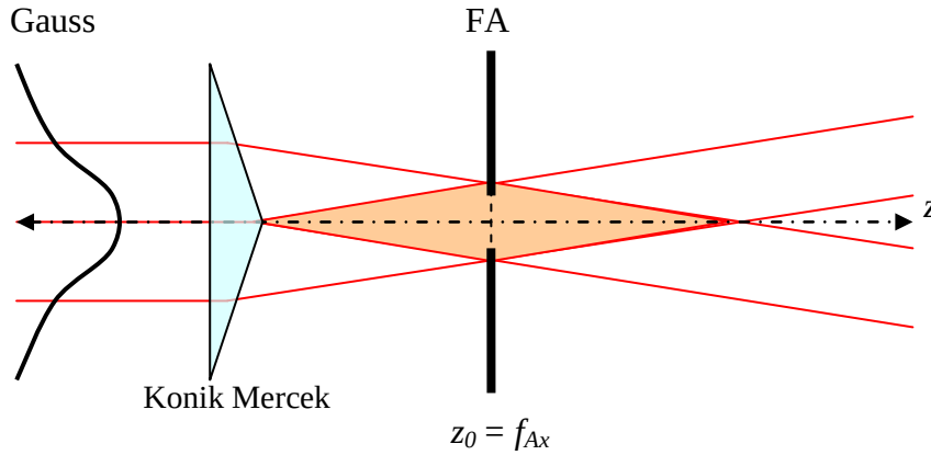
Şekil 4.8 : 'Aksikon' ile odaklanan lazer huzmesinin fotoaralıktan geçişi.
