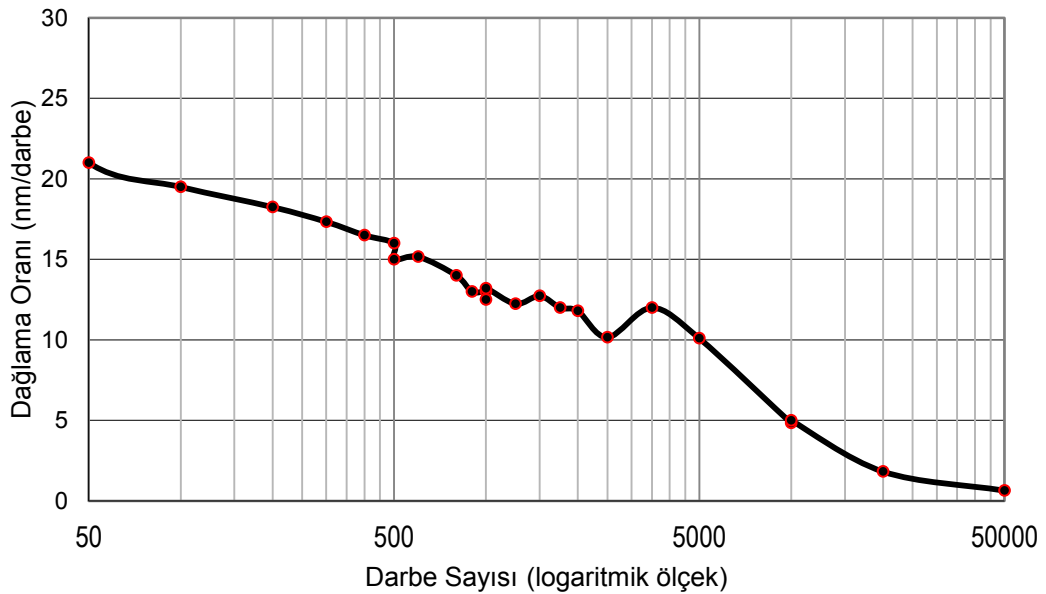
Şekil 6.16 : Alüminyumda dağlama oranının darbe sayısına göre değişimi.
