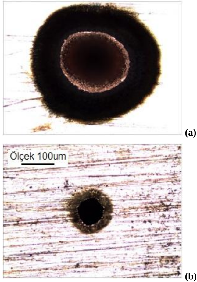
Şekil 6.26 : 0.1 mm kalınlıklı bakır numunede açılan geçen delik görüntüleri. f = 200 mm, P=125 mW (a) üstten görünüm (b) alttan görünüm.
