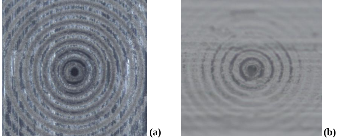
Şekil 6.10 : Alüminyumda bir Bessel huzmesi deliği (a) ve replikası (b).
