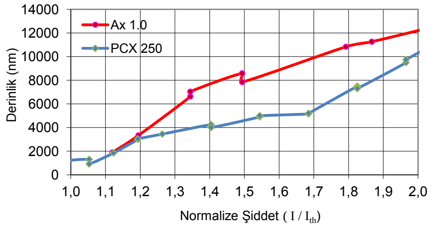
Şekil 8.1 : Gauss ve Bessel huzmelerinin bakırda dağlama derinlikleri.
