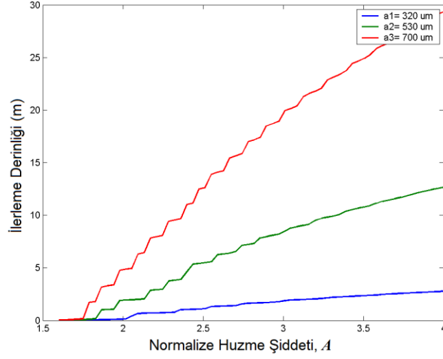
Şekil 5.2 : Gauss huzmelerinin bakırda teorik ilerleme mesafesi analizi.
