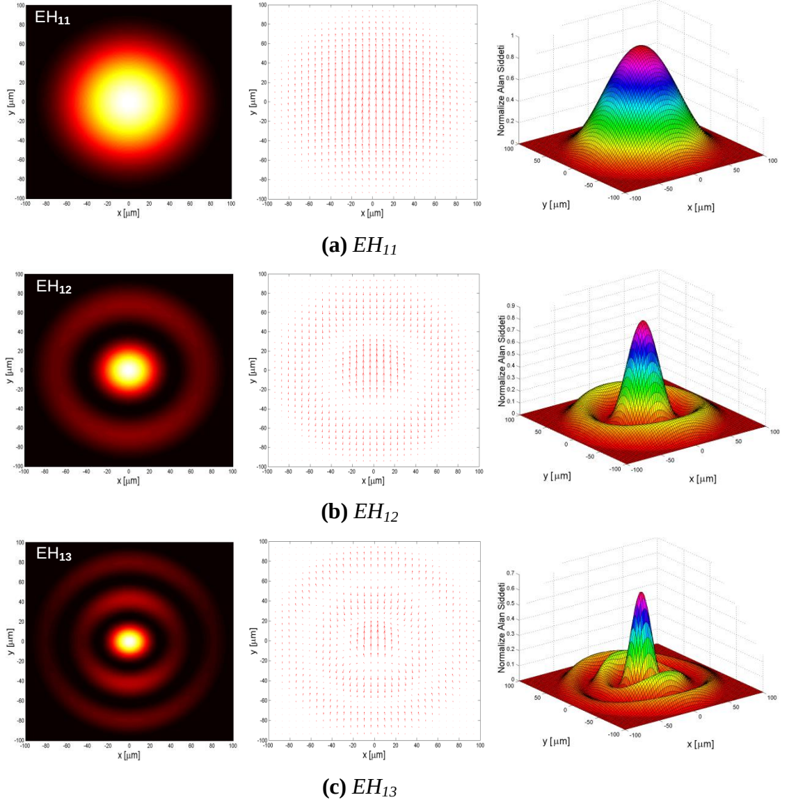
Şekil 3.6 : Temel ilk üç EH_{1m} hibrit modları şiddet dağılımları, alan çizgileri ve üç boyutlu şiddet profil gösterimleri.
