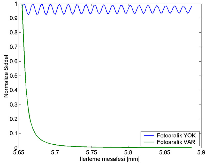
Şekil 4.10 : Yatay profillerin karşılaştırılması.
