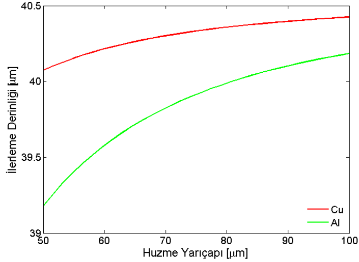
Şekil 7.13 : Farklı boyutlu huzmelerin ilerleme analizi ( I=1.5 \times I_{th} ).
