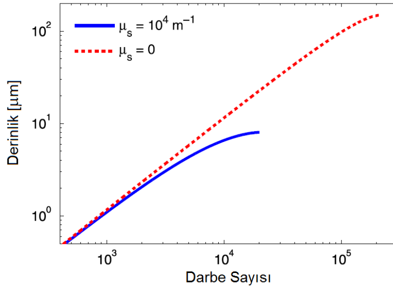
Şekil 7.5 : Bakırda darbe sayısına göre dağlama derinliği değişimi.
