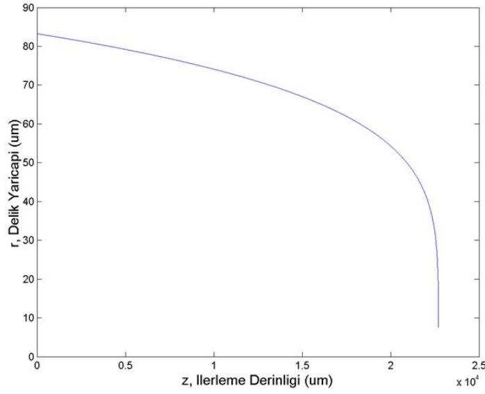
Şekil 5.4 : Gauss tipi huzmenin bakırda sönümlü ilerleme kesiti.
