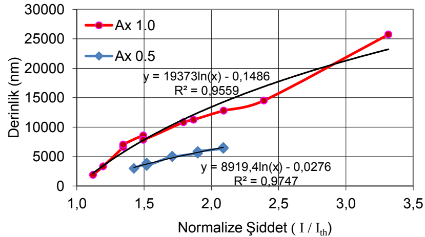
Şekil 6.25 : Bakırda eşik dağlama değerinin belirlenmesi (Konik mercek).
