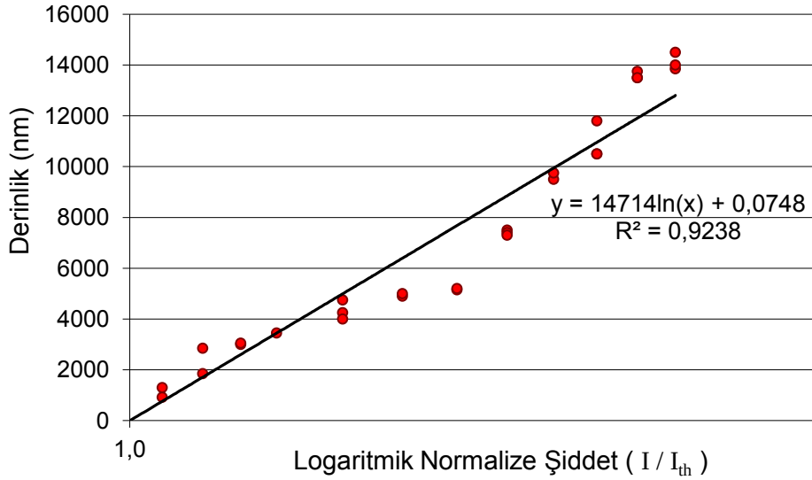
Şekil 6.23 : Bakırda eşik şiddeti değerinin belirlenmesi ( f = 250 mm).
