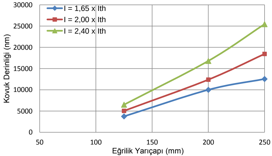
Şekil 7.14 : Alüminyumda farklı boyutlu huzmelerin derinlik analizi.
