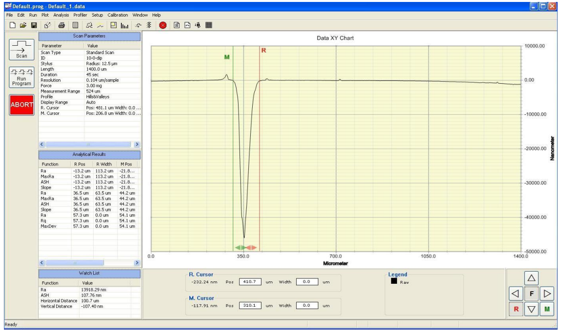
Şekil 6.13 : Bakırda 46 µm derinlikli ve 101 µm çaplı profil ölçümü ( I=1.33 \times I_{th} ) .
