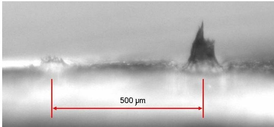
Şekil 6.11 : Replika yöntemi ile elde edilmiş açılı negatif derinlik profilleri.
