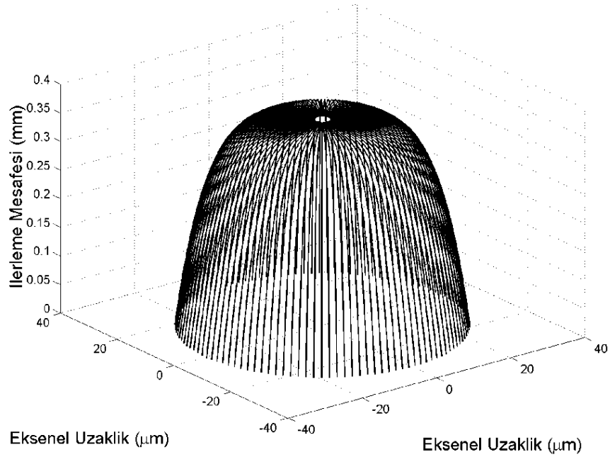
Şekil 5.6 : Gauss tipi huzme deliğinin 3-boyutlu gösterimi.
