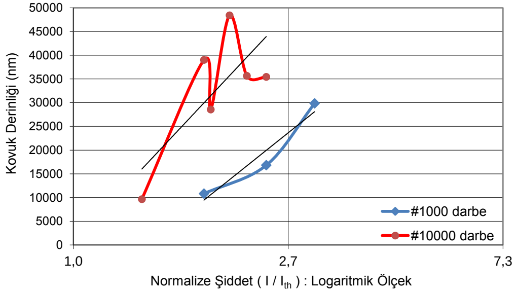
Şekil 6.20 : Eşik dağlama değerinin grafiksel belirlenmesi.
