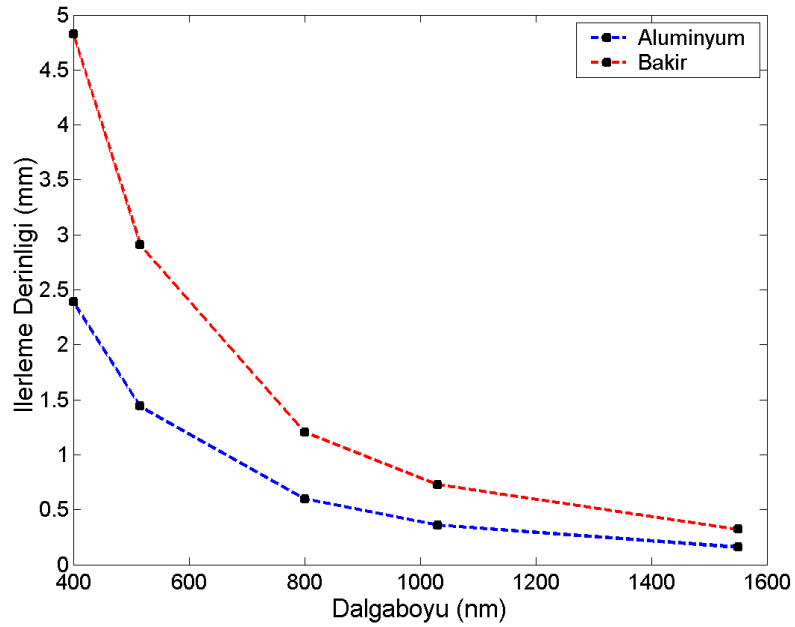
Şekil 5.10 : Dalgaboyunun ilerlemeye etkisi.
