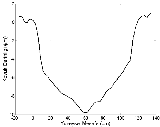
Şekil 6.14 : Delik profili yakın gösterimi.
