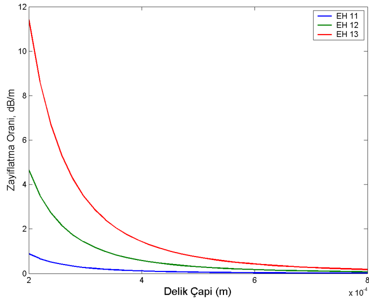
Şekil 3.10 : Mod zayıflama oranları.
