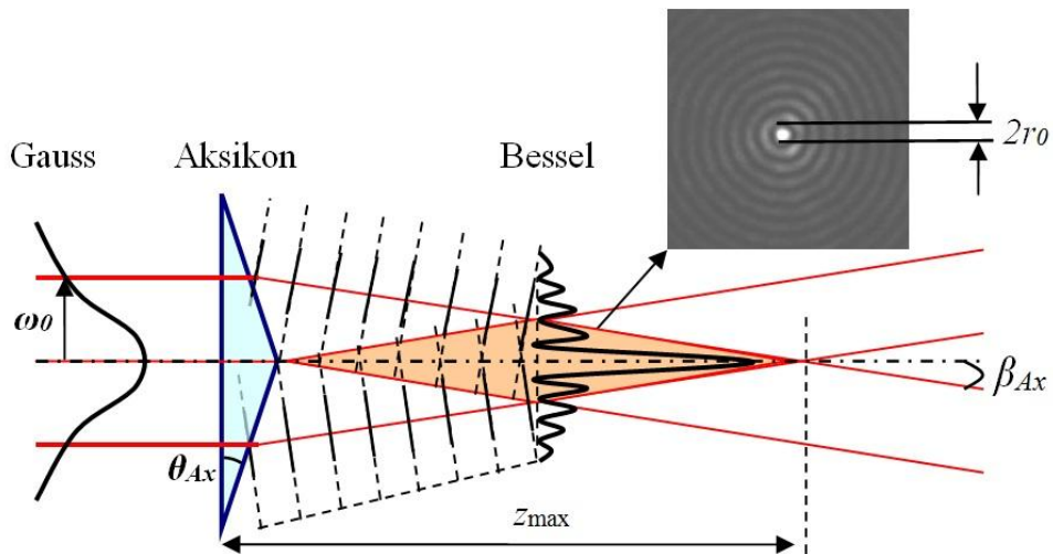
Şekil 4.6 : Konik mercek ile Bessel huzmesi oluşturulması.
