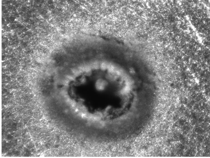
Şekil 6.6 : Alüminyumda derin bir dağlama deliği kenarında birikinti.
