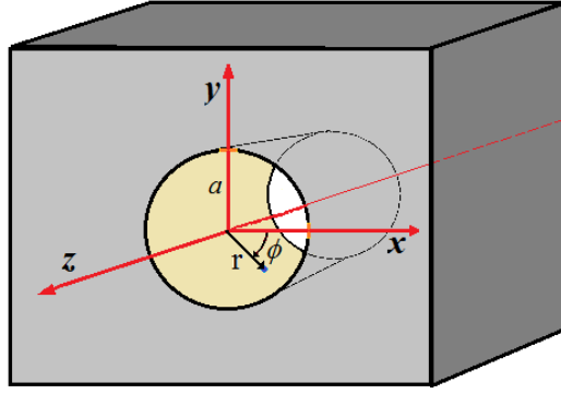
Şekil 3.1 : Silindirik dalgakılavuzunda koordinatlar.
