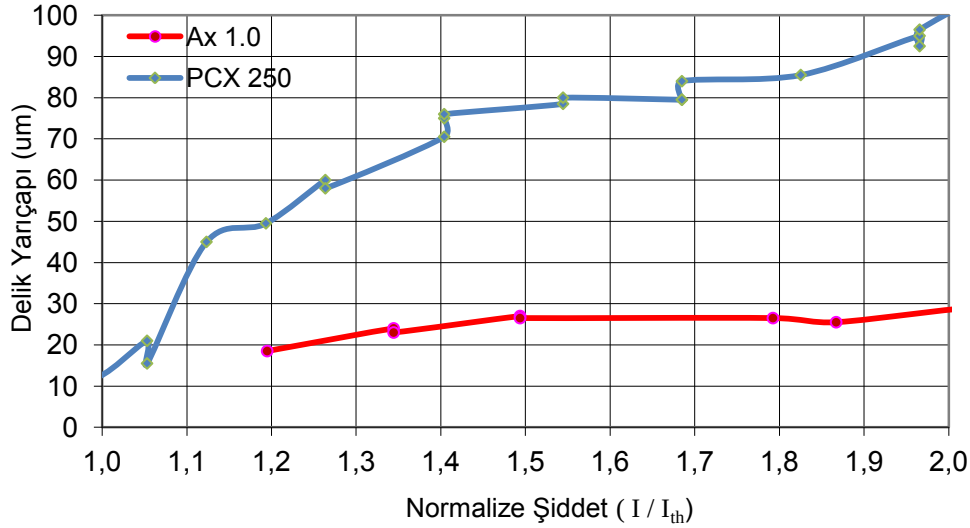
Şekil 8.2 : Gauss ve Bessel huzmelerinin bakırda dağlama yarıçapları.
