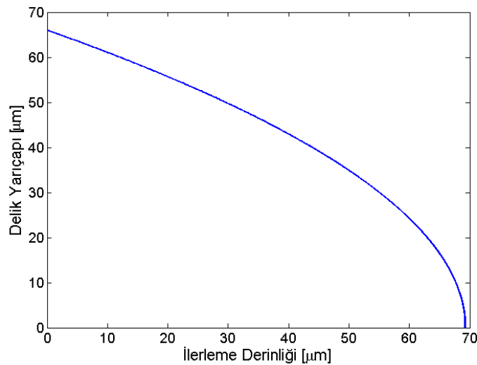
Şekil 7.2 : Gauss tipi huzmenin bakırda sönümlü ilerlemesi ( I=2.0 \times I_{th} ).
