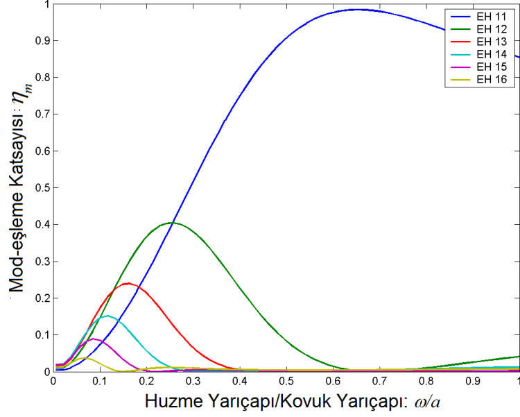
Şekil 3.7 : Gauss tipi huzme için mod-eşleme katsayıları.
