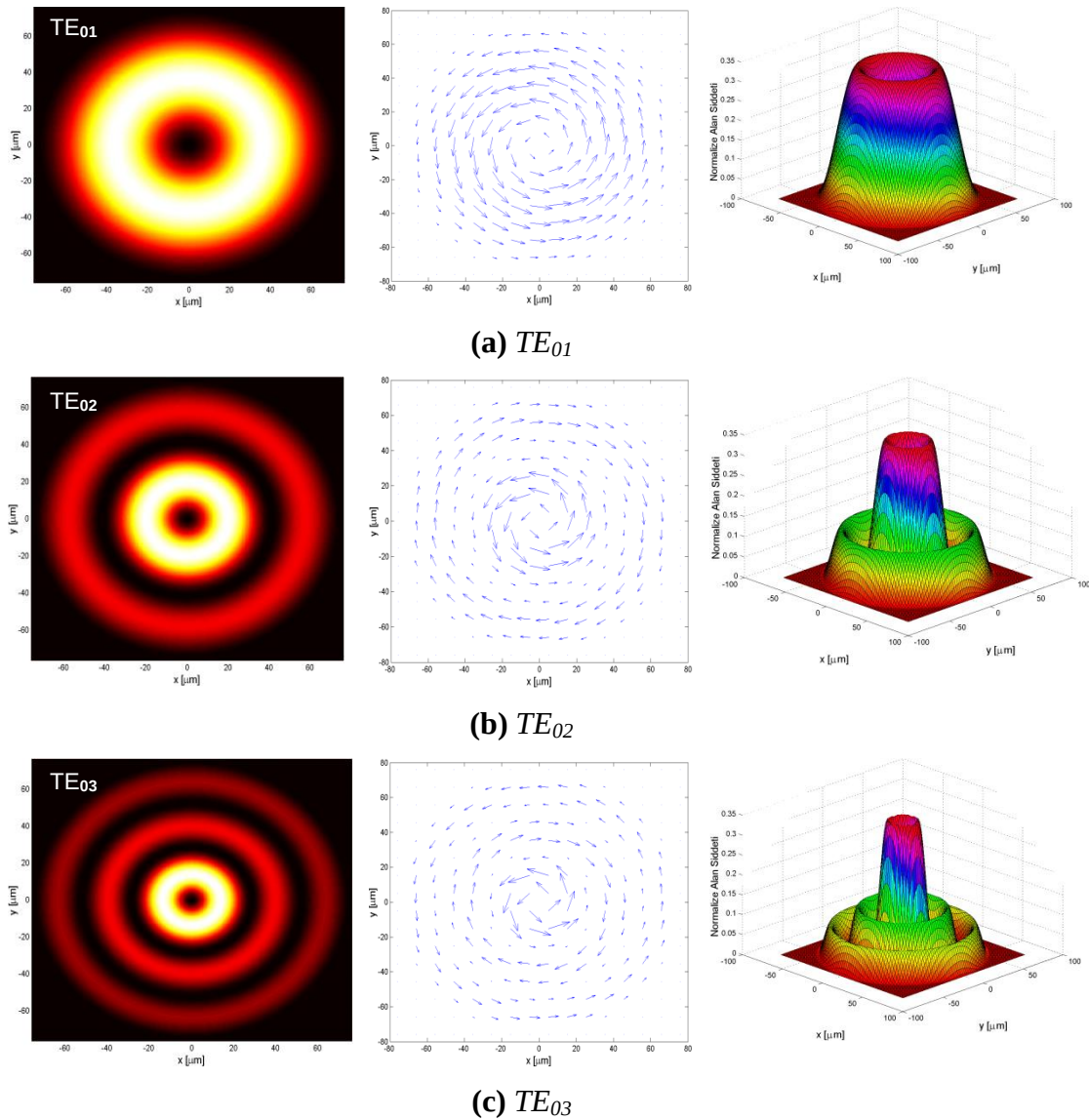
Şekil 3.3 : Bazı TE_{0m} dairesel modları şiddet dağılımları, alan çizgileri ve üç boyutlu şiddet profil gösterimleri.
