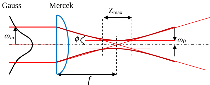
Şekil 4.2 : Gauss huzmesinin ince kenarlı merceklerle odaklanması.
