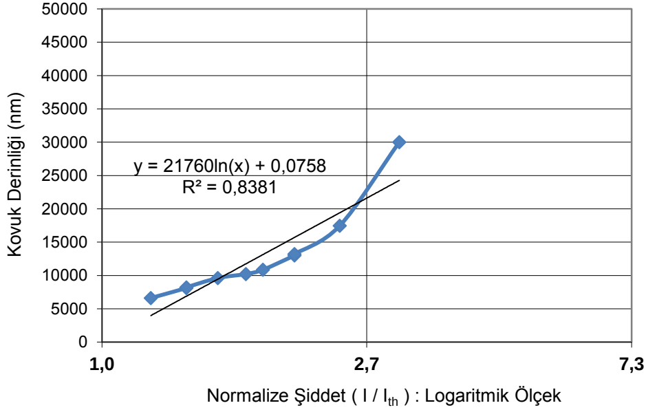
Şekil 6.21 : Alüminyumda eşik dağlama değerinin belirlenmesi ( f=200 mm).
