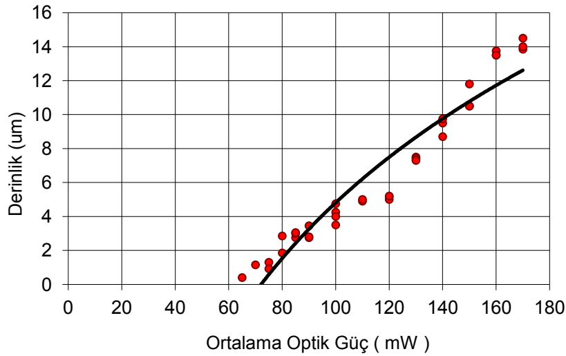
Şekil 6.19 : Dağlama eşiğinin belirlenmesi.
