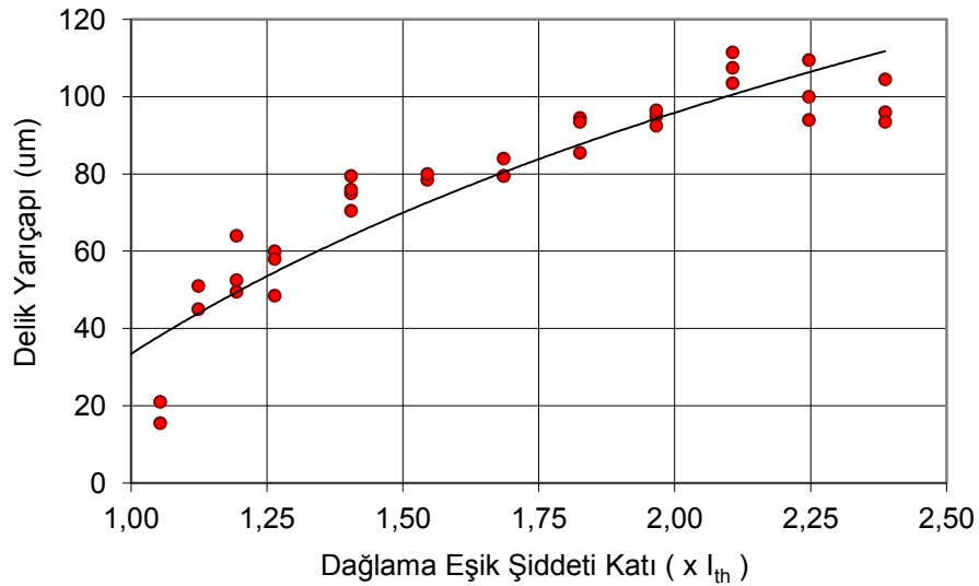
Şekil 7.11 : Bakırda farklı şiddetle açılmış deliklerin yarıçap analizi ( f=250 mm).
