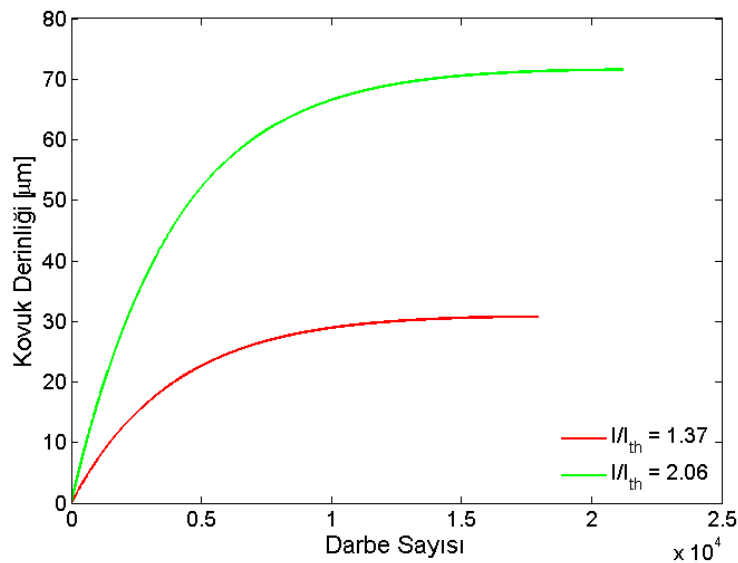
Şekil 7.7 : Kovuk derinliğinin darbe sayısı ile değişimi hesaplaması.
