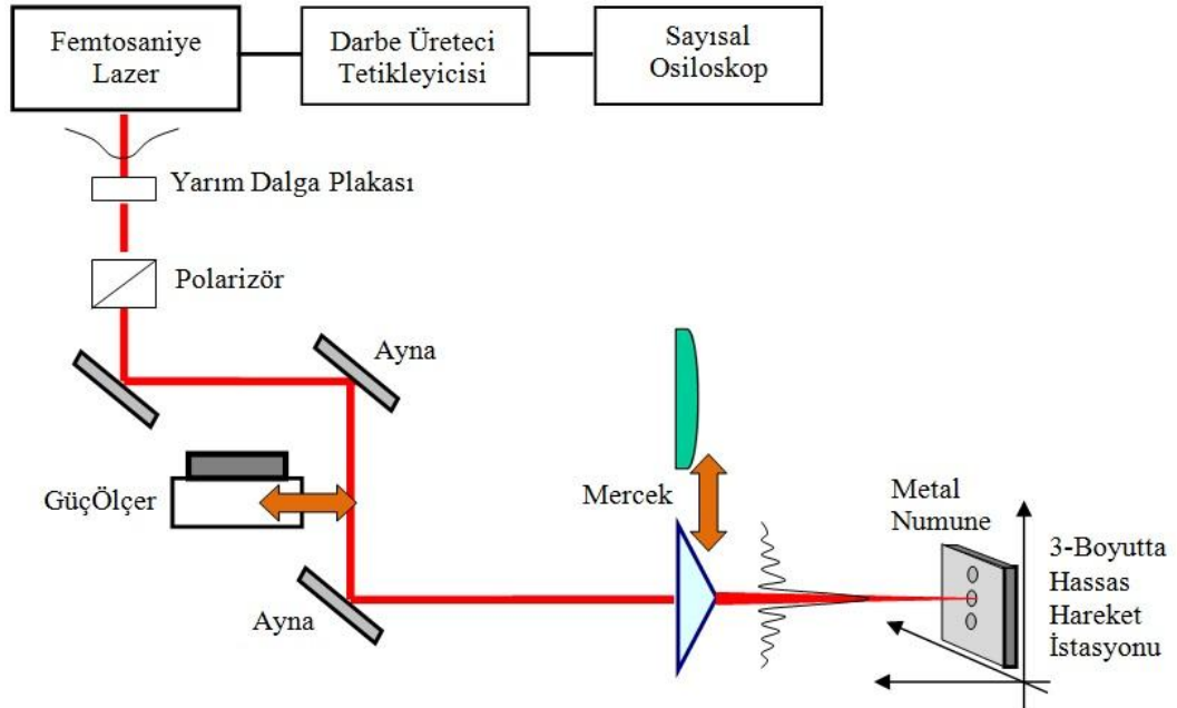
Şekil 6.1 : Femtosaniye lazerle metal işleme optik düzeneği.
