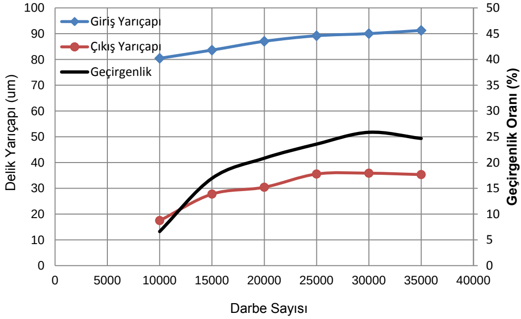
Şekil 6.27 : Bakırda açılan deliklerin boyutları ve huzme geçirme oranı değişimi.
