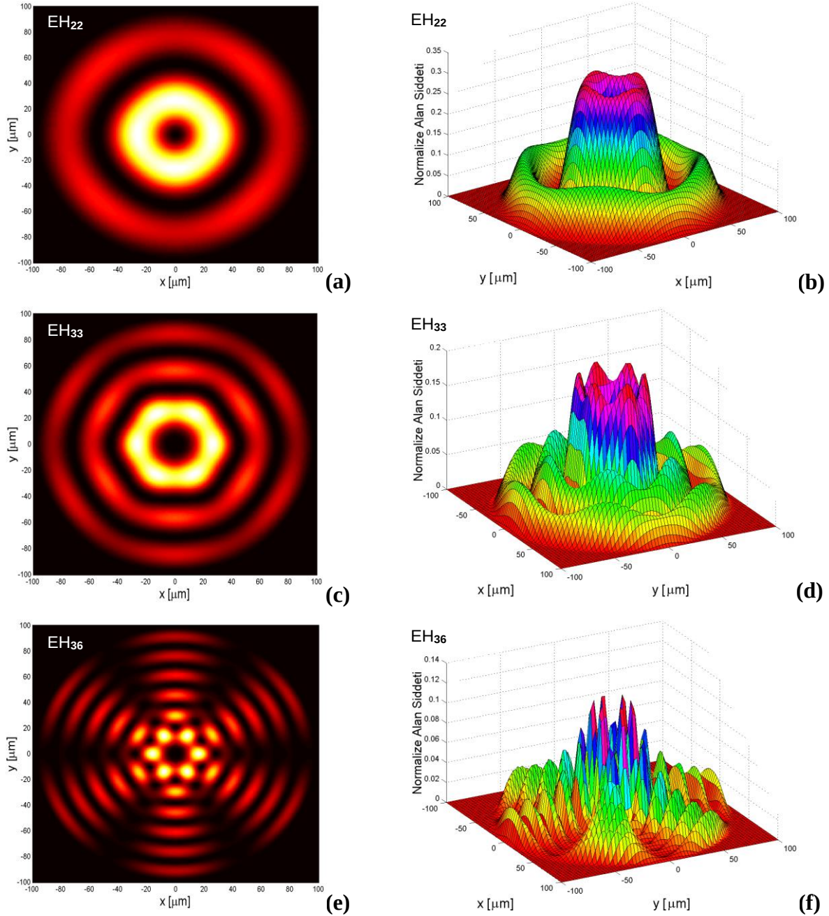
Şekil 3.5 : Bazı karmaşık EH hibrit mod şiddet dağılımları ve üç boyutlu şiddet profili gösterimleri.
