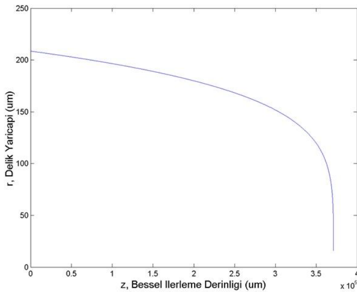
Şekil 5.5 : Bessel tipi huzmenin sönümlü ilerleme kesiti.
