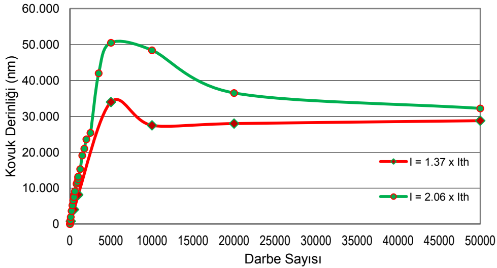
Şekil 7.4 : Alüminyumda kovuk derinliğinin darbe sayısı ile değişimi.
