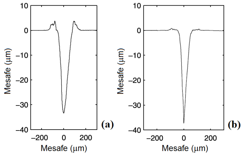
Şekil 7.1 : Bakırda (a) A=3.5 şiddetli 2500 darbe ve (b) A=1.4 şiddetli 15000 darbe ile açılan kovuk profilleri.
