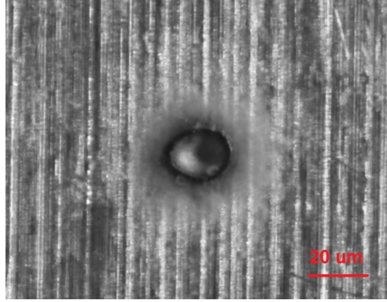
Şekil 6.4 : Alüminyumda Gauss huzmesi ile oluşan dağlama kovuğu.
