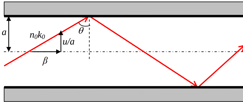
Şekil 3.9 : Boş kılavuz için optik geometrisi.
