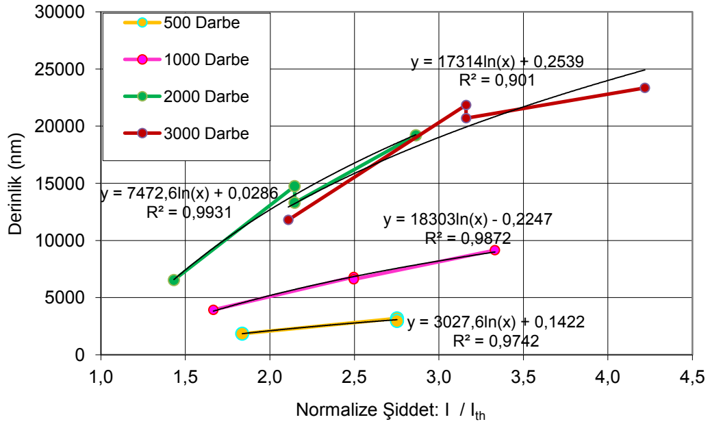
Şekil 6.22 : Alüminyumda eşik dağlama değeri (f=125 mm).
