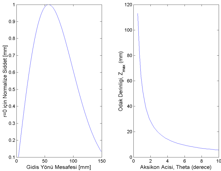
Şekil 4.5 : Merkezi bessel huzmesi şiddeti ve odak derinliğinin değişimi.
