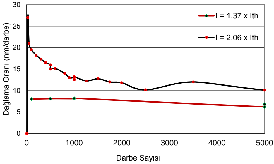
Şekil 6.15 : Alüminyumda dağlama oranının uygulanan şiddete göre değişimi.
