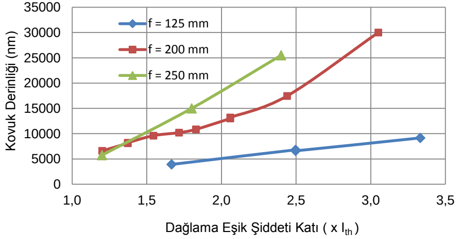
Şekil 7.12 : Alüminyumda farklı şiddetli ve boyutlu huzmelerin derinlik analizi.
