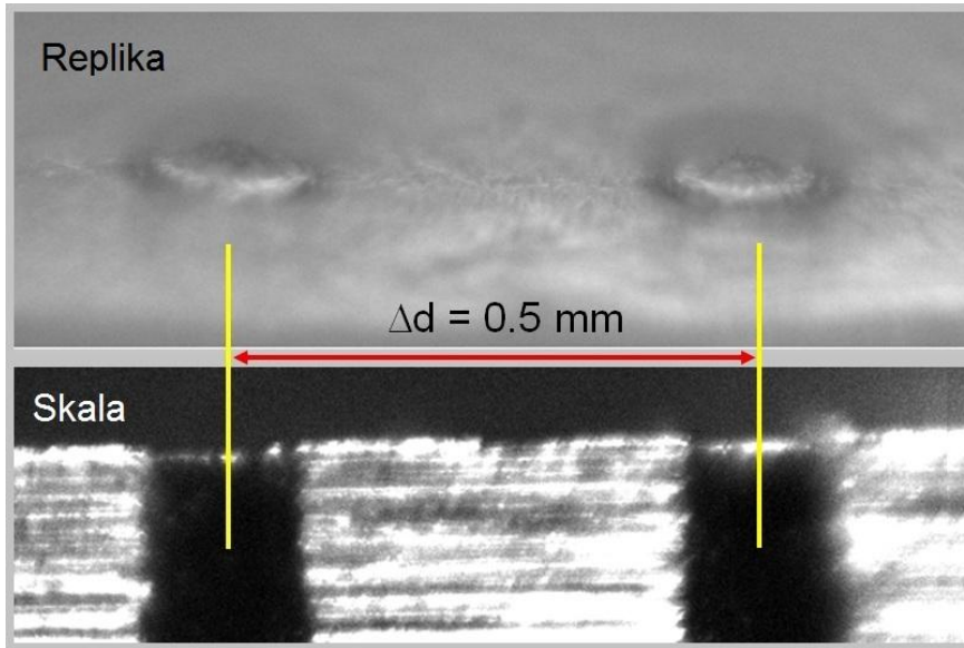
Şekil 6.9 : Replika üzerinde mesafe ölçümü.
