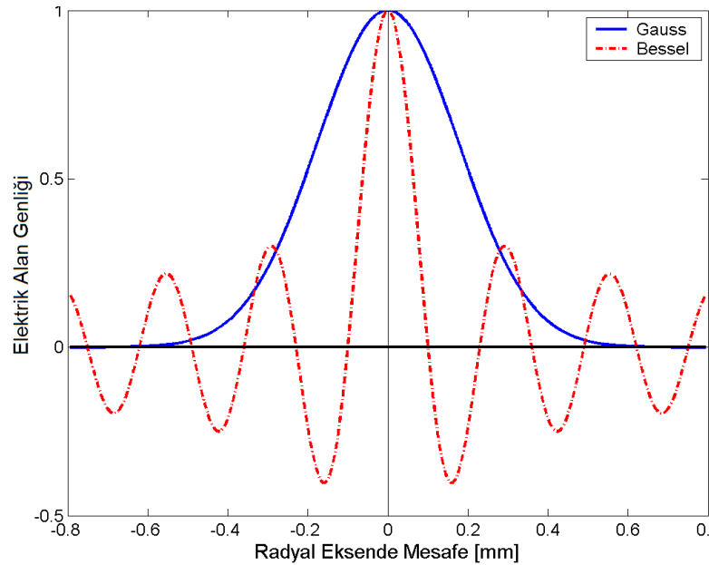
Şekil 4.3 : Gauss ve Bessel huzmelerinin dalga formları.
