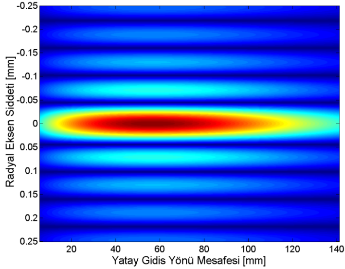
Şekil 4.4 : 1° Konik mercek odaklaması.
