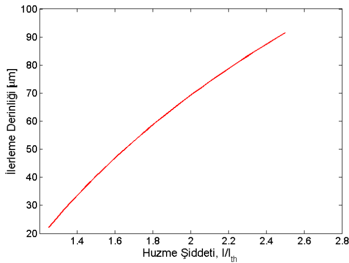
Şekil 7.8 : Bakırda farklı eşik şiddetleri için ilerleme.
