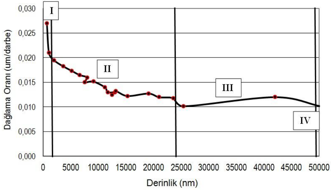
Şekil 6.17 : Alüminyumda dağlama oranının derinliğe göre değişimi.
