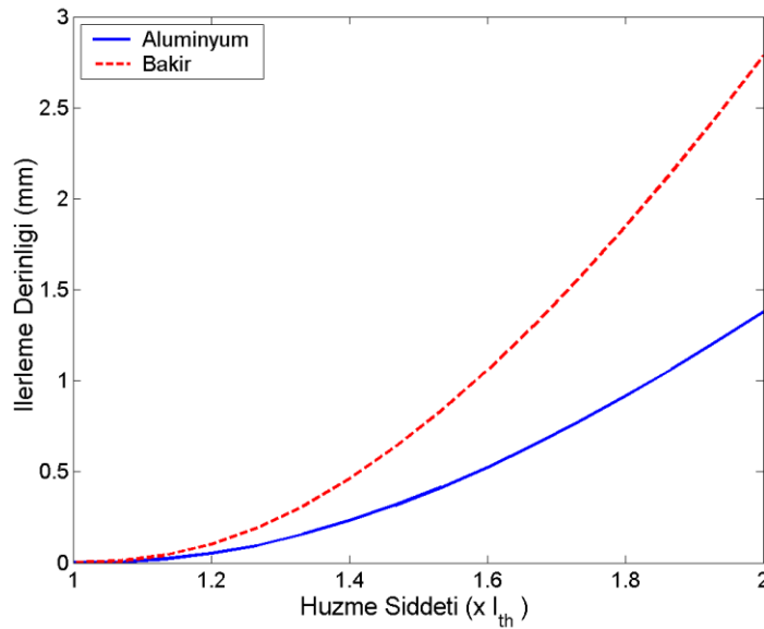
Şekil 5.8 : Aluminyum ve Bakır’da farklı eşik şiddeti katları için ideal ilerleme hesaplamaları.
