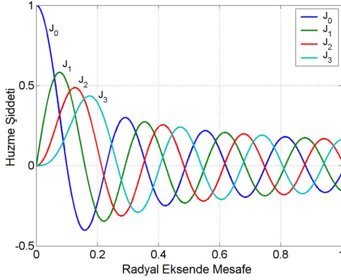
Şekil 3.2 : Birinci tip J_n Bessel fonksiyonları.
