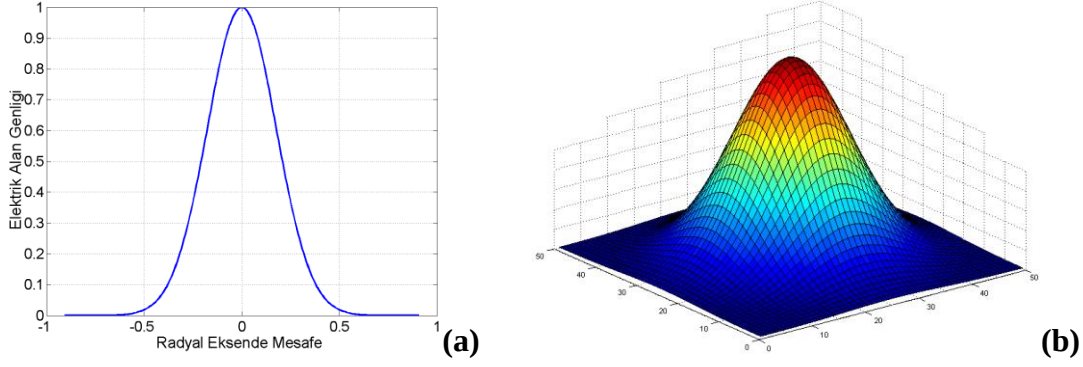
Şekil 4.1 : Gauss fonksiyonu (a) ve üç boyutlu dağılımı (b).
