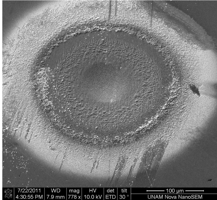
Şekil 6.8 : Silinebilir atomik buhar kümeleri.
