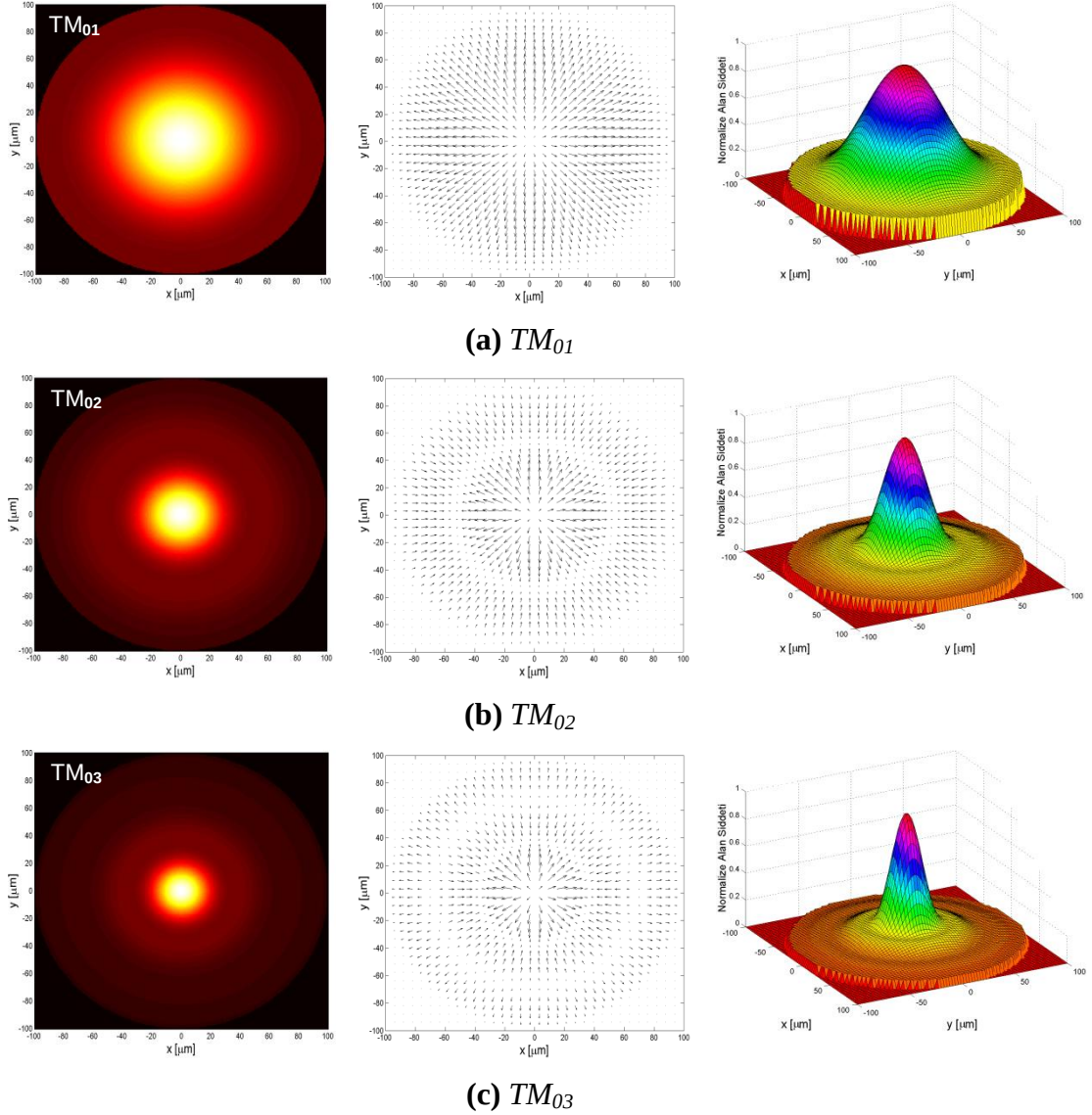
Şekil 3.4 : Bazı TM_{0m} dairesel modları şiddet dağılımları, alan çizgileri ve üç boyutlu şiddet profil gösterimleri.
