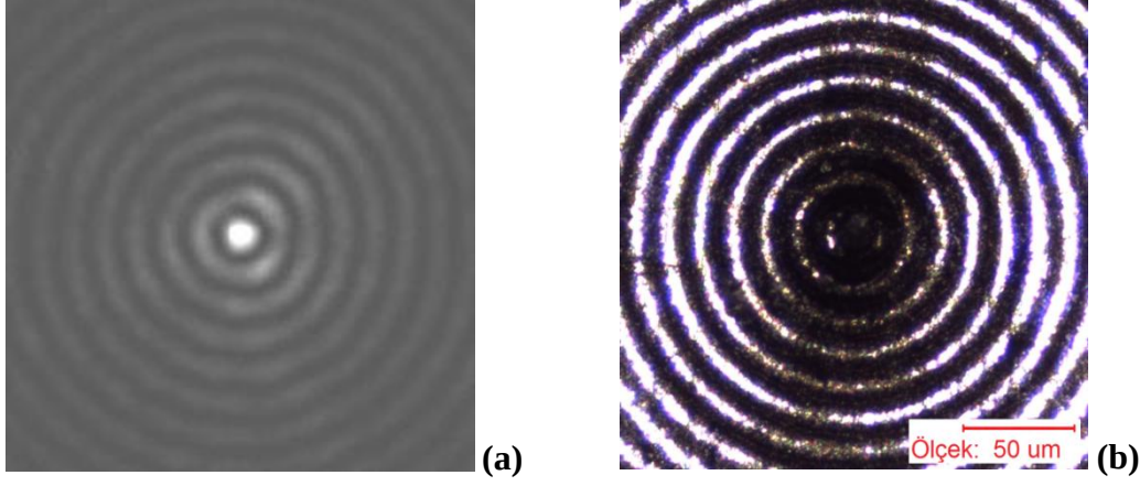
Şekil 4.7 : Bessel huzmesi kesiti ve alüminyumda oluşturduğu dağlama görüntüsü.
