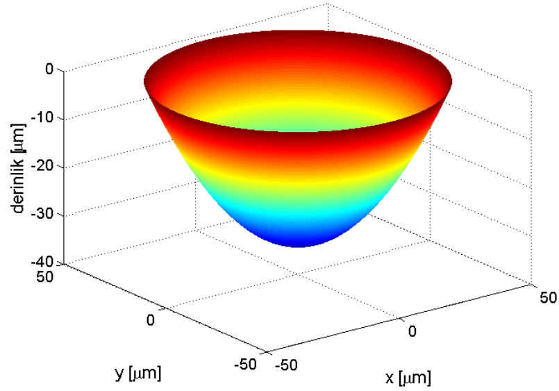
Şekil 7.3 : A=1.4 şiddeti için hesaplanmış üç boyutlu kovuk profili.
