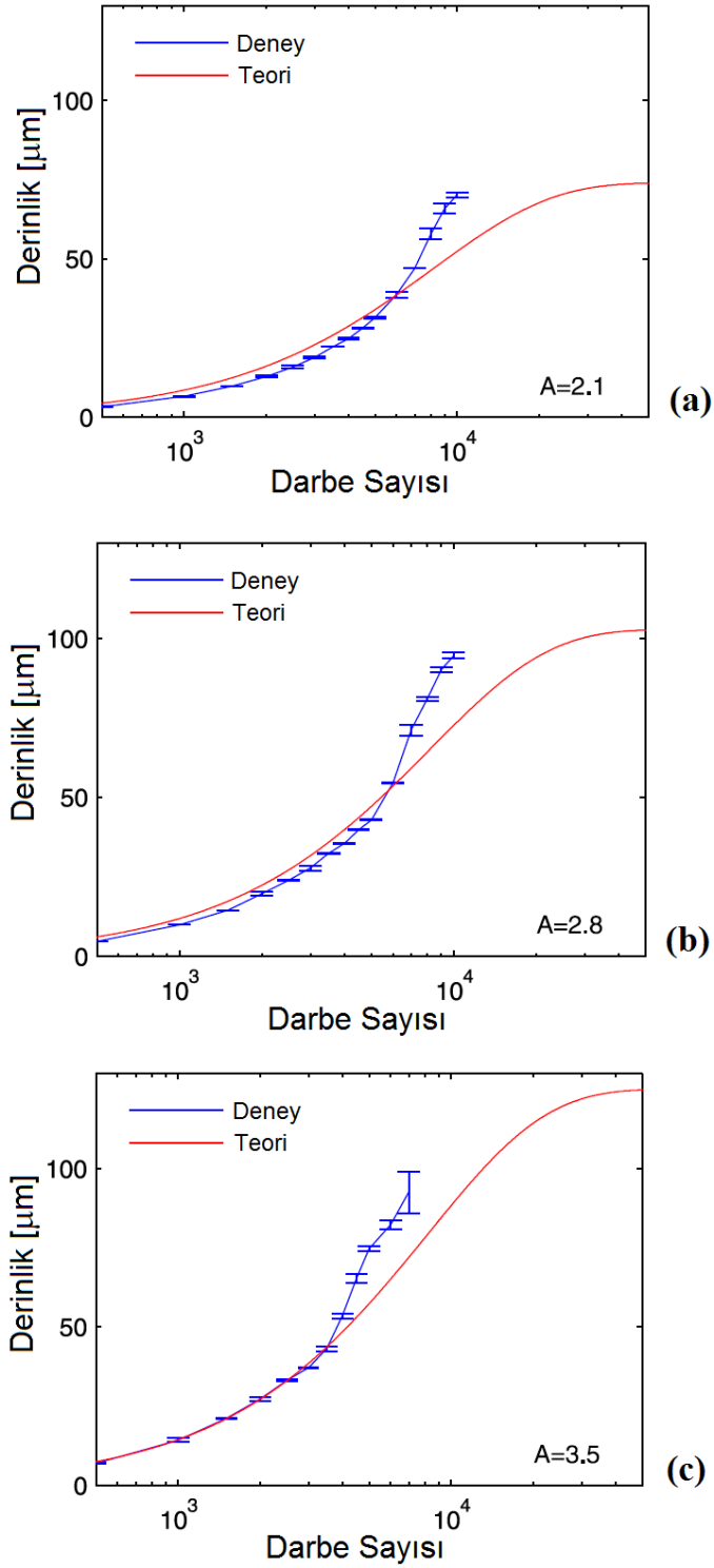
Şekil 7.6 : Kovuk derinliğinin darbe sayısı ile değişimi.
