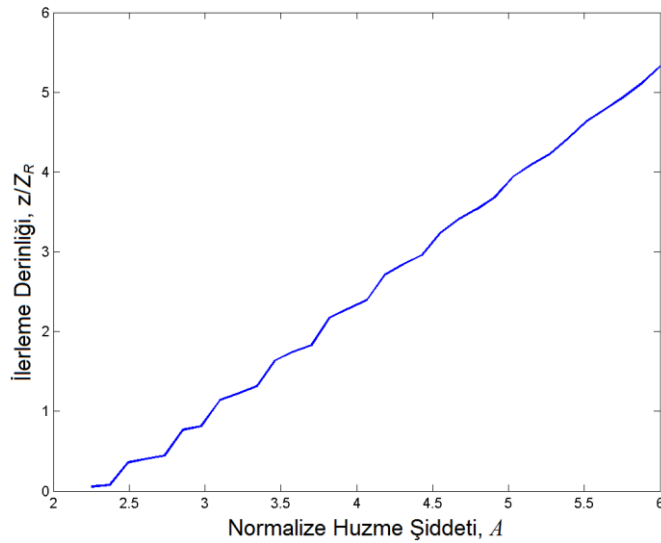
Şekil 5.3 : Bessel huzmelerinin şiddetlerine göre teorik ilerleme mesafesi analizi.
