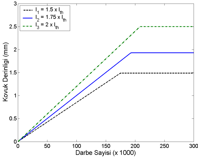
Şekil 5.7 : Alüminyumda darbe sayısının ilerlemeye etkisi.
