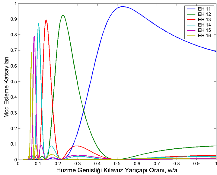
Şekil 3.8 : Bessel tipi huzme için mod-eşleme katsayıları.
