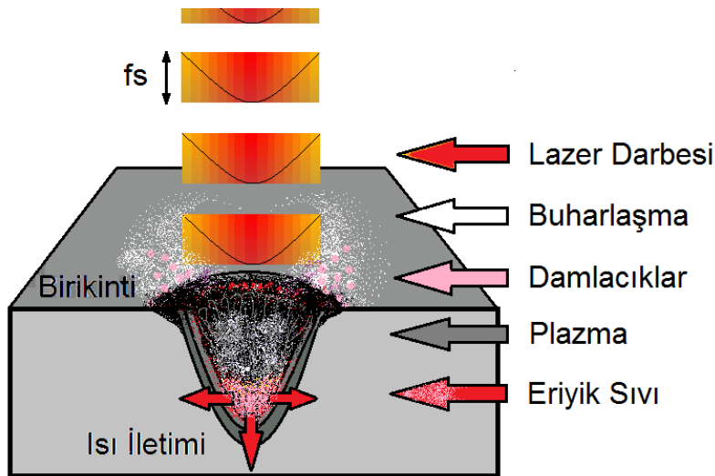
Şekil 2.1 : Daėlamada lazer-metal etkileřimi.
