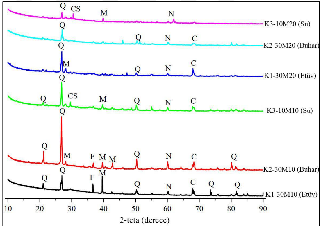
Şekil 4.12 AAHÇ karışımlarının XRD deseni
