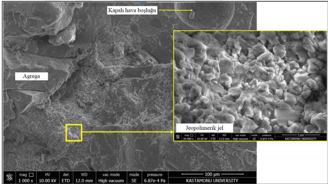
Şekil 4.11 \text{MgSO}_4 saldırısında AAHÇ mikro yapıları
