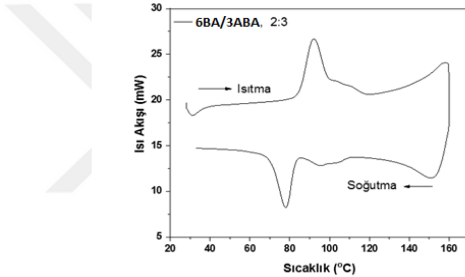
Şekil 4.6: 2:3 oranındaki 6BA/3ABA sıvı kristal karışımının DSC'den elde edilen devamlı ısıtma ve soğutma grafiği
