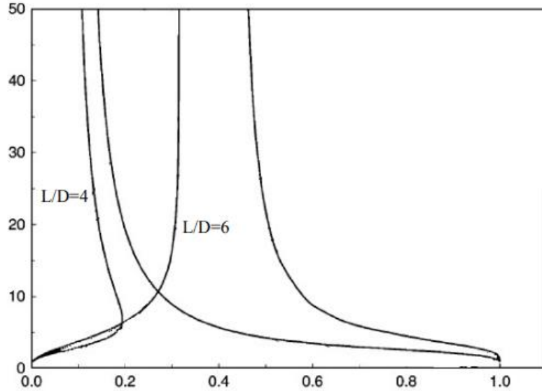
Şekil 1.11: Esnek bir polimer ve "uzun" bir sıvı kristalin karışımlarının faz diyagramları
