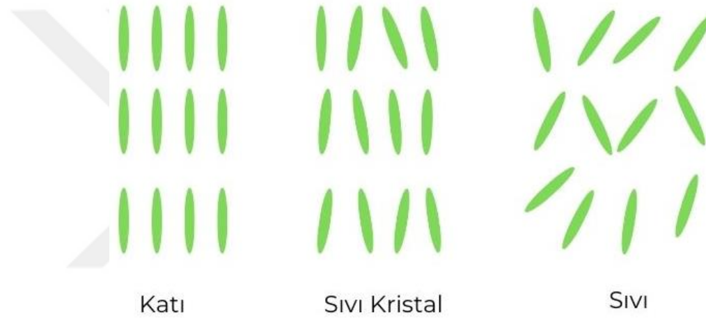
Şekil 1.1: Moleküllerin katı, sıvı ve sıvı kristal fazlarındaki dizilişi
