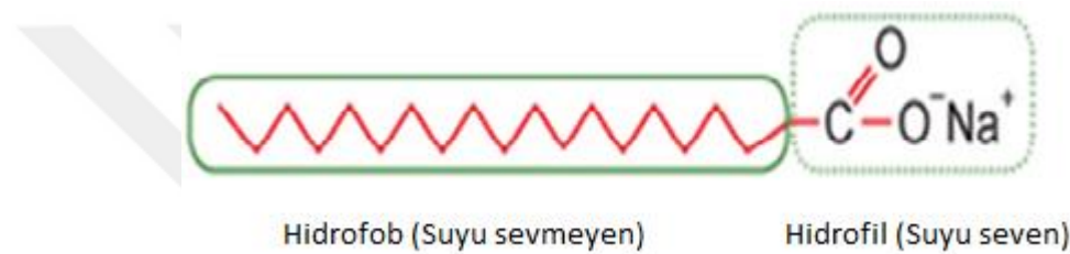
Şekil 1.9: Sabunun kimyasal yapısı
