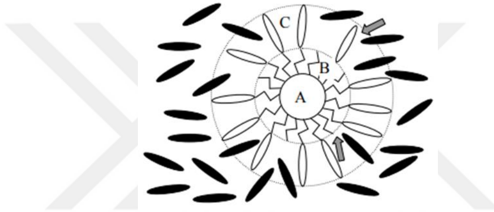
Şekil 1.12: LC varlığında karışık bir ligand tabakası ile kaplanmış bir parçacığın şeması çözücü (siyah elipsoidler).
