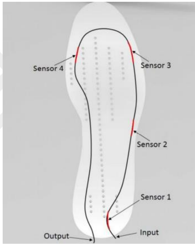
Şekil 2.8: Polimer optik fiber sensörlerinin konumları ile iç tabanın alt kısmı (Leal – Junior ve diğ, 2018).
