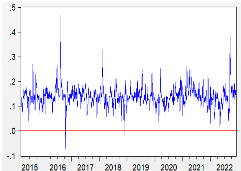
Şekil 4.7: Bitcoin-BİST100 DCC Grafiği
