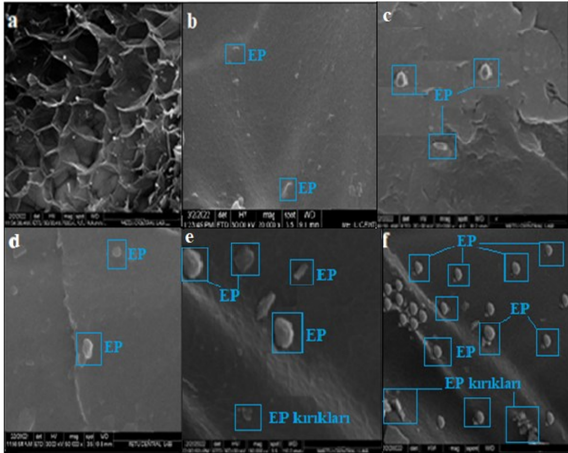
Şekil 4.4. EP takviyeli EPS nanokompozit köpüklerin SEM görüntüleri; (a) EP takviyeli boncukların iç yapısının SEM görüntüsü ( \times 200 \mu\text{m} ), (b ve c) Sırasıyla TPP takviyeli EPS nanokompozitlerin dış yüzeyinin ( \times 5 \mu\text{m} ), (d, e ve f) Sırasıyla %1EP, %3EP ve %5EP takviyeli EPS nanokompozit köpüklerin ( \times 100 \mu\text{m} ) SEM görüntüsü
