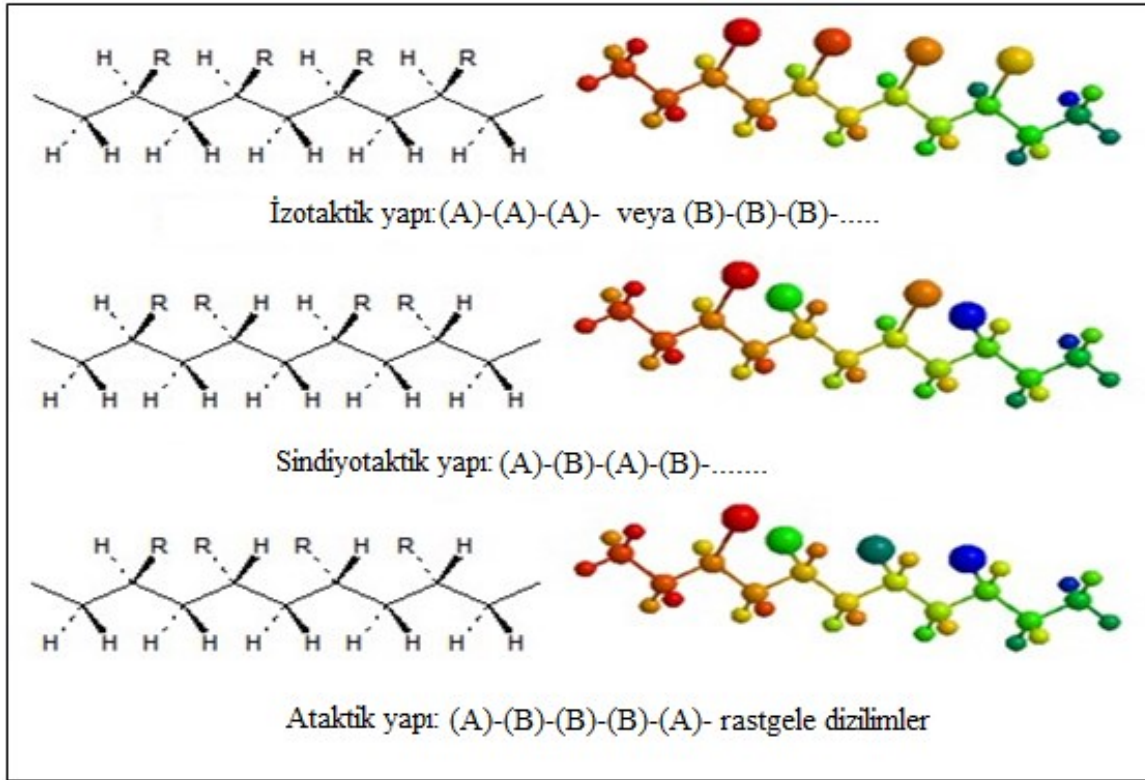
Şekil 2.9. PS'nin kimyasal yapısı
