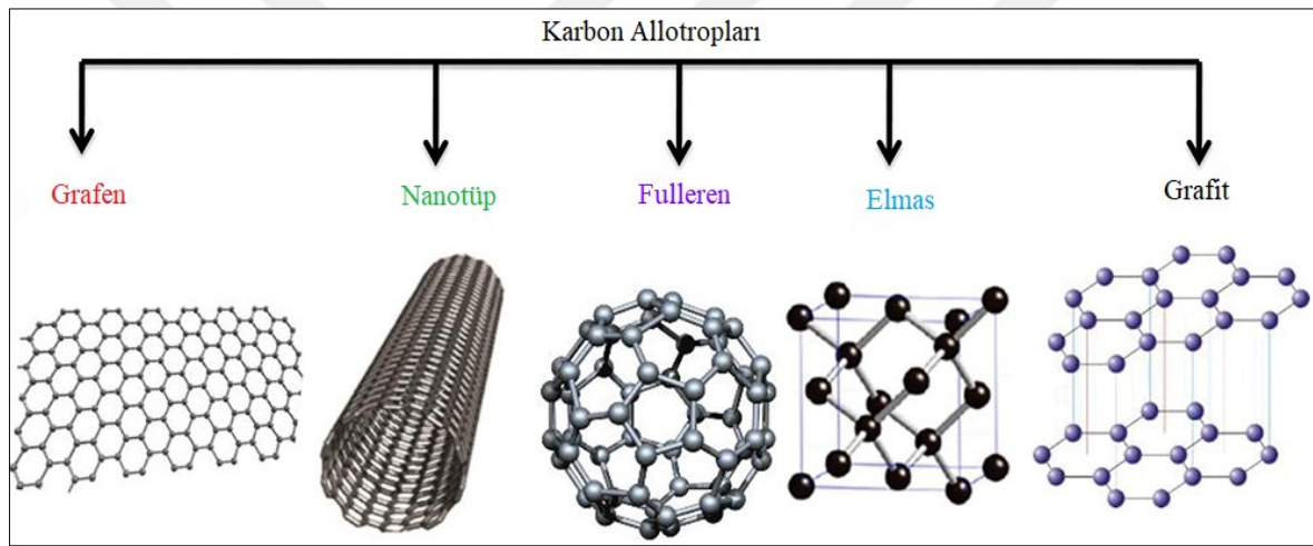
Şekil 2.32. Karbon allotropları [58]
