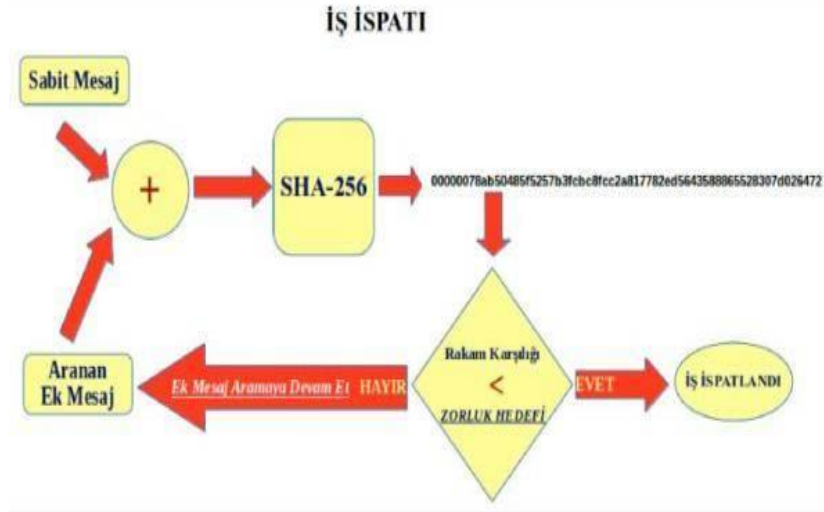
Resim 31. İş İspatı Algoritması. 412
