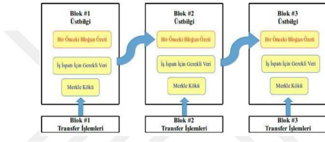
Resim 26. Blok Zinciri Veri Yapısı. 378
