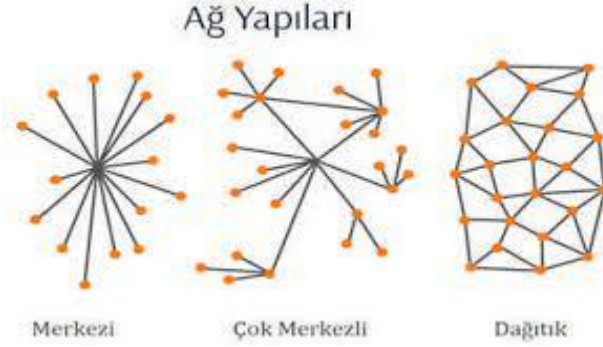
Resim 27. Ağ Yapıları. 381
