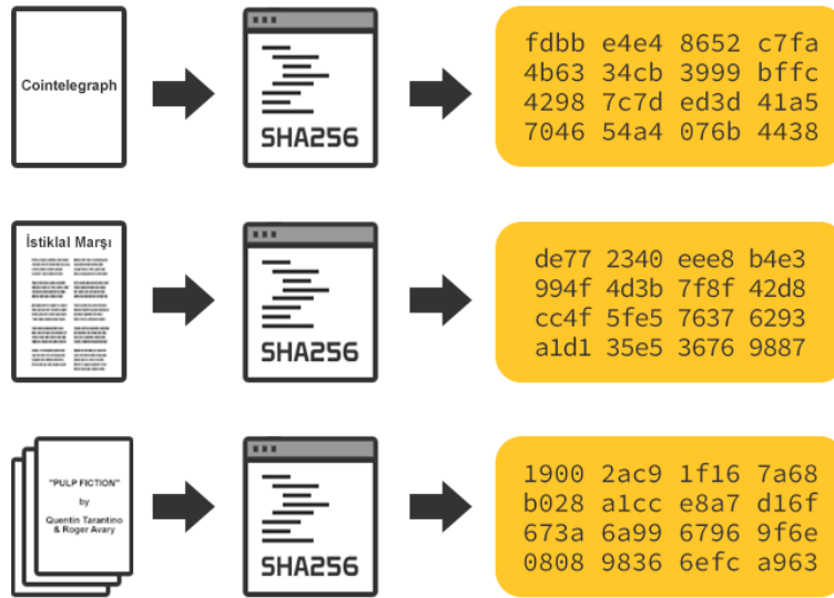
Resim 30. Bitcoin Ağında Kullanılan SHA-256 HASH Algoritması. 408
