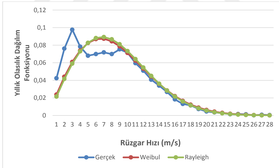
Şekil 7.113. Ural bölgesi 2016 yılı için olasılık dağılım fonksiyonlarının rüzgâr hızı ile değişimi
