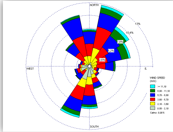
Şekil 7.44. Çeşme istasyonunun 2020 yılı için hakim rüzgar yönü
