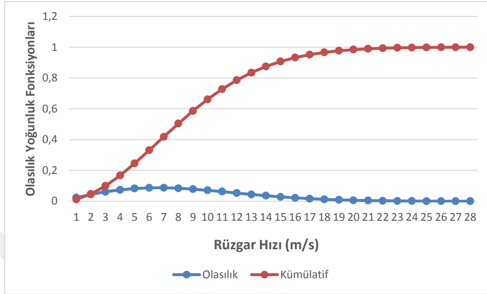
Şekil 7.112. Ural Bölgesi 2016 yılı için olasılık yoğunluk fonksiyonlarının rüzgâr hızı ile değişimi
