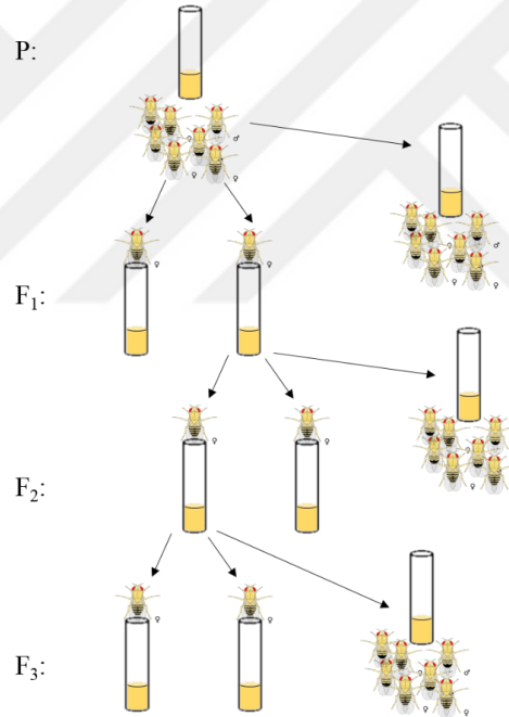
Şekil 3.2. Kardeş eşleşmesi ile tek bir dişisi kullanarak bir sonraki kuşağın kurulması prensibine dayanan "Full-sib" kendileşme yönteminin şematik gösterimi [113].
