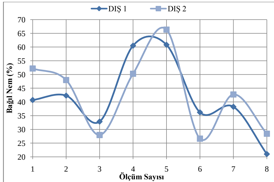
Şekil 4.11. Dış 1 ve Dış 2 için bağıl nem grafiği
