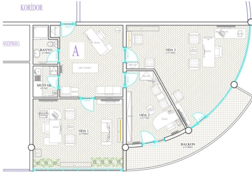
Şekil 4.17. A ofisi plan krokisi
