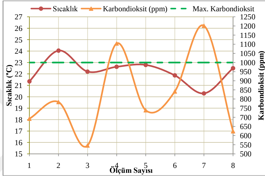
Şekil 4.32. B ofisi için Sıcaklık-CO 2 ilişkisi
