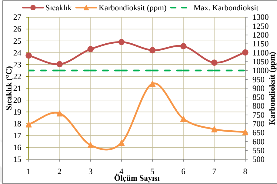
Şekil 4.22. A ofisi için Sıcaklık-CO 2 ilişkisi
