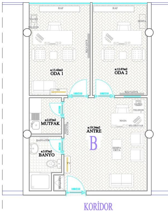
Şekil 4.27. B ofisi plan krokisi
