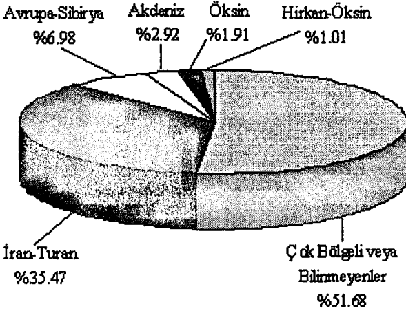
Şekil 4.1. Araştırma alanındaki bitkilerin fitocoğrafik bölge spektrumu.
