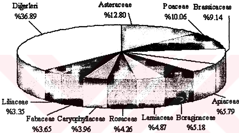
Şekil 4.3. Araştırma alanındaki cinslerin familyalara dağılım spektrumu.
