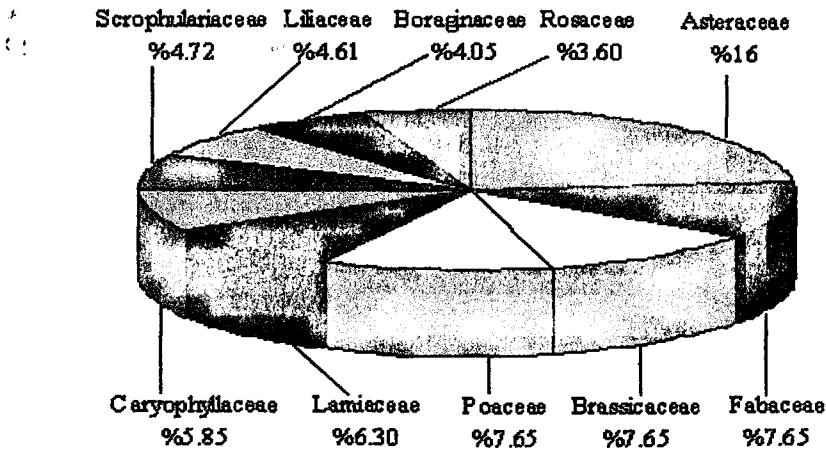
Şekil 4.2. Araştırma alanındaki familyaların spektrumu.
