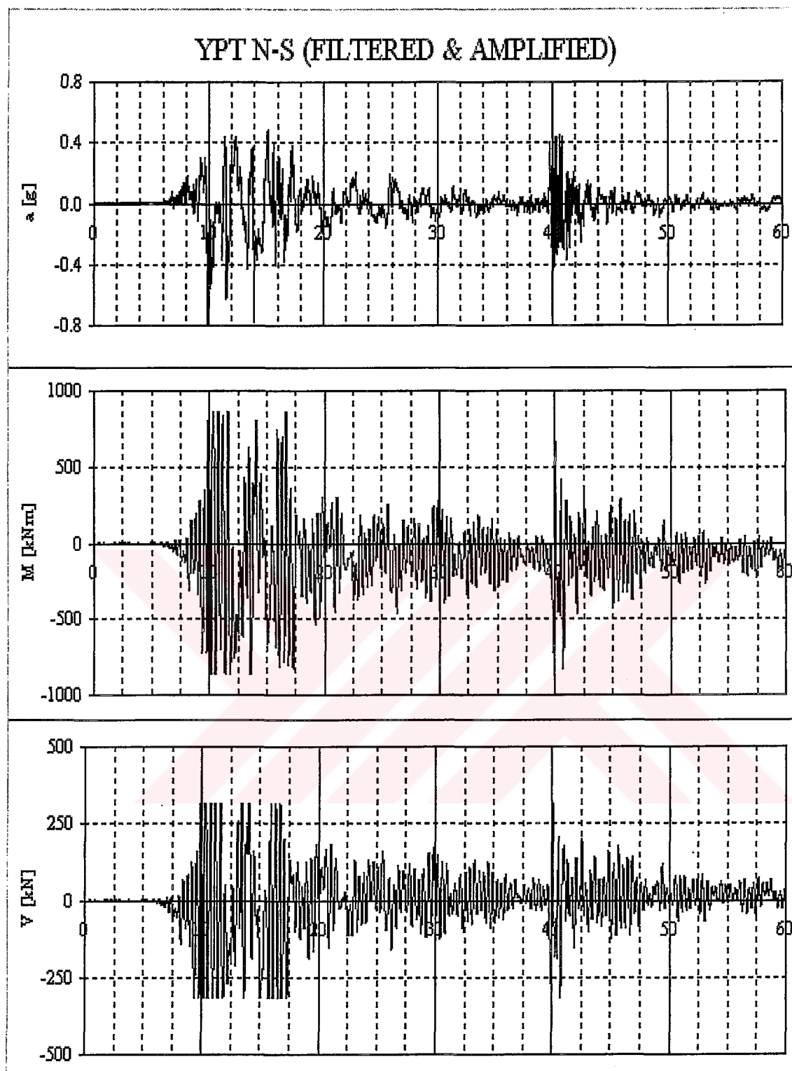
Figure 7-13 (1) YPT N-S (2) M33 (3) V22 (Element ID: 18)
