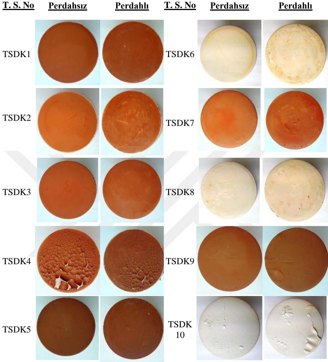
Çizelge 5: Terra Sigillata (T.S.) astarların elektrikli fırında 1000 °C’de pişirim sonuçları
