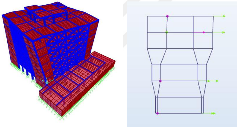
(d) Third mode
