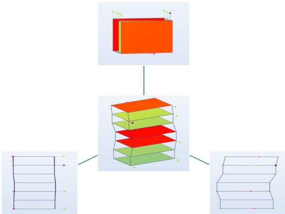
(d) Second translational mode in the NS direction
