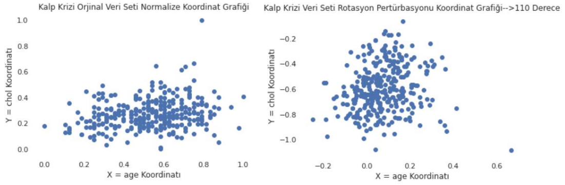
Şekil 5.13. Kalp krizi veri setinin age ve chol değişkenlerinin koordinat düzleminde döndürülmesi.
