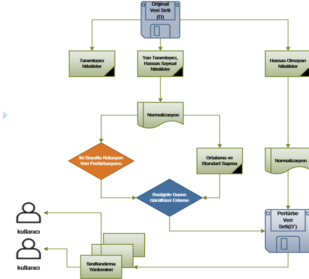
Şekil 5.1. Uygulamanın işlem adımları/temel yapının blok diyagramı.
