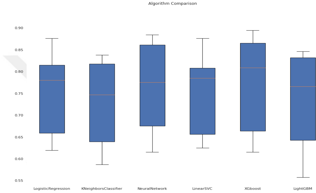
Şekil 5.5. Titanic veri seti sınıflandırma doğruluk sonuçları kutu grafiği.
