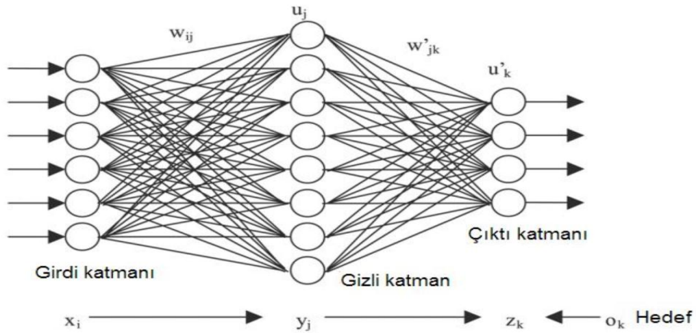
Şekil 4.8. Çok katmanlı yapay sinir ağı örneği.
